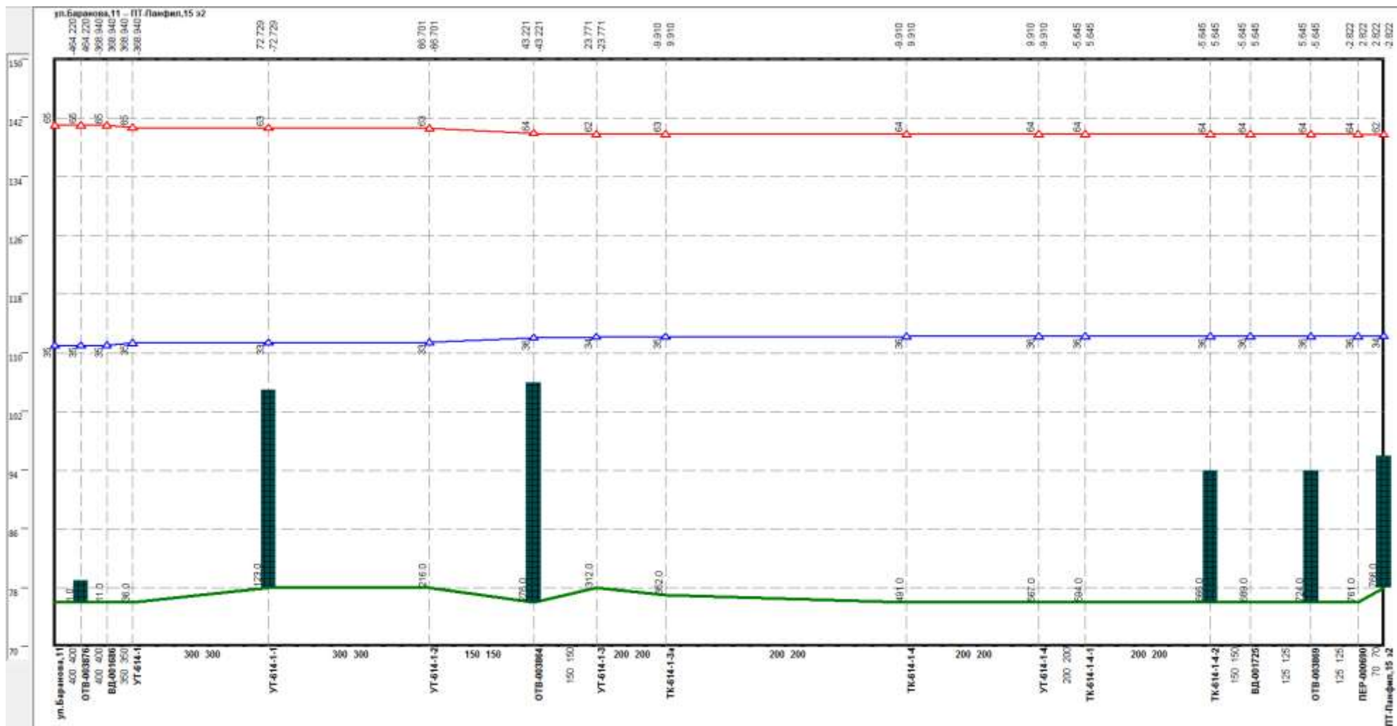
Рисунок 3.28 –Результат гидравлического расчета - график гидравлических режимов по пути теплоносителя от котельной Баранова, 11 до ПТ-Панфила,15 э2
