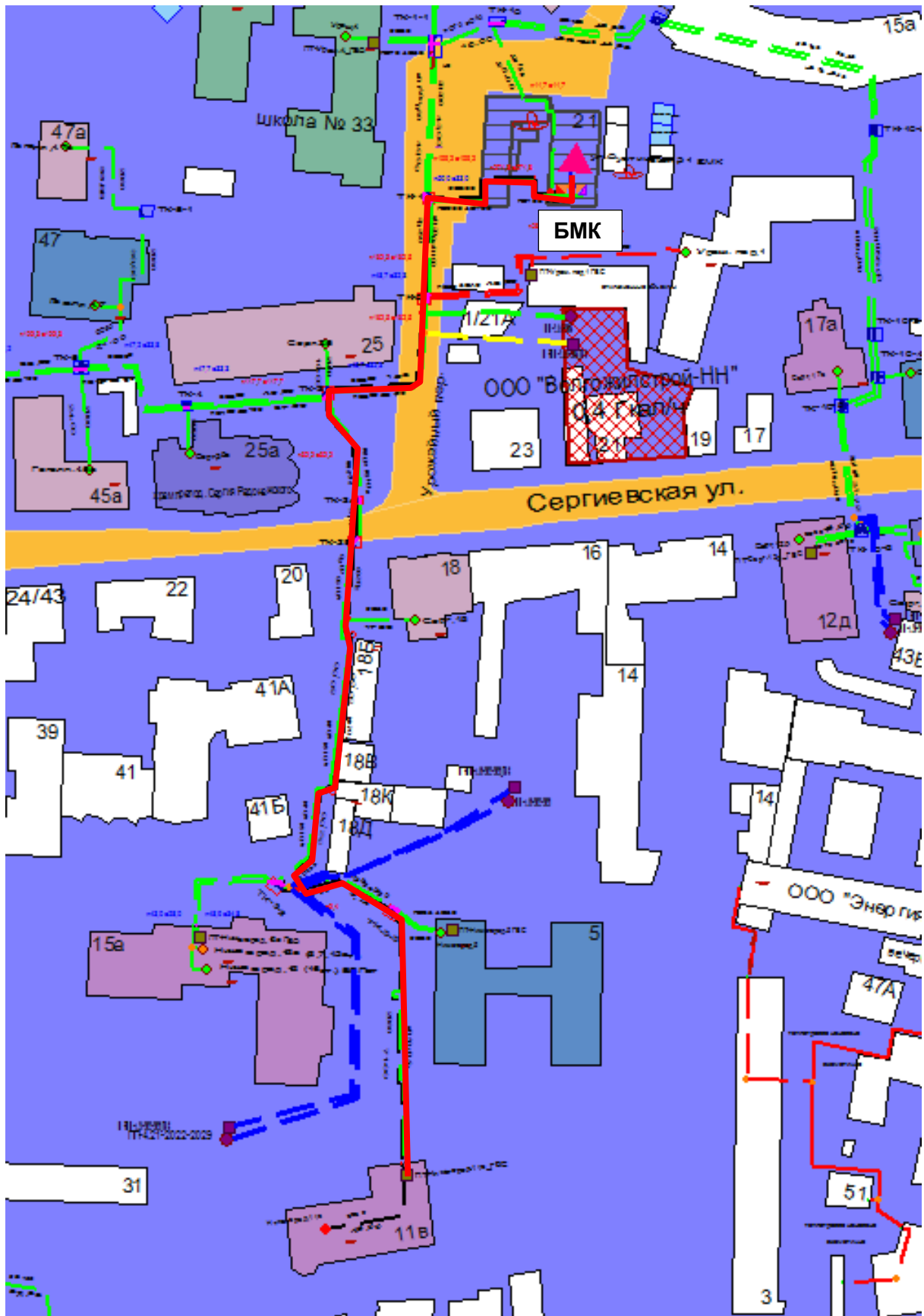
Рисунок 3.9 – Результат гидравлического расчета - расчетный путь теплоносителя от котельной Суетенская, 21 до ПТ-Нижгород, 11в
