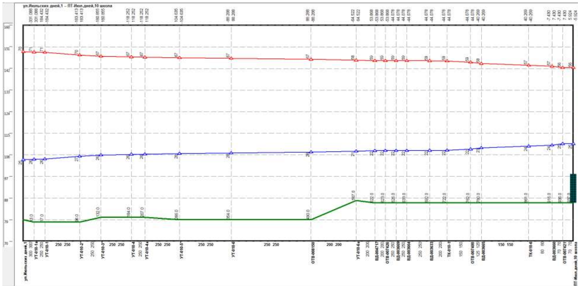
Рисунок 3.22 –Результат гидравлического расчета - график гидравлических режимов по пути теплоносителя от Июльских дней, 1 до ПТ-Июльских дней, 10 школа
