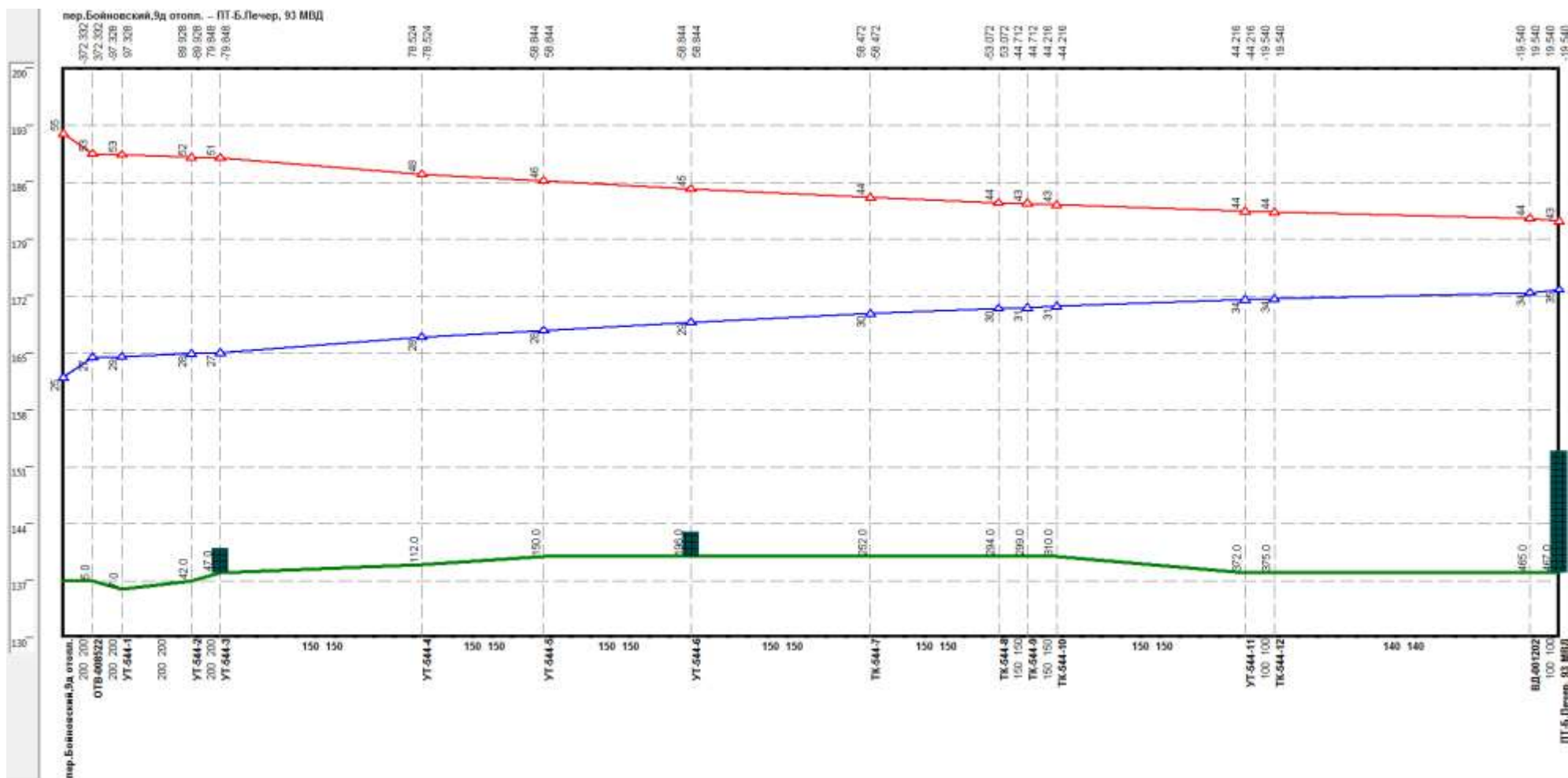
Рисунок 3.14 –Результат гидравлического расчета - график гидравлических режимов по пути теплоносителя от Бойновский, 9д до ПТ-Б.Печер, 93 МВт
