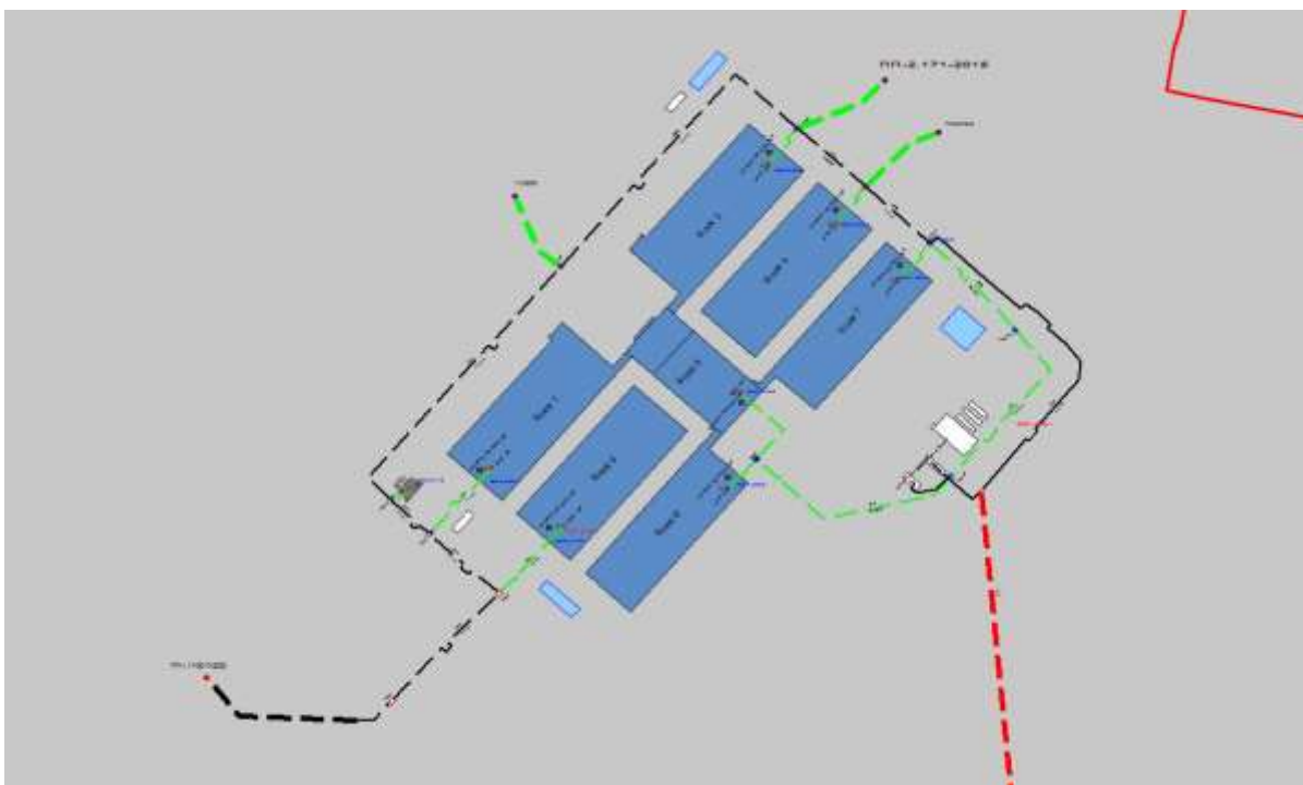
Рисунок 3.55 – Результат гидравлического расчета - расчетный путь теплоносителя от котельной "Сбербанк" БМК №1. до ПТ-ПП-1.17-2017-2022
