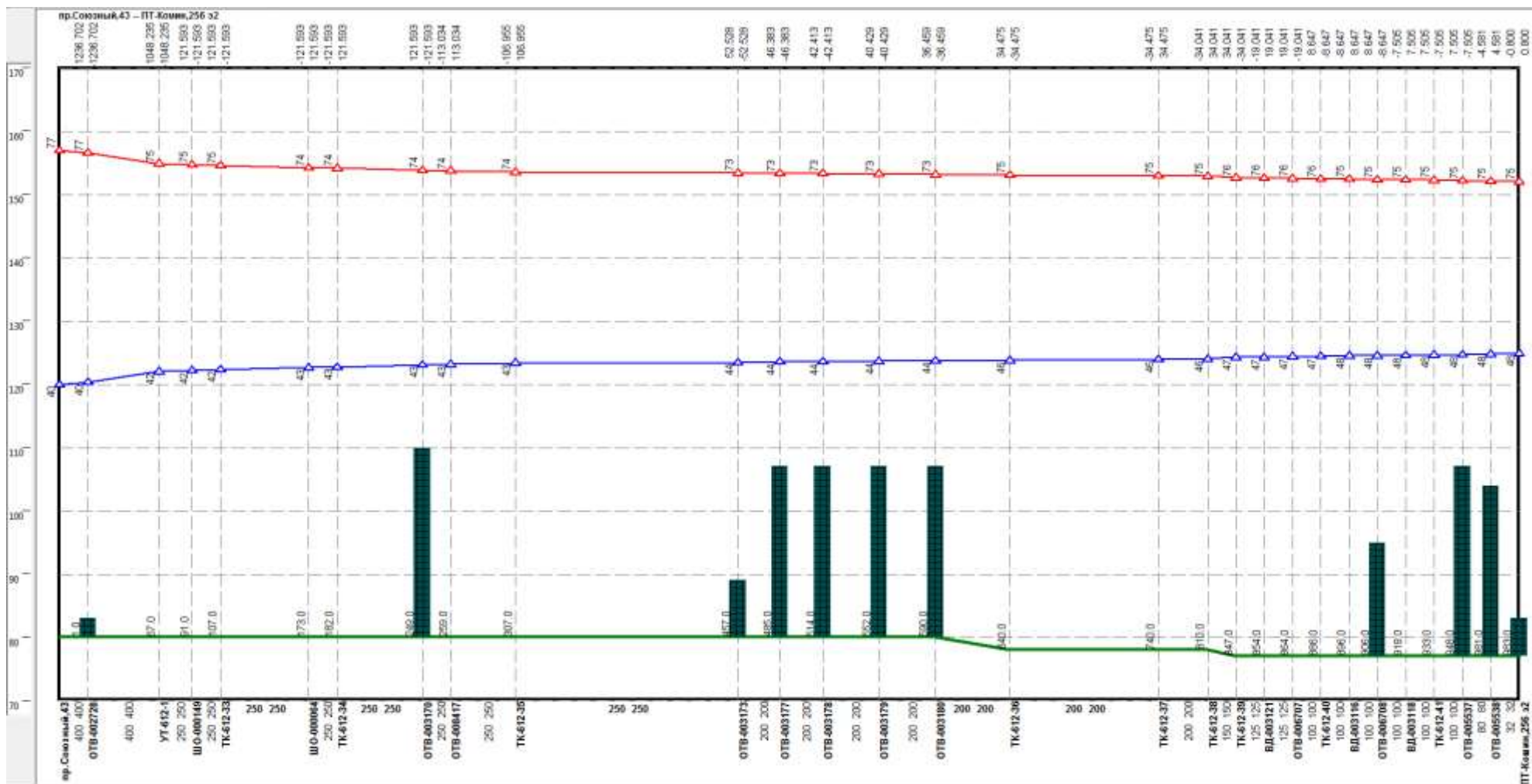
Рисунок 3.50 –Результат гидравлического расчета - график гидравлических режимов по пути теплоносителя от котельной пр. Союзный, 43 до ПТ-Комин,256 э2
