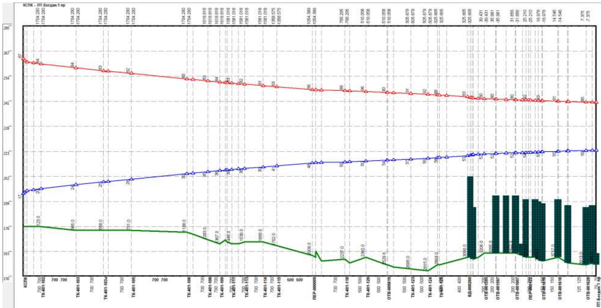
Рисунок 3.54 Результат гидравлического расчета - график гидравлических режимов по пути теплоносителя от котельной ул. Родионова, 1946 до ПТ-Богдан.1 пр
