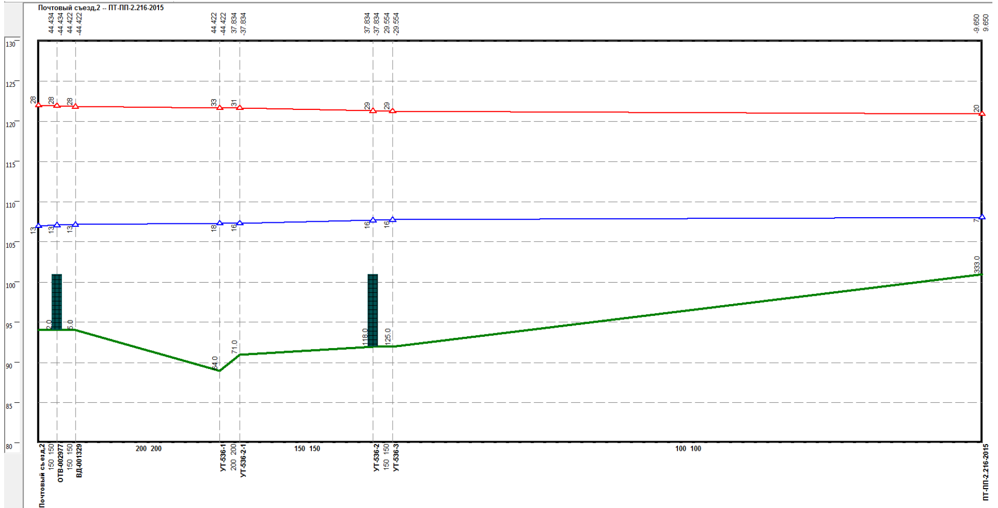
Рисунок Ошибка! Текст указанного стиля в документе отсутствует.67 –Результат гидравлического расчета - график гидравлических режимов по пути теплоносителя от котельной Почтовый съезд, 2, 24 до ПТ-ПП-2.216-2015
