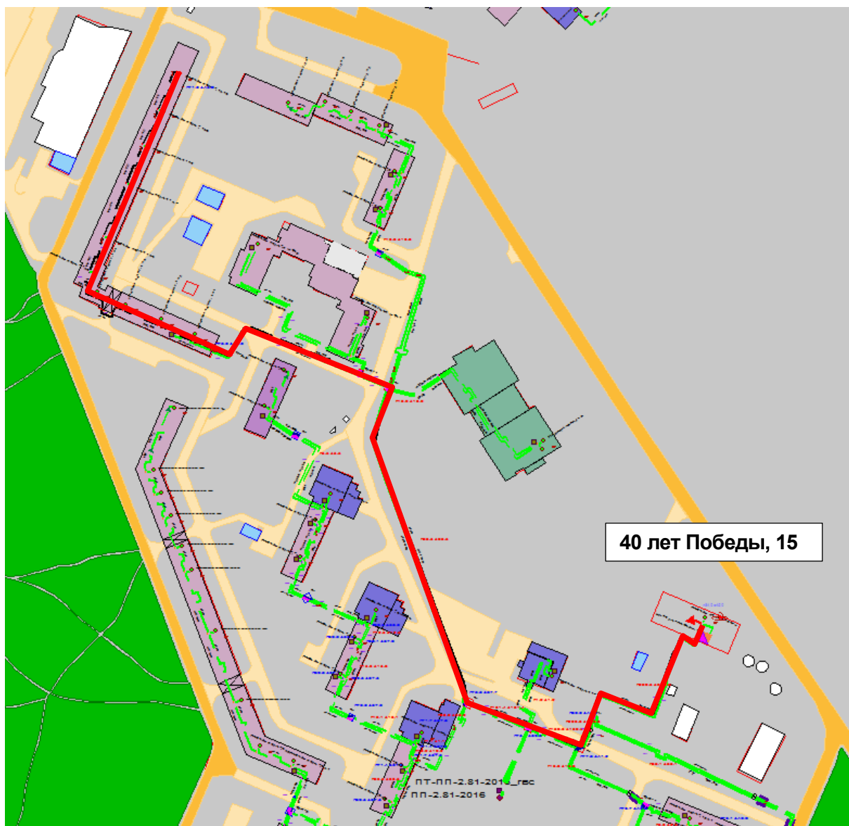
Рисунок Ошибка! Текст указанного стиля в документе отсутствует..62 – Результат гидравлического расчета - расчетный путь теплоносителя от котельной 40 лет Победы, д.15 до ПТ-Победы 40лет,1 э10
