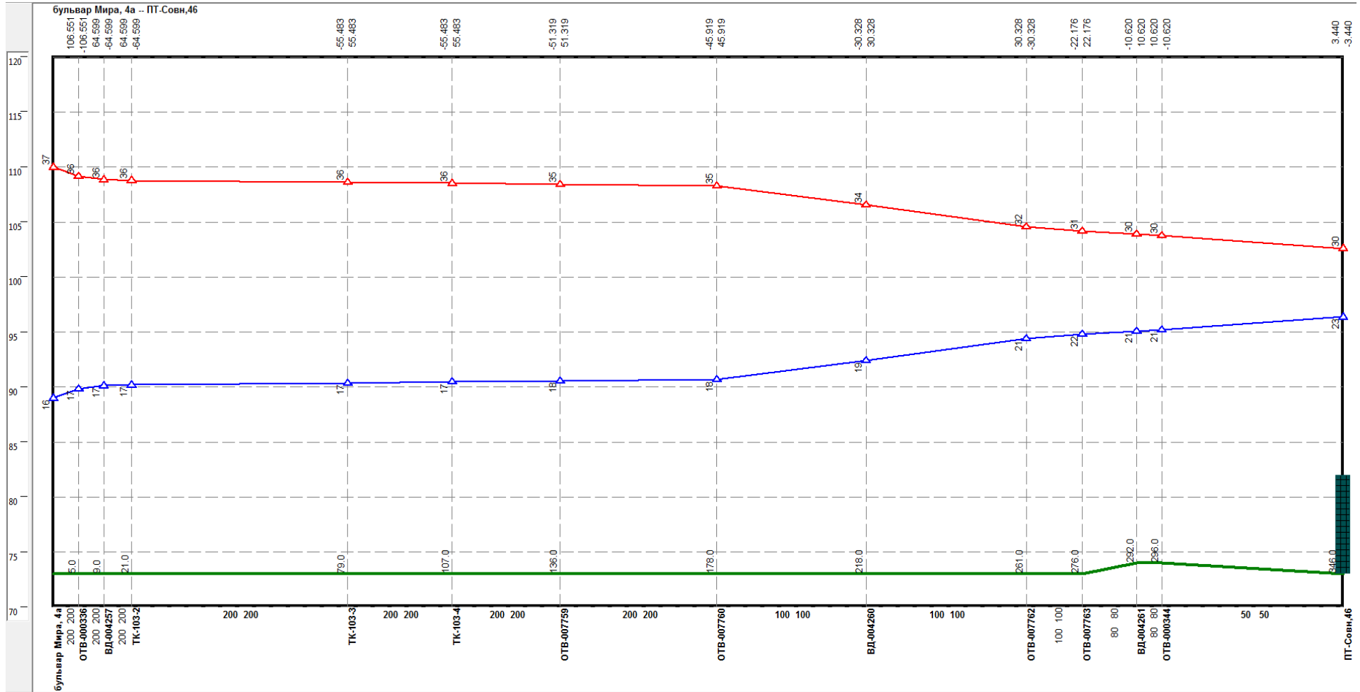
Рисунок Ошибка! Текст указанного стиля в документе отсутствует..31 –Результат гидравлического расчета - график гидравлических режимов по пути теплоносителя от котельной Бульвар Мира, 4-а до ПТ-Совн,46
