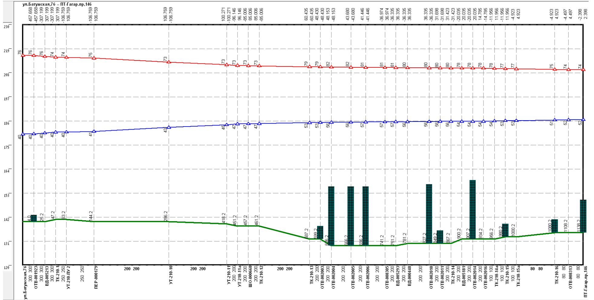
Рисунок Ошибка! Текст указанного стиля в документе отсутствует...15 –Результат гидравлического расчета - график гидравлических режимов по пути теплоносителя от котельной Батумская, 76 до ПТ-Гагар.пр,146
