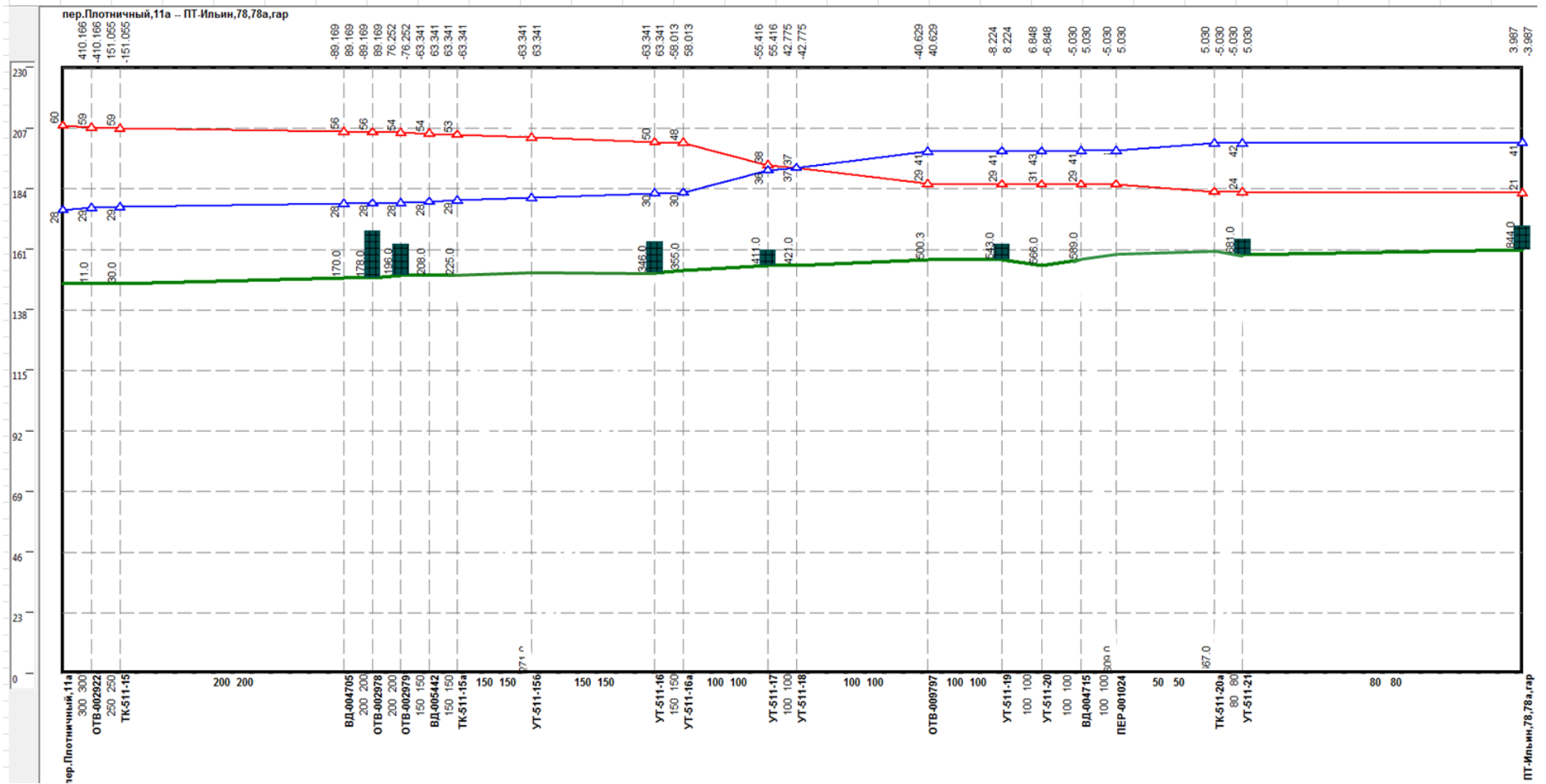
Рисунок 4.3 – Результат гидравлического расчета - график гидравлических режимов по пути теплоносителя от котельной пер. Плотничный, 11 до ПТ-Ильин,78,78а,гар
