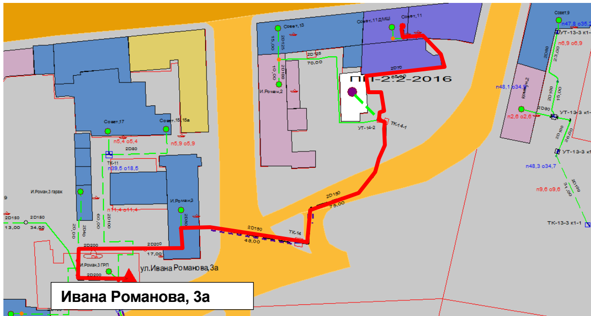
Рисунок 1.144 - Результат гидравлического расчета - расчетный путь теплоносителя от котельной Ивана Романова до ПТ-Совет,11 Основные характеристики теплопровода и режимные параметры теплоносителя приведены в таблице 1.113.
