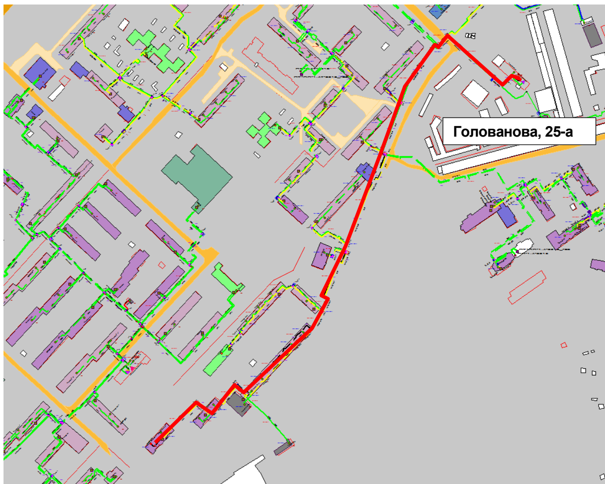
Рисунок Ошибка! Текст указанного стиля в документе отсутствует..78 – Результат гидравлического расчета - расчетный путь теплоносителя от котельной Голованова, 25-а до ПТ-Голован,57 э2
