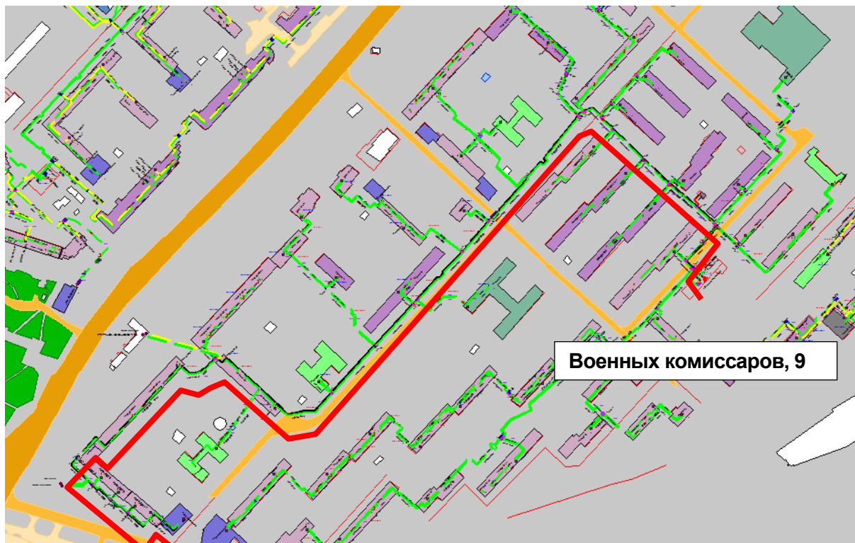
Рисунок Ошибка! Текст указанного стиля в документе отсутствует..64 – Результат гидравлического расчета - расчетный путь теплоносителя от котельной Военных комиссаров, 9 до ПТ-Гагар.пр,226 пристр
