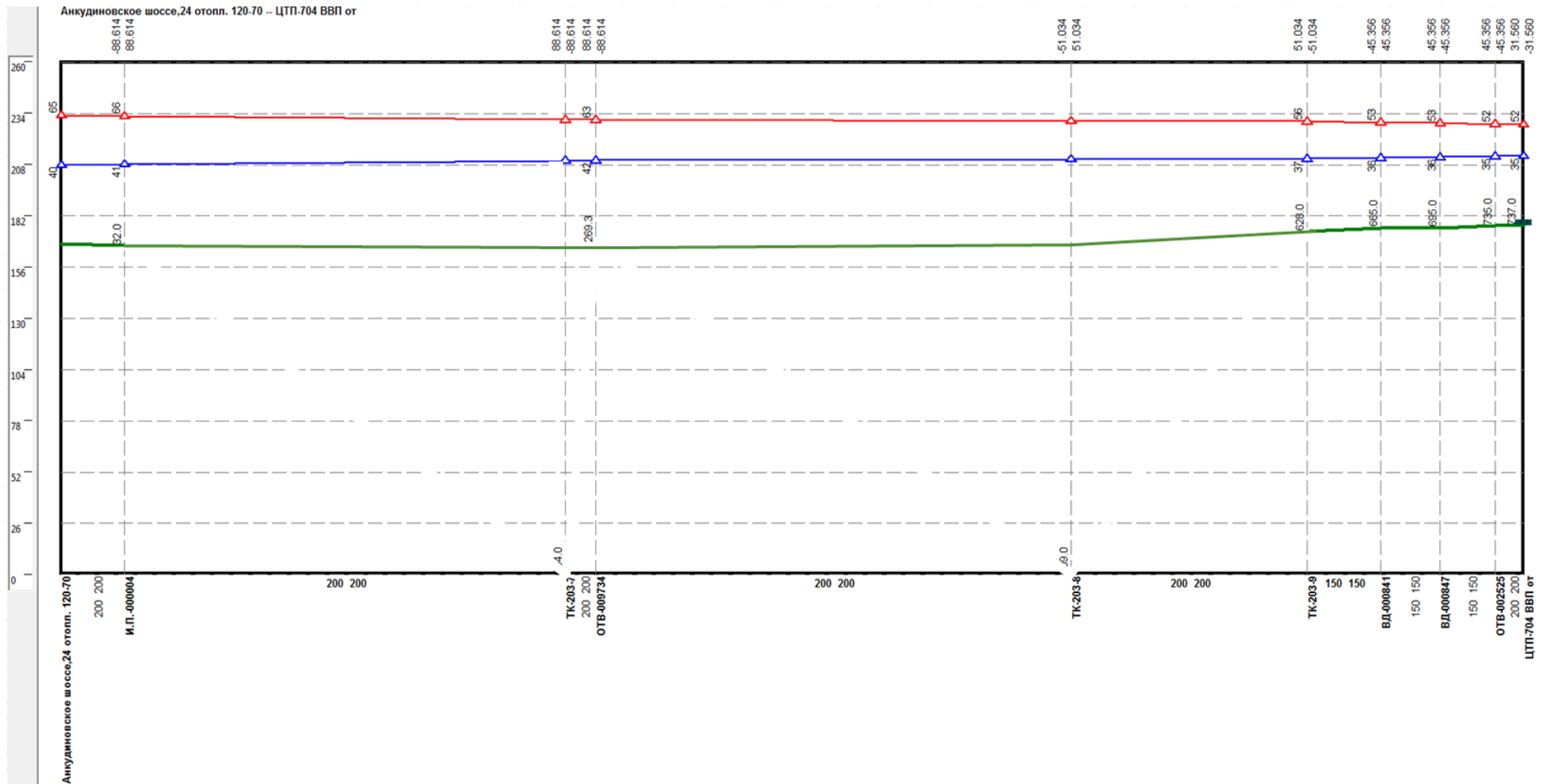
Рисунок 55 – Результат гидравлического расчета - график гидравлических режимов по пути теплоносителя от котельной Анкудиновское шоссе, 24 до ЦТП-704 ВВП от
