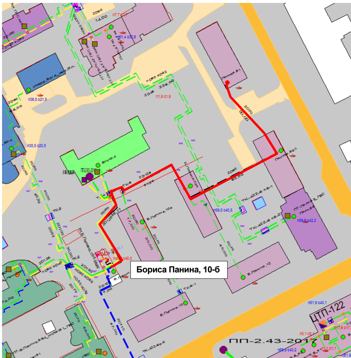
Рисунок Ошибка! Текст указанного стиля в документе отсутствует..36 – Результат гидравлического расчета - расчетный путь теплоносителя от котельной Бориса Панина, 10-6 до ПТ-Полтава,51
