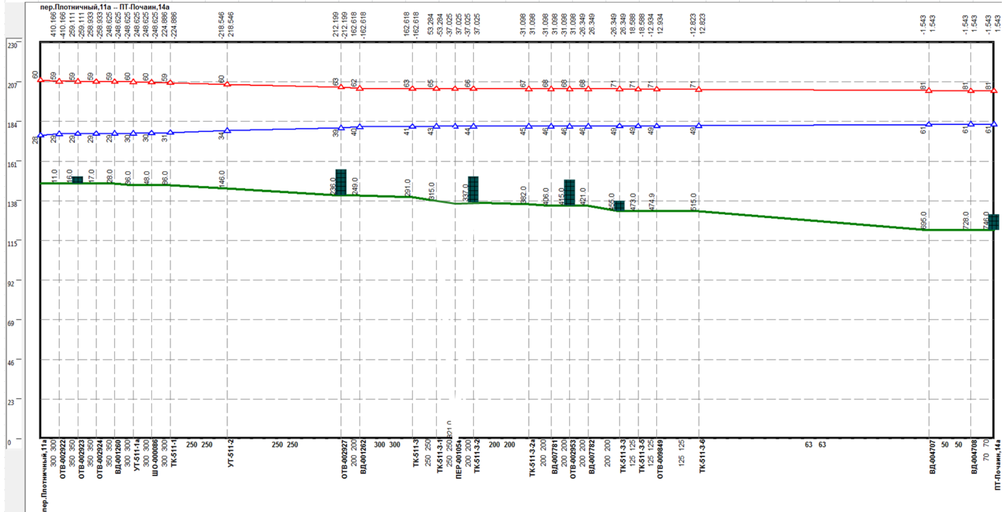
Рисунок Ошибка! Текст указанного стиля в документе отсутствует..47 –Результат гидравлического расчета - график гидравлических режимов по пути теплоносителя от котельной пер. Плотничный, 11а до ПТ-Почаин, 14а
