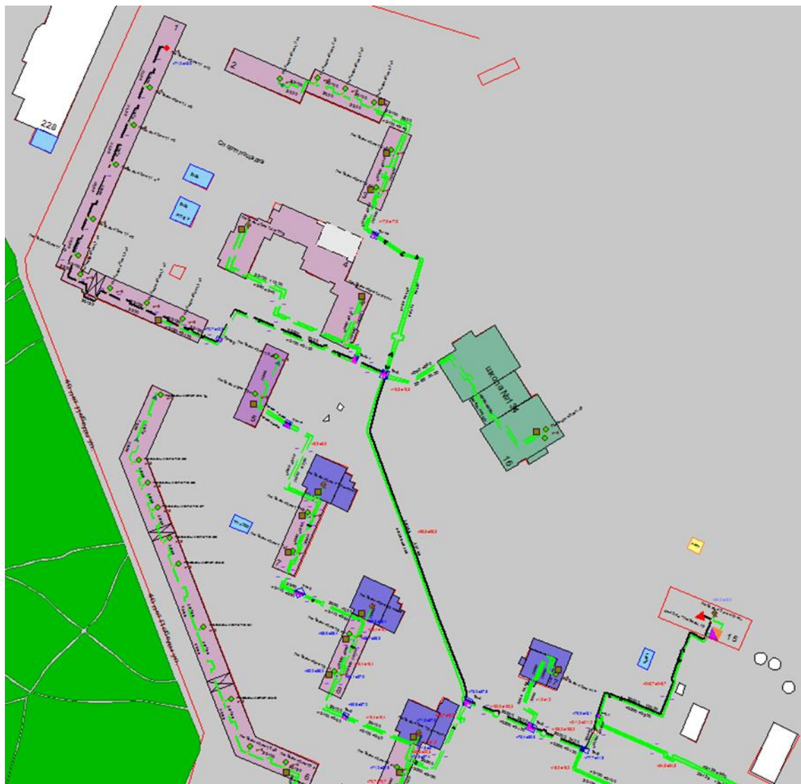
Рисунок Ошибка! Текст указанного стиля в документе отсутствует..43 Результат гидравлического расчета - расчетный путь теплоносителя от котельной 40 лет Победы, 15 до ПТ-Победы 40лет,1 э10
