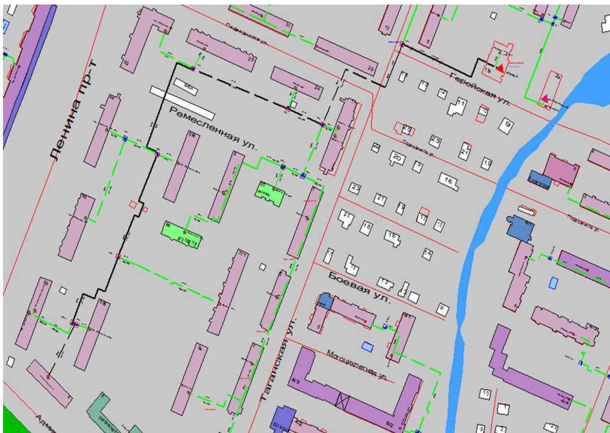
Рисунок Ошибка! Текст указанного стиля в документе отсутствует..11 Результат гидравлического расчета -
