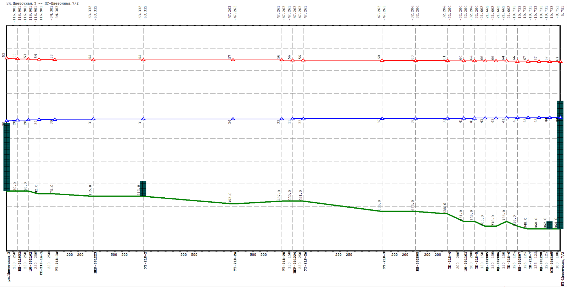
Рисунок Ошибка! Текст указанного стиля в документе отсутствует..48 Результат гидравлического расчета - график гидравлических режимов по пути теплоносителя от котельной Цветочная, 3-а до ПТ-Цветочная,7/2
