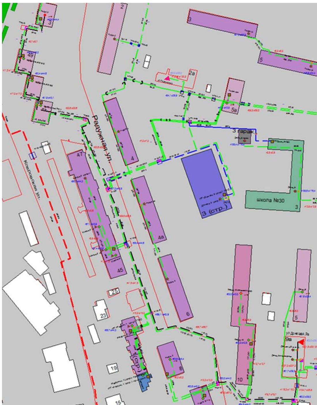
Рисунок Ошибка! Текст указанного стиля в документе отсутствует..89 – Трассировка теплопровода от котельной АО «Теплоэнерго» по ул. Донецкая, д. 9В до конечного потребителя «ПТ-Радуж,3»
