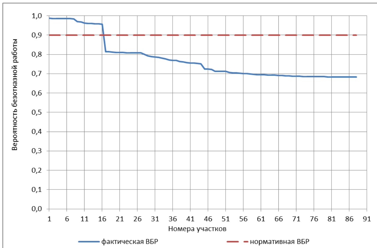
Рисунок 3.23 – ВБР относительно ТК конечного потребителя «ПТ-Малин, 2 пристрой» тепловодов зоны котельной АО «Теплоэнерго» «Нагорная теплоцентраль» (НТЦ) по ул. Ветеринарная, д.5 (расчетный путь 4-1) к 2030 году без проведения мероприятий по реконструкции участков тепловой сети
