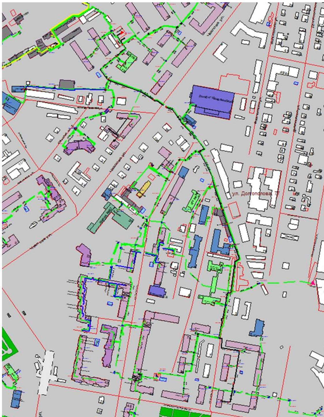
Рисунок 3.106 – Трассировка теплопровода от котельной АО «Теплоэнерго» по ул. Чкалова, д. 9Г до конечного потребителя «ПТ-Вольск,8»
