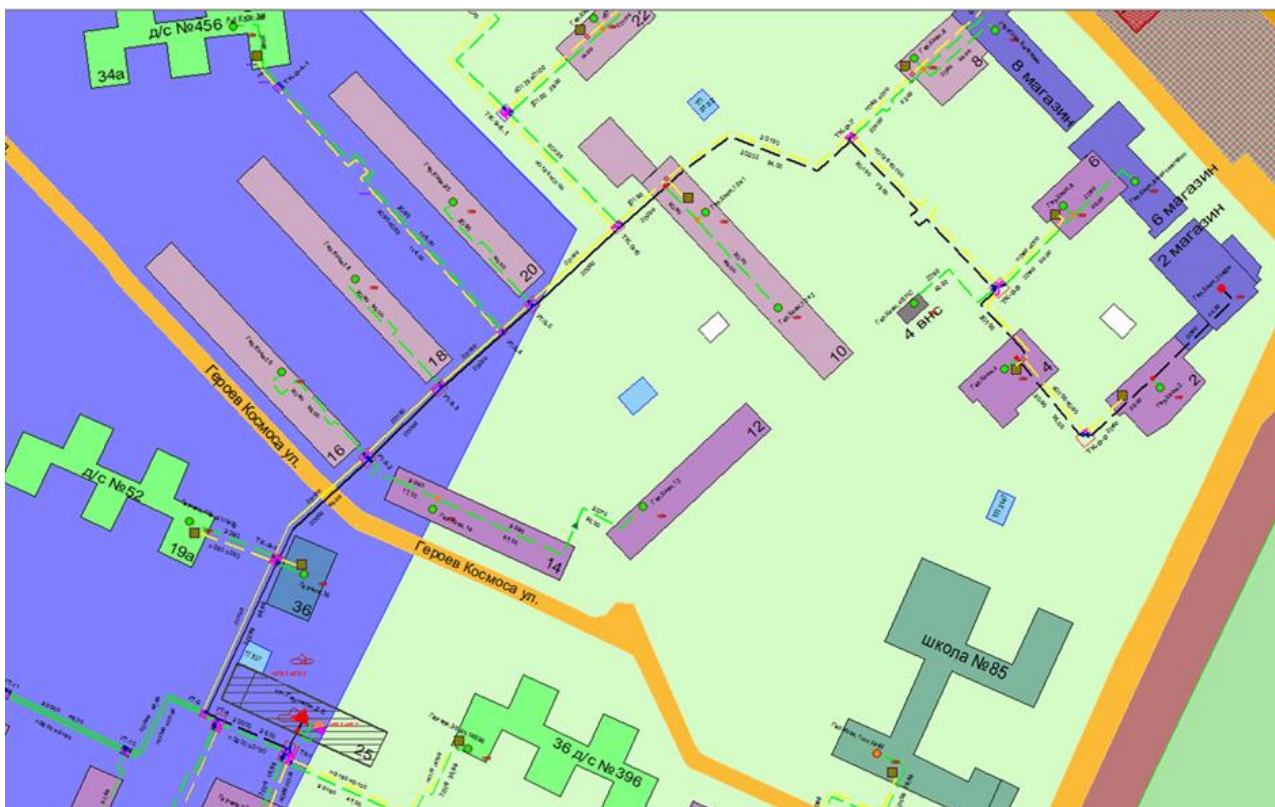
Рисунок 3.86 – Трассировка теплопровода от котельной АО «Теплоэнерго» «7 МР Сормово №2» по ул. Гаугеля, д. 25 до конечного потребителя «ПТ-Гер.Косм,2 кафе»
