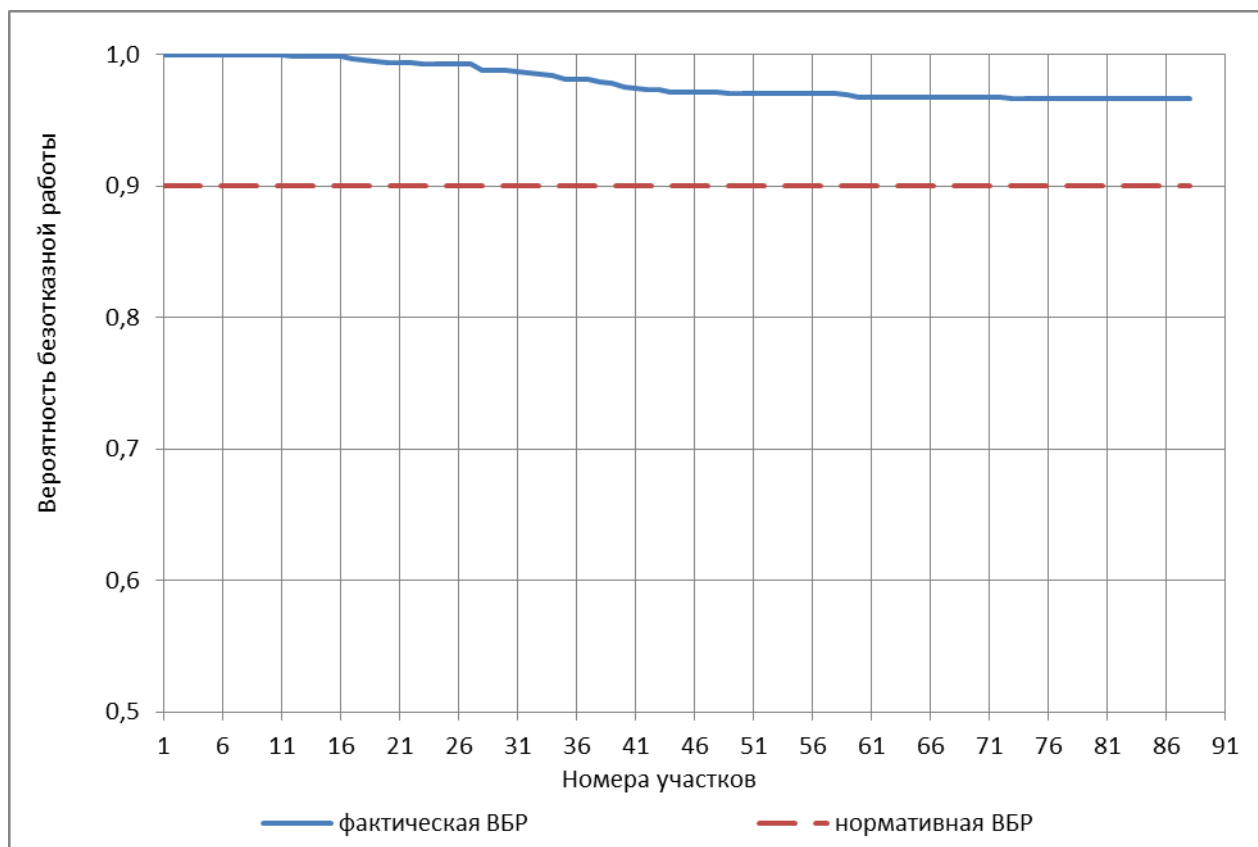
Рисунок 3.24 – ВБР относительно ТК конечного потребителя «ПТ-Малин, 2 пристрой» тепловодов зоны котельной АО «Теплоэнерго» «Нагорная теплоцентраль» (НТЦ) по ул. Ветеринарная, д.5 (расчетный путь 4-1) при поэтапной реконструкции участков тепловой сети, осуществляемой за период до 2030 года
