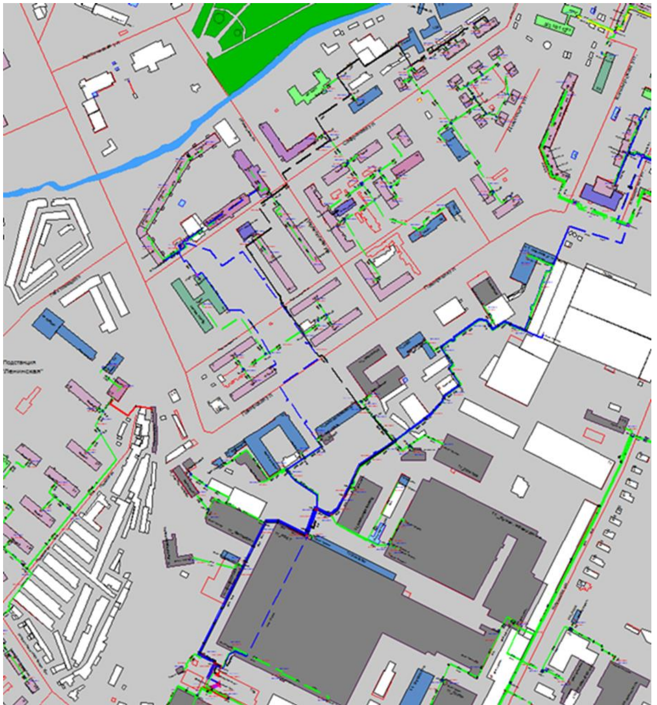
Рисунок 3.35 – Трассировка теплопровода от котельной АО «Теплоэнерго» по ул. Памирская, д. 11 до конечного потребителя «ПТ-Сафрон,15 вв2»
