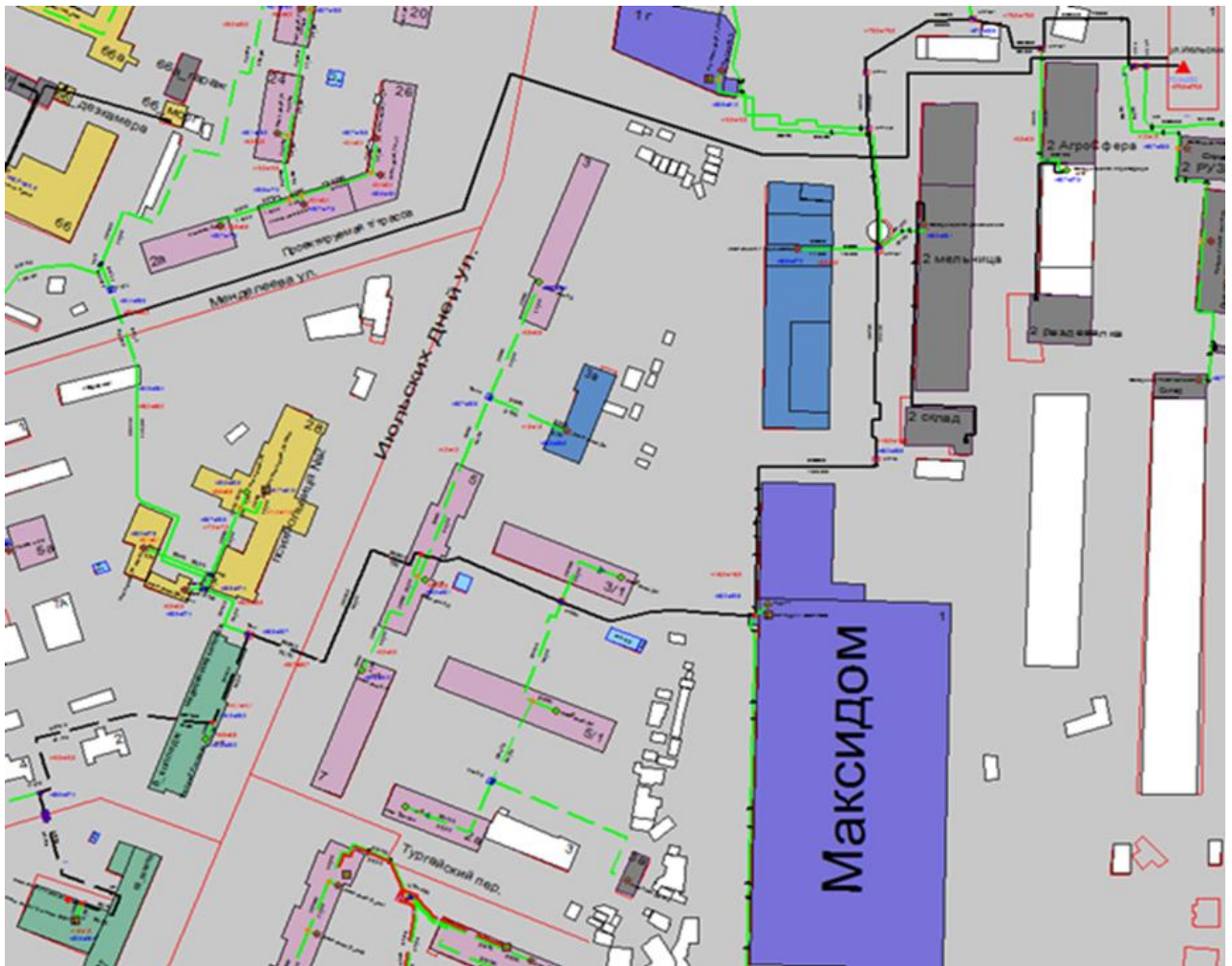
Рисунок 3.43 – Трассировка теплопровода от котельной АО «Теплоэнерго» по ул. Июльских дней, д. 1 до конечного потребителя «ПТ-Июл.дней,10 школа»
