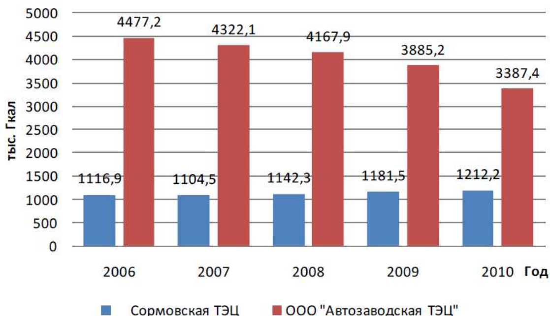
Рисунок 2.2 – Динамика отпуски тепловой энергии с ТЭЦ
