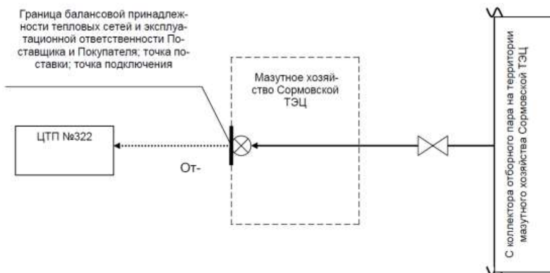
Рисунок 2.7 – Схема присоединения Покупателя №3
