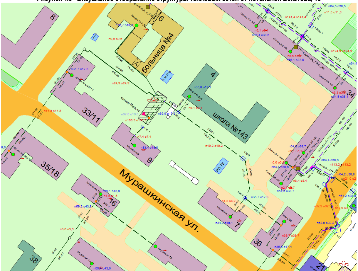
Рисунок 4.7 - Визуальное отображение структуры тепловых сетей от Котельной бульвар Мира, 4а
