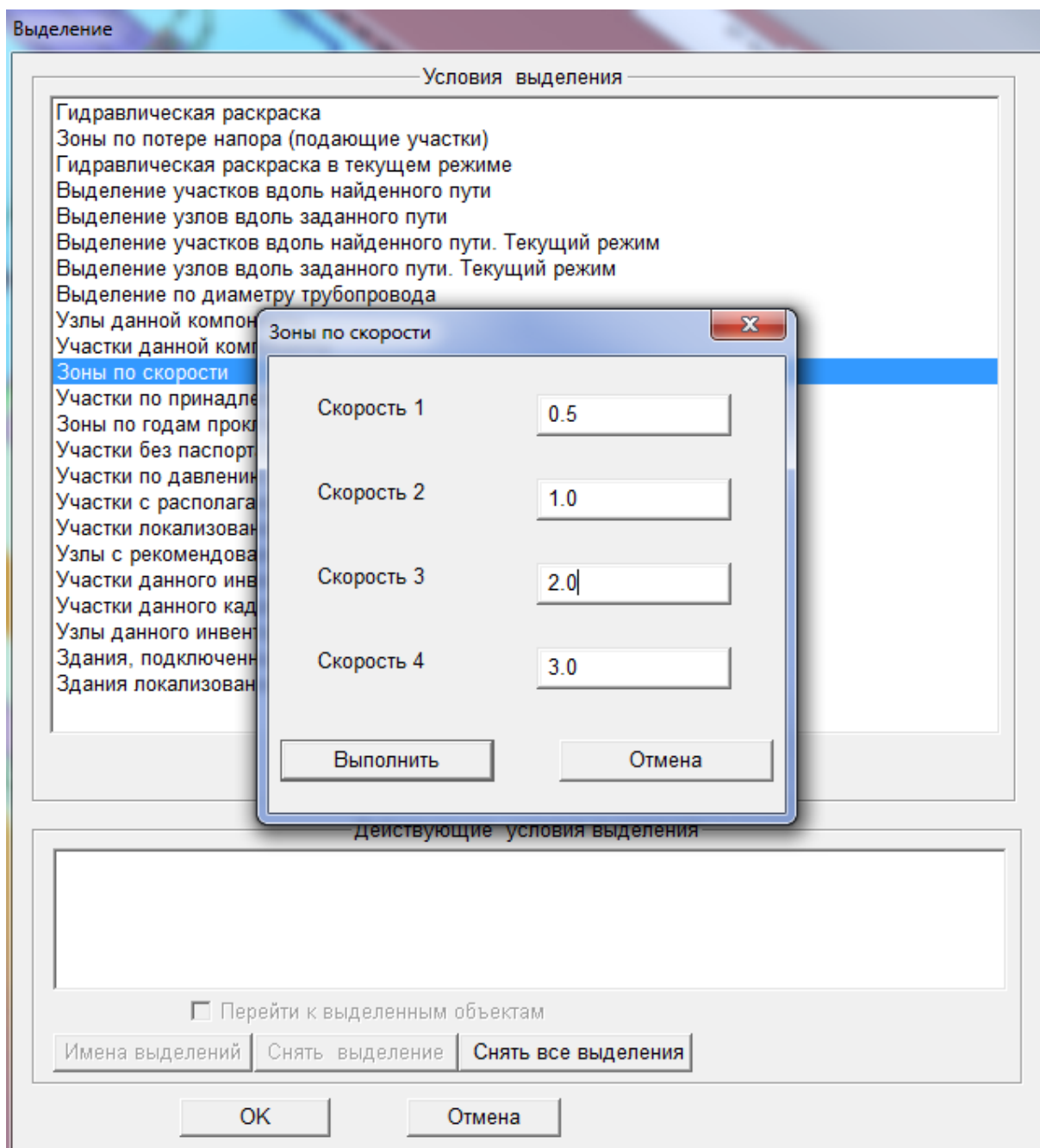
Рисунок 3.10 – Меню Выделение
