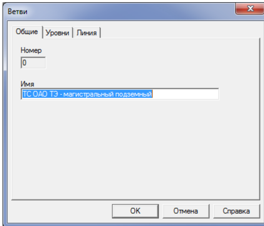
Рисунок 3.143 – Меню Общие
