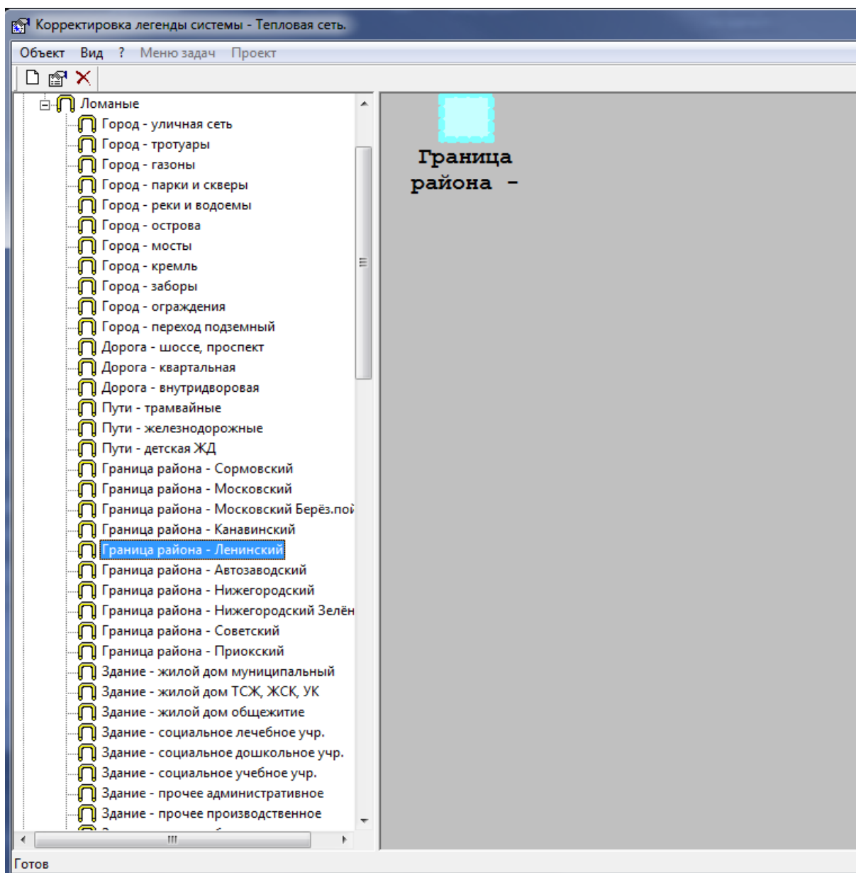
Рисунок 3.146 – Меню Ломаные
