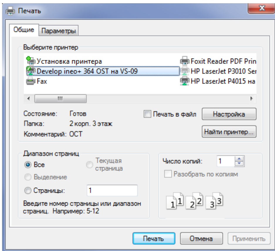
Рисунок 3.102 – Меню Печать
