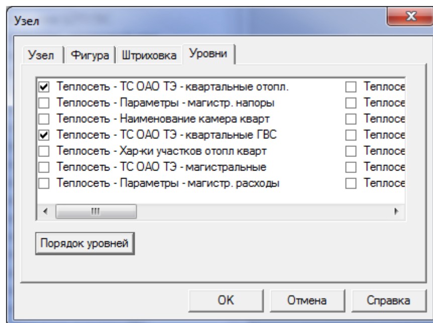
Рисунок 3.140 – Меню Уровни
