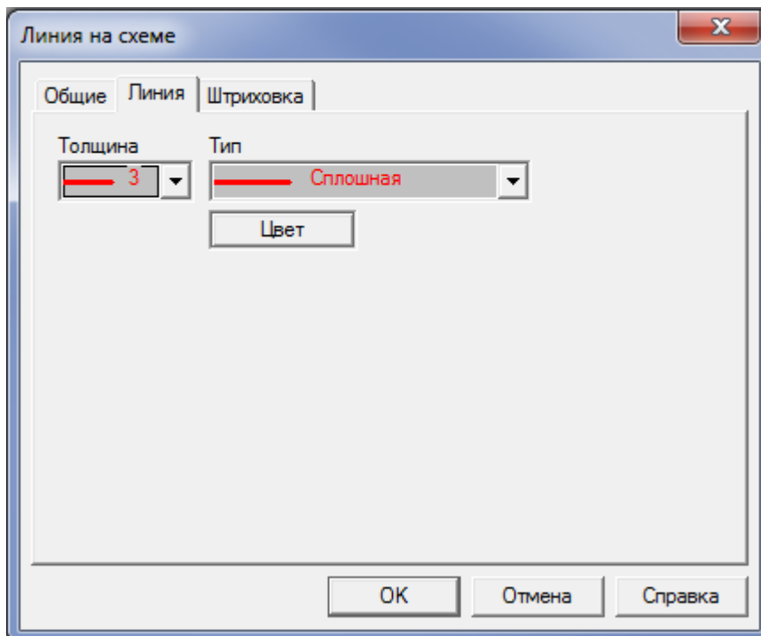
Рисунок 3.156 – Меню Линия
