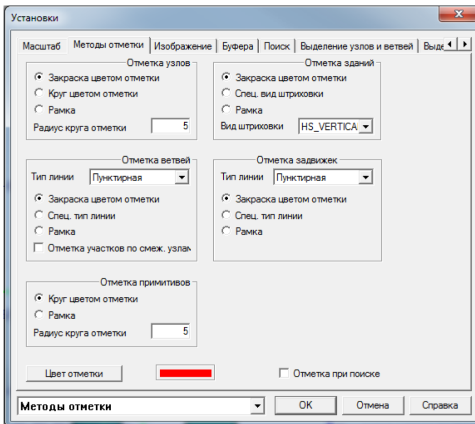
Рисунок 3.131 – Меню Установки
