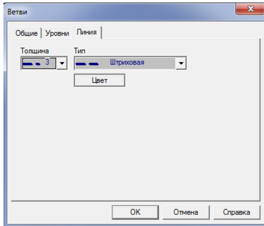
Рисунок 3.145 – Меню Линия
