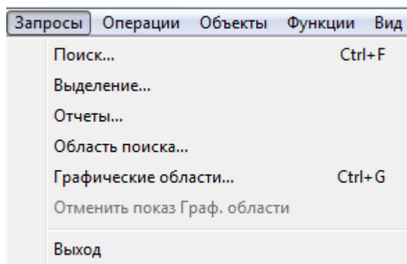
Рисунок 3.4 – Меню Запросы
