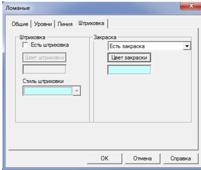
Рисунок 3.150 – Меню Штриховка
