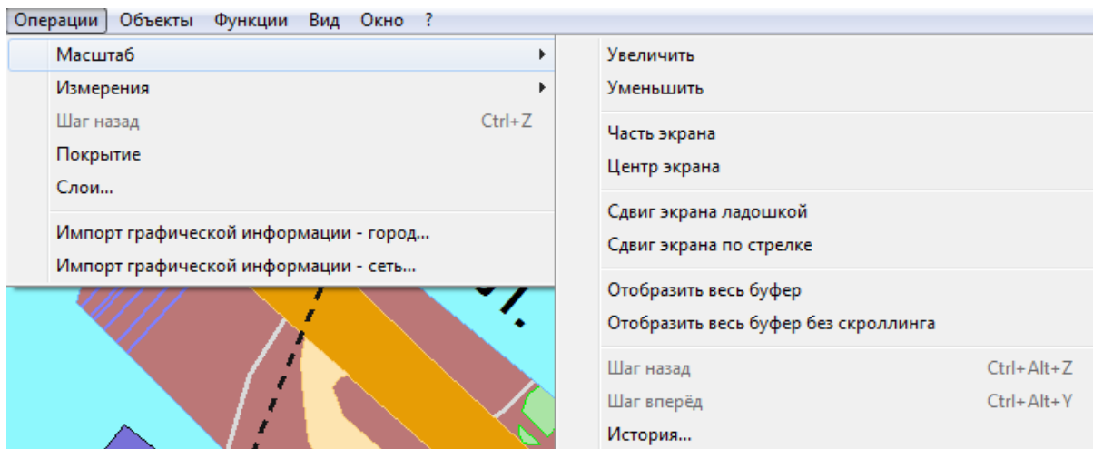
Рисунок 3.18 – Меню Масштаб
