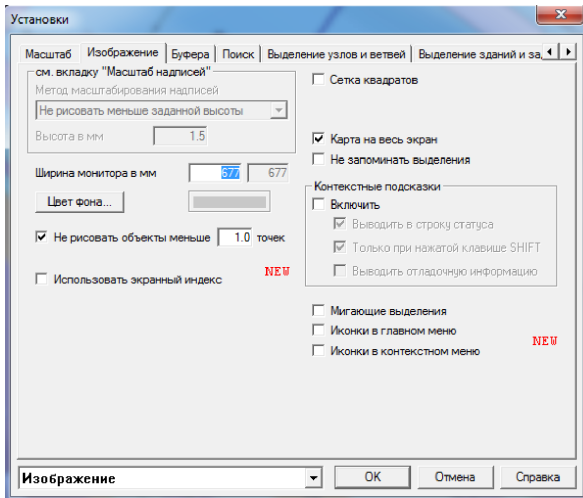
Рисунок 3.78 - Меню Установки
