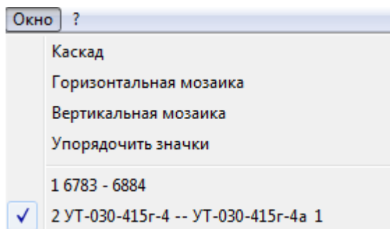
Рисунок 3.107 – Меню Окно
