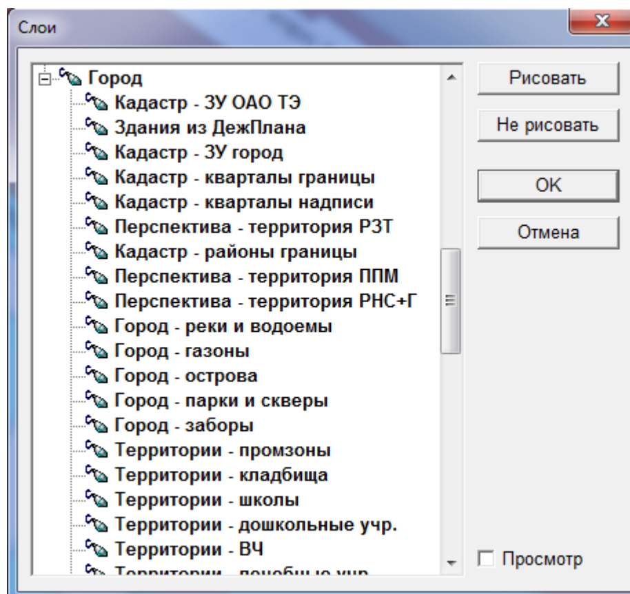
Рисунок 3.25 – Меню Слои
