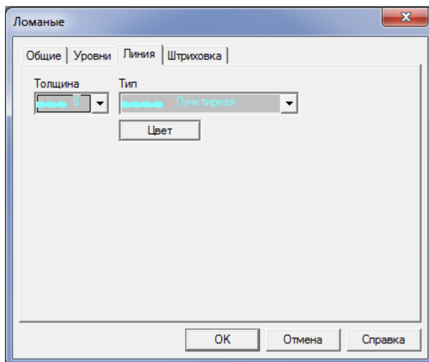
Рисунок 3.149 – Меню Линия
