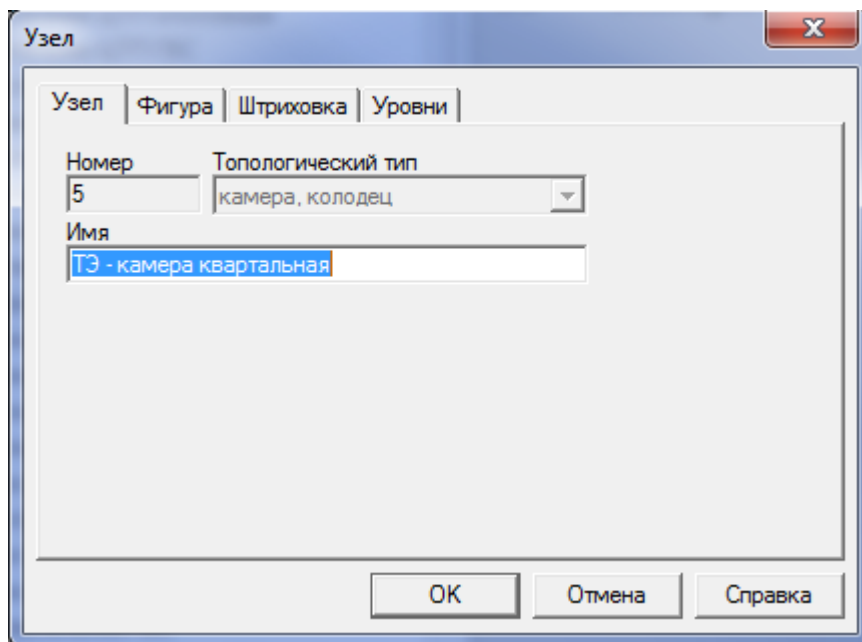
Рисунок 3.137 – Меню Узел
