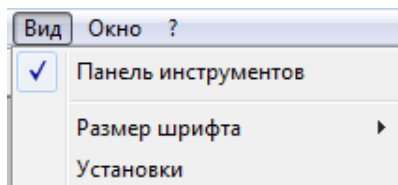
Рисунок 3.104 – Меню Вид
