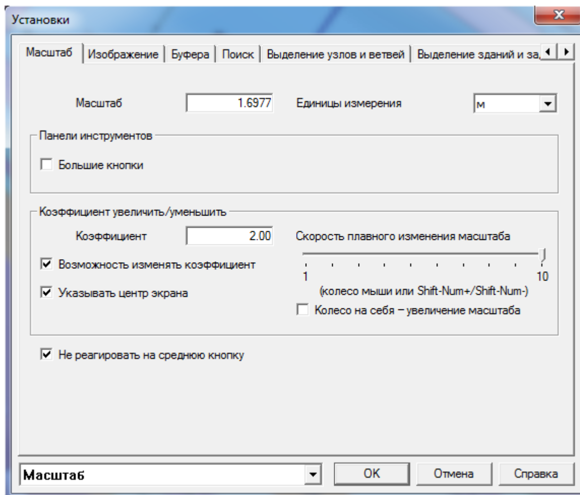
Рисунок 3.77 – Меню Установки
