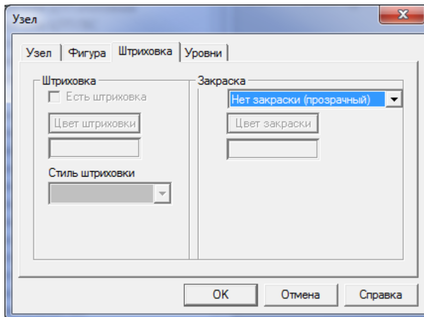
Рисунок 3.139 – Меню Штриховка
