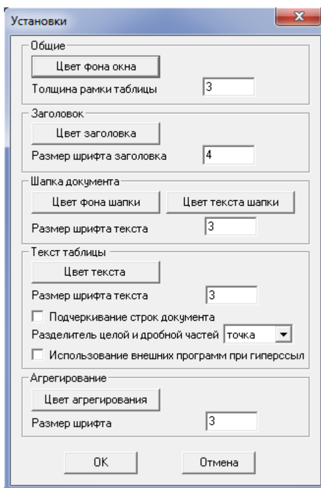
Рисунок 3.106 – Меню Установки
