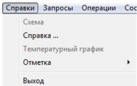
Рисунок 3.96 – Меню Справки
