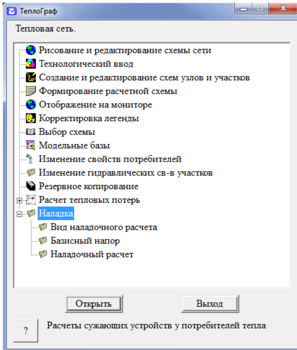
Рисунок 3.166 – Меню Наладка
