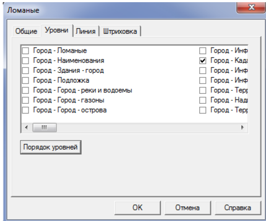
Рисунок 3.148 – Меню Уровни
