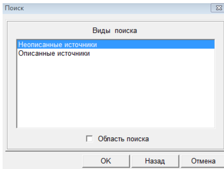
Рисунок 3.85 – Меню Поиск
