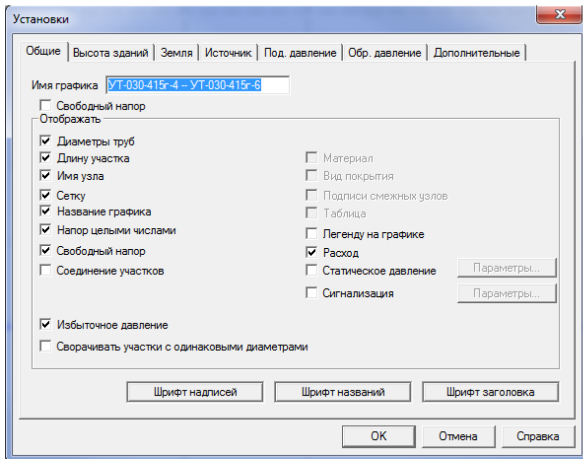
Рисунок 3.123 – Меню Установки
