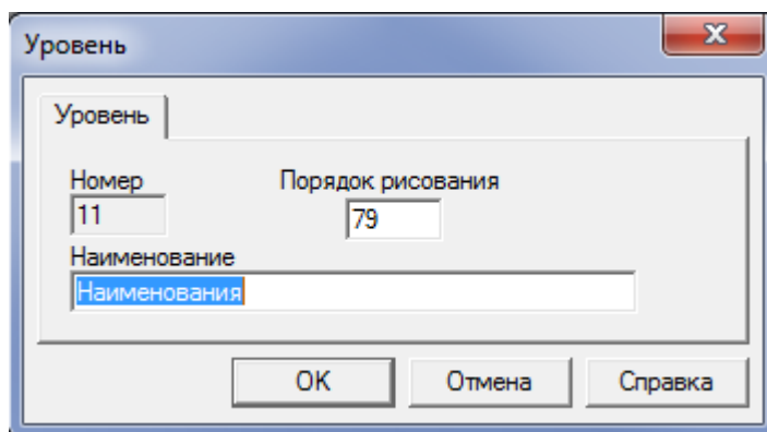
Рисунок 3.135 – Меню Уровень
