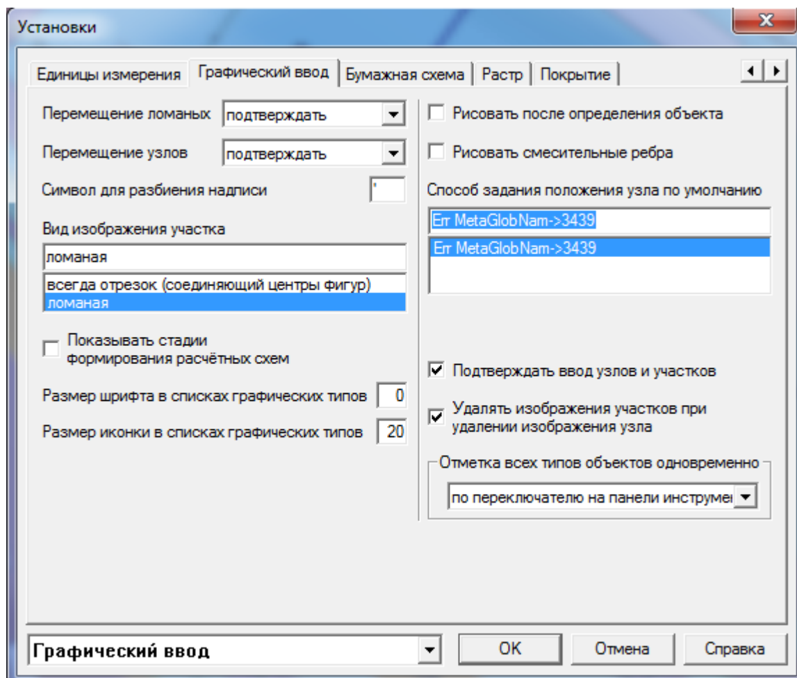
Рисунок 3.76 – Меню Установки
