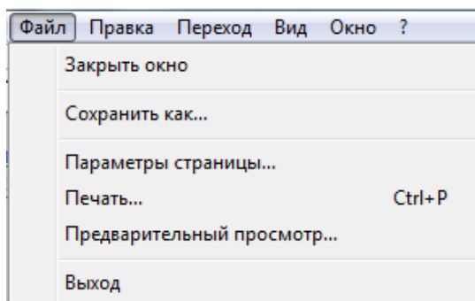
Рисунок 3.100 – Меню Файл
