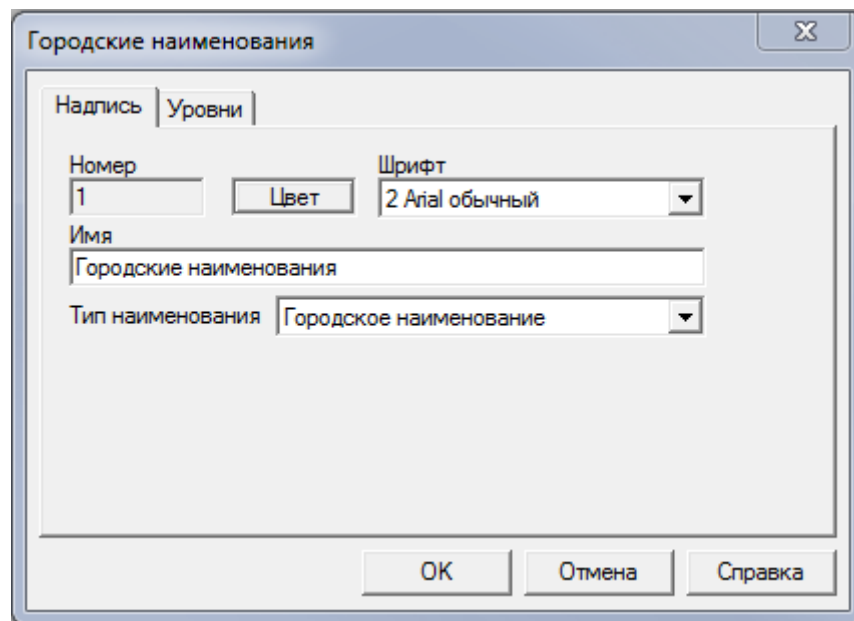
Рисунок 3.152 – Меню Надпись
