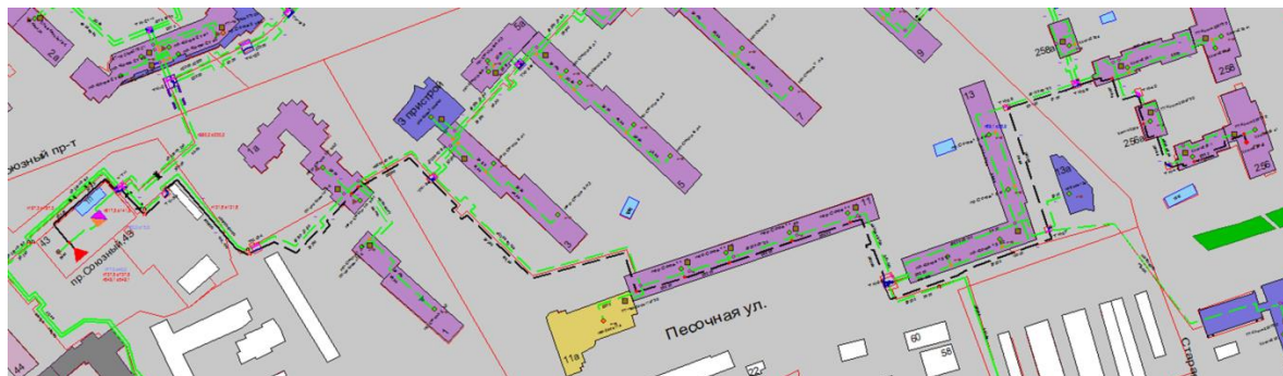
Рисунок 1.61 Результат гидравлического расчета - расчетный путь теплоносителя от котельной пр. Союзный, 43 до ПТ-Комин,256 э2
