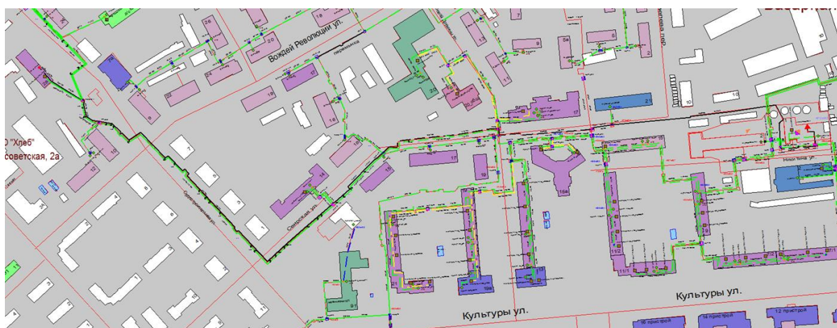
Рисунок 1.103 Результат гидравлического расчета - расчетный путь теплоносителя от котельной Пугачева, 1 до ПТ-Судостр.28
