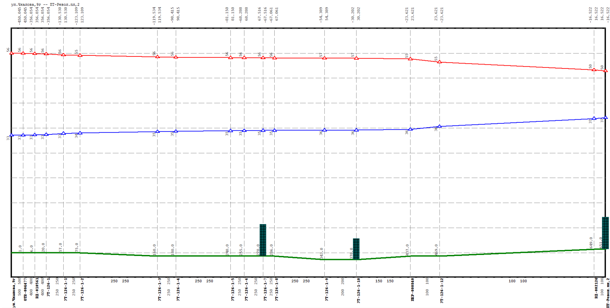
Рисунок 1.96 Результат гидравлического расчета - график гидравлических режимов по пути теплоносителя от котельной Чкалова, 9д до ПТ-Революции, пл.2
