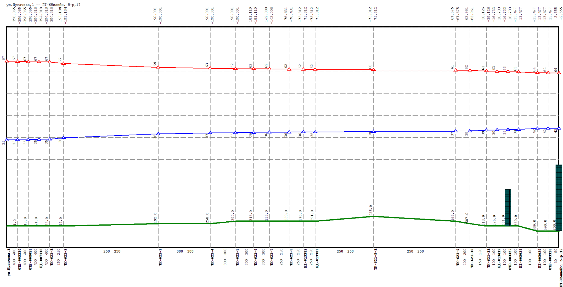
Рисунок 1.106 Результат гидравлического расчета - график гидравлических режимов по пути теплоносителя от котельной Пугачева, 1 до ПТ-Юбилейн. б-р,17
