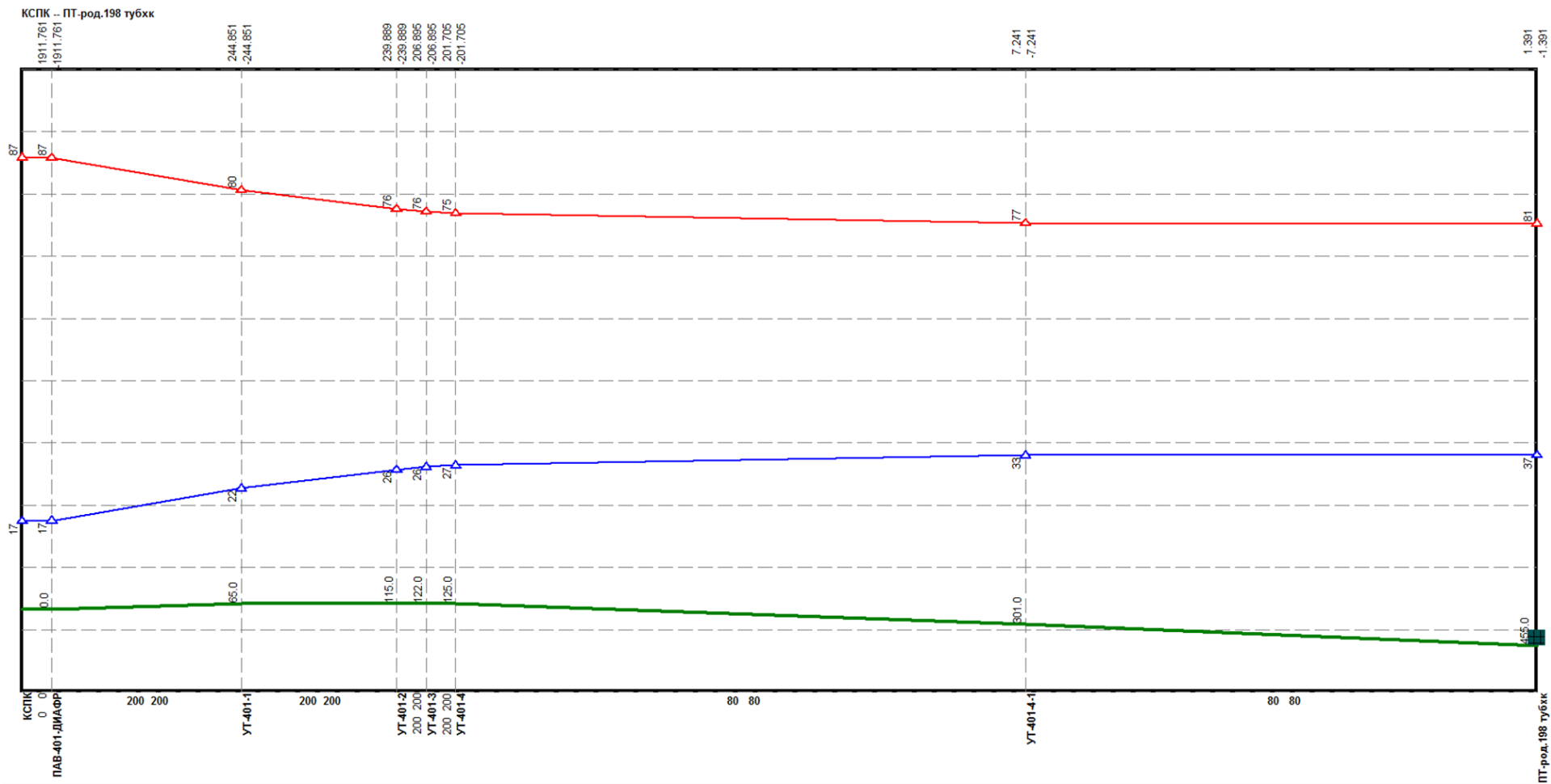
Рисунок 1.68 Результат гидравлического расчета - график гидравлических режимов по пути теплоносителя от котельной ул. Родионова, 1946 до ПТ-род.198 тубхк
