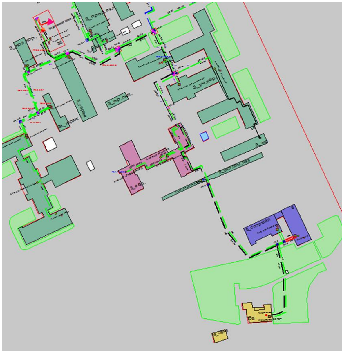
Рисунок 1.91 Результат гидравлического расчета - расчетный путь теплоносителя от котельной Анкудиновское шоссе, 3-б до ПТ-Анкуд.ш,5а
