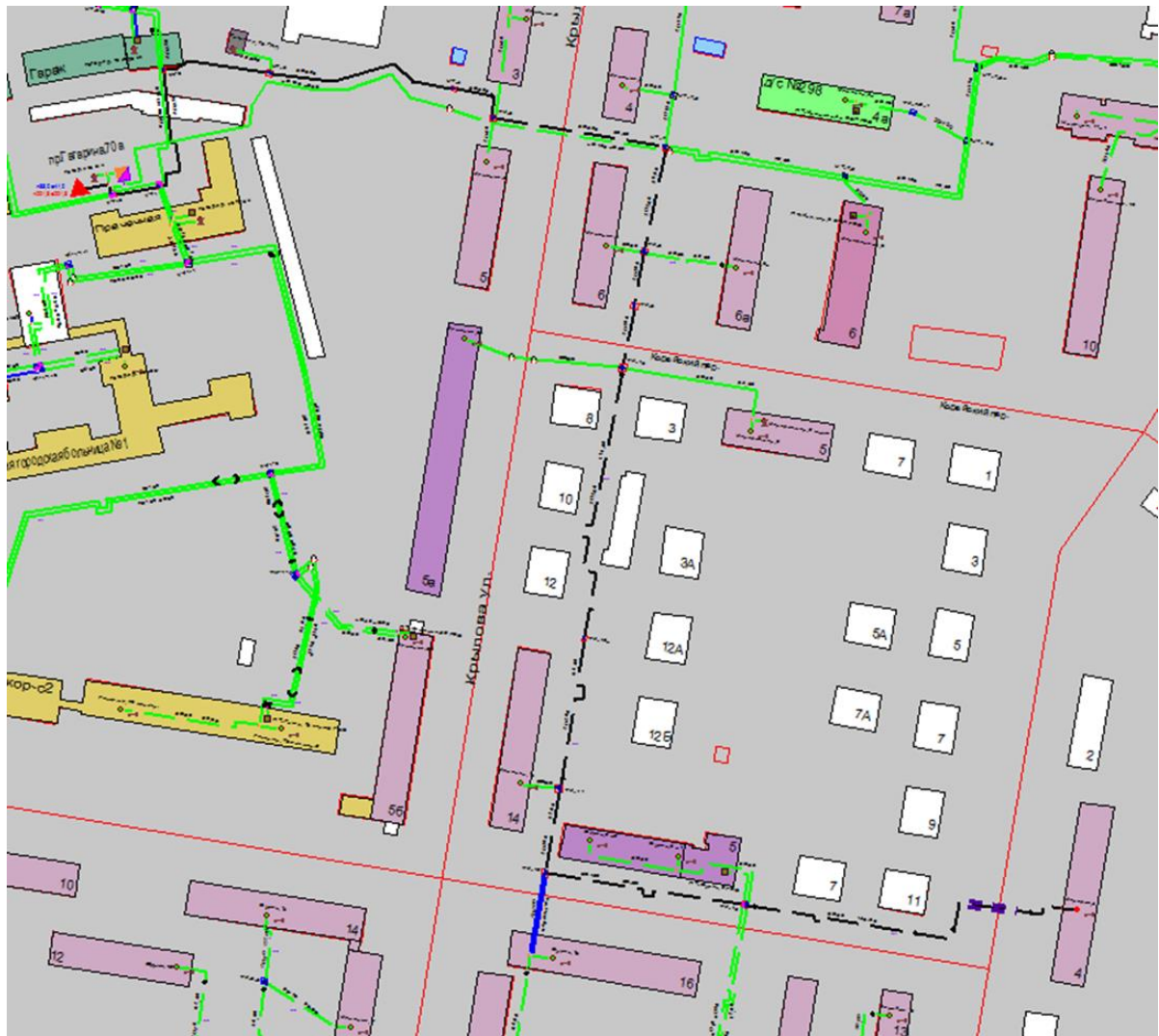
Рисунок 1.45 Результат гидравлического расчета - расчетный путь теплоносителя от котельной пр. Гагарина, 70а до ПТ-Корейск,4
