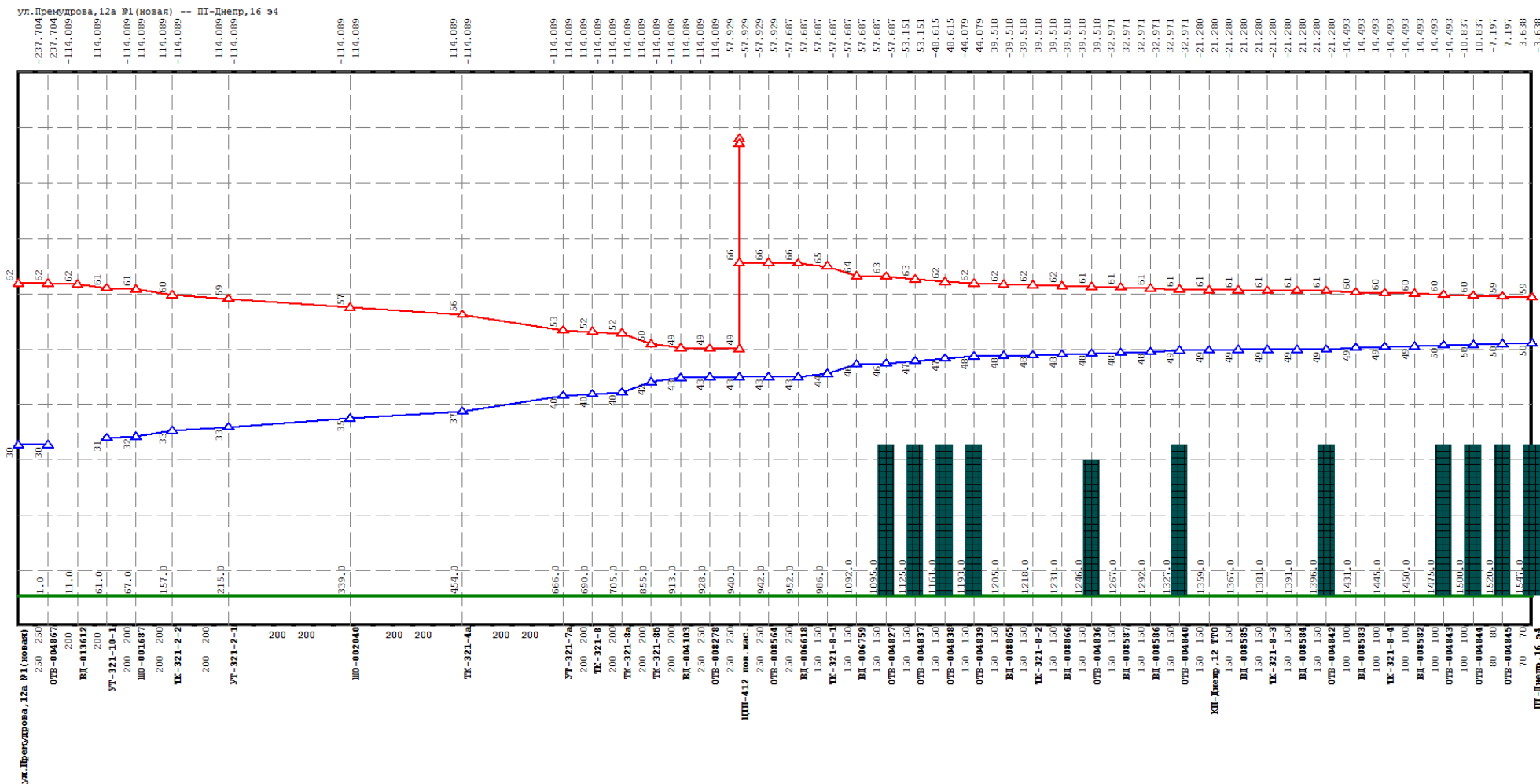
Рисунок 1.110 Результат гидравлического расчета - график гидравлических режимов по пути теплоносителя от котельной Премудрова, 12а до ПТ-Днепр, 16 э4
