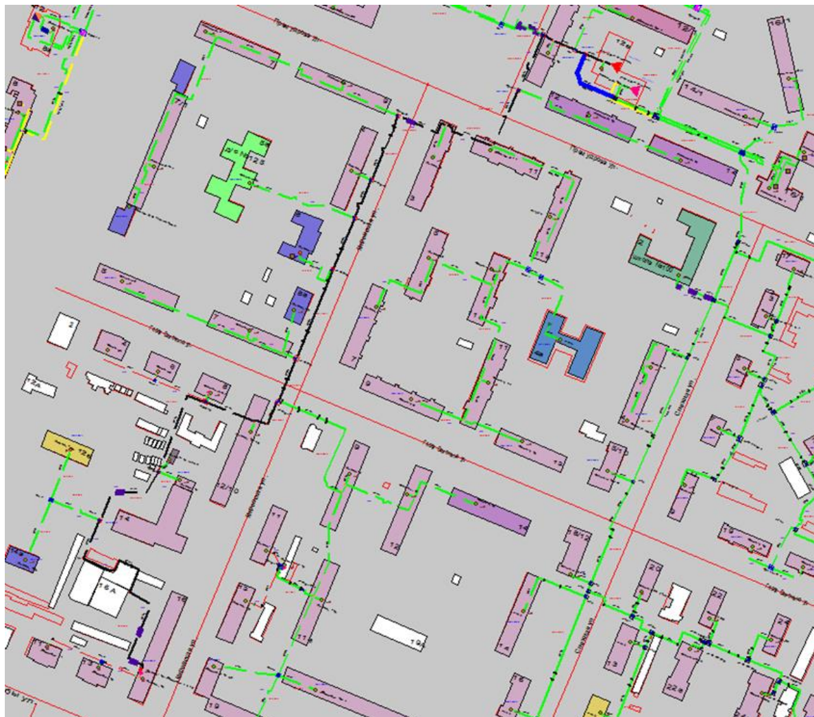
Рисунок 1.113 Результат гидравлического расчета - расчетный путь теплоносителя от котельной Премудрова, 12а до ПТ-Дружбы,11
