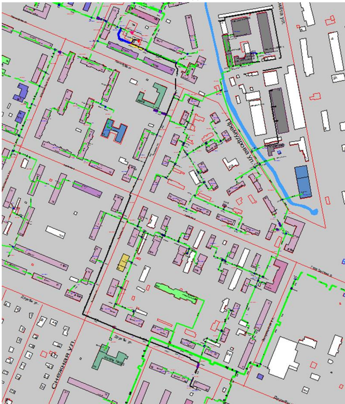
Рисунок 1.107 Результат гидравлического расчета - расчетный путь теплоносителя от котельной Премудрова, 12а до ПТ-Друбы,56
