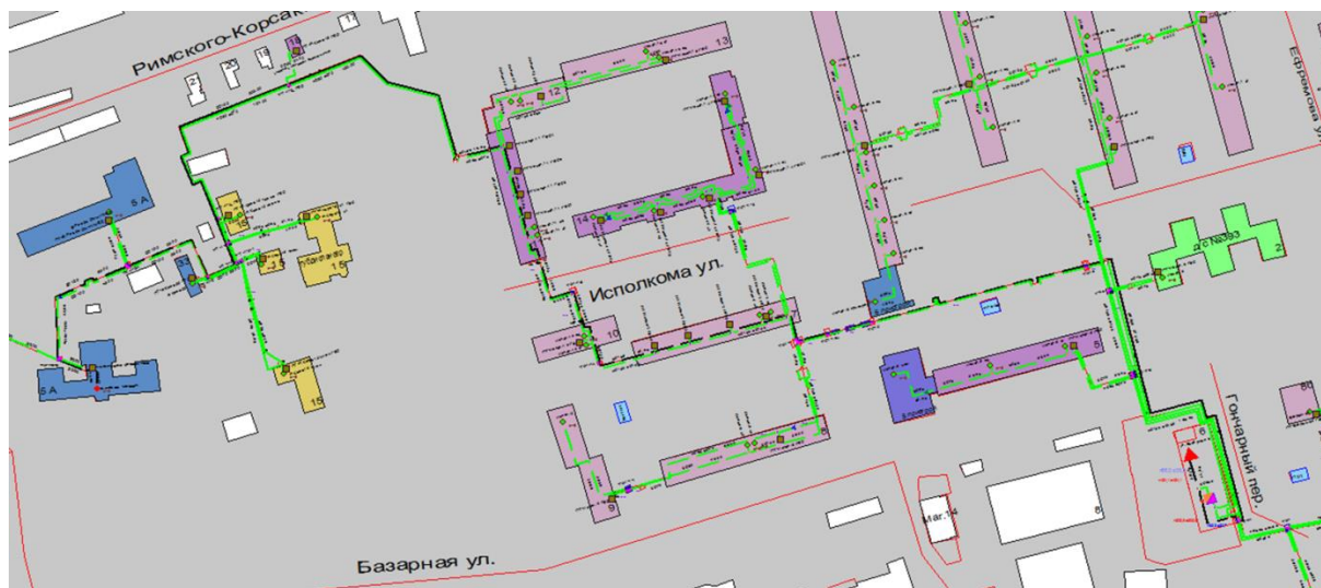
Рисунок 1.79 Результат гидравлического расчета - расчетный путь теплоносителя от котельной ул. Базарная, 6 до ПТ-В.Рев,5а УФССП
