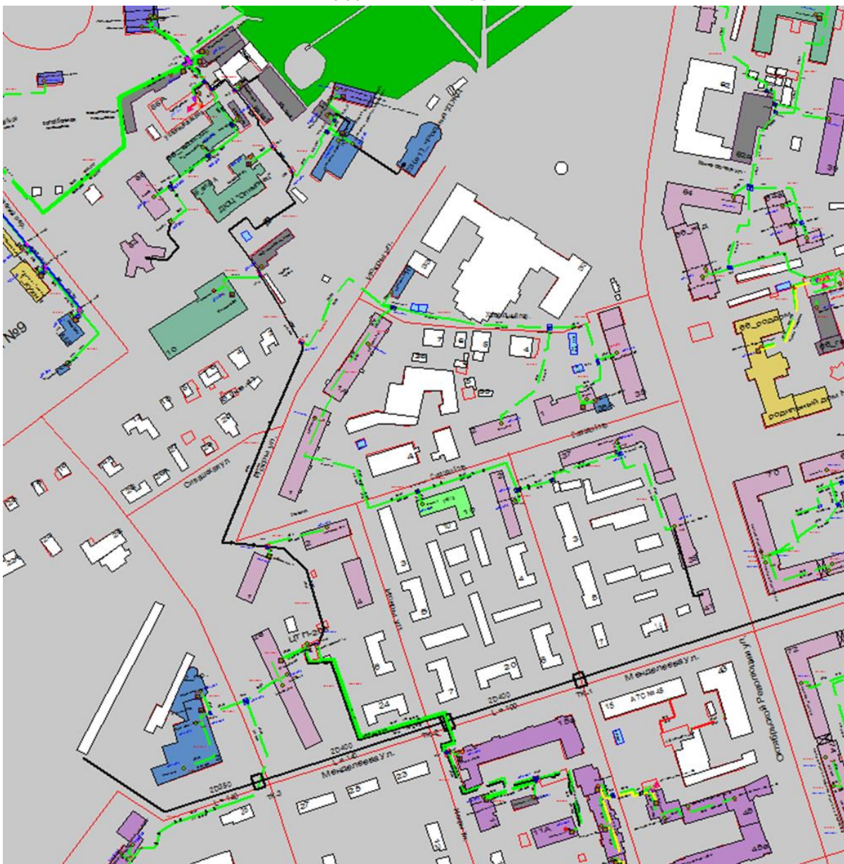
Рисунок 1.37 Результат гидравлического расчета - расчетный путь теплоносителя от котельной Климковская, 86а до ПТ-Искры, 11а
