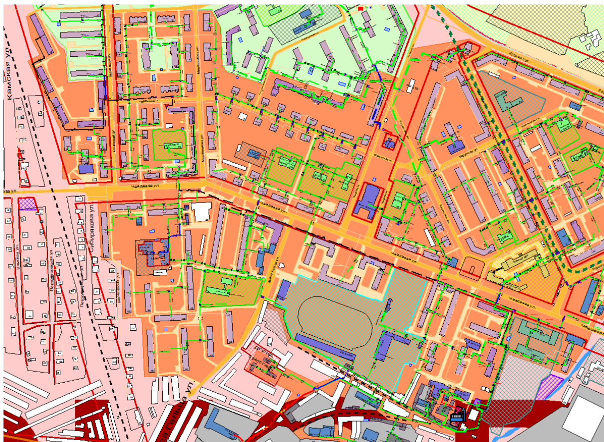
Рисунок 1.93 Результат гидравлического расчета - расчетный путь теплоносителя от котельной Чаадаева, 10 до ПТ-Мечн,63.
