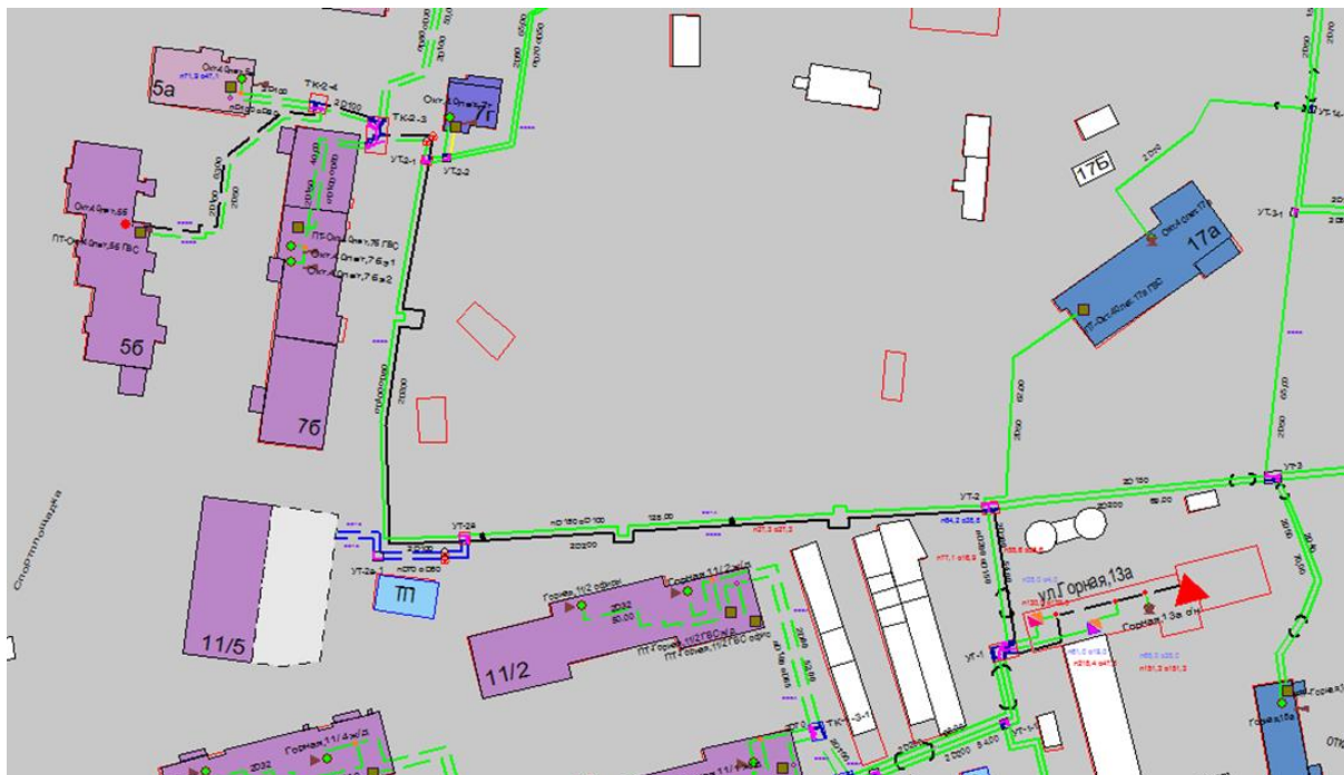
Рисунок Ошибка! Текст указанного стиля в документе отсутствует..41 Результат гидравлического расчета - расчетный путь теплоносителя от котельной Горная, 13 до ПТ-Окт.40лет,56
