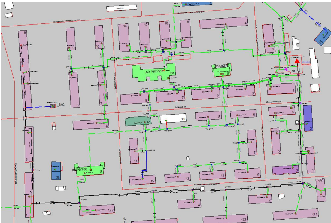
Рисунок Ошибка! Текст указанного стиля в документе отсутствует..19 Результат гидравлического расчета - расчетный путь теплоносителя от котельной Гастелло, 1-а до ПТ-Березов,5 вв3
