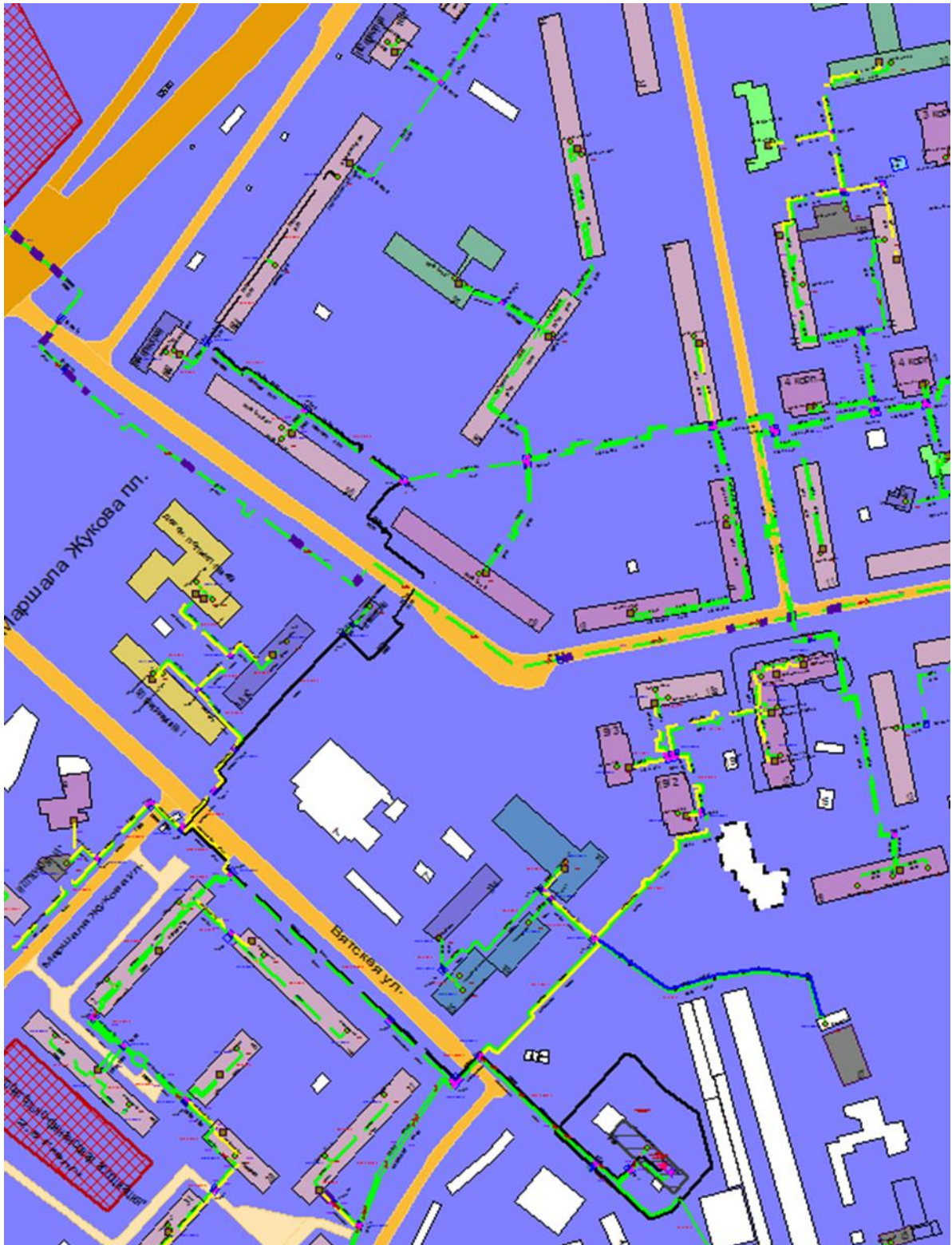
Рисунок Ошибка! Текст указанного стиля в документе отсутствует..35 Результат гидравлического расчета - расчетный путь теплоносителя от котельной ул. Голованова, 25-а до ПТ-Гагар.пр,184 э2
