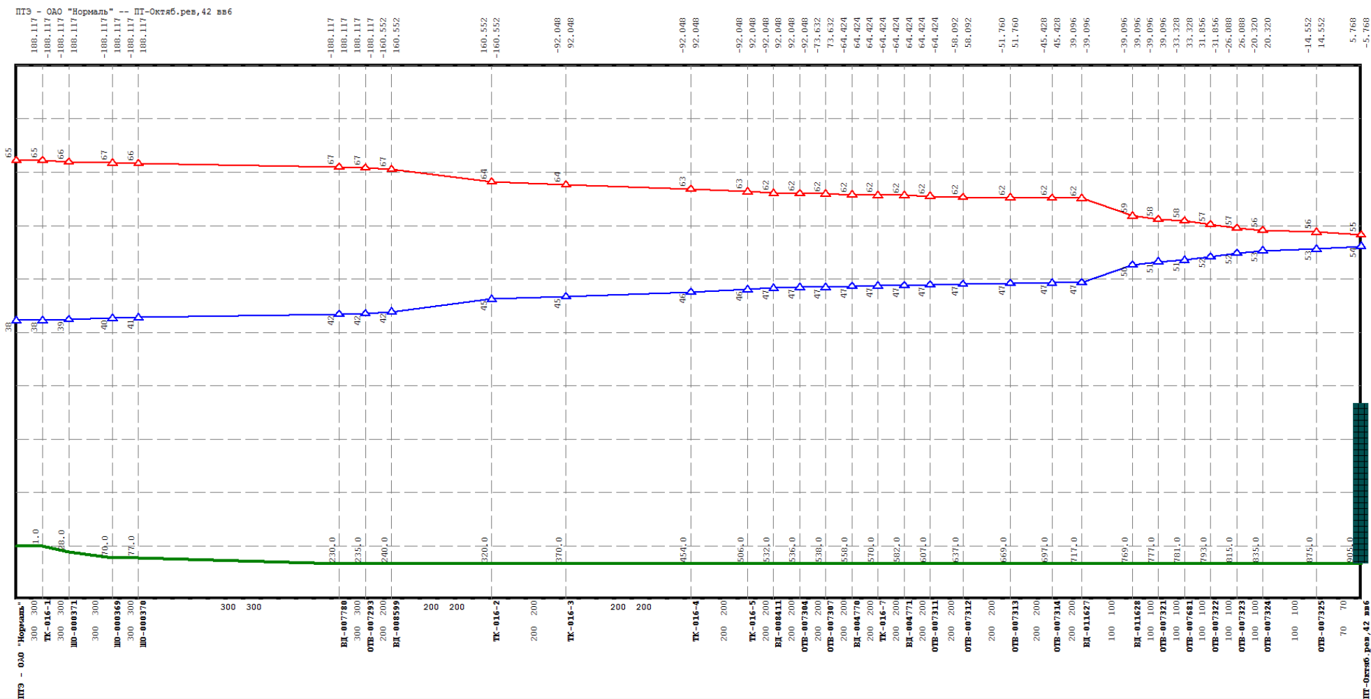
Рисунок Ошибка! Текст указанного стиля в документе отсутствует..68 Результат гидравлического расчета - график гидравлических режимов по пути теплоносителя от котельной Литвинова, 74 до ПТ-Октяб.рев,42 вв6
