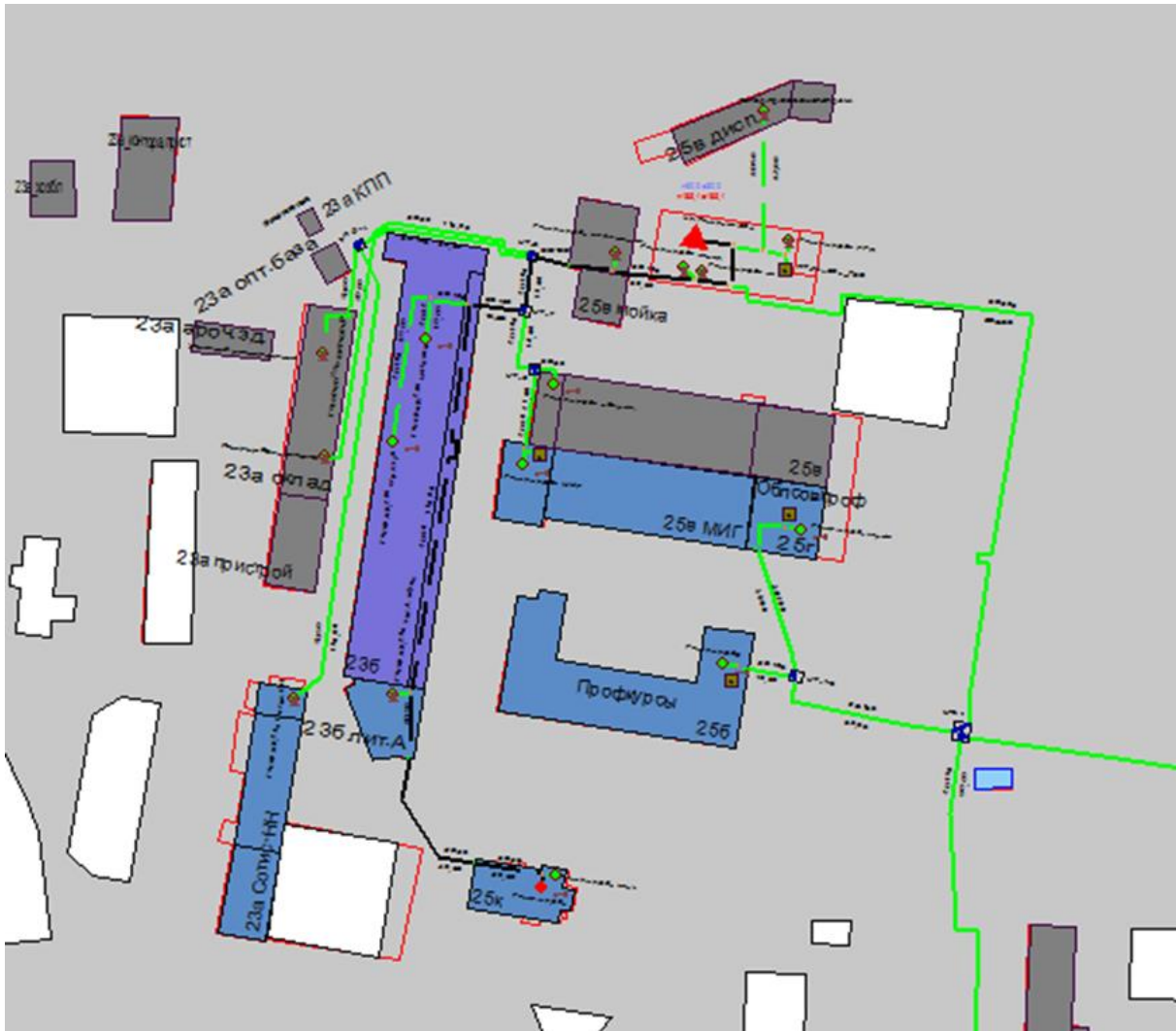
Рисунок Ошибка! Текст указанного стиля в документе отсутствует..55 Результат гидравлического расчета - расчетный путь теплоносителя от котельной Гагарина, 25-е до ПТ-Гагар.пр,25к
