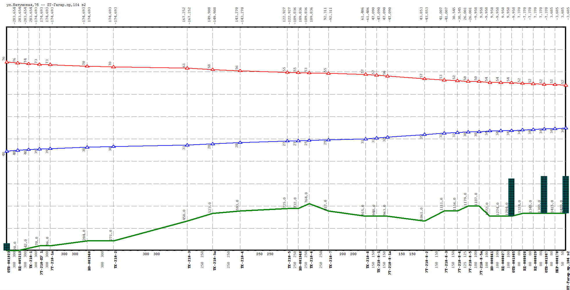
Рисунок Ошибка! Текст указанного стиля в документе отсутствует..30 Результат гидравлического расчета - график гидравлических режимов по пути теплоносителя от котельной Батумская, 7-б до ПТ-Гагар.пр,104 э2
