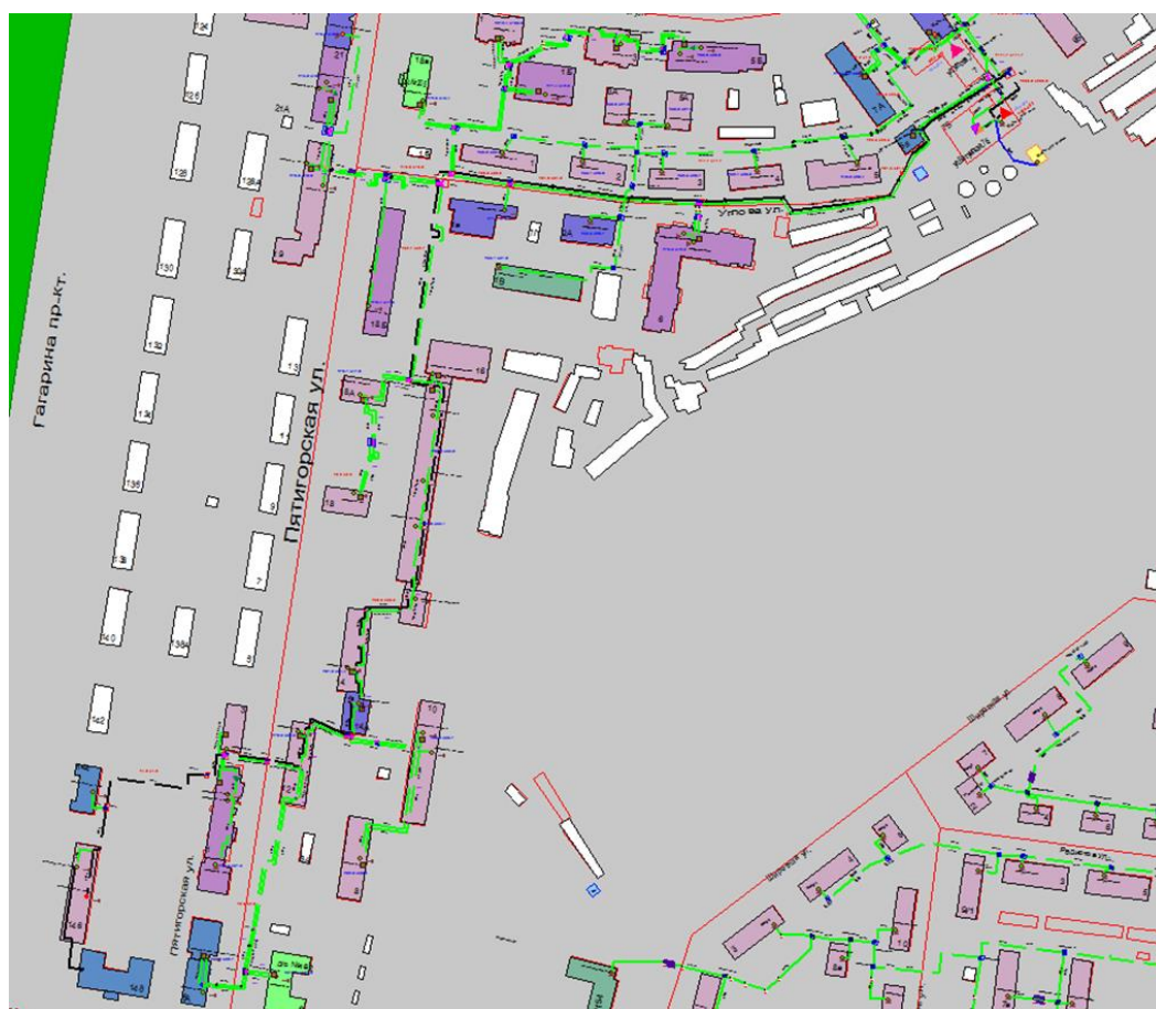
Рисунок Ошибка! Текст указанного стиля в документе отсутствует. 27 Результат гидравлического расчета - расчетный путь теплоносителя от котельной Батумская, 7-б до ПТ-Гагар.пр,146
