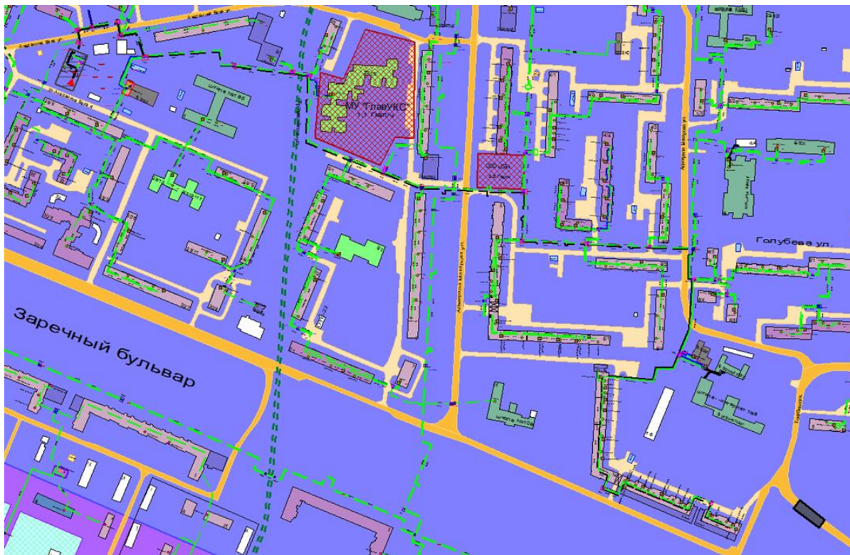
Рисунок Ошибка! Текст указанного стиля в документе отсутствует..9 Результат гидравлического расчета - расчетный путь теплоносителя от котельной Академика Баха, 4-а до ПТ-Макар,18 э2
