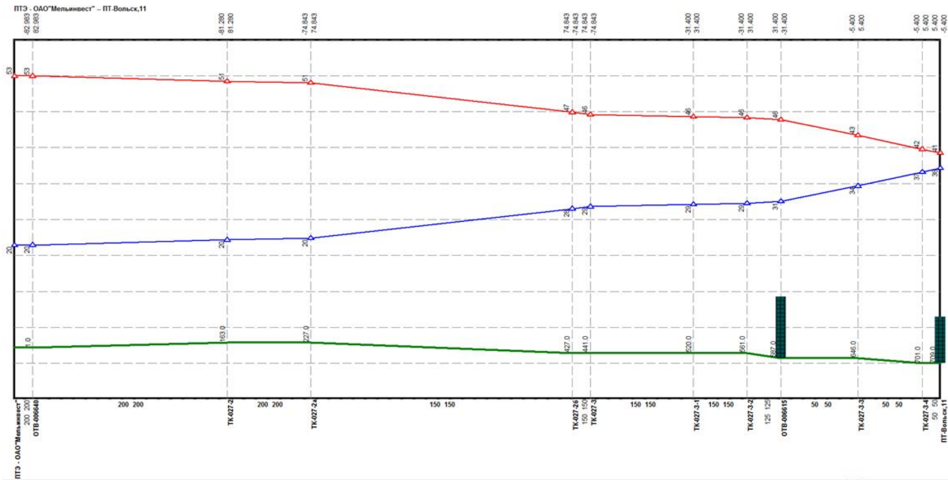
Рисунок Ошибка! Текст указанного стиля в документе отсутствует..118 Результат гидравлического расчета - график гидравлических режимов по пути теплоносителя от котельной Интернациональная, 95 до ПТ-Вольск,11
