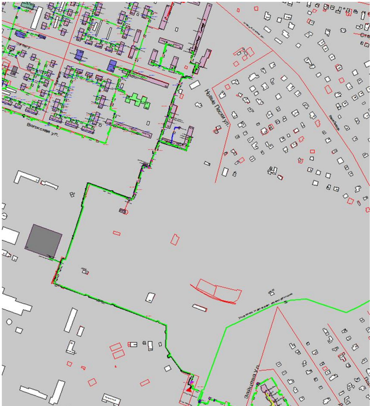
Рисунок Ошибка! Текст указанного стиля в документе отсутствует..59 Результат гидравлического расчета - расчетный путь теплоносителя от котельной Зайцева, 31 до ПТ-Ясная,33 э3
