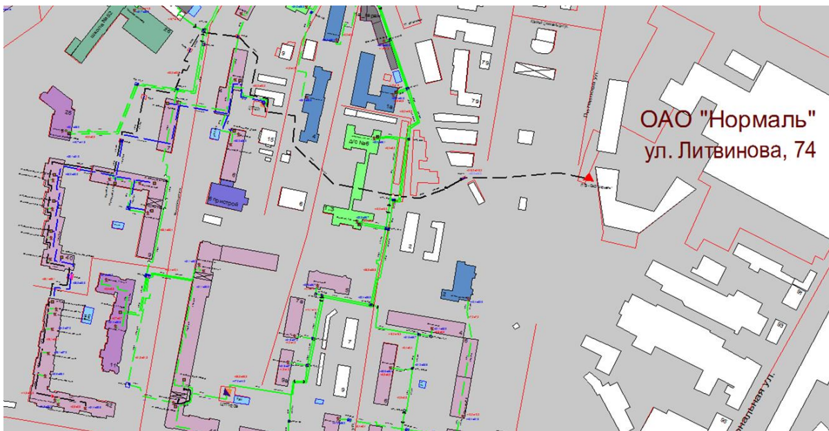
Рисунок 67 Результат гидравлического расчета - расчетный путь теплоносителя от котельной Литвинова, 74 до ПТ-Октяб.рев,42 вв6
