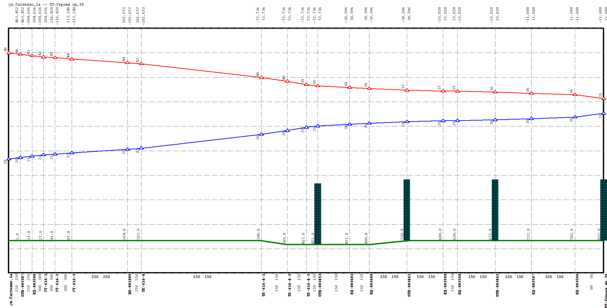
Рисунок Ошибка! Текст указанного стиля в документе отсутствует..22 Результат гидравлического расчета - график гидравлических режимов по пути теплоносителя от котельной Гастелло, 1-а до ПТ-Героев пр., 39
