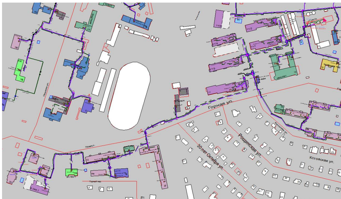
Рисунок 1.161 Результат гидравлического расчета - расчетный путь теплоносителя от котельной Горная, 13 до ПТ-Горная,2а
