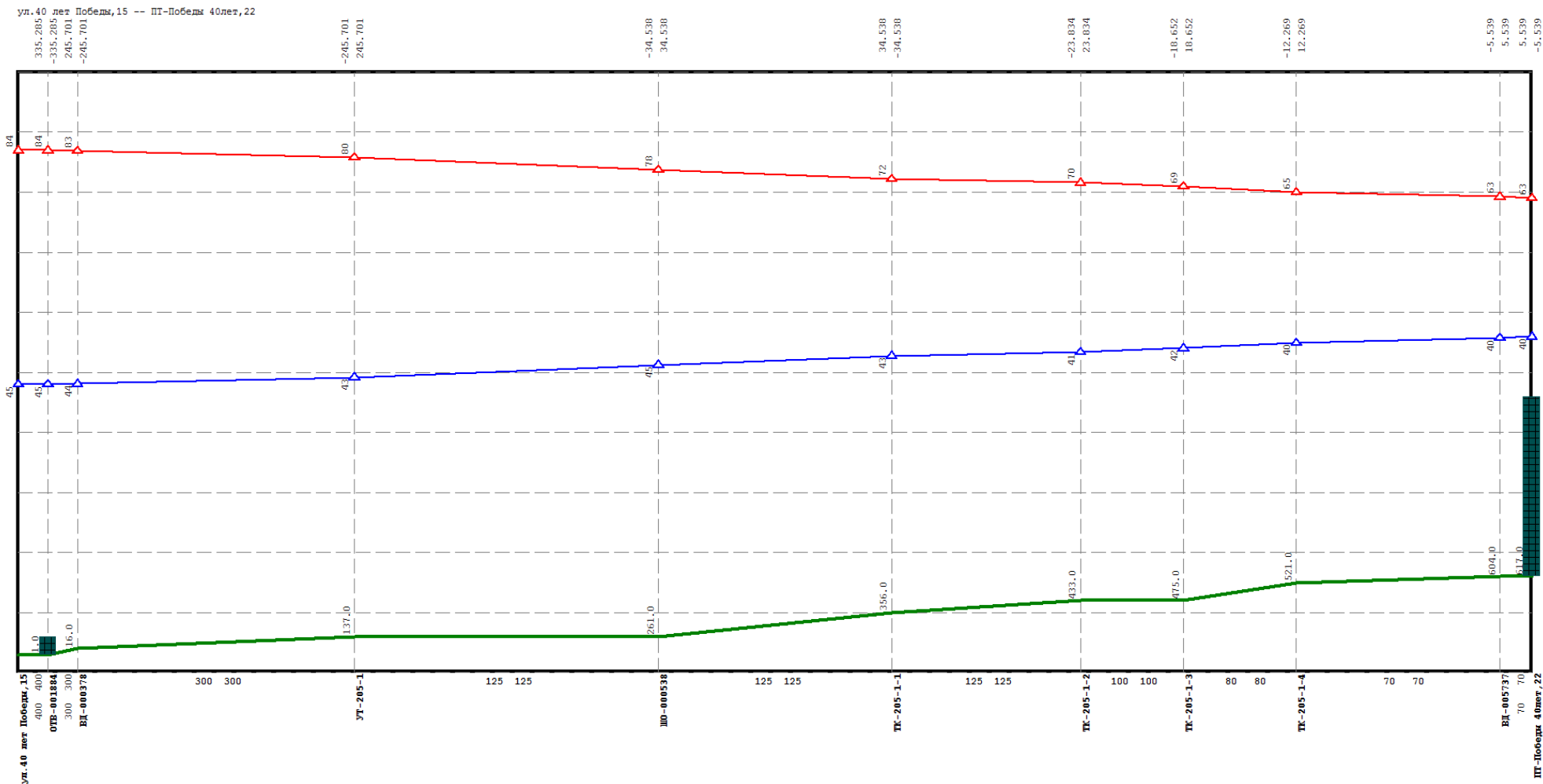
Рисунок Ошибка! Текст указанного стиля в документе отсутствует..46 Результат гидравлического расчета - график гидравлических режимов по пути теплоносителя от котельной 40 лет Победы, 15 до ПТ-Победы 40лет,22
