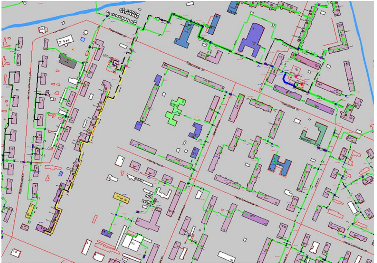
Рисунок 3.118 – Трассировка теплопровода от котельной АО «Теплоэнерго» по ул. Премудрова, д. 12А до конечного потребителя «ПТ-Днепр,16 34»
