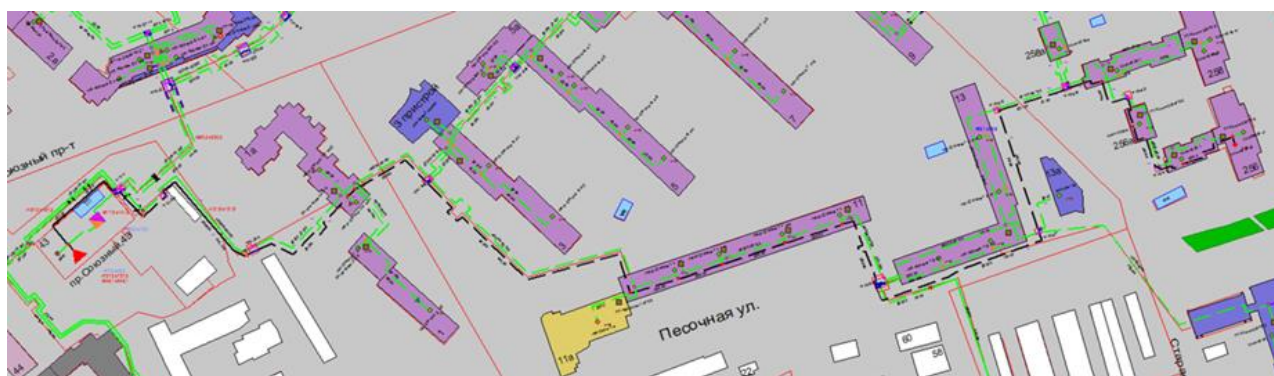
Рисунок 3.78 – Трассировка теплопровода от котельной АО «Теплоэнерго» по пр. Союзный, д. 43 до конечного потребителя «ПТ-Комин,256 э2»
