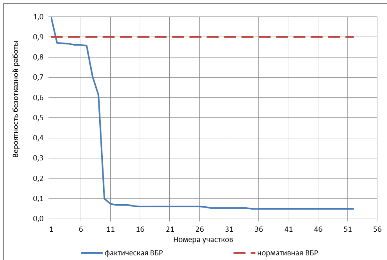
Рисунок 3.5 – Вероятность безотказной работы относительно ТК потребителя «ПТ-Люкина, 5 аптека» тепловых сетей зоны Сормовской ТЭЦ (расчетный путь 1-2) к 2030 году без проведения мероприятий по реконструкции участков тепловой сети
