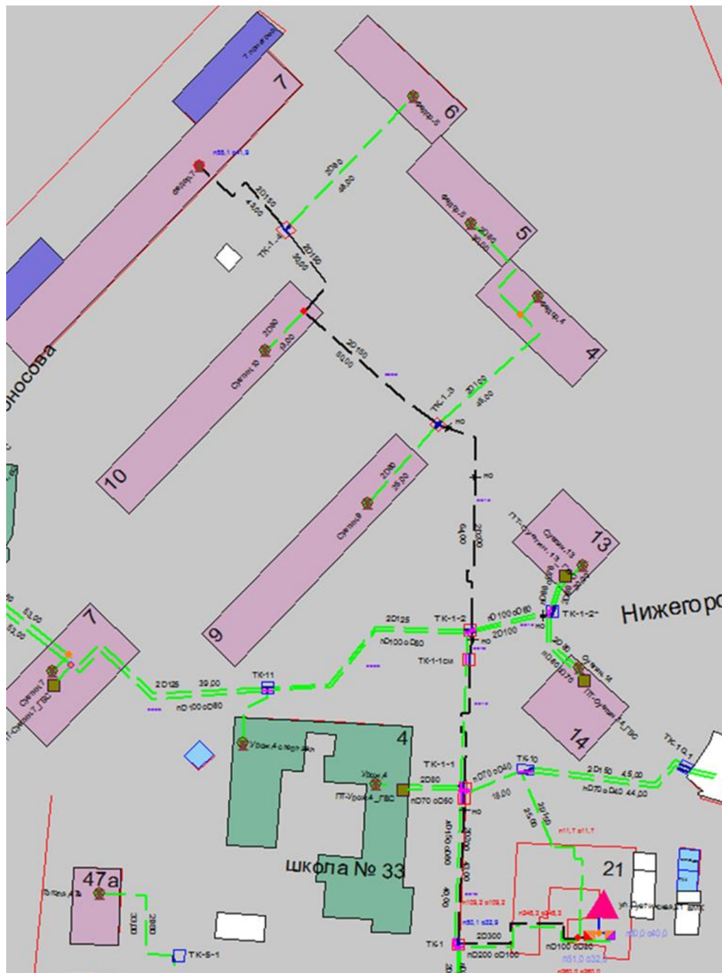
Рисунок 3.33 – Трассировка теплопровода от котельной АО «Теплоэнерго» по ул. Суетинская, д. 21 (БМК) до конечного потребителя «ПТ-Федор,7
