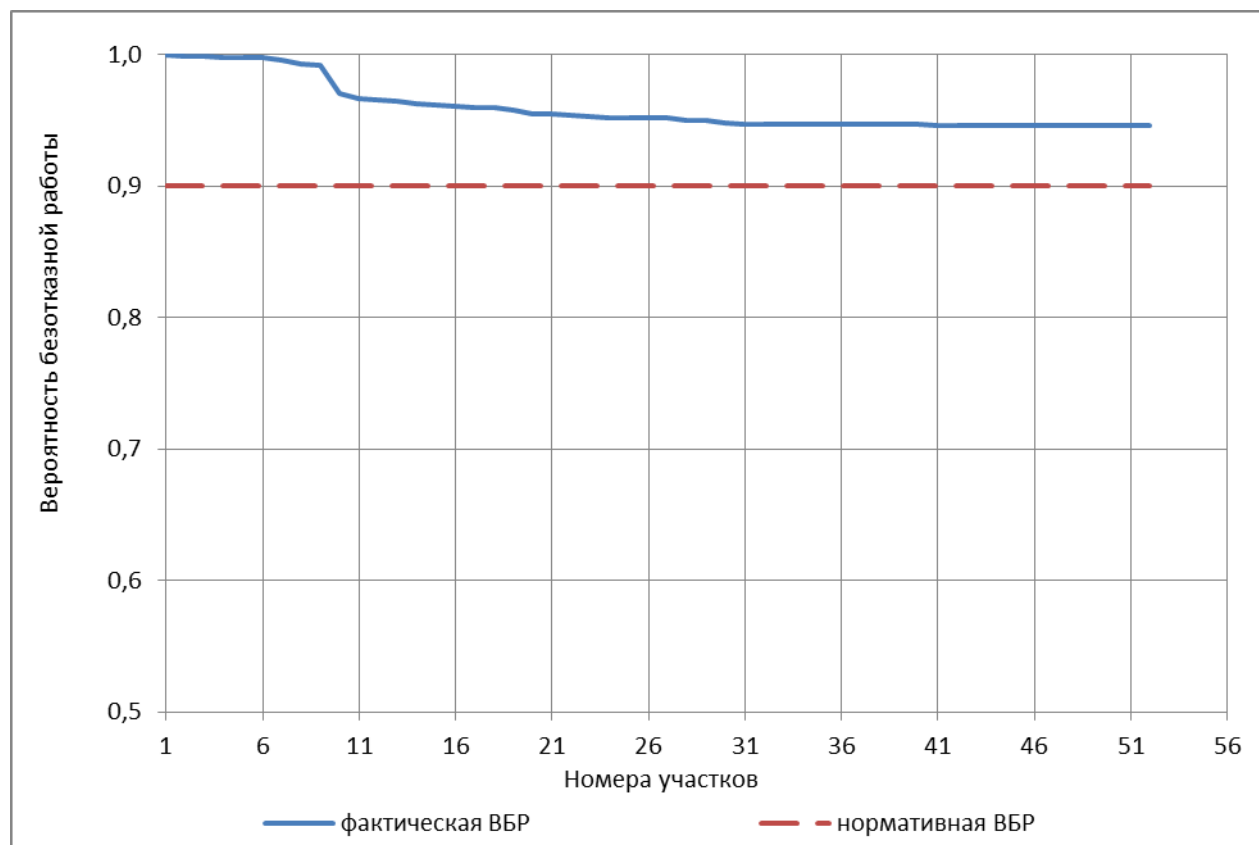
Рисунок 3.6 – Вероятность безотказной работы относительно ТК потребителя «ПТ-Люкина, 5 аптека» тепловых сетей зоны Сормовской ТЭЦ (расчетный путь 1-2) при поэтапной реконструкции участков тепловой сети, осуществляемой за период до 2030 года
