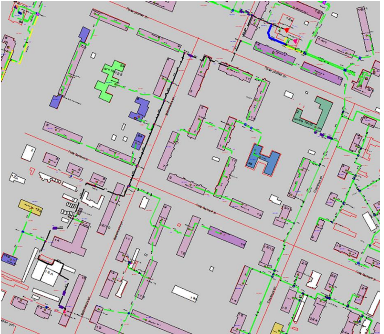
Рисунок 3.122 – Трассировка теплопровода от котельной АО «Теплоэнерго» по ул. Премудрова, д. 12А до конечного потребителя «ПТ-Дружбы,11»
