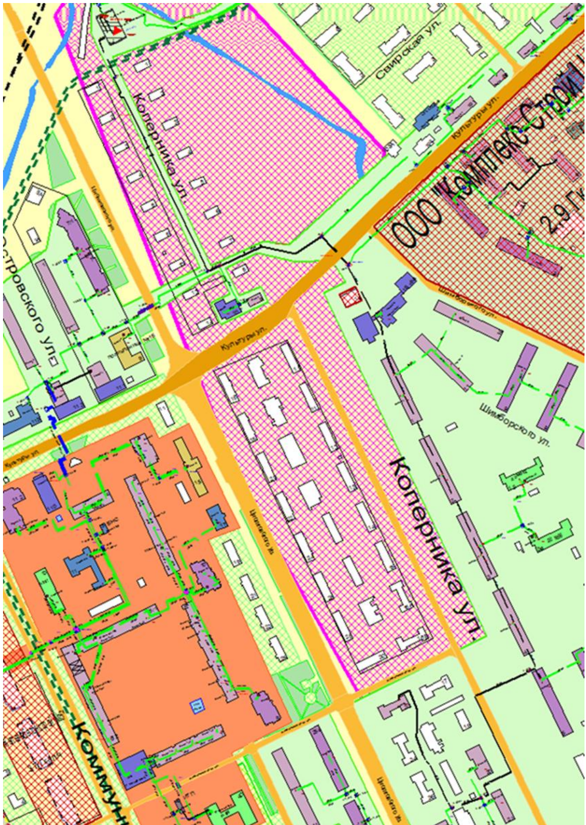
Рисунок 3.128 – Трассировка теплопровода от котельной АО «Теплоэнерго» «Циолковского, 5» по ул. Коперника, д. 1А до конечного потребителя «ПТ-Циол,32»
