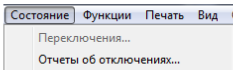
Рисунок 3.115 – Меню Состояние
