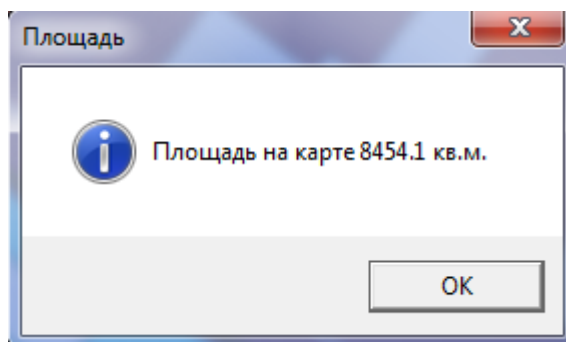
Рисунок 3.24 – Измерение площади
