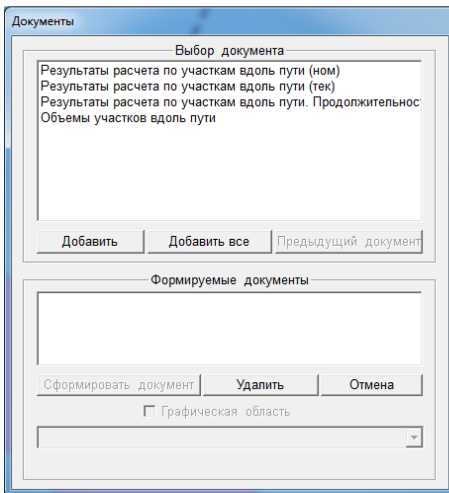
Рисунок 3.121 – Меню Документы
