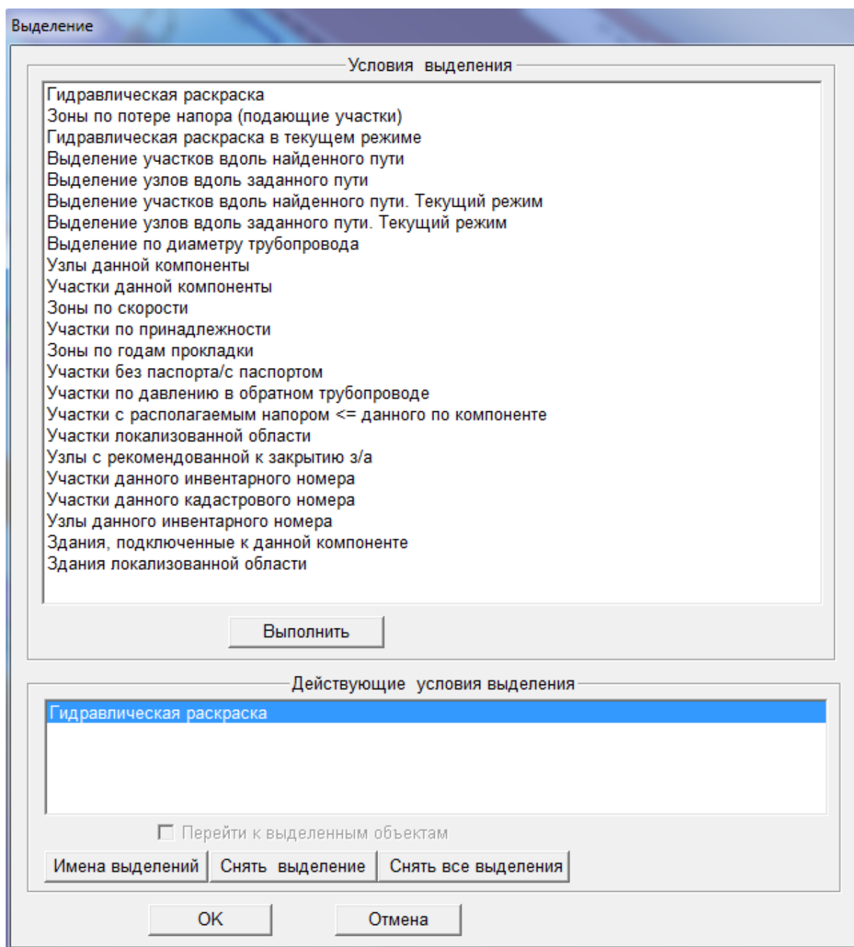
Рисунок 3.9 – Меню Выделение
