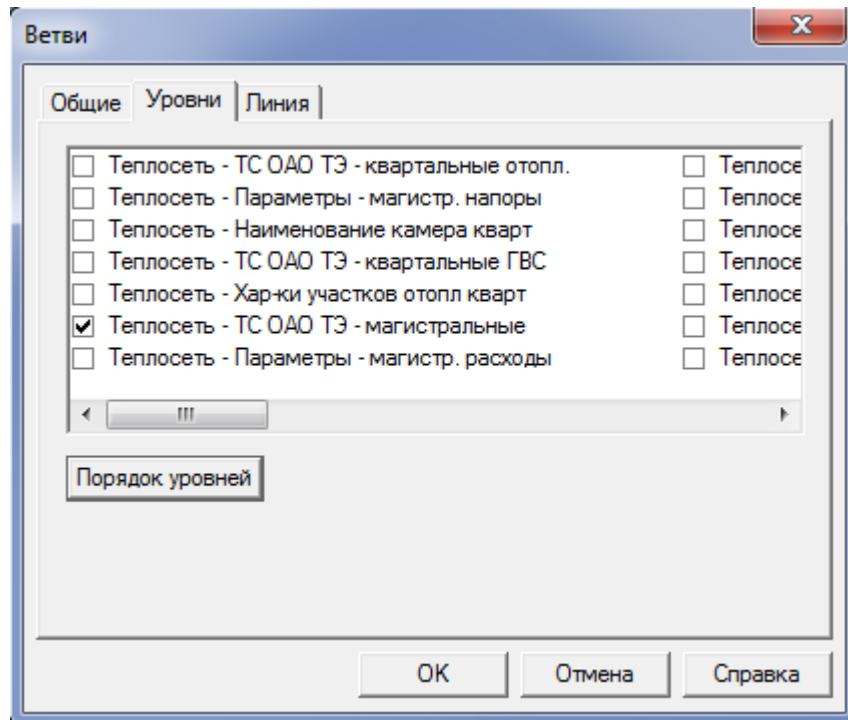
Рисунок 3.144 – Меню Уровни
