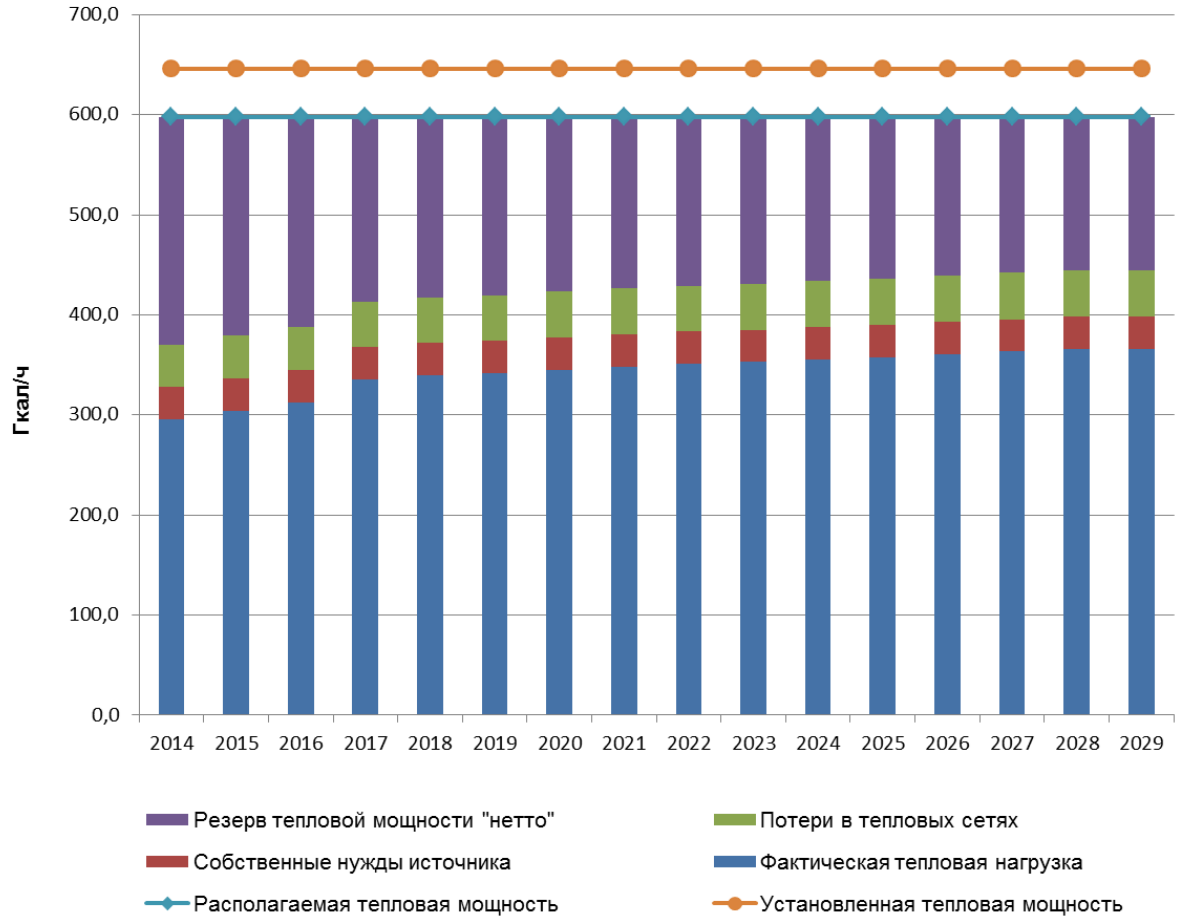
Рисунок 2.1 - Структура тепловых нагрузок и резервов тепловой мощности Сормовской ТЭЦ ПАО «Т Плюс»
