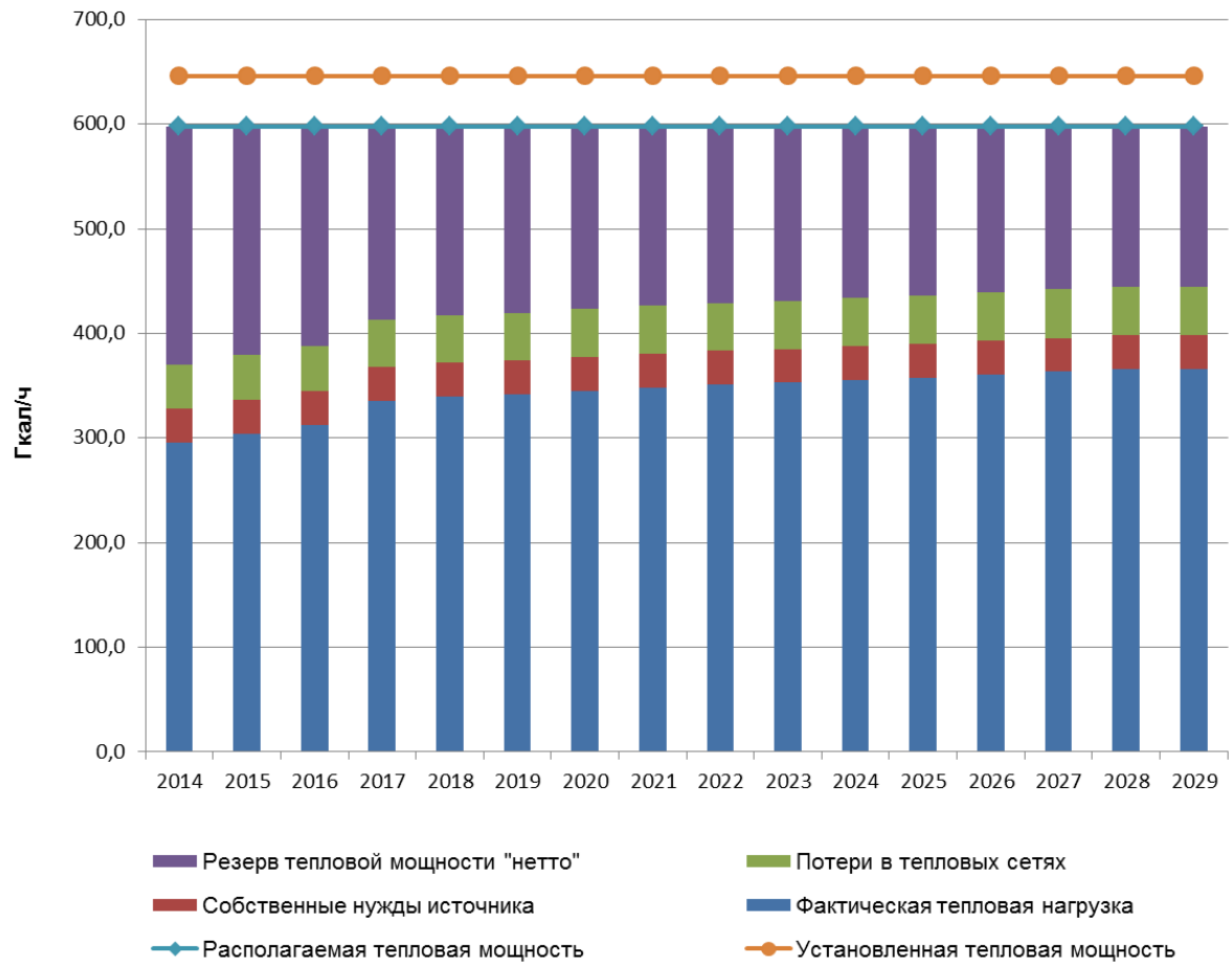
Рисунок 2.2 - Структура тепловых нагрузок и резервов тепловой мощности котельных, эксплуатируемых ОАО «Теплоэнерго»
