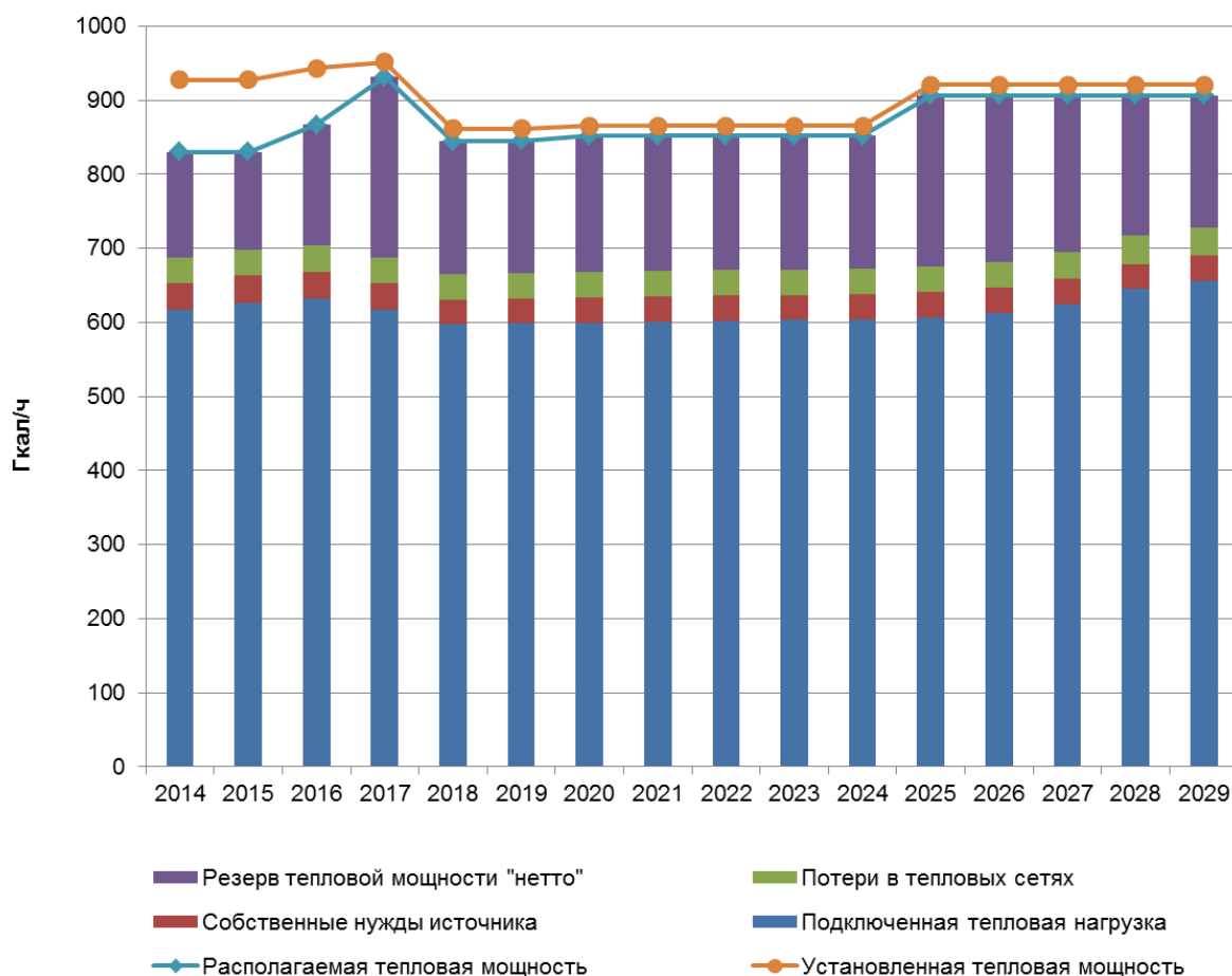
Рисунок 17.6 – Тепловые балансы по теплоисточникам прочих ТСО
