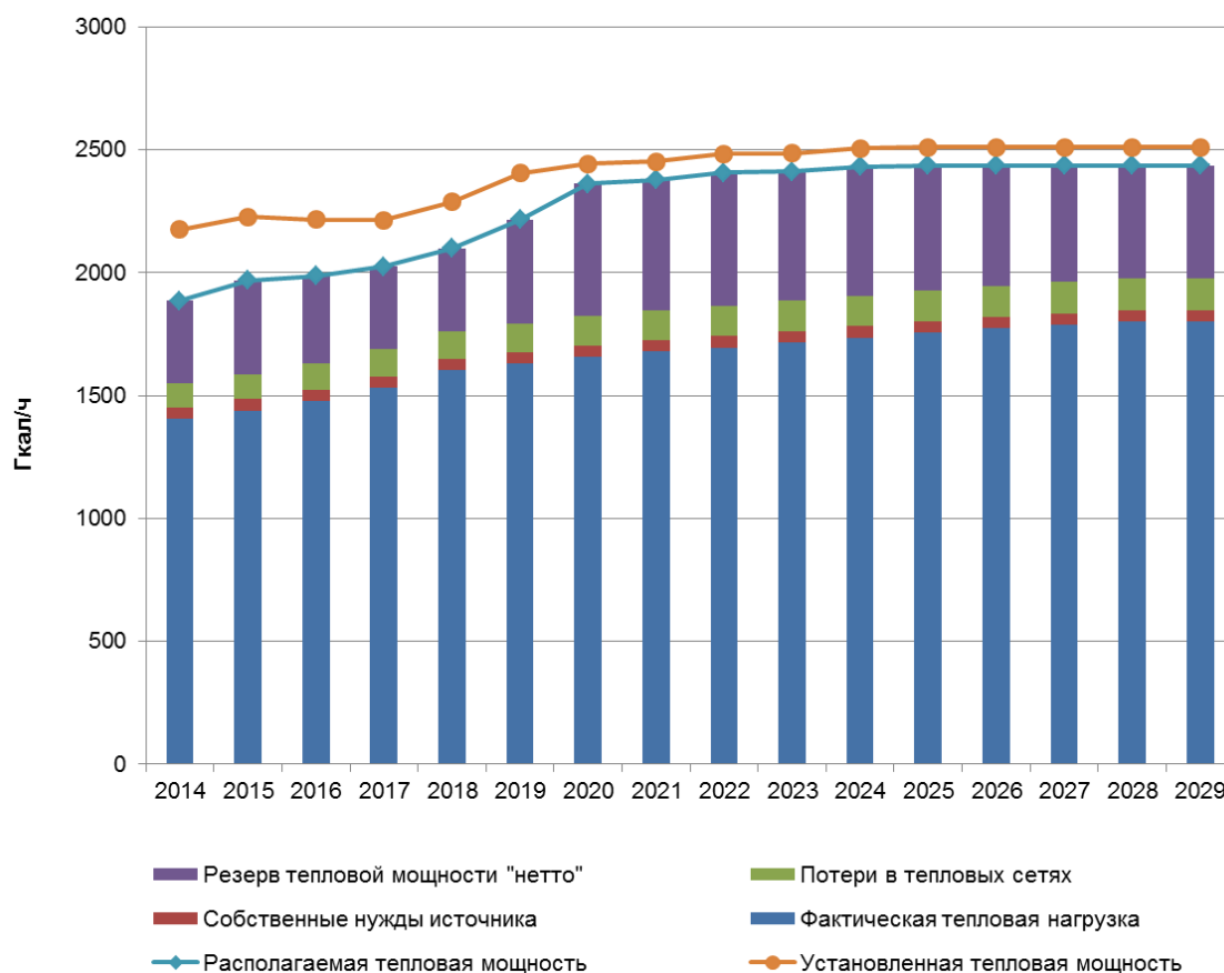
Рисунок 17.5 – Тепловые балансы по котельным ОАО «Теплоэнерго»
