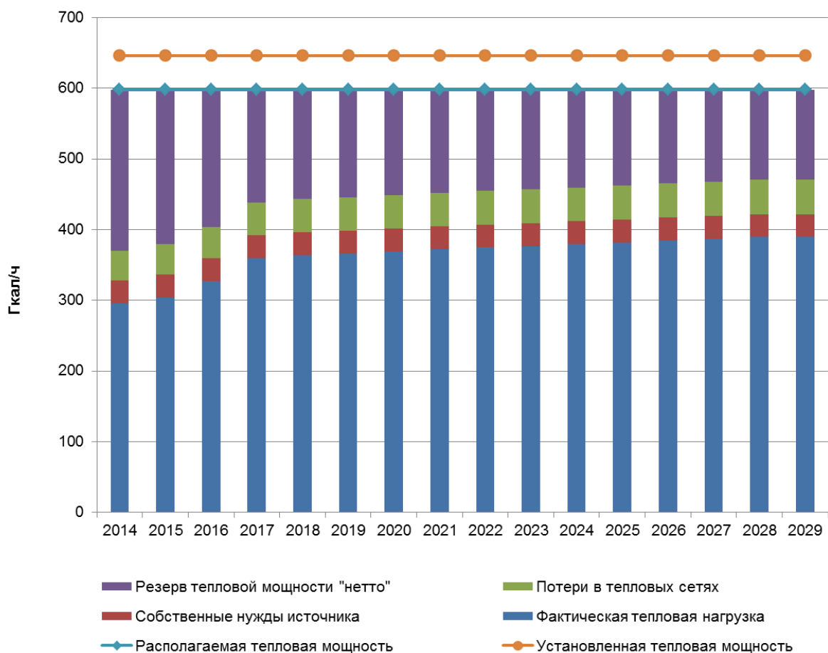
Рисунок 17.3 – Тепловые балансы по Сормовской ТЭЦ
