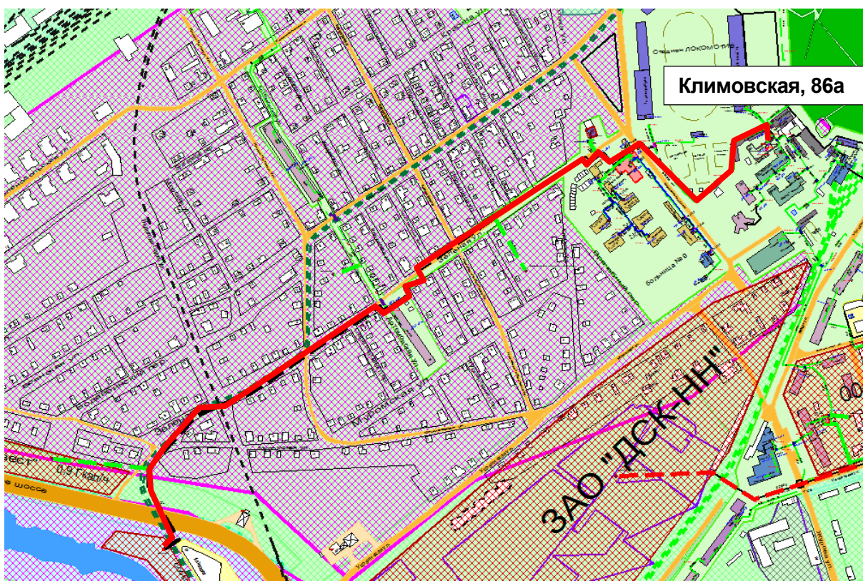
Рисунок 3.31 – Результат гидравлического расчета - расчетный путь теплоносителя от котельной Климовская, 86а до ПТ-ПП-2.227-2016
