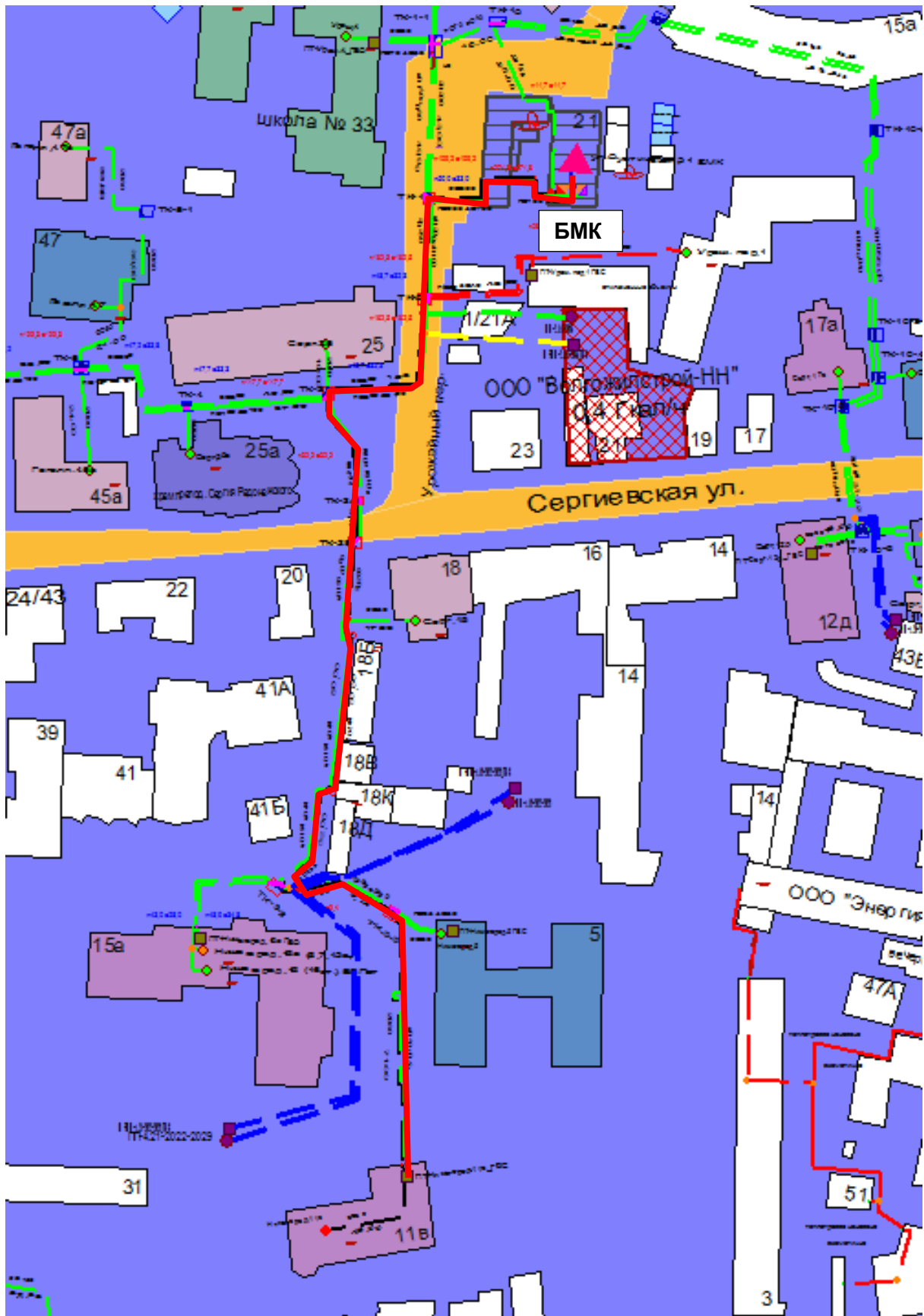
Рисунок 3.9 – Результат гидравлического расчета - расчетный путь теплоносителя от котельной Суетинская, 21 до ПТ-Нижгород, 11в
