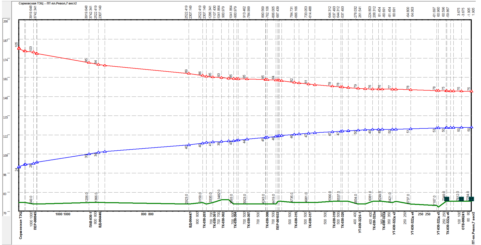
Рисунок 3.6 –Результат гидравлического расчета - график гидравлических режимов по пути теплоносителя от СТЭЦ до ПТ-пл.Револ,7 вест2
