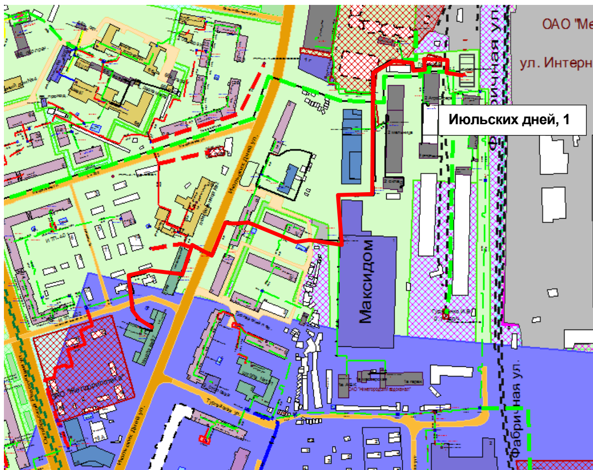
Рисунок 3.21 – Результат гидравлического расчета - расчетный путь теплоносителя от Июльских дней, 1 до ПТ-Июльские дни, 10 школа
