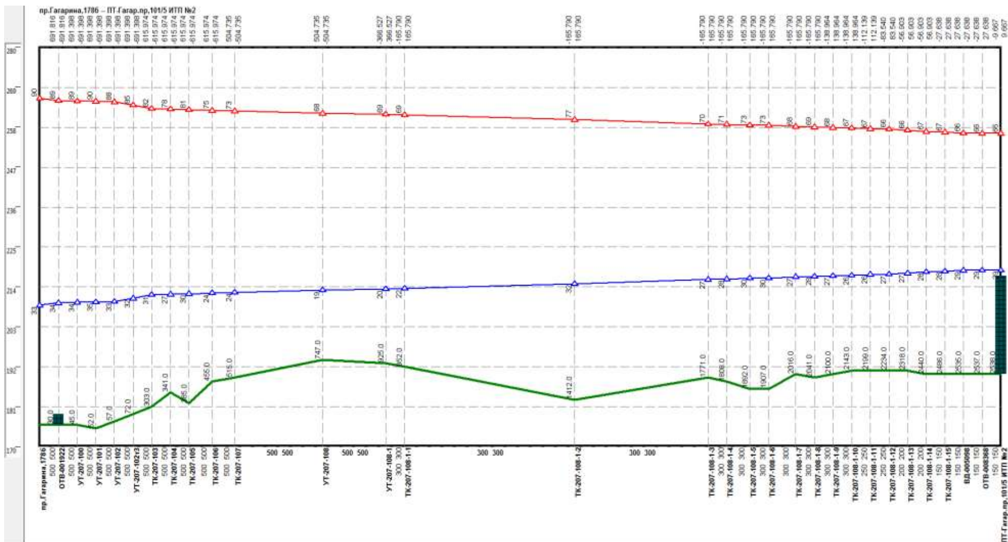
Рисунок 2.70 –Результат гидравлического расчета - график гидравлических режимов по пути теплоносителя от котельной пр. Гагарина, 1786 до ПТ-Гагар.пр.101/5 ИТП №2.
