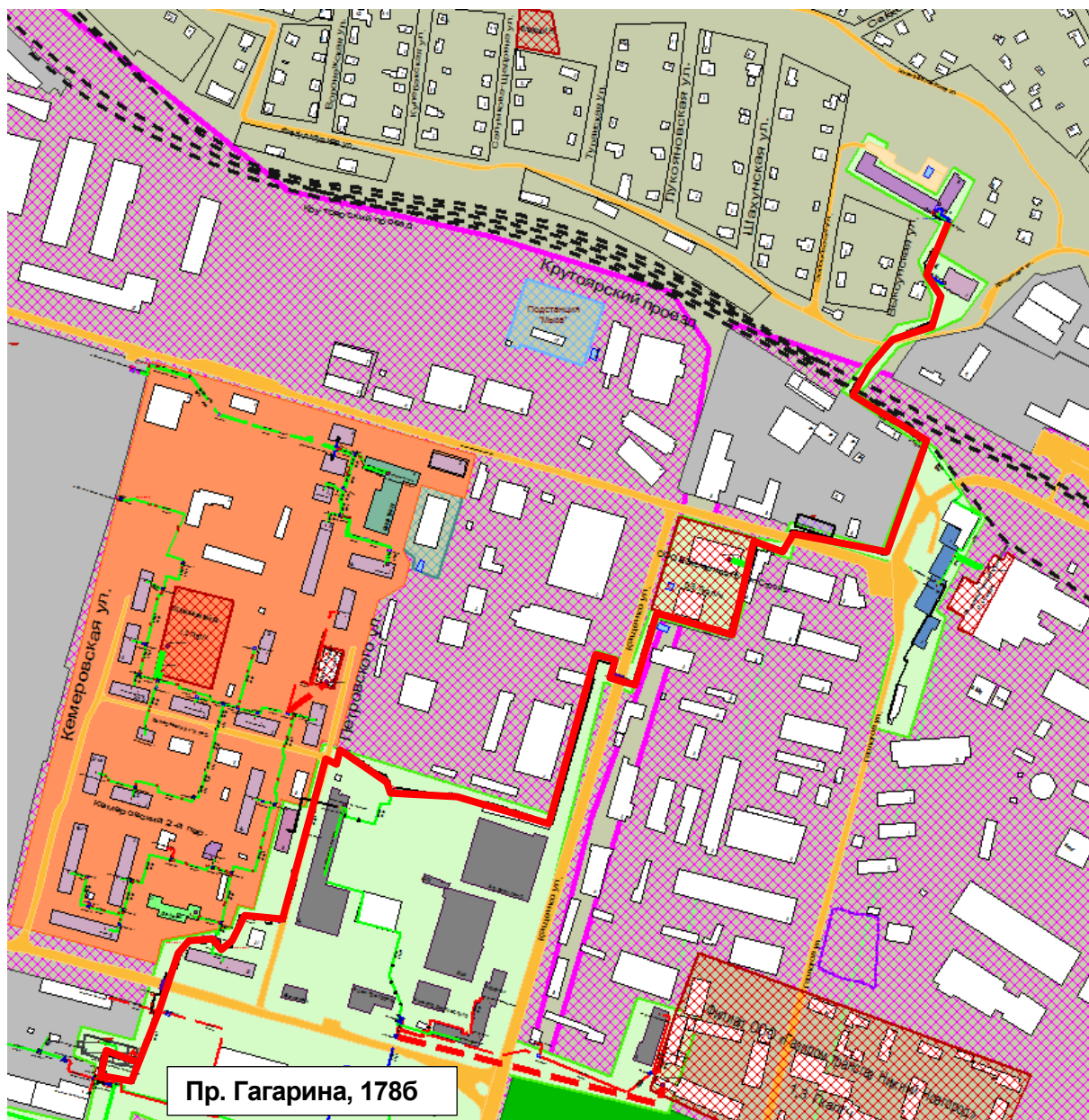
Рисунок 2.67 – Результат гидравлического расчета - расчетный путь теплоносителя от котельной пр. Гагарина, 1786 до ЦТП-706
