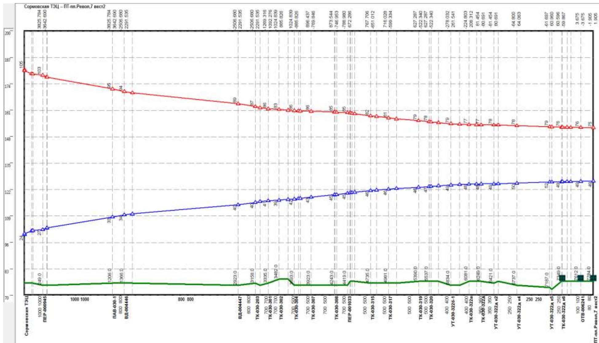
Рисунок 2.6 –Результат гидравлического расчета - график гидравлических режимов по пути теплоносителя от СТЭЦ до ПТ-пл.Революция, 7 вест 2.
