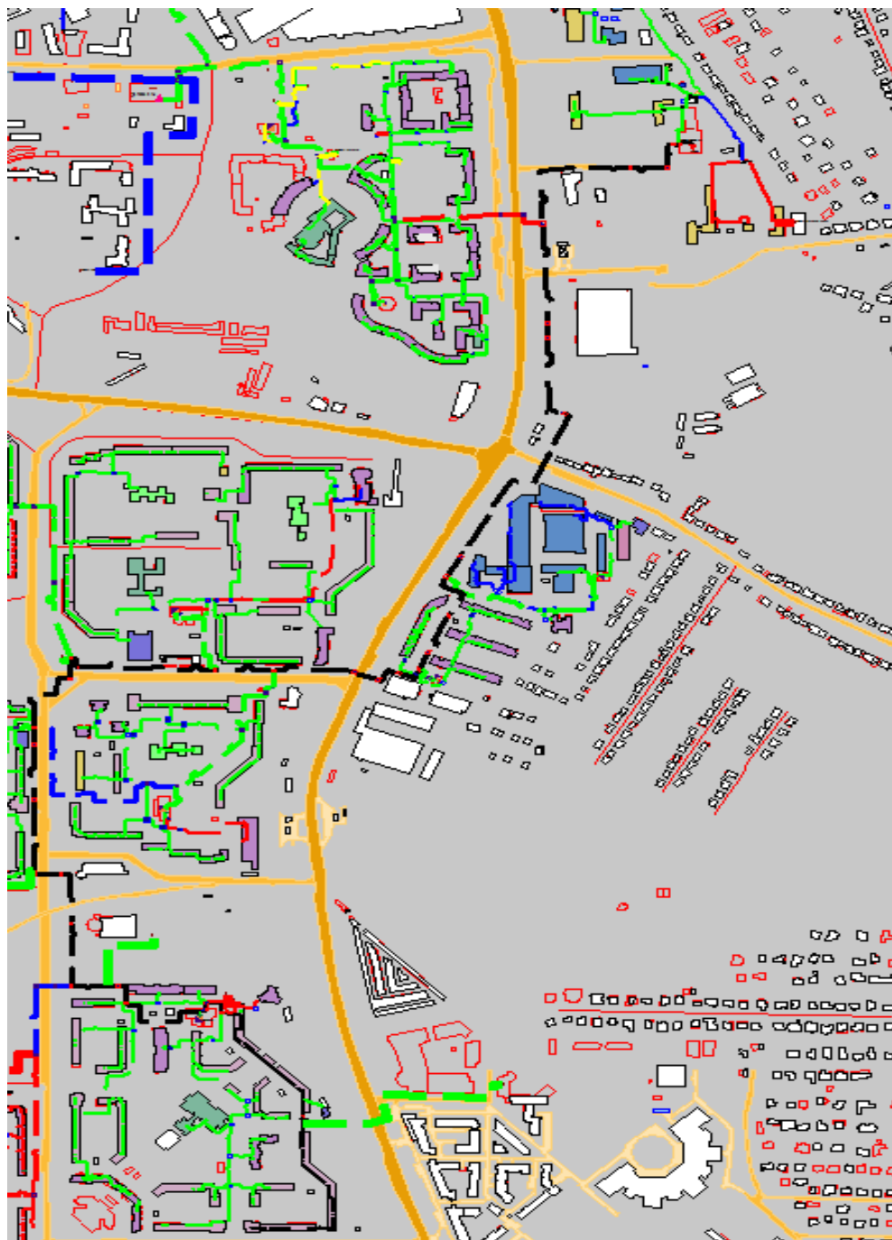
Рисунок 2.79 – Результат гидравлического расчета - расчетный путь теплоносителя от котельной ул. Родионова, 194б до ПТ-Богдан, 1 пр.
