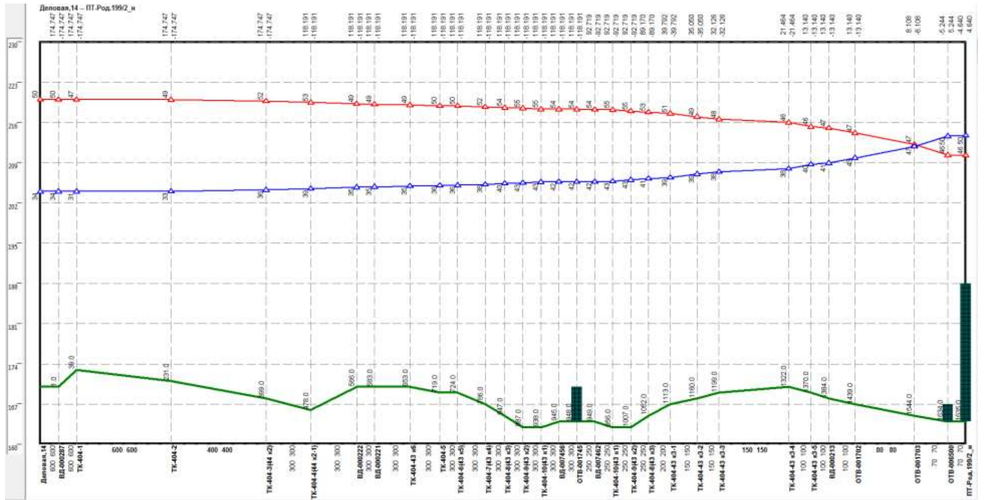
Рисунок 2.28 –Результат гидравлического расчета - график гидравлических режимов по пути теплоносителя от котельной Деловая, 14 до ПТ-Род.199/2_н
