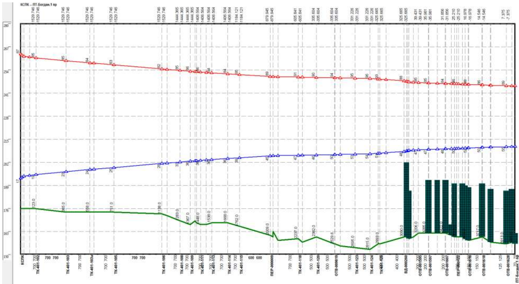
Рисунок 2.80 –Результат гидравлического расчета - график гидравлических режимов по пути теплоносителя от котельной ул. Родионова, 1946 до ПТ-Богдан, 1 пр.
