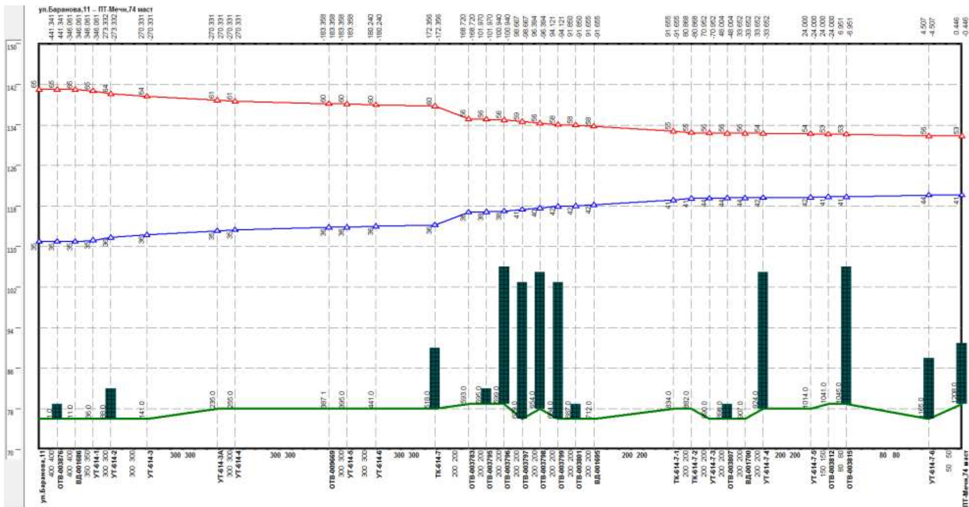
Рисунок 2.40 –Результат гидравлического расчета - график гидравлических режимов по пути теплоносителя от котельной Баранова, 11 до ПТ-Мечн,74 маст
