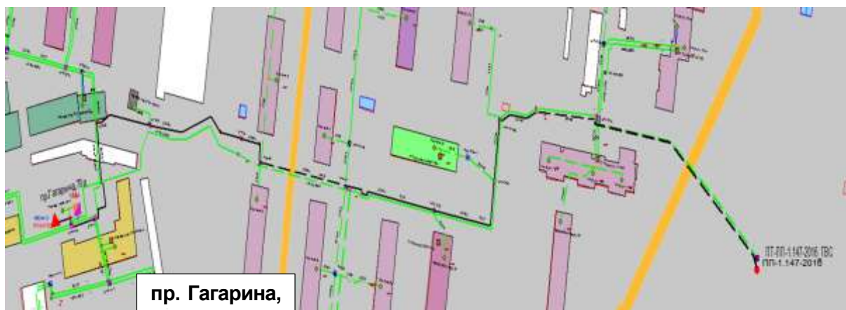
Рисунок 2.57 – Результат гидравлического расчета - расчетный путь теплоносителя от котельной пр. Гагарина, 70а до ПТ- ПП-1.147-2016
