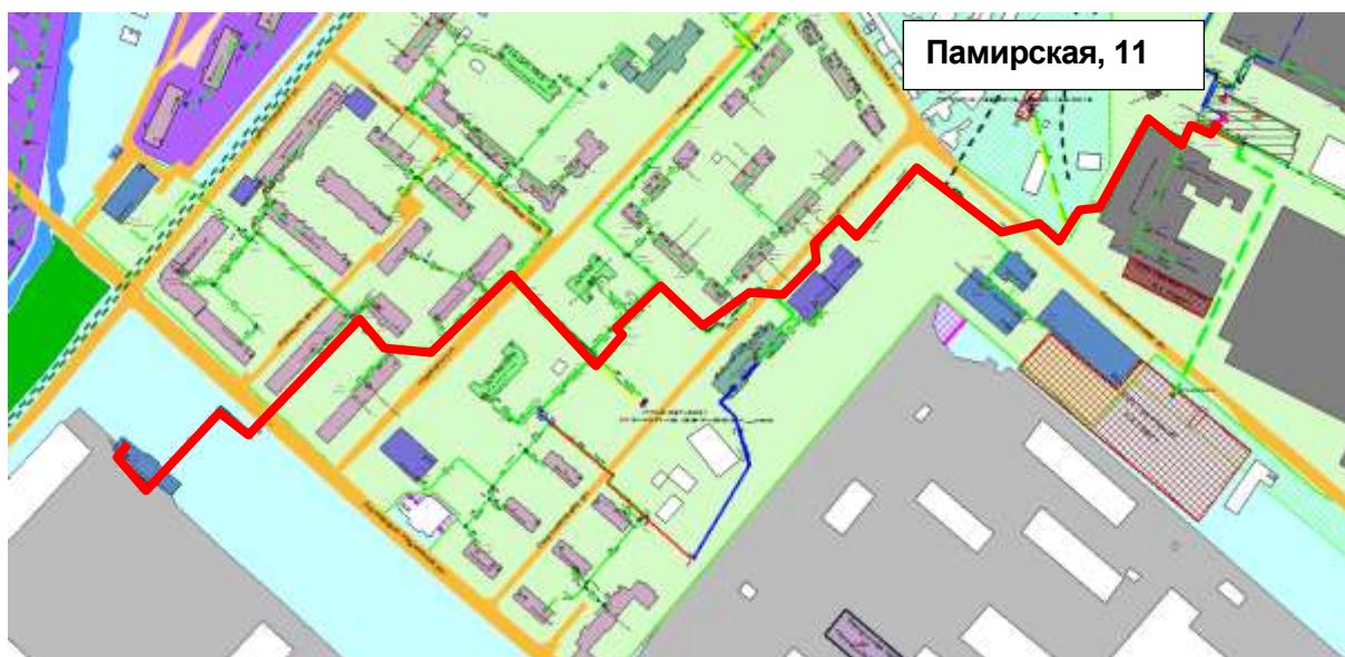
Рисунок 2.15 – Результат гидравлического расчета - расчетный путь теплоносителя от котельной Памирская, 11 до ПТ-Нахимова,3
