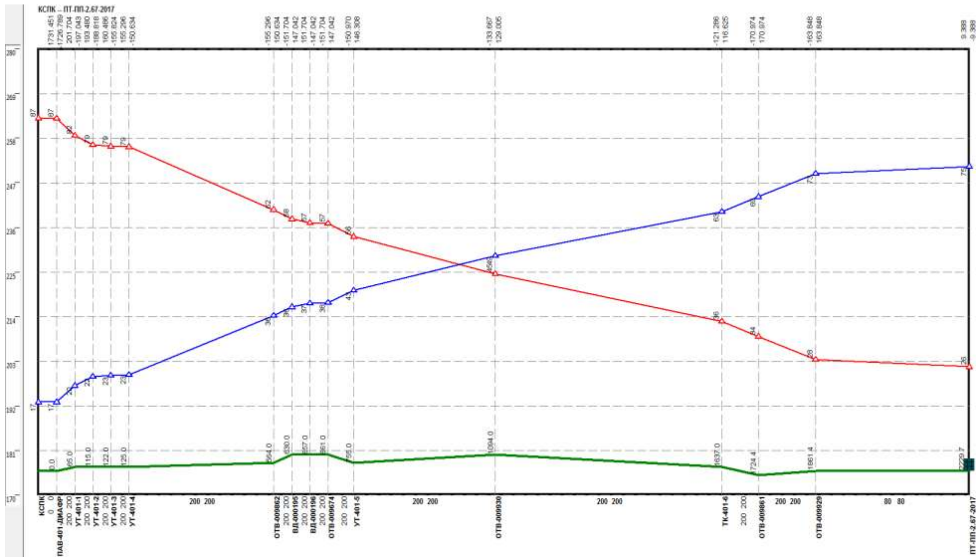
Рисунок 2.78 –Результат гидравлического расчета - график гидравлических режимов по пути теплоносителя от котельной ул. Родионова, 1946 до ПТ-ПП-2.67-2017
