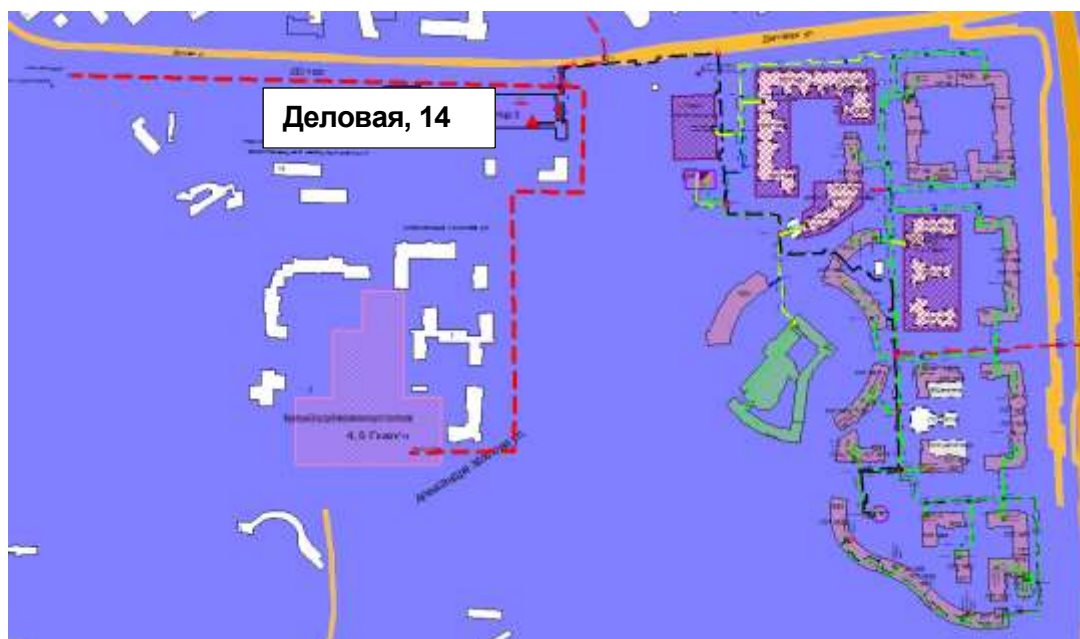
Рисунок 2.27 – Результат гидравлического расчета - расчетный путь теплоносителя от котельной Деловая, 14 до ПТ-Род.199/2_н
