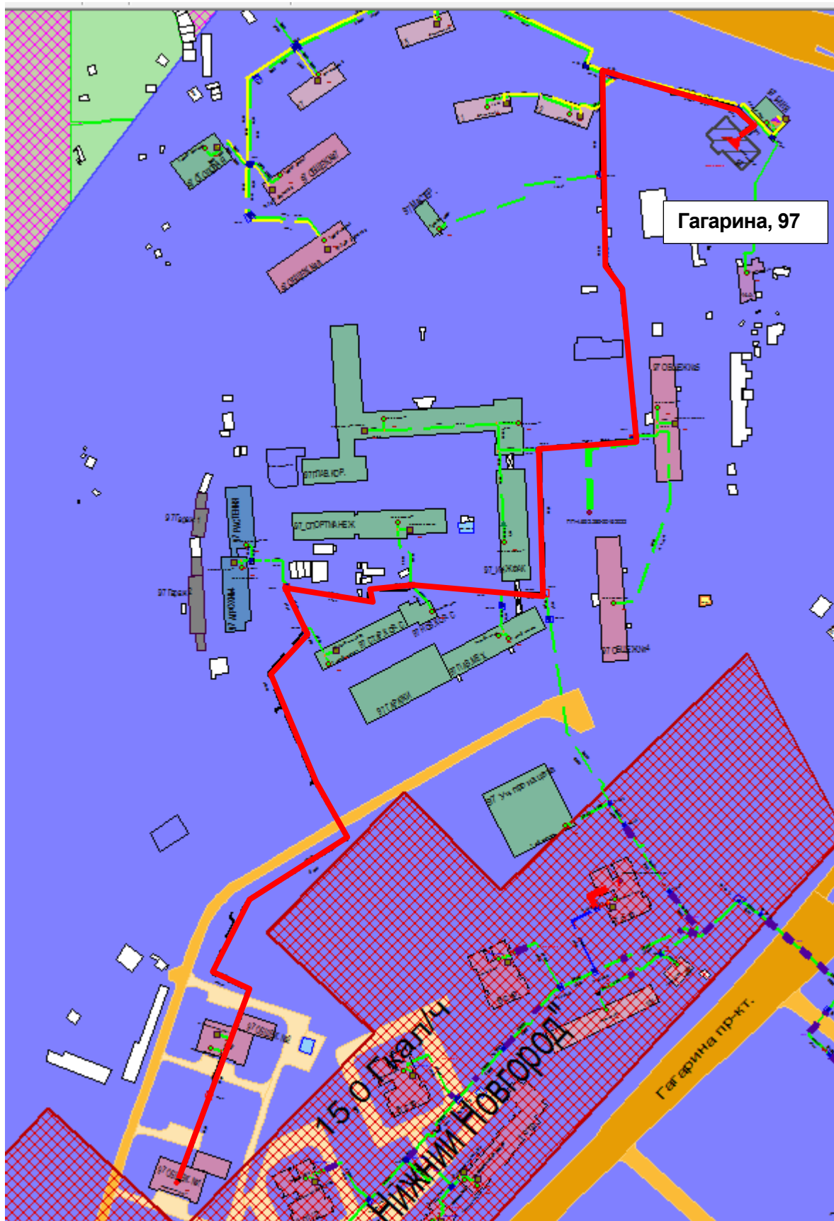
Рисунок 2.37 – Результат гидравлического расчета - расчетный путь теплоносителя от котельной пр. Гагарина, 97 до ПТ-Гагар,97 общ.№1
