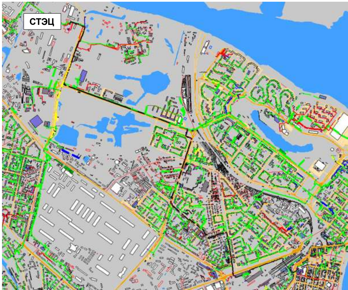
Рисунок 2.5 - Результат гидравлического расчета - расчетный путь теплоносителя от СТЭЦ до ПТ-Сорм.ш,20 э2
