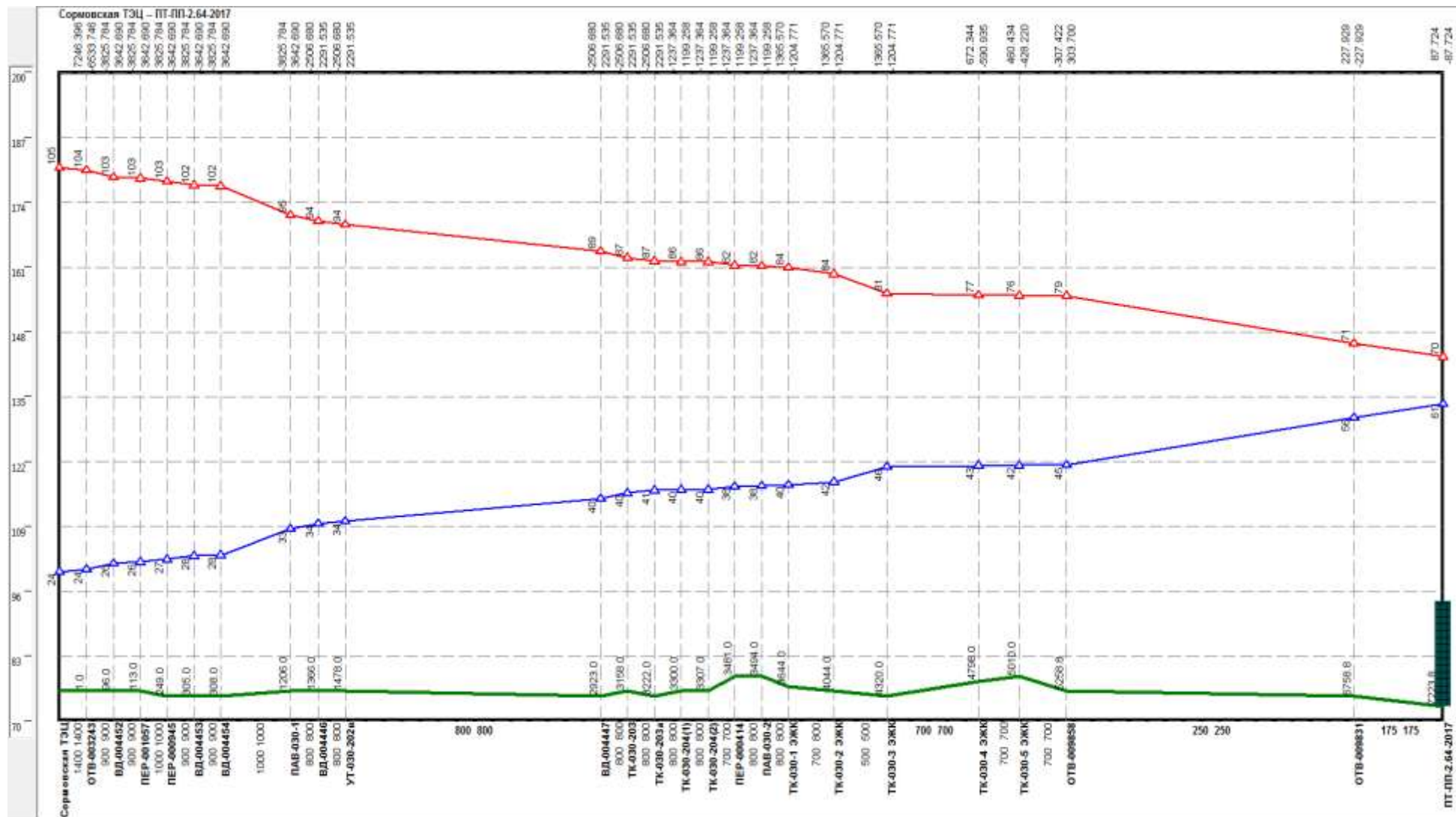
Рисунок 2.4 –Результат гидравлического расчета - график гидравлических режимов по пути теплоносителя от СТЭЦ до ПТ-ПП-2.64-2017
