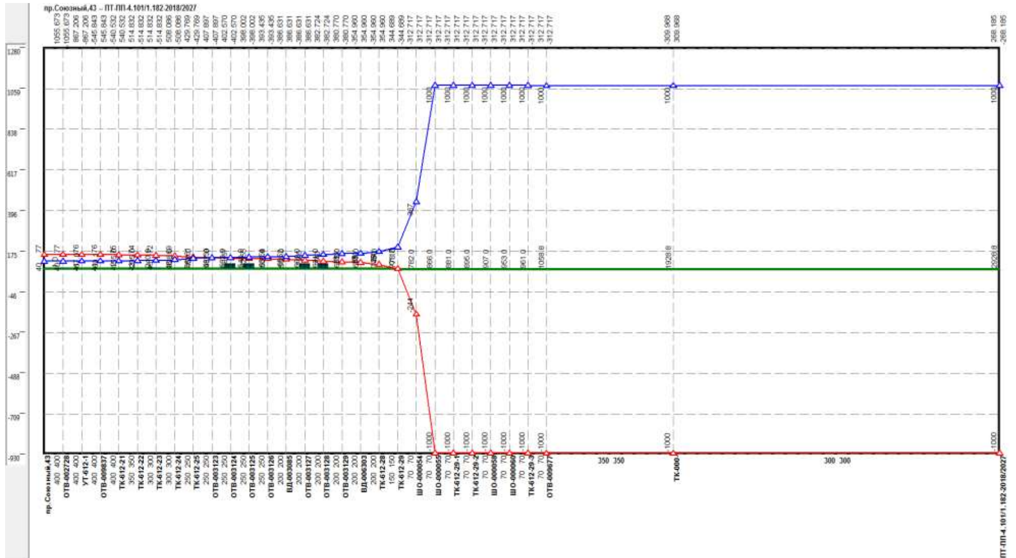
Рисунок 2.74 –Результат гидравлического расчета - график гидравлических режимов по пути теплоносителя от котельной пр. Союзный, 43 до ПТ-ПП-4.101/1.182-2018/2027
