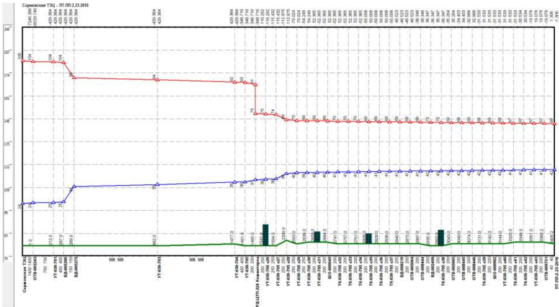
Рисунок 2.8 –Результат гидравлического расчета - график гидравлических режимов по пути теплоносителя от СТЭЦ до ПТ-ПП-2.23-2016
