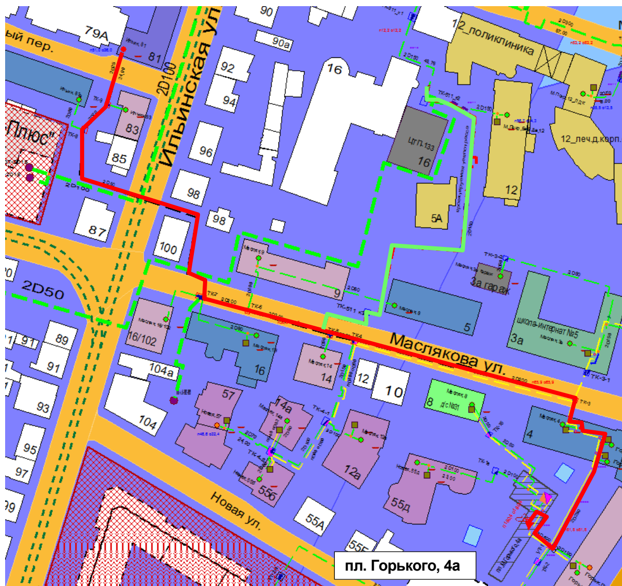
Рисунок 2.71 – Результат гидравлического расчета - расчетный путь теплоносителя от котельной пл. Горького, 4а до ПТ-Ильин,81
