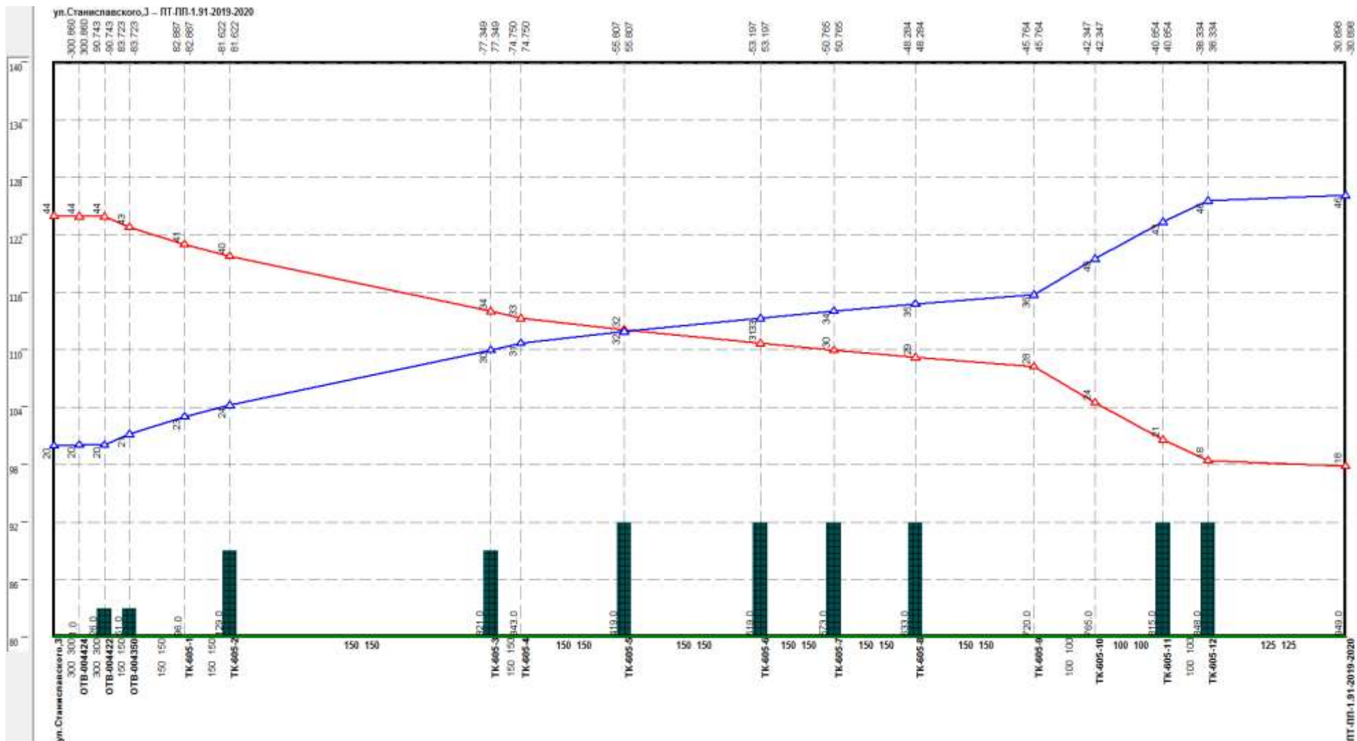
Рисунок 2.48 –Результат гидравлического расчета - график гидравлических режимов по пути теплоносителя от котельной Станиславского, 3 до ПТ- ПП-1,91-2019-2020.
