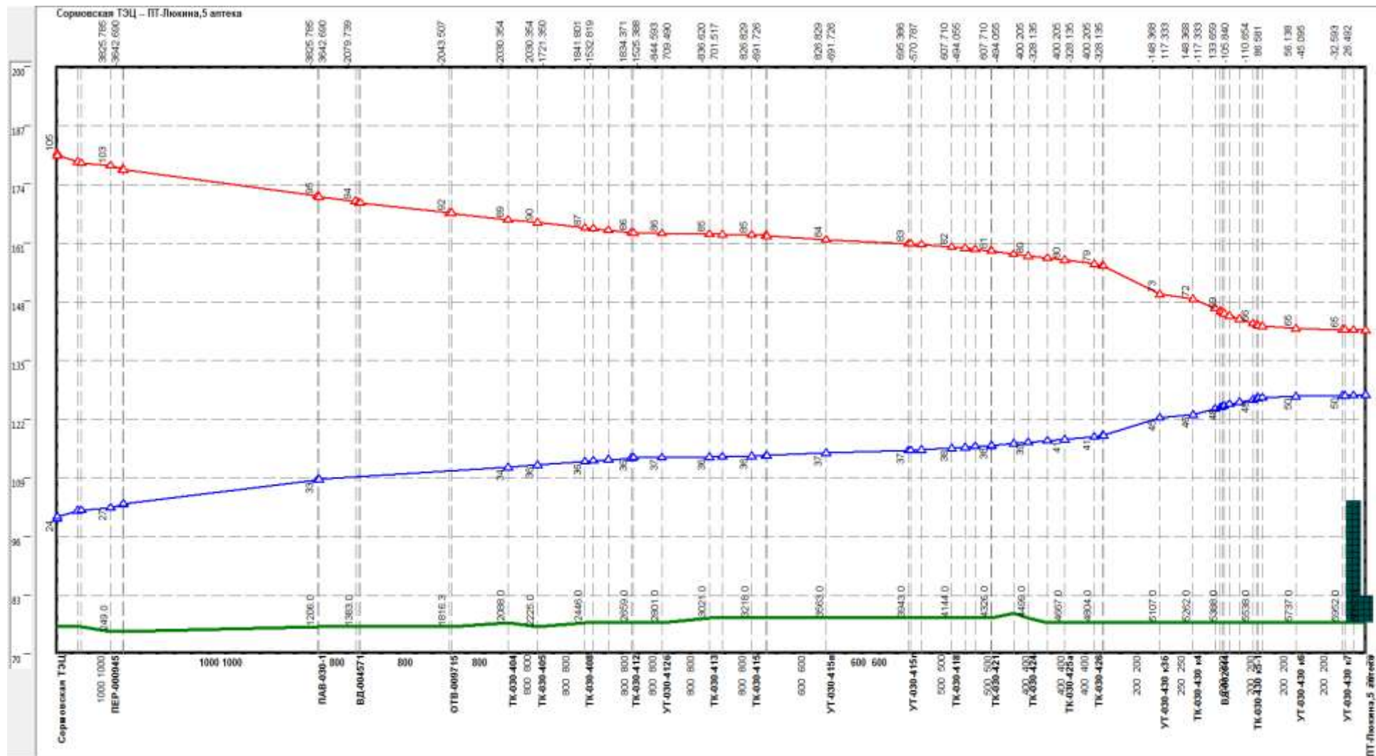
Рисунок 2.2 –Результат гидравлического расчета - график гидравлических режимов по пути теплоносителя от СТЭЦ до ПТ-Люкина,5 аптека
