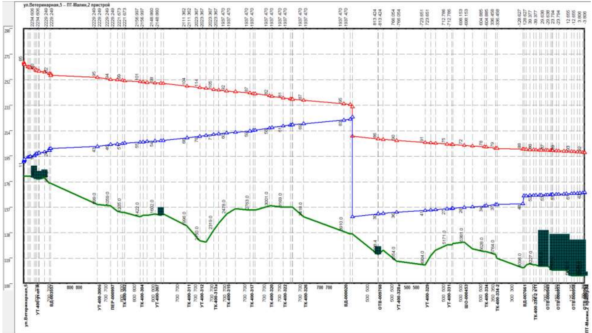
Рисунок 2.60 –Результат гидравлического расчета - график гидравлических режимов по пути теплоносителя от котельной НТЦ до ПТ-Малин,2 пристрой
