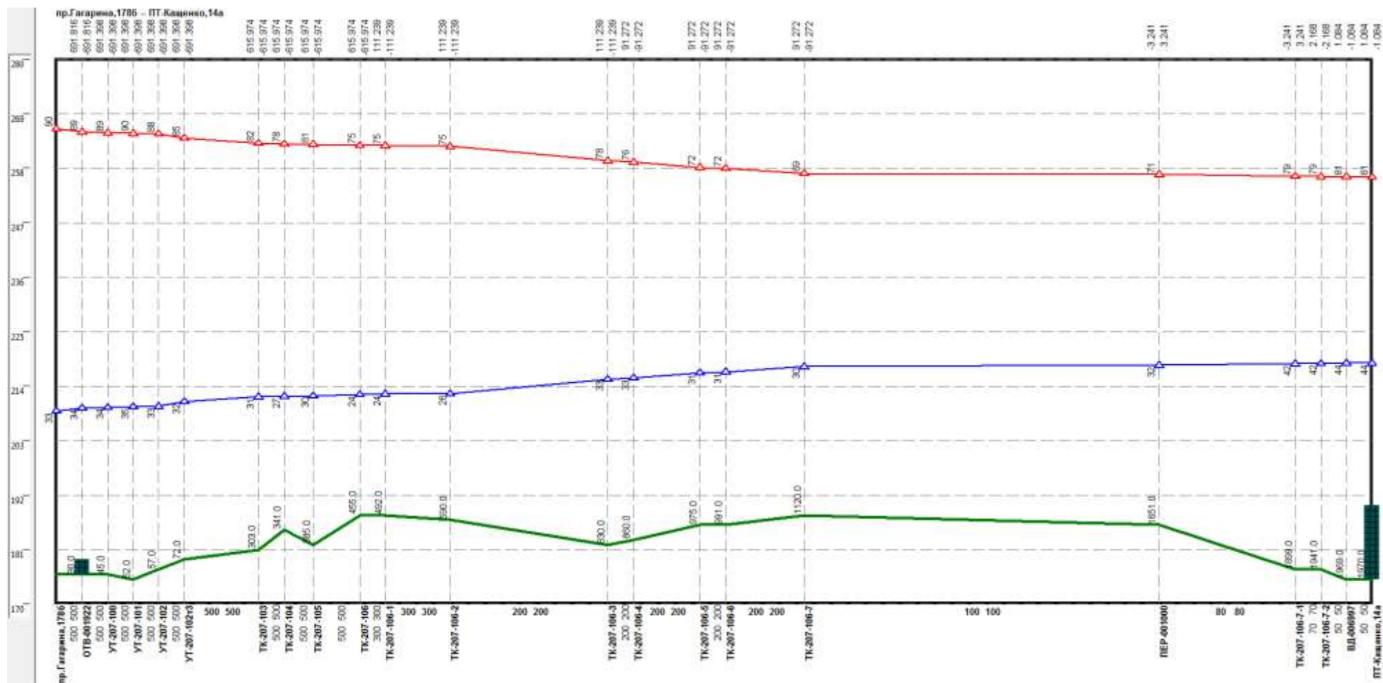
Рисунок 2.66 –Результат гидравлического расчета - график гидравлических режимов по пути теплоносителя от котельной пр. Гагарина, 1786 до ПТ-Кащенко,14а
