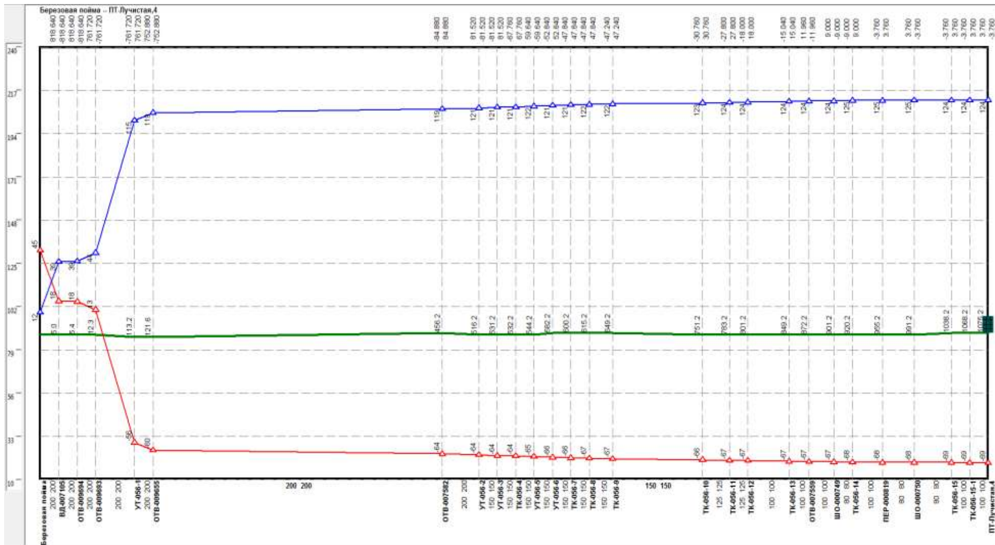
Рисунок 2.26 –Результат гидравлического расчета - график гидравлических режимов по пути теплоносителя от котельной Березовая пойма до ПТ-Лучистая, 4
