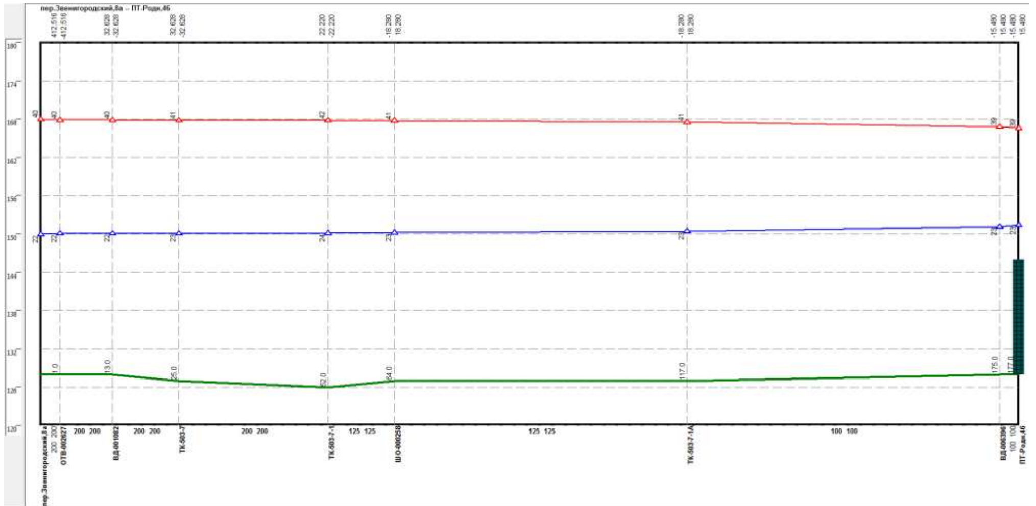
Рисунок 2.54 –Результат гидравлического расчета - график гидравлических режимов по пути теплоносителя от котельной пер. Звенигородский до ПТ-Родн,46
