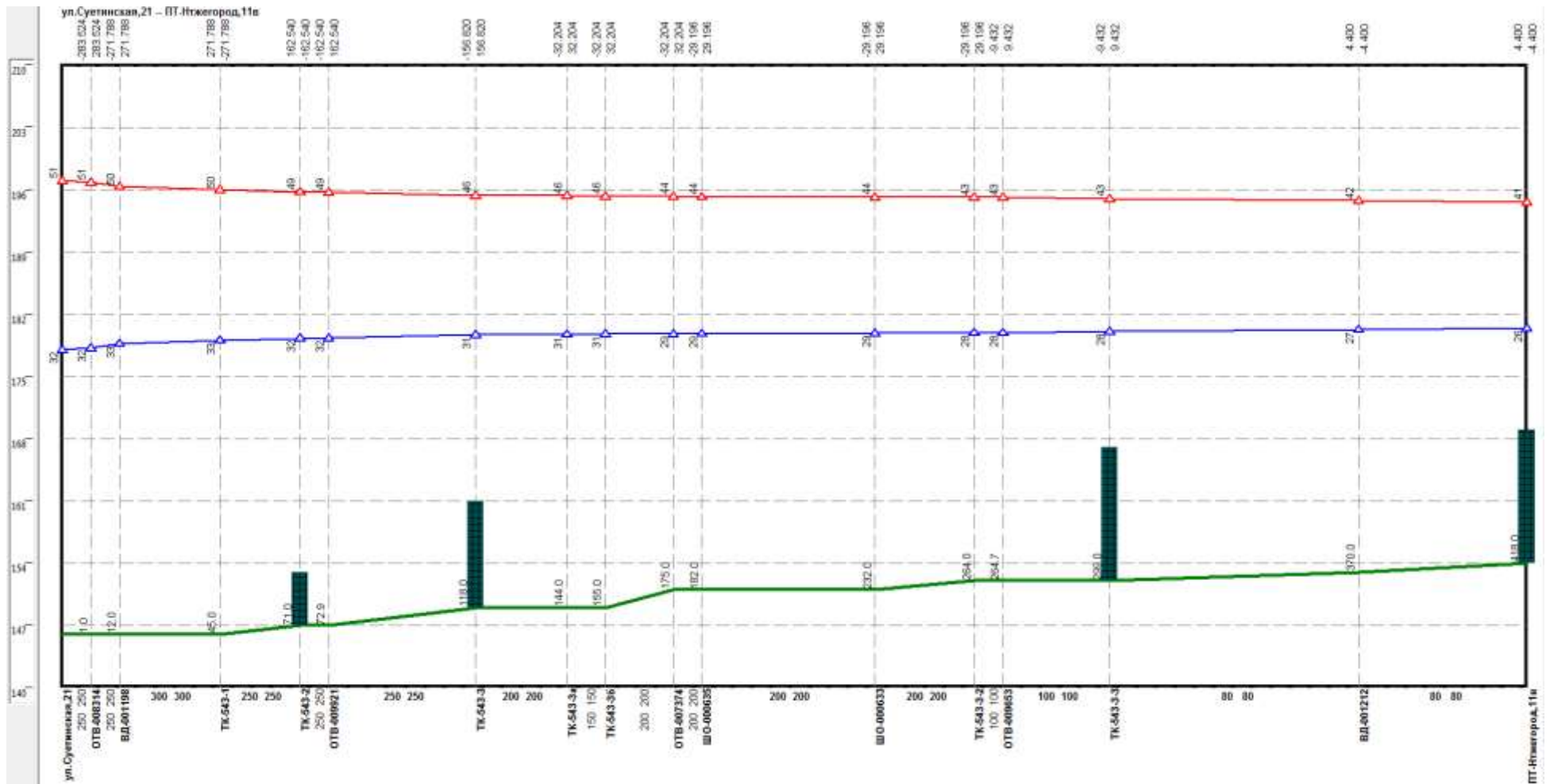
Рисунок 2.10 –Результат гидравлического расчета - график гидравлических режимов по пути теплоносителя от котельной Суетенская, 21 до ПТ-Нтжегород,11в
