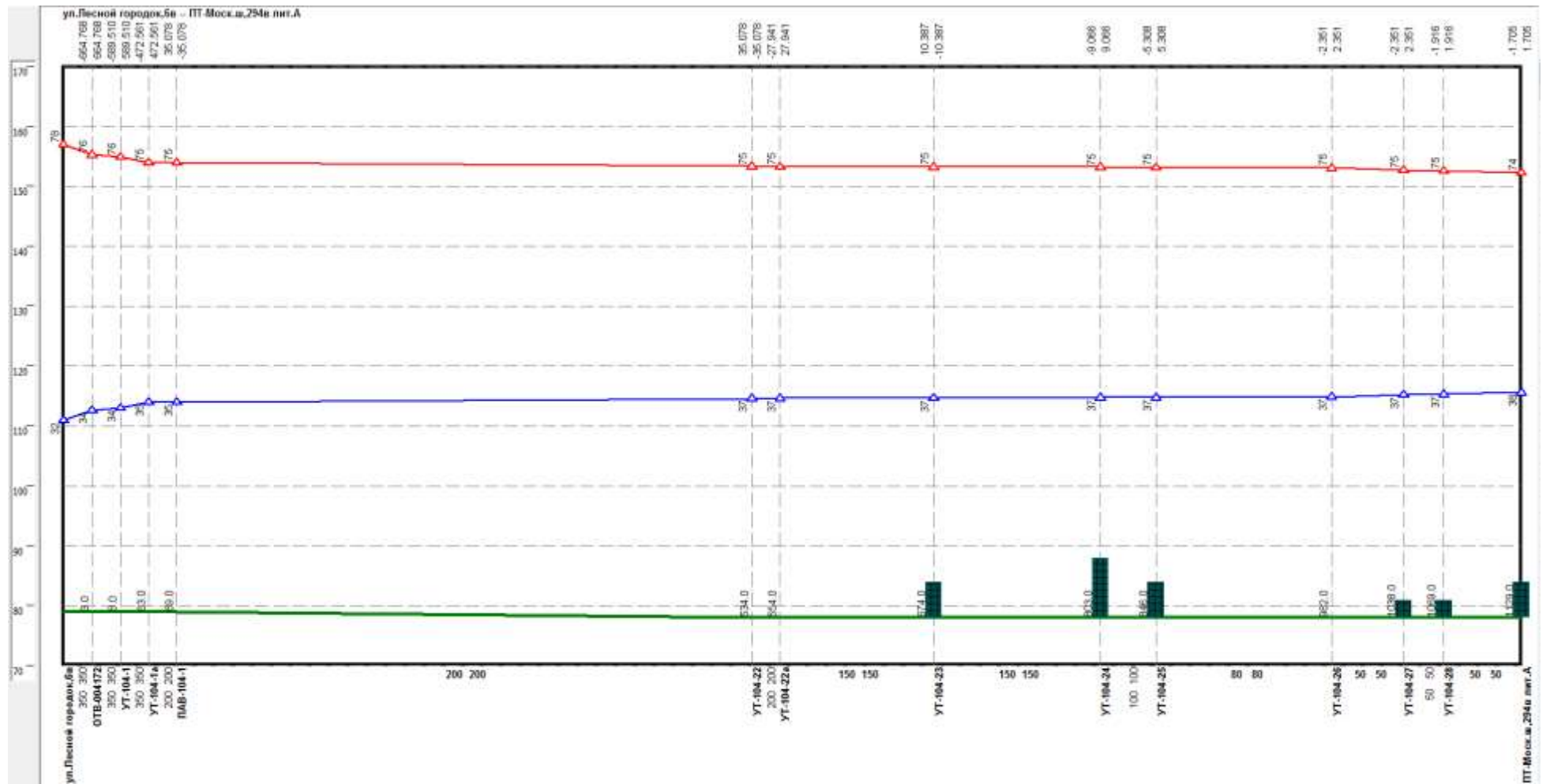
Рисунок 2.20 –Результат гидравлического расчета - график гидравлических режимов по пути теплоносителя от Лесной городок, б/в до ПТ-Моск.ш.294в лит.А
