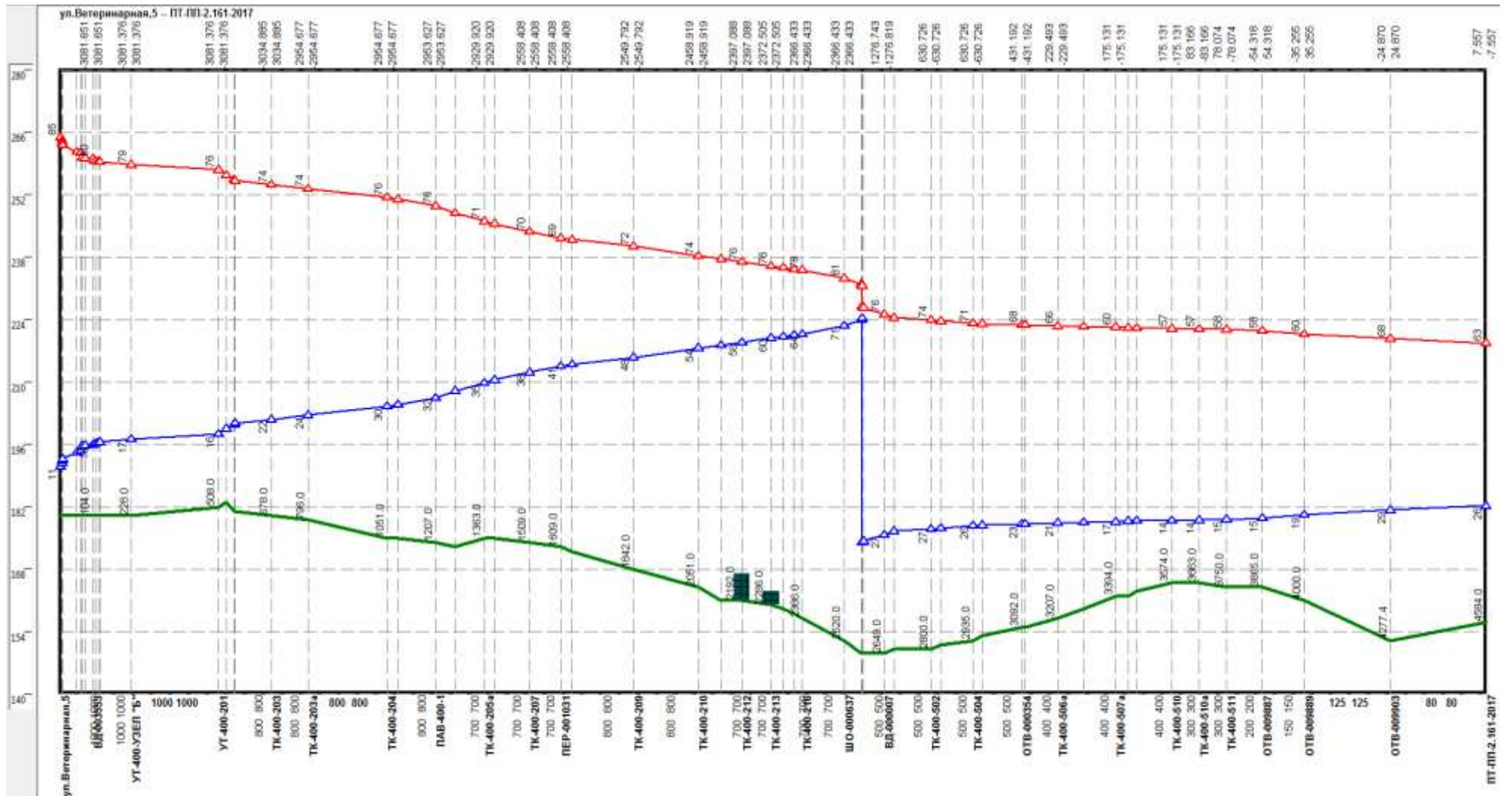
Рисунок 2.64 –Результат гидравлического расчета - график гидравлических режимов по пути теплоносителя от котельной НТЦ до ОТВ-009903
