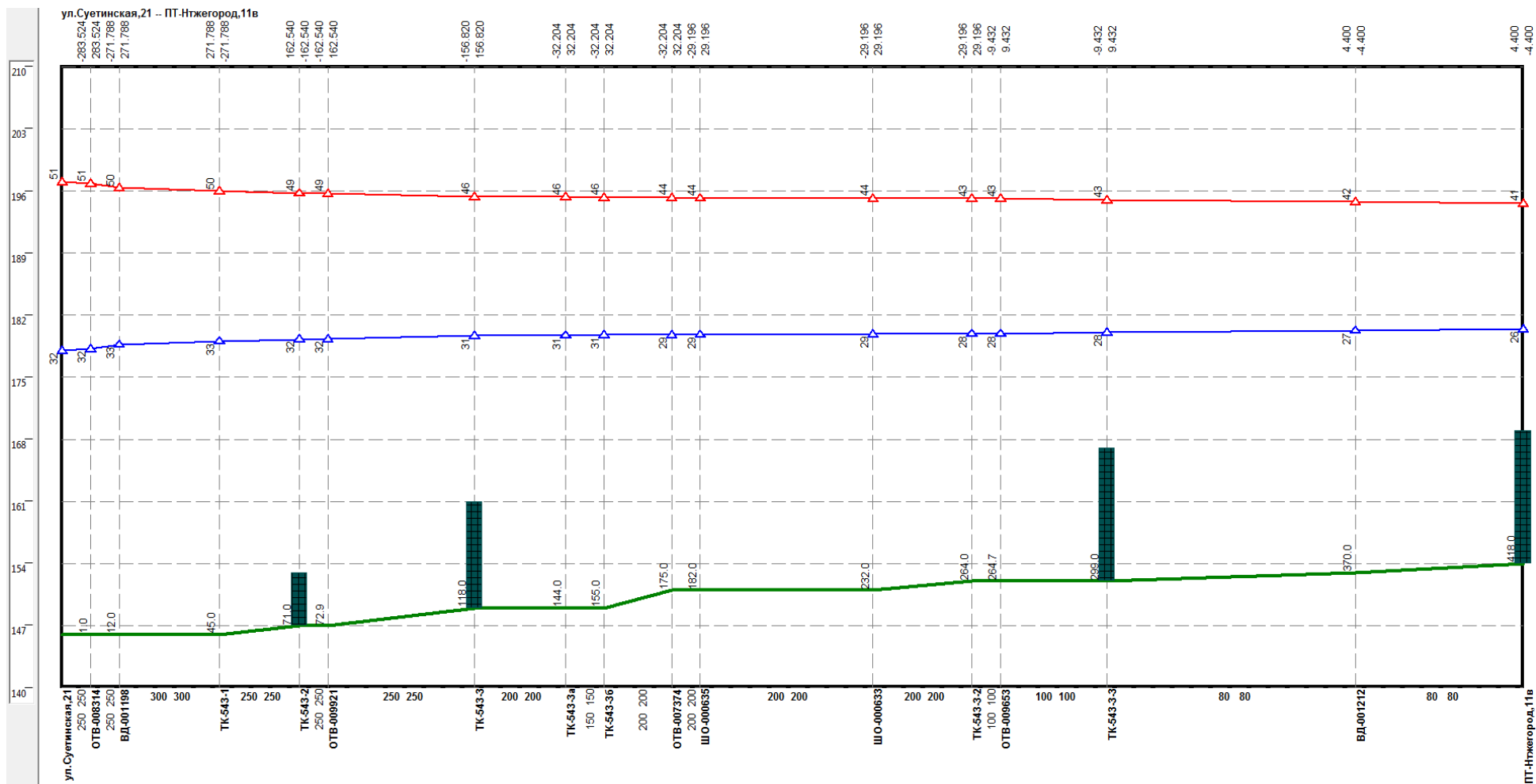
Рисунок 2.10 –Результат гидравлического расчета - график гидравлических режимов по пути теплоносителя от котельной Суетинская, 21 до ПТ-Нтжегород,11в
