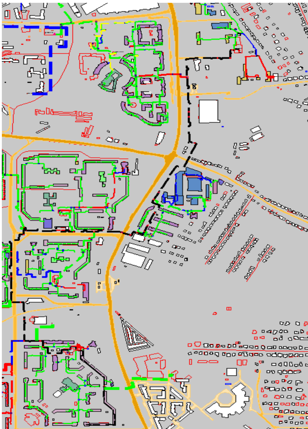
Рисунок 2.79 – Результат гидравлического расчета - расчетный путь теплоносителя от котельной ул. Родионова, 1946 до ПТ-Богдан, 1 пр.
