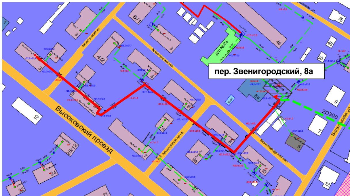
Рисунок 2.51 – Результат гидравлического расчета - расчетный путь теплоносителя от котельной пер. Звенигородский, 8а до ПТ-Выс.пр,3 в1
