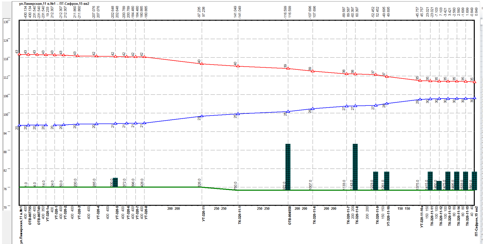
Рисунок 2.14 –Результат гидравлического расчета - график гидравлических режимов по пути теплоносителя от котельной Памирская, 11 до ПТ-Сафрон,15 вв2
