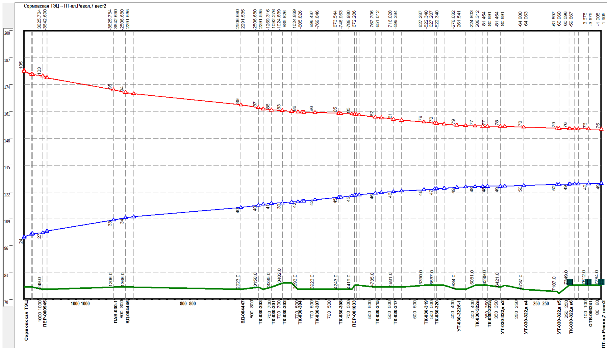
Рисунок 2.6 –Результат гидравлического расчета - график гидравлических режимов по пути теплоносителя от СТЭЦ до ПТ-пл.Револ,7 вест2.
