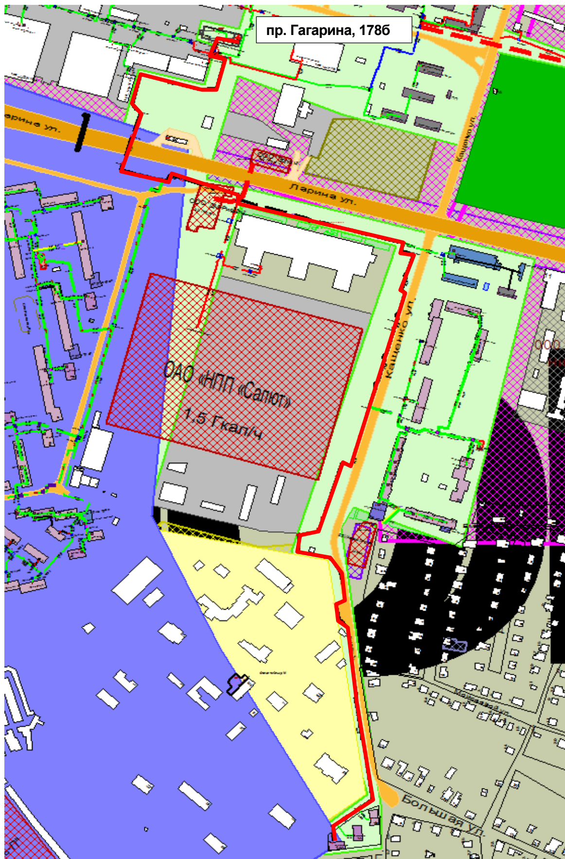
Рисунок 2.65 – Результат гидравлического расчета - расчетный путь теплоносителя от котельной пр. Гагарина, 1786 до ПТ-Кашенко,14а
