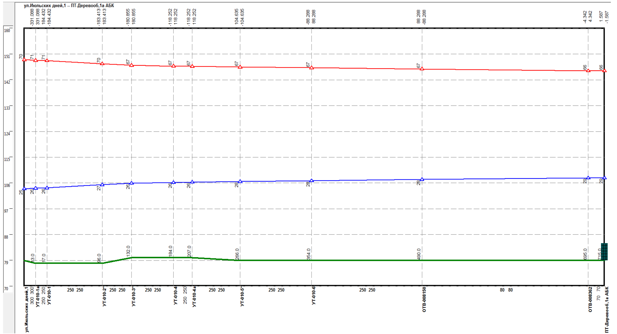
Рисунок 2.34 –Результат гидравлического расчета - график гидравлических режимов по пути теплоносителя от Июльских дней, 1 до ПТ-Деревооб, 1а АБК
