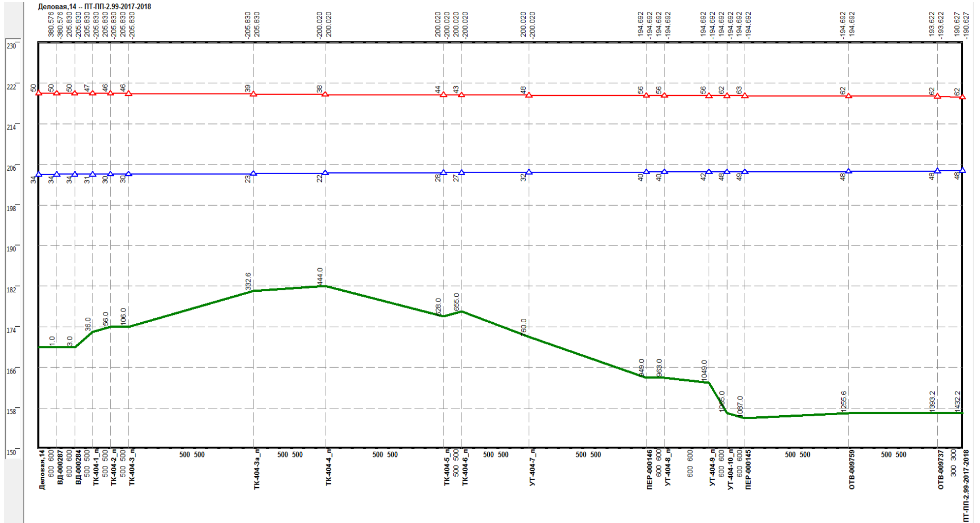
Рисунок 2.30 –Результат гидравлического расчета - график гидравлических режимов по пути теплоносителя от котельной Деловая, 14 до ПТ-ПП-2.99-2017-2018.
