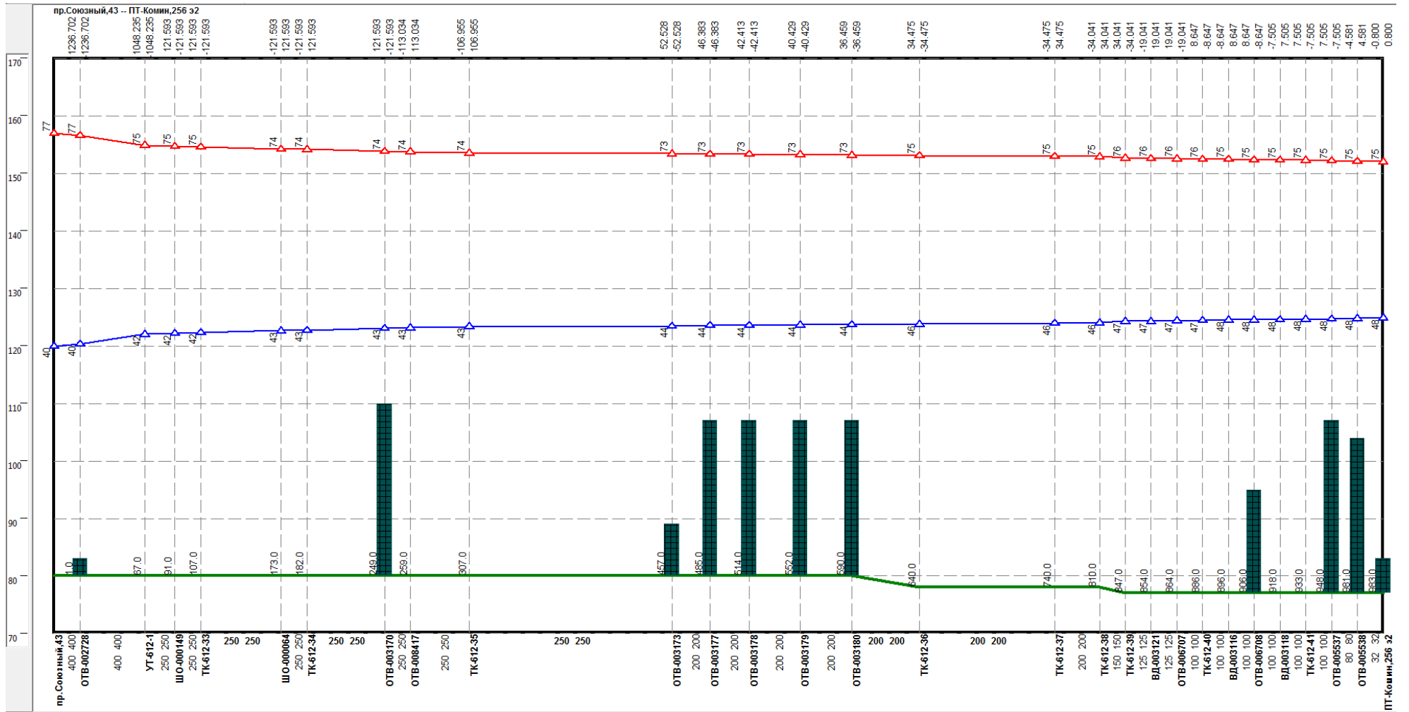
Рисунок 0.48 –Результат гидравлического расчета - график гидравлических режимов по пути теплоносителя от котельной пр. Союзный, 43 до ПТ-Комин,256 э2
