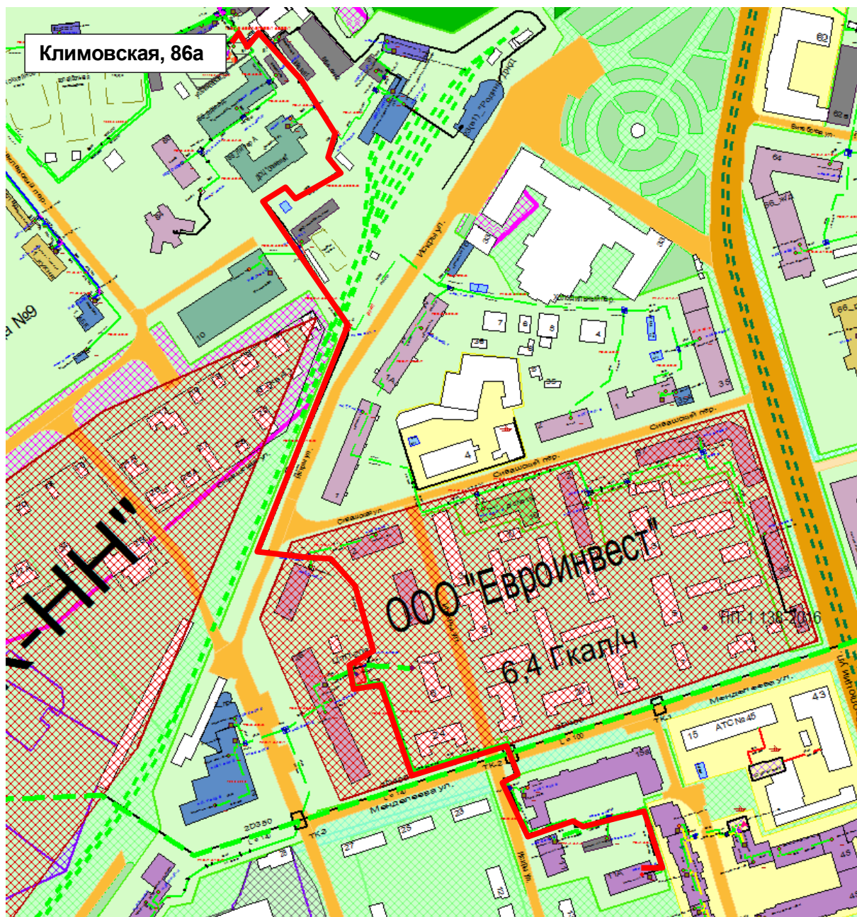
Рисунок 0.102 – Результат гидравлического расчета - расчетный путь теплоносителя от котельной Климовская, 86а до ПТ-Искры,11а
