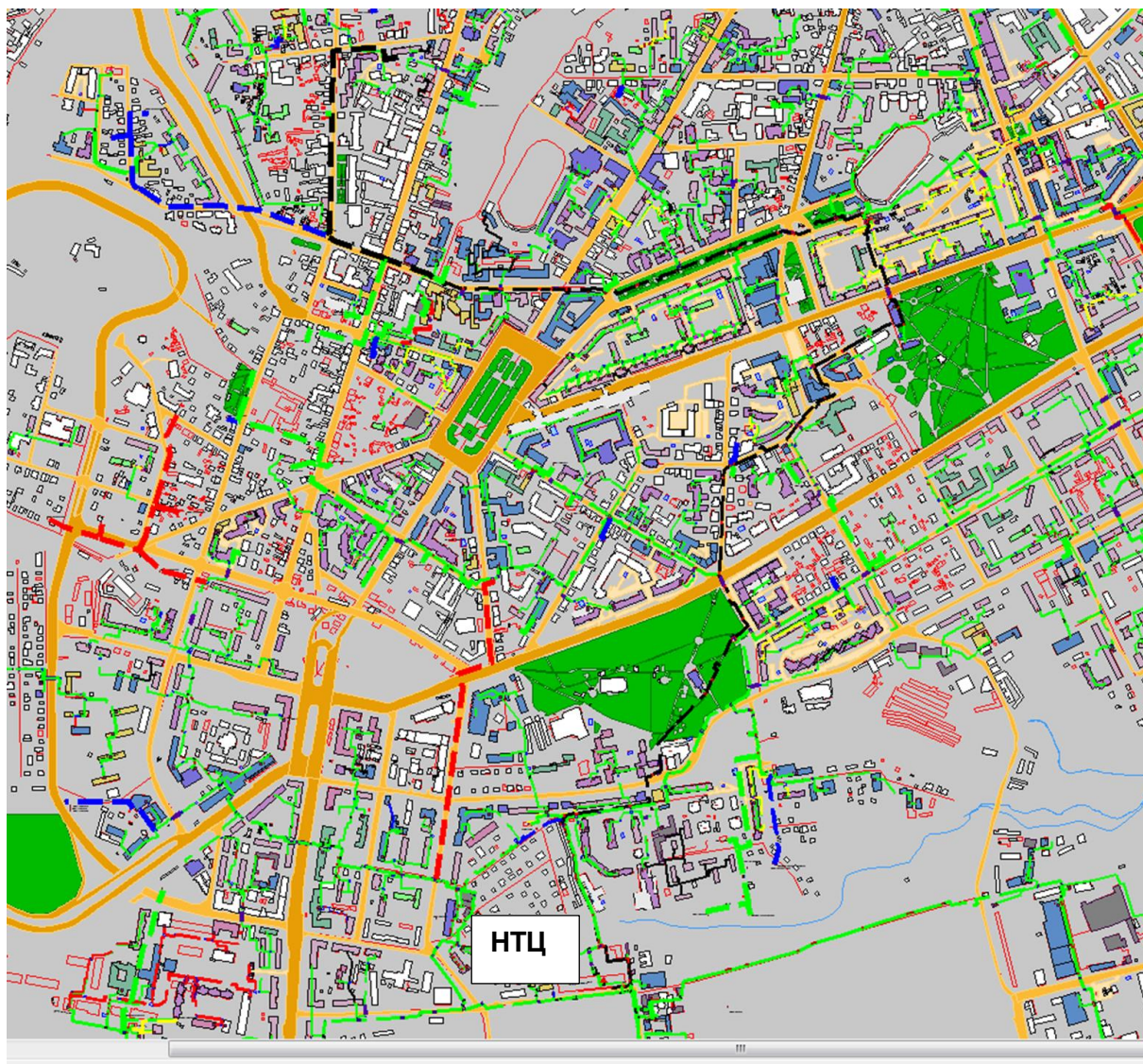
Рисунок 0.63 – Результат гидравлического расчета - расчетный путь теплоносителя от котельной НТЦ до ОТВ-009903
