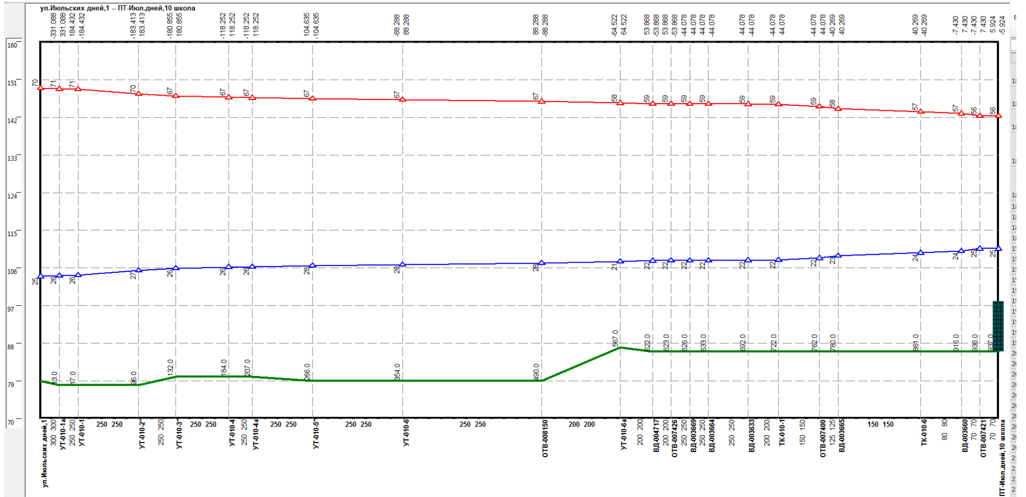
Рисунок 0.95 –Результат гидравлического расчета - график гидравлических режимов по пути теплоносителя от Июльских дней, 1 до ПТ-Июл.дней, 10 школа
