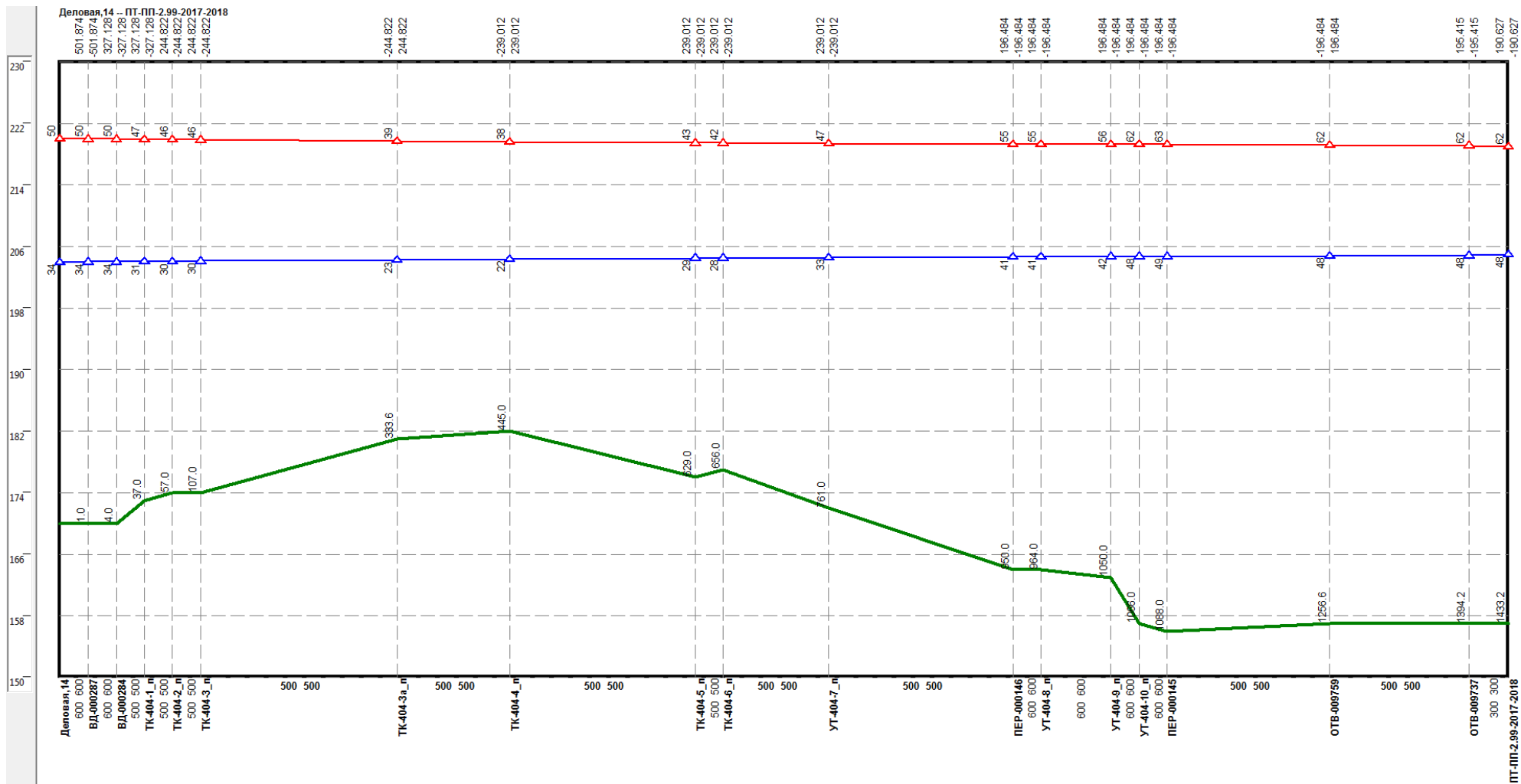
Рисунок 0.93 –Результат гидравлического расчета - график гидравлических режимов по пути теплоносителя от котельной Деловая, 14 до ПТ-ПП-2.99-2017-2018.
