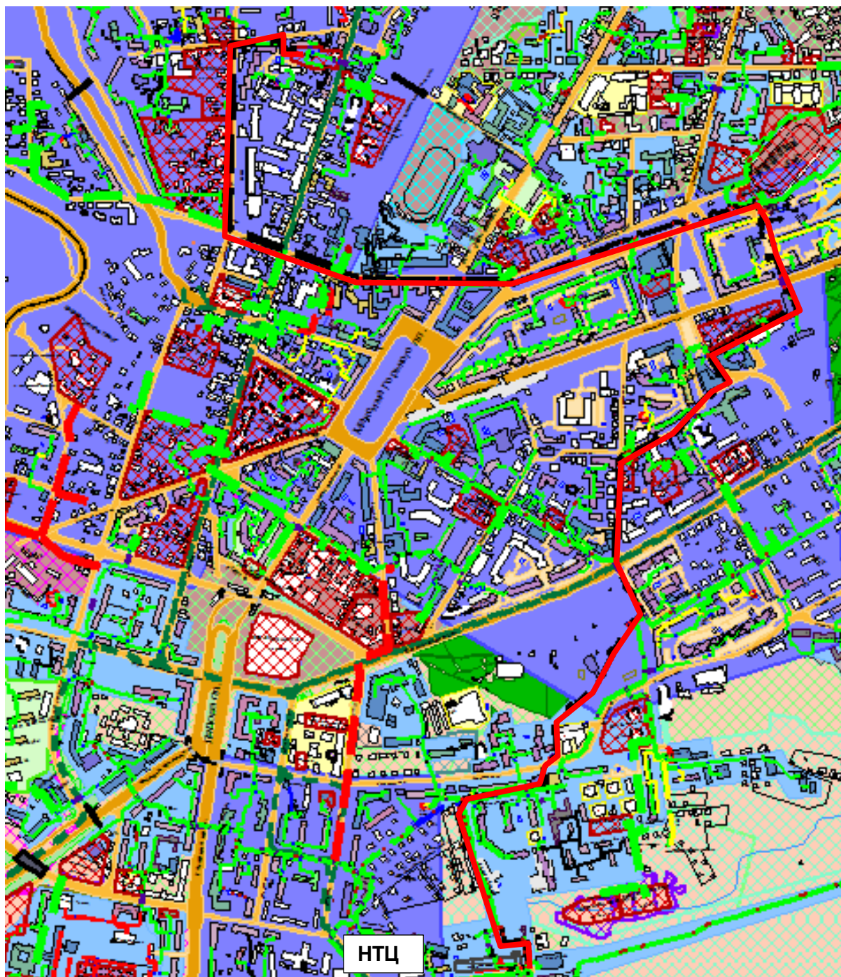
Рисунок 0.110 – Результат гидравлического расчета - расчетный путь теплоносителя от котельной НТЦ до ОТВ-009903
