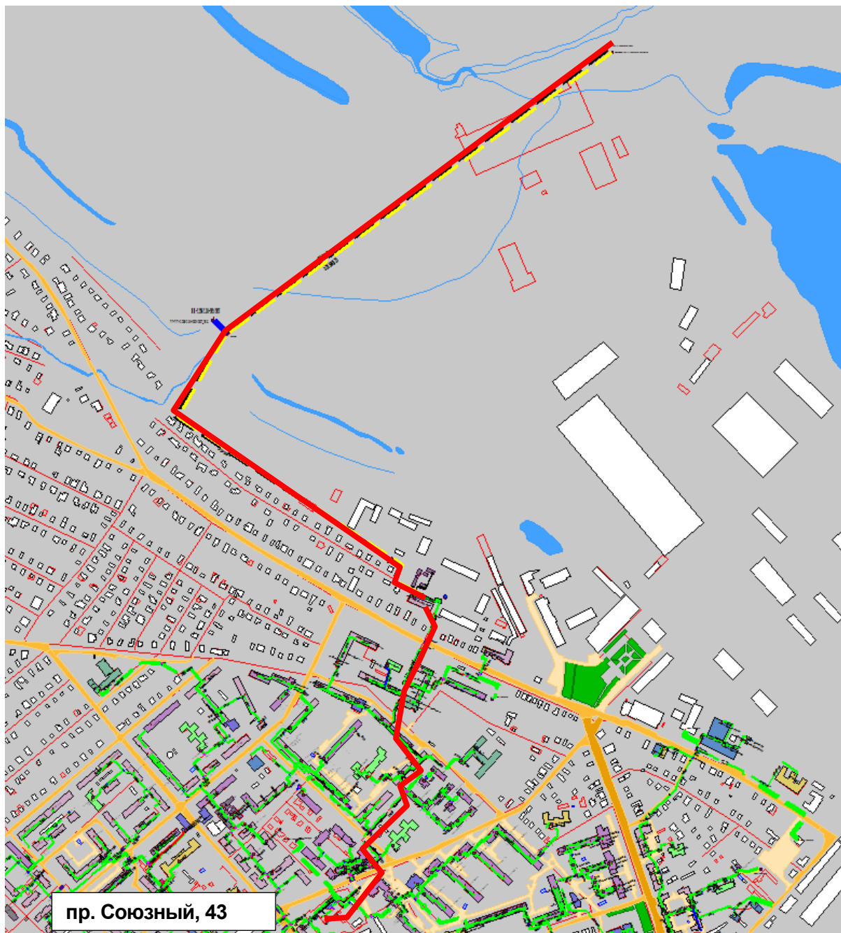
Рисунок 0.118 –Результат гидравлического расчета – расчетный путь теплоносителя от котельной пр. Союзный, 43 до ПТ-ПП-4.101/1.182-2018/2027
