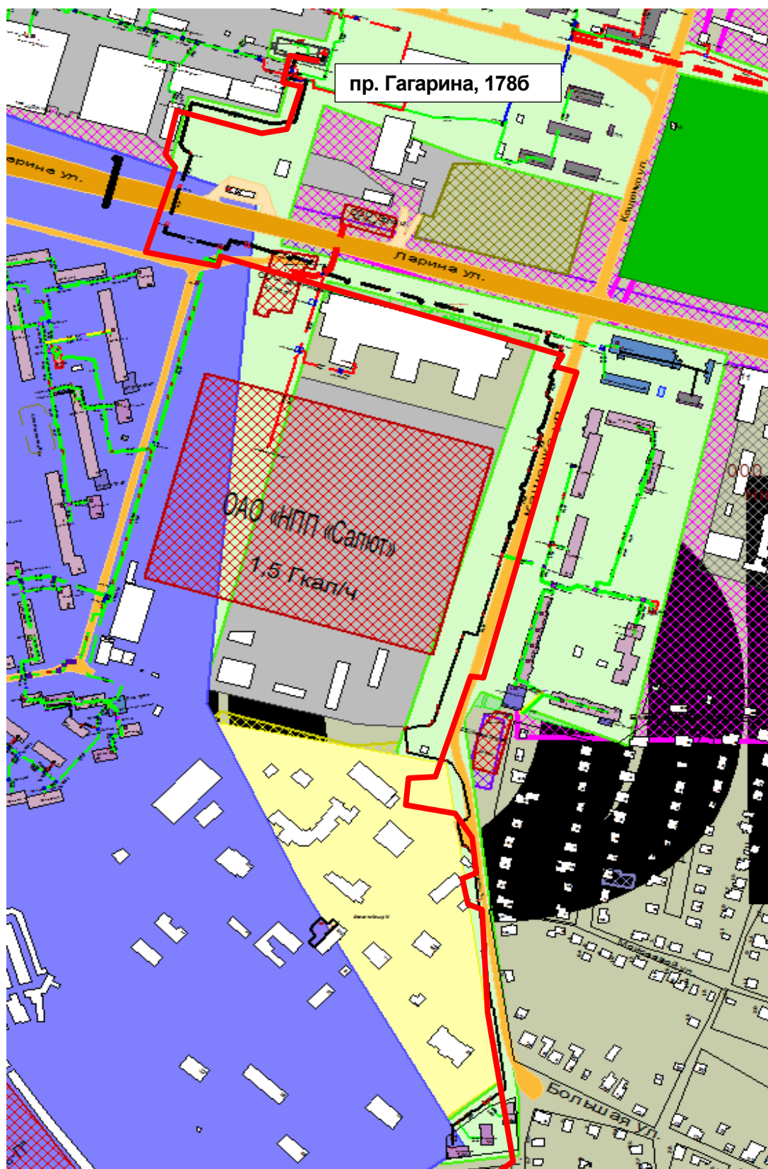
Рисунок 0.112 – Результат гидравлического расчета - расчетный путь теплоносителя от котельной пр. Гагарина, 1786 до ПТ-Кащенко, 4а
