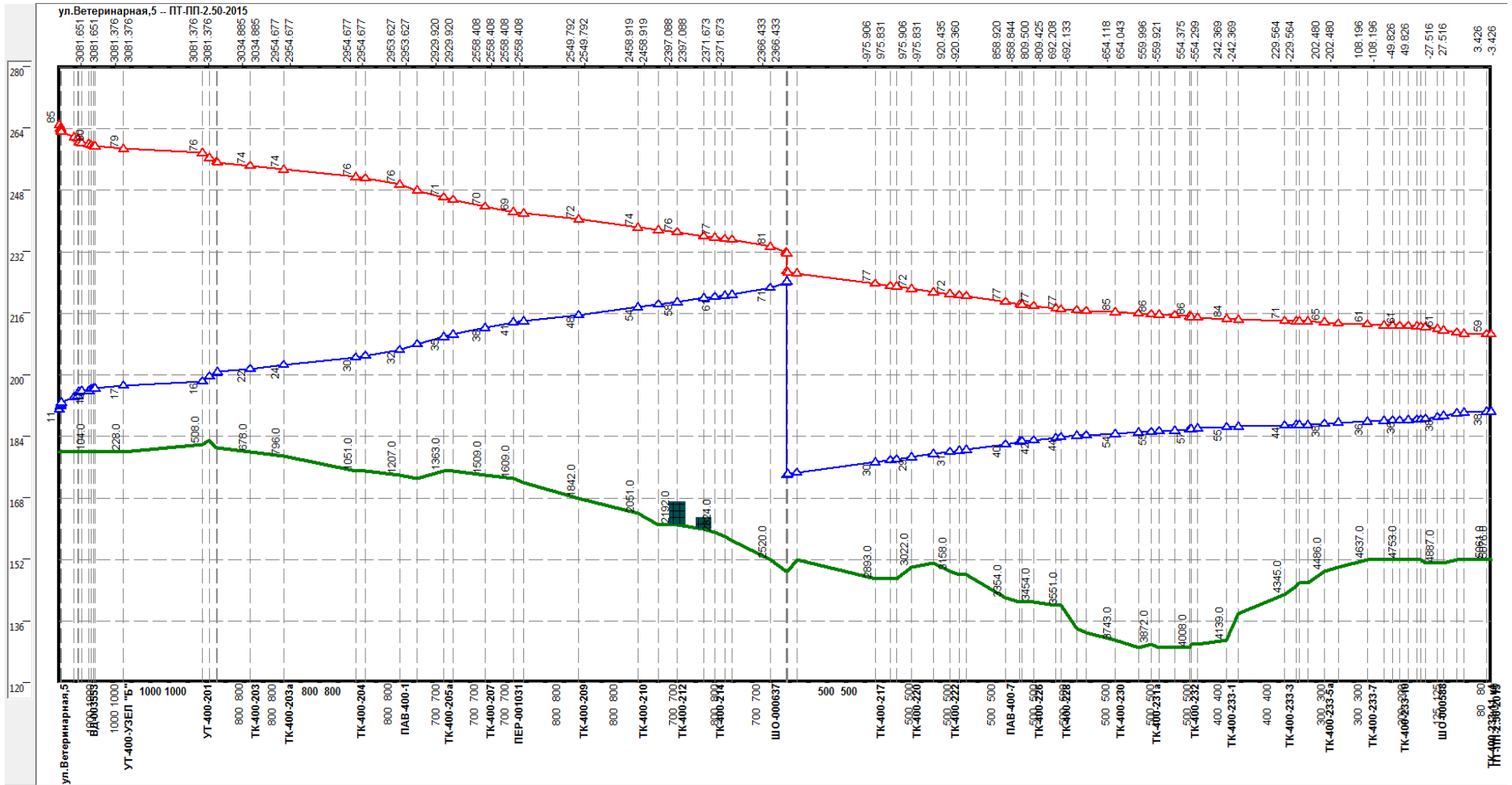
Рисунок 0.62 –Результат гидравлического расчета - график гидравлических режимов по пути теплоносителя от котельной НТЦ до ПТ-В.Волж.наб, проект.
