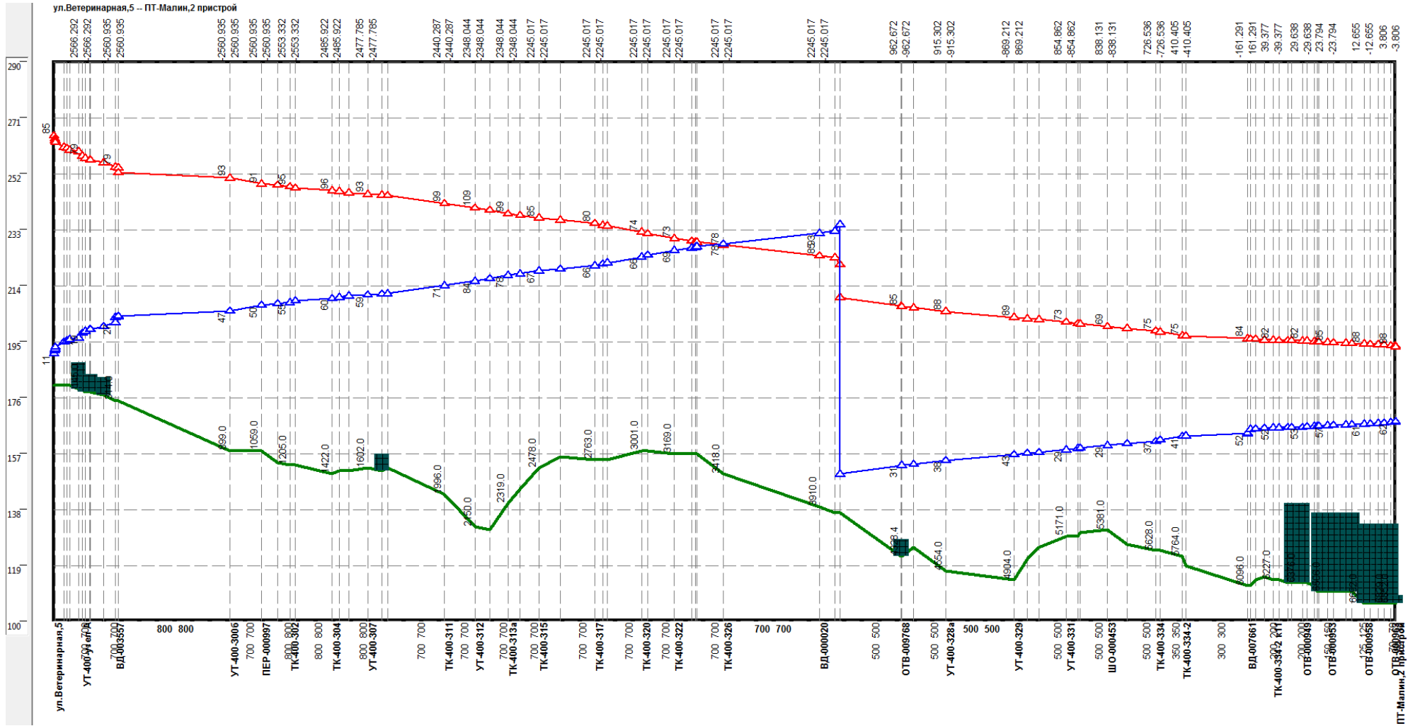
Рисунок 0.107 –Результат гидравлического расчета - график гидравлических режимов по пути теплоносителя от котельной НТЦ до ПТ-Малин,2 пристрой
