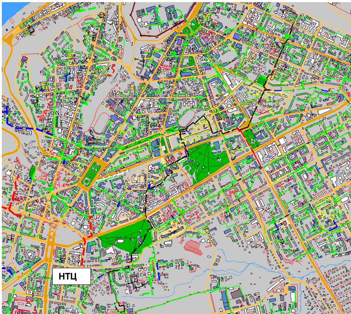
Рисунок 0.61 – Результат гидравлического расчета - расчетный путь теплоносителя от котельной НТЦ до ПТ-В.Волж.наб, проект.
