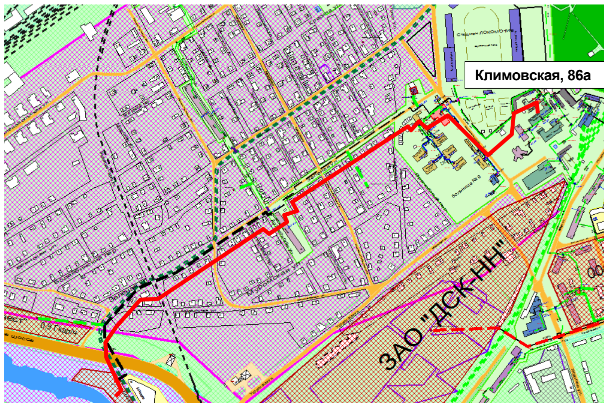
Рисунок 0.104 – Результат гидравлического расчета - расчетный путь теплоносителя от котельной Климовская, 86а до ПТ-ПП-2.227-2016
