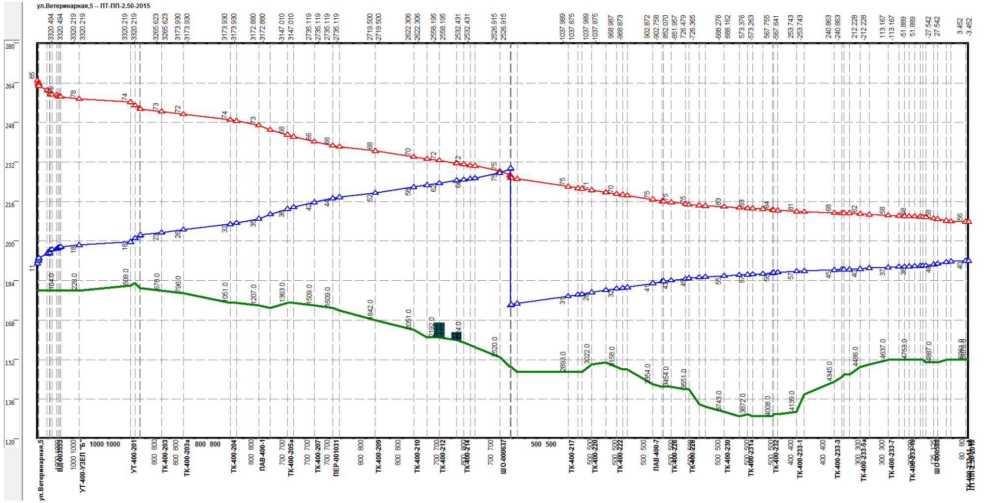
Рисунок 0.109 –Результат гидравлического расчета - график гидравлических режимов по пути теплоносителя от котельной НТЦ до ПТ-В.Волж.наб, проект
