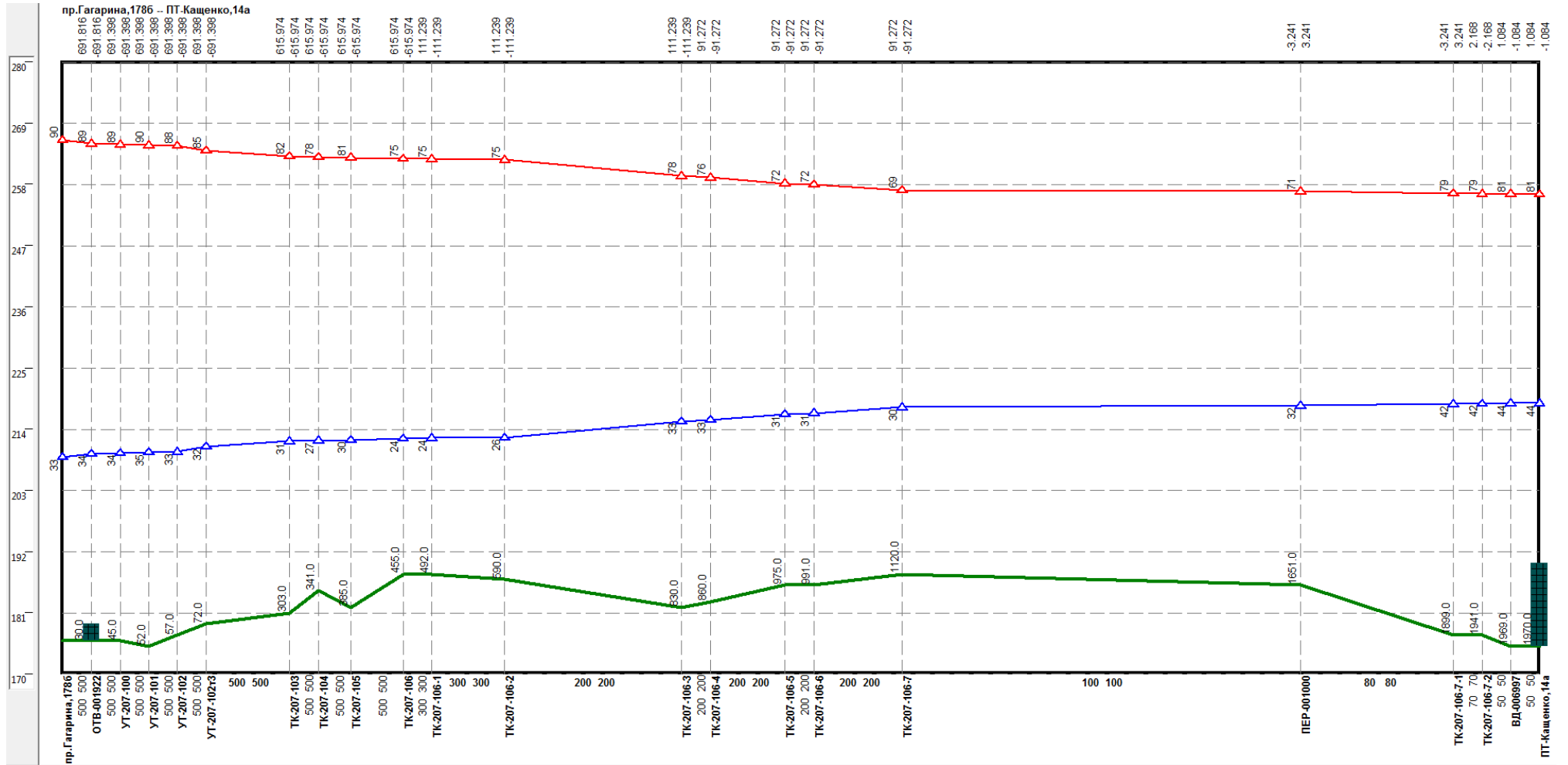
Рисунок 0.113 –Результат гидравлического расчета - график гидравлических режимов по пути теплоносителя от котельной пр. Гагарина, 1786 до ПТ-Кашенко, 14а
