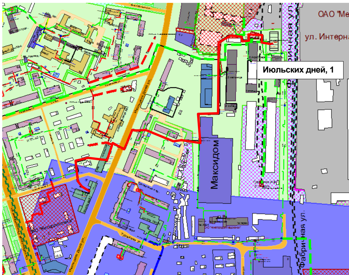
Рисунок 0.94 – Результат гидравлического расчета - расчетный путь теплоносителя от Июльских дней, 1 до ПТ-Июльских дней, 10 школа
