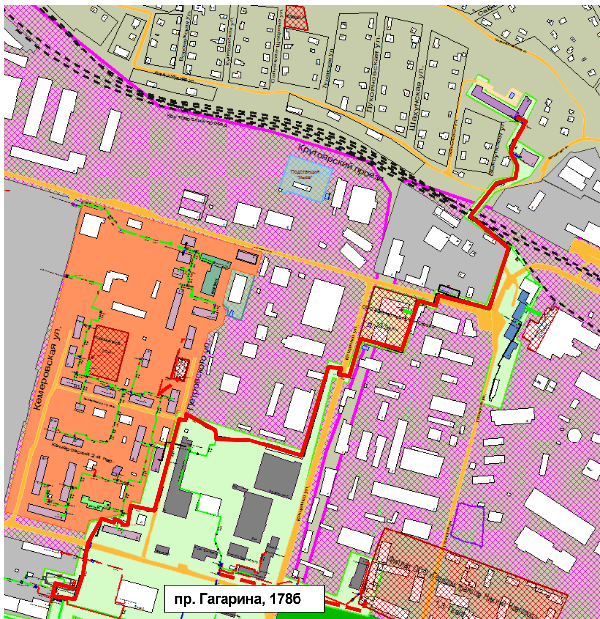
Рисунок 0.114 – Результат гидравлического расчета - расчетный путь теплоносителя от котельной пр. Гагарина, 1786 до ЦТП-706
