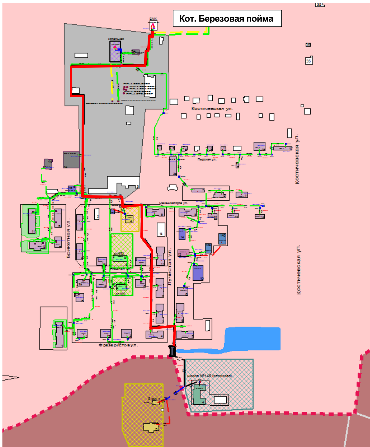
Рисунок 0.88 – Результат гидравлического расчета - расчетный путь теплоносителя от котельной Березовая пойма до ПТ-Лучистая,4
