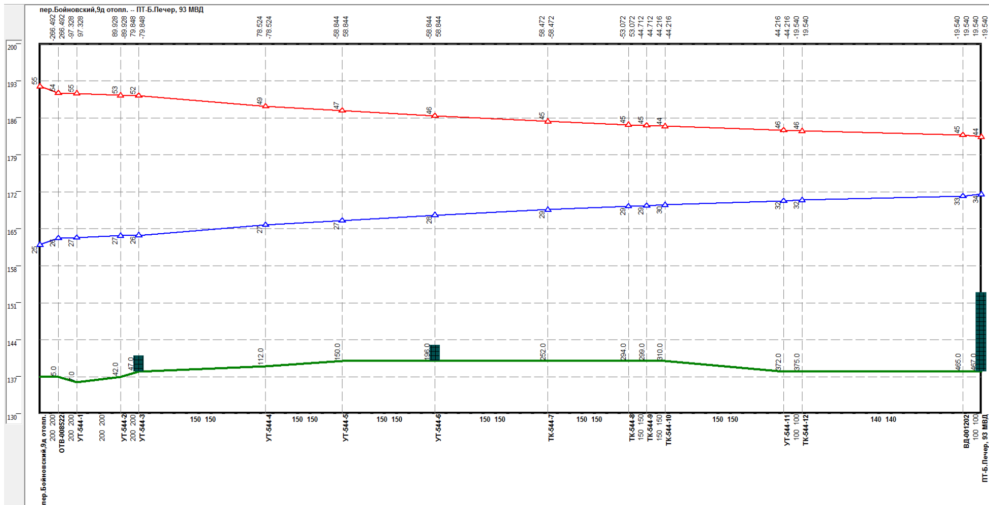
Рисунок 0.24 –Результат гидравлического расчета - график гидравлических режимов по пути теплоносителя от Бойновский, 9д до ПТ-Б.Печер, 93 МВД
