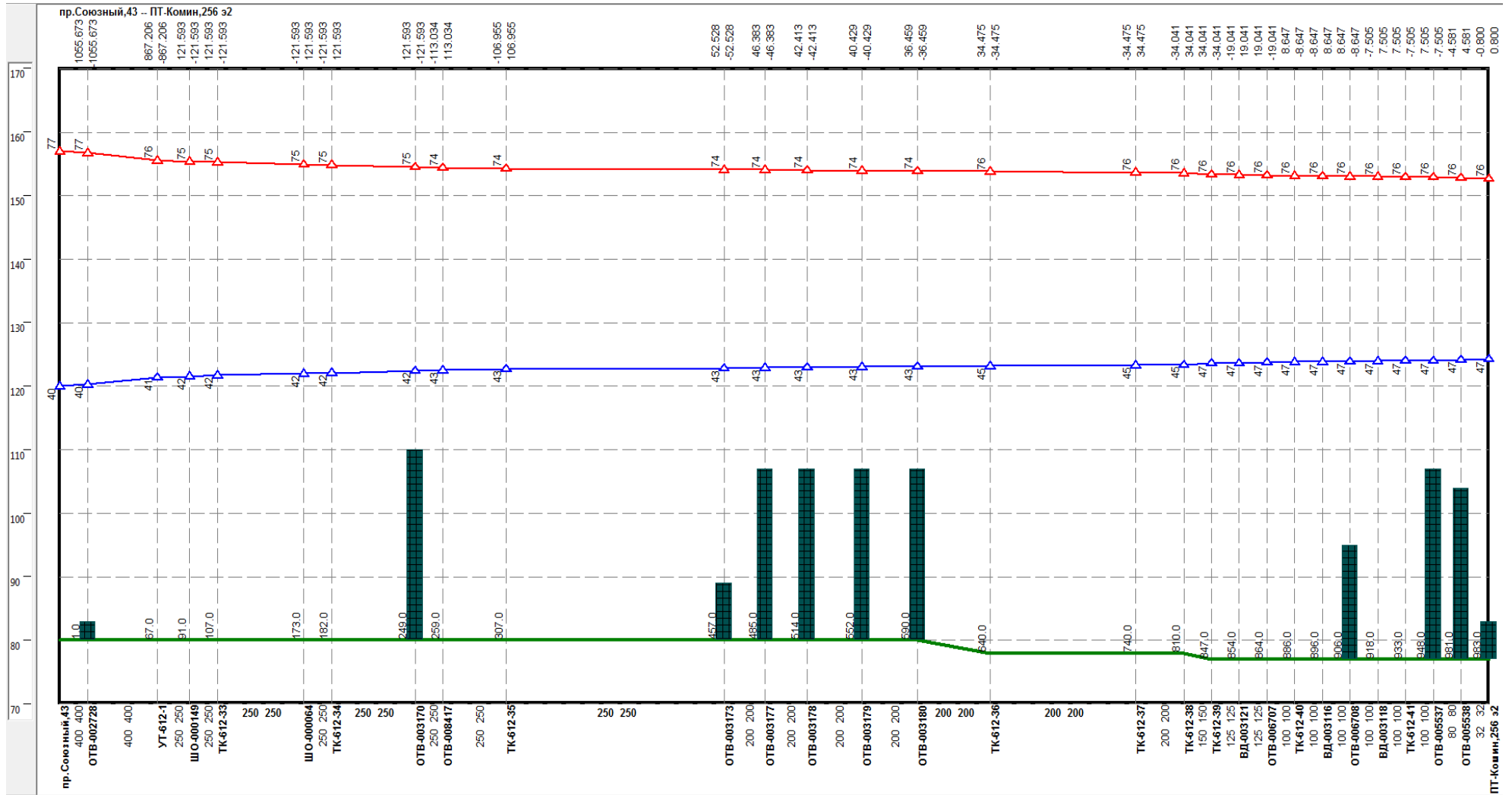
Рисунок 0.42 –Результат гидравлического расчета - график гидравлических режимов по пути теплоносителя от котельной пр. Союзный, д.43 до ПТ-Комин, 256 э2
