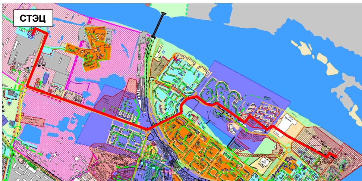
Рисунок 0.76 - Результат гидравлического расчета - расчетный путь теплоносителя от СТЭЦ до ПТ-ПП-2.64-2017
