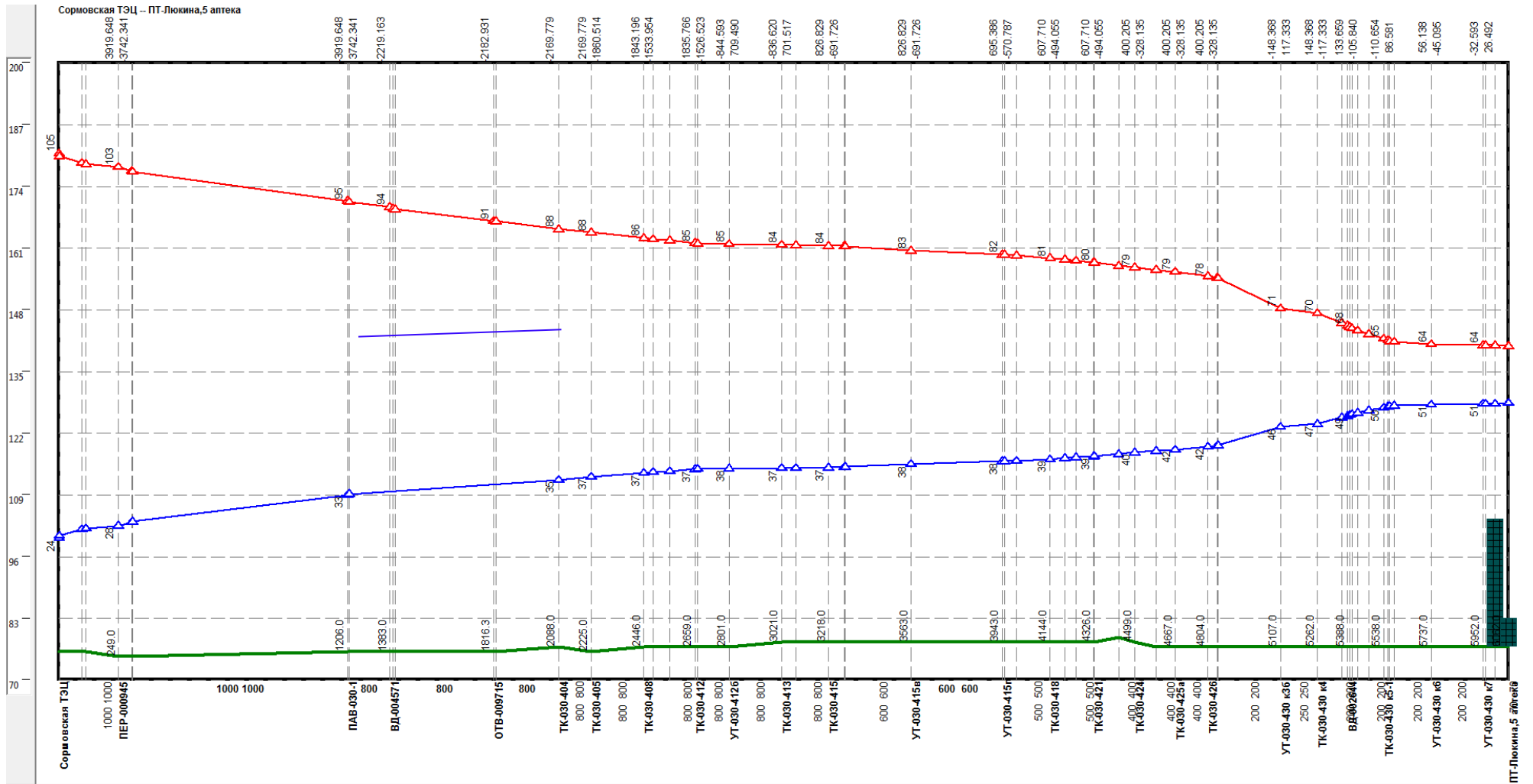
Рисунок 0.75 –Результат гидравлического расчета - график гидравлических режимов по пути теплоносителя от СТЭЦ до ПТ-Люкина,5 аптека
