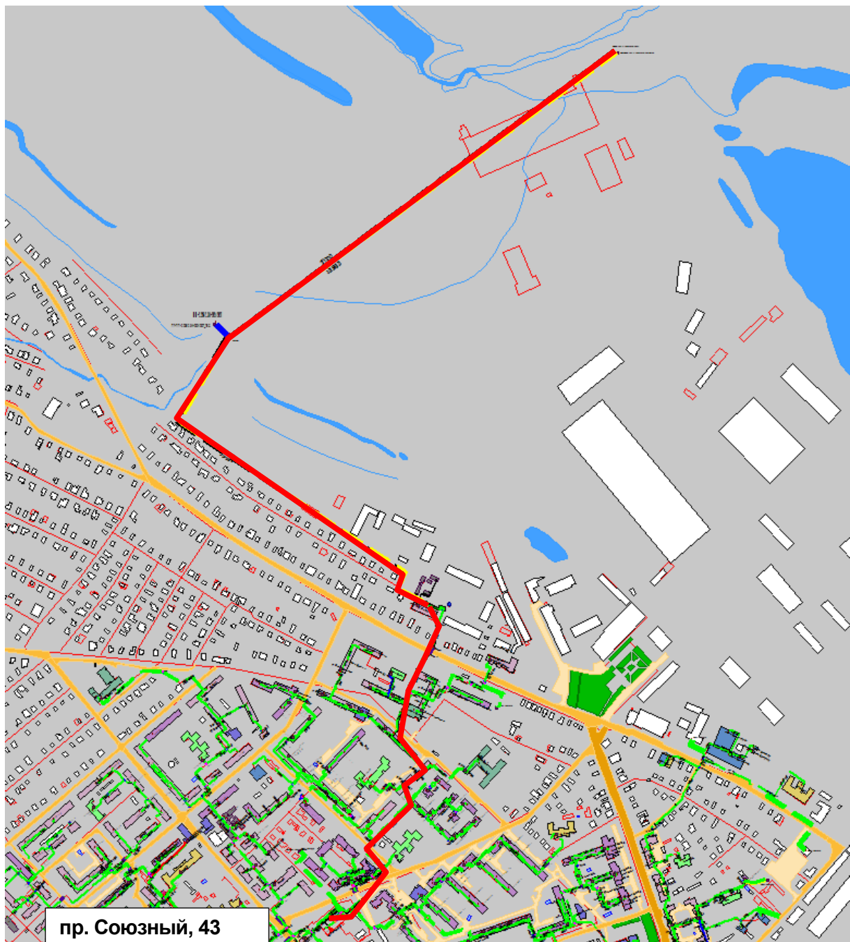
Рисунок 0.39 – Результат гидравлического расчета - расчетный путь от котельной пр. Союзный, 43 до ПТ-ПП-4.101/1.182-2018/2027.
