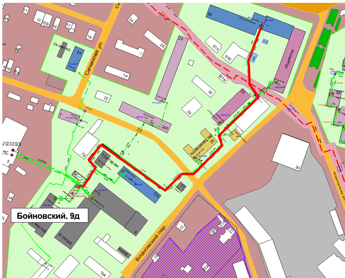
Рисунок 0.86 – Результат гидравлического расчета - расчетный путь теплоносителя от Бойновский, 9д до ПТ-Б.Печер, 93 МВт
