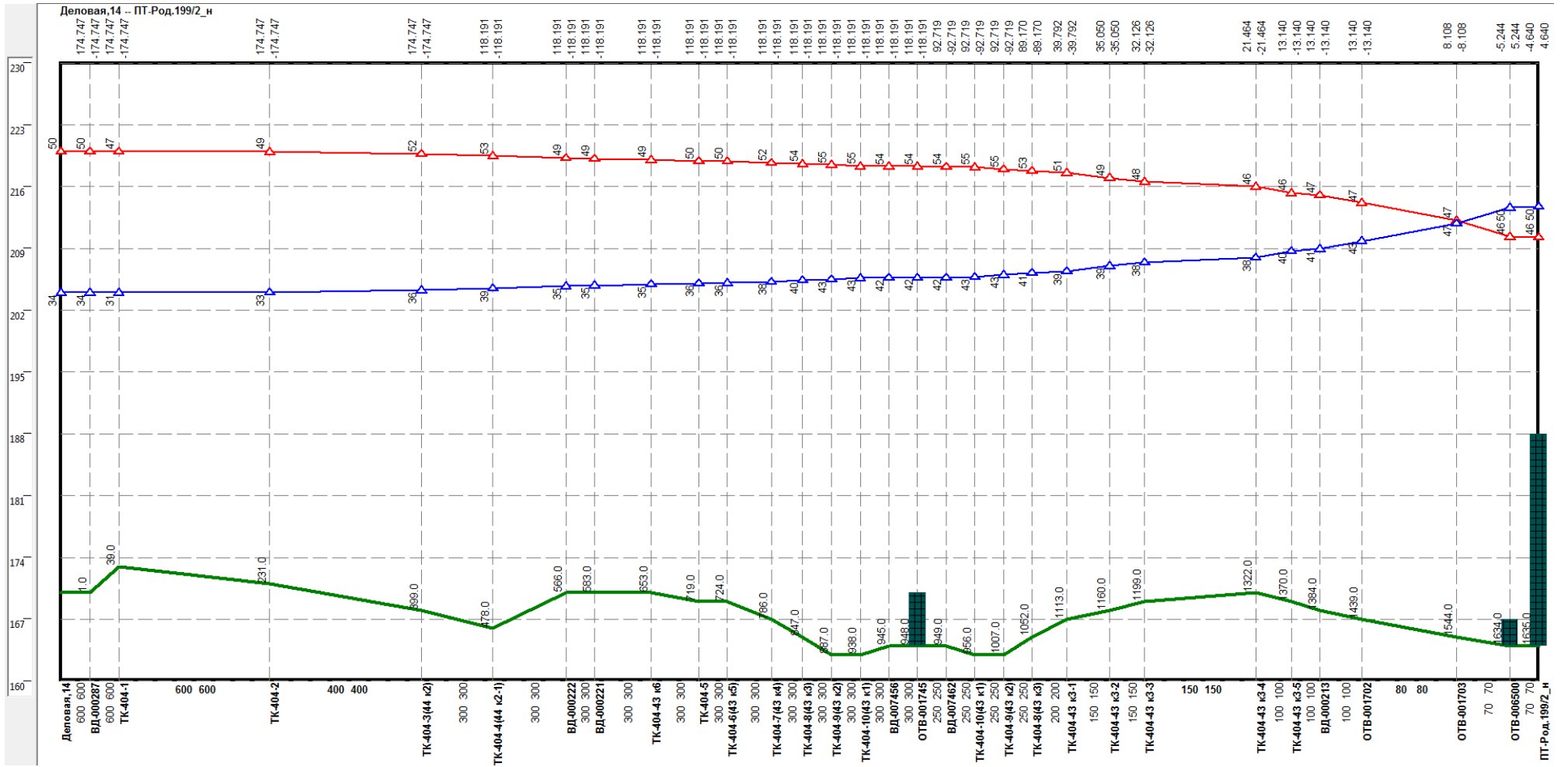
Рисунок 0.91 –Результат гидравлического расчета - график гидравлических режимов по пути теплоносителя от котельной Деловая, 14 до ПТ-Род.199/2_н
