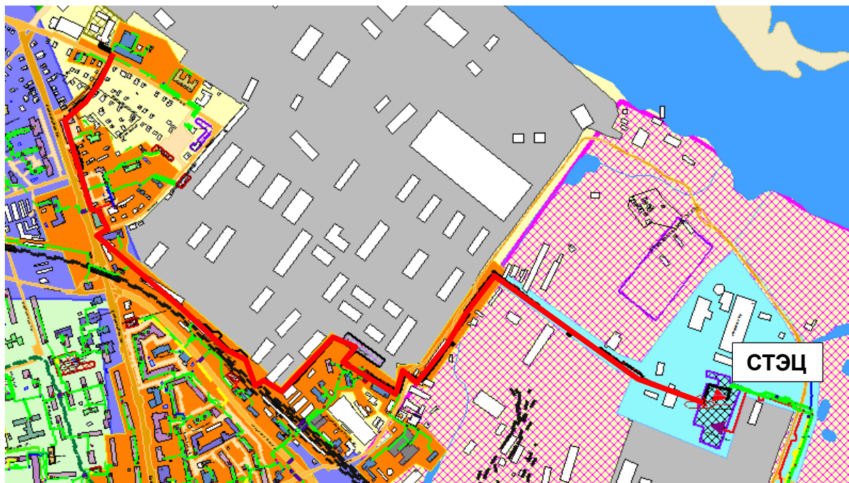
Рисунок 0.80- Результат гидравлического расчета - расчетный путь теплоносителя от СТЭЦ до ПТ-ПП-2.23-2016
