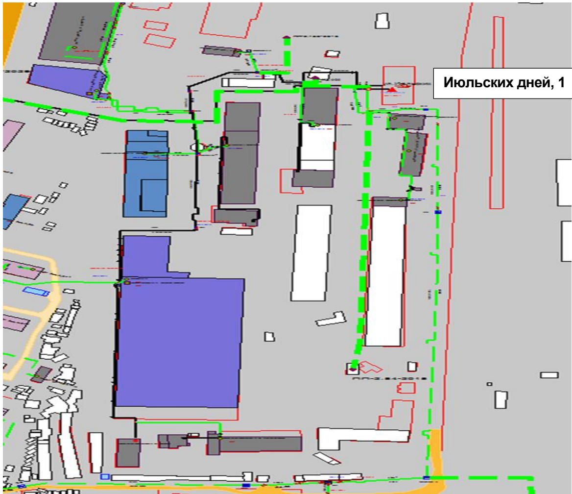
Рисунок 0.96 – Результат гидравлического расчета - расчетный путь теплоносителя от котельной Июльских дней, 1 до ПТ-Деревооб,1а АБК
