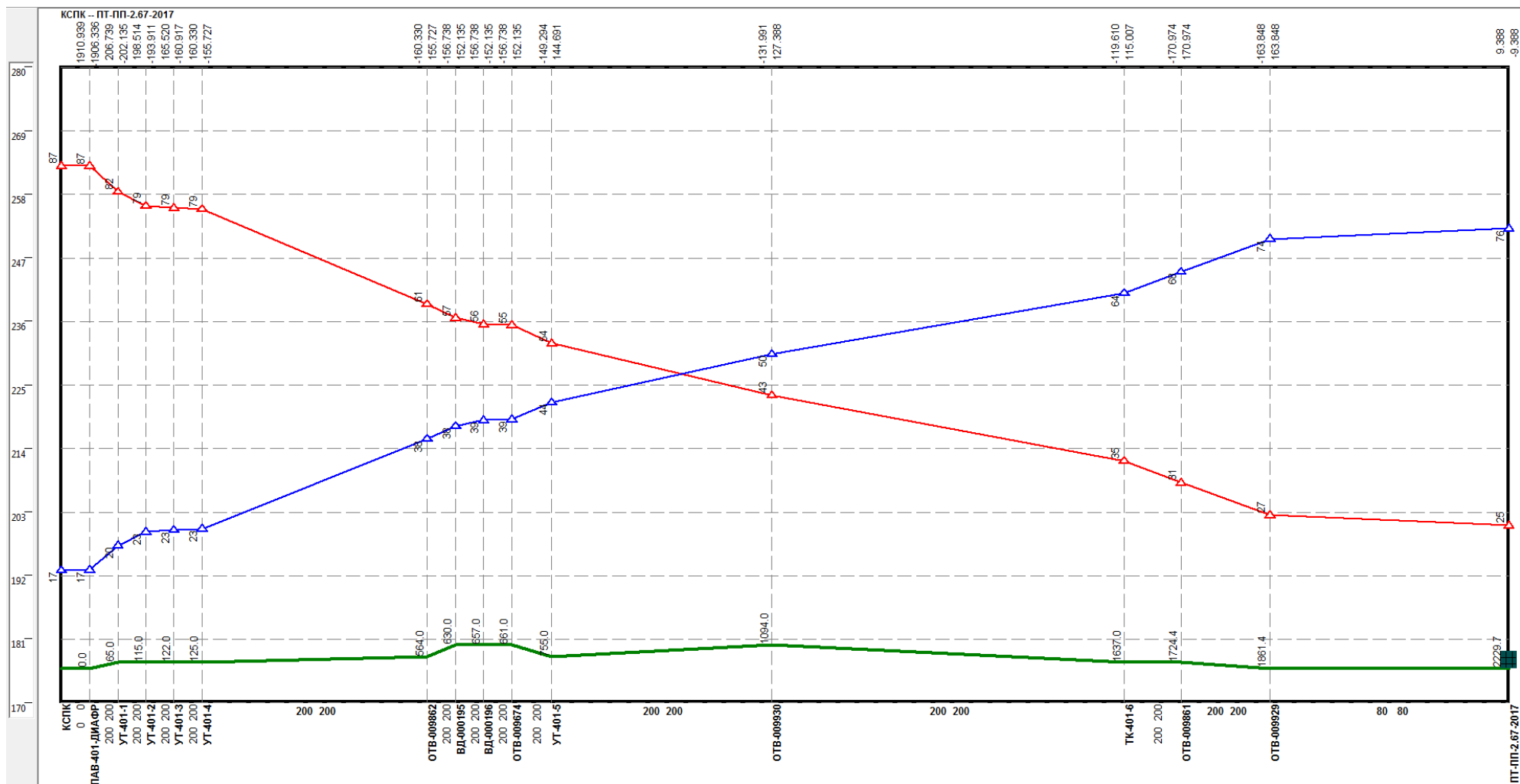
Рисунок 0.99 – Результат гидравлического расчета - график гидравлических режимов по пути теплоносителя от котельной ул. Родионова, 1946 до ПТ-ПП-2.67-2017
