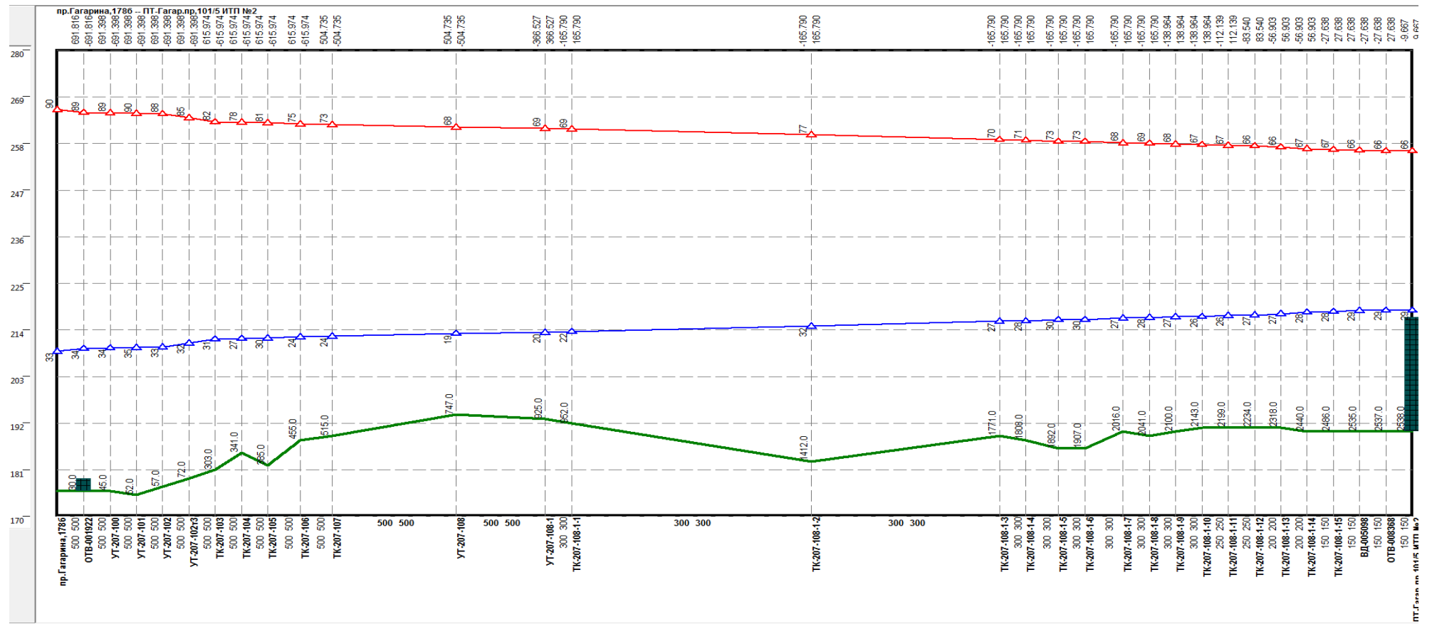
Рисунок 0.117 - Результат гидравлического расчета - расчетный путь теплоносителя от котельной пр. Гагарина, 1786 до ПТ-Гагар.пр.101/5 ИТП №2
