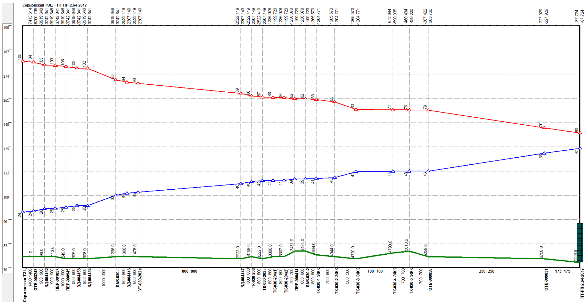
Рисунок 0.77 –Результат гидравлического расчета - график гидравлических режимов по пути теплоносителя от СТЭЦ до ПТ-ПП-2.64-2017
