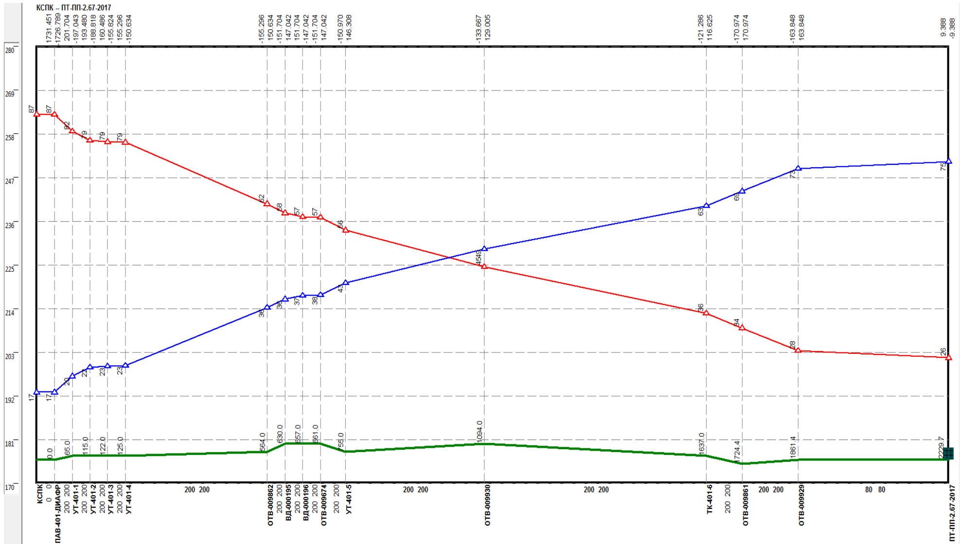
Рисунок 0.72 –Результат гидравлического расчета - график гидравлических режимов по пути теплоносителя от котельной ул. Родионова, 1946 до ПТ-ПП-2.67-2017
