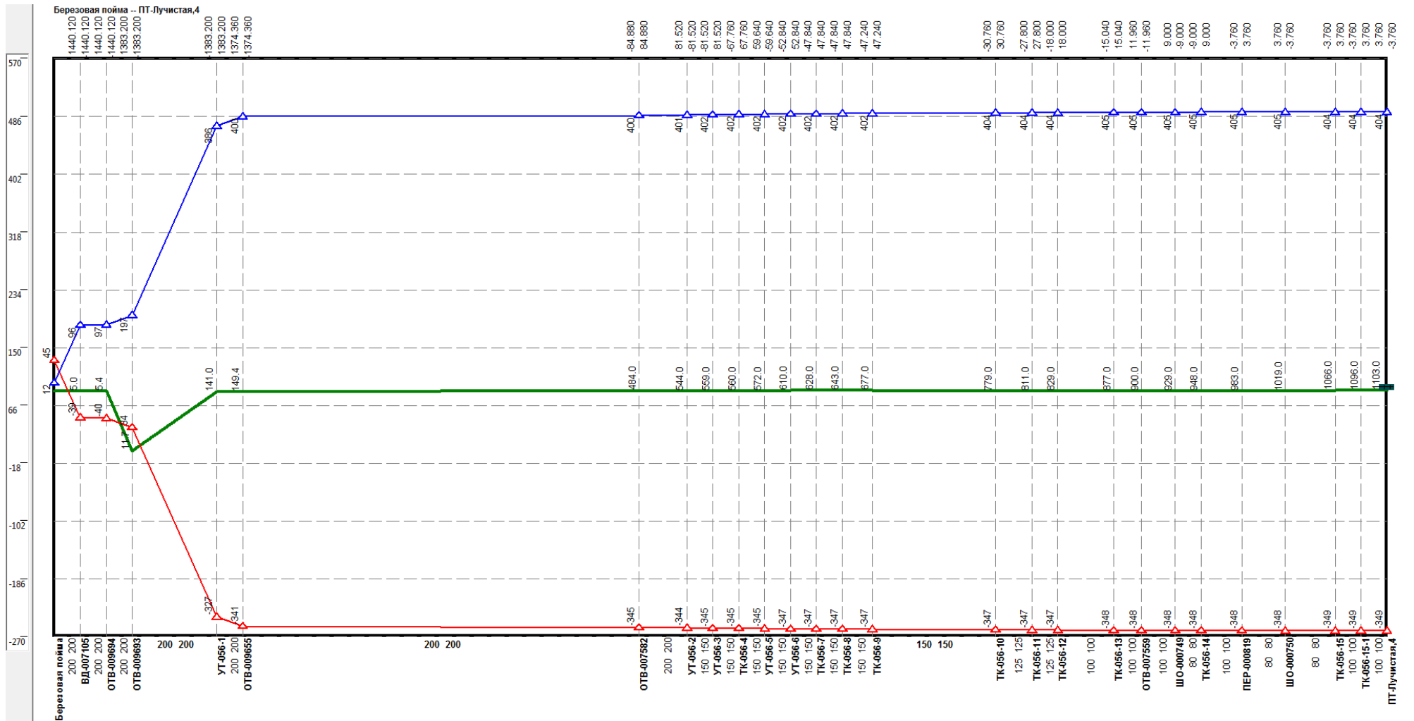
Рисунок 0.89 –Результат гидравлического расчета - график гидравлических режимов по пути теплоносителя от котельной Березовая пойма до ПТ-Лучистая, 4
