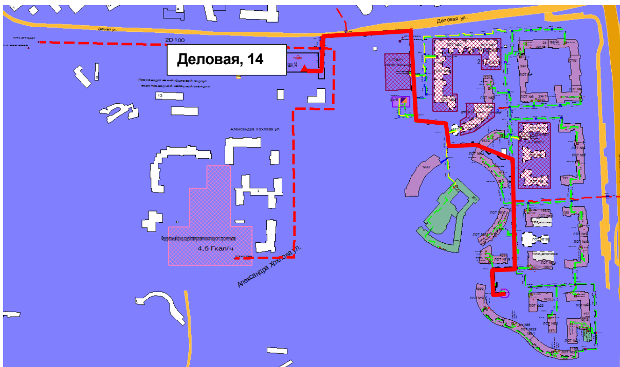
Рисунок 0.90 – Результат гидравлического расчета - расчетный путь теплоносителя от котельной Деловая, 14 до ПТ-Род.199/2_н
