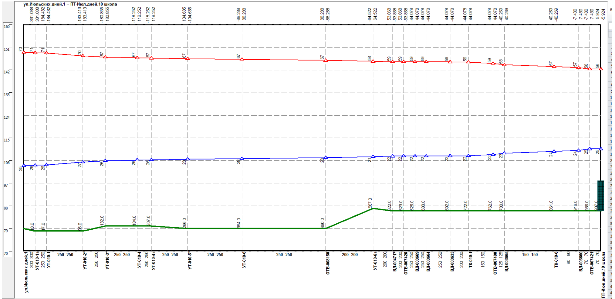
Рисунок 0.32 –Результат гидравлического расчета - график гидравлических режимов по пути теплоносителя от Июльских дней, 1 до ПТ-Июльских дней, 10 школа
