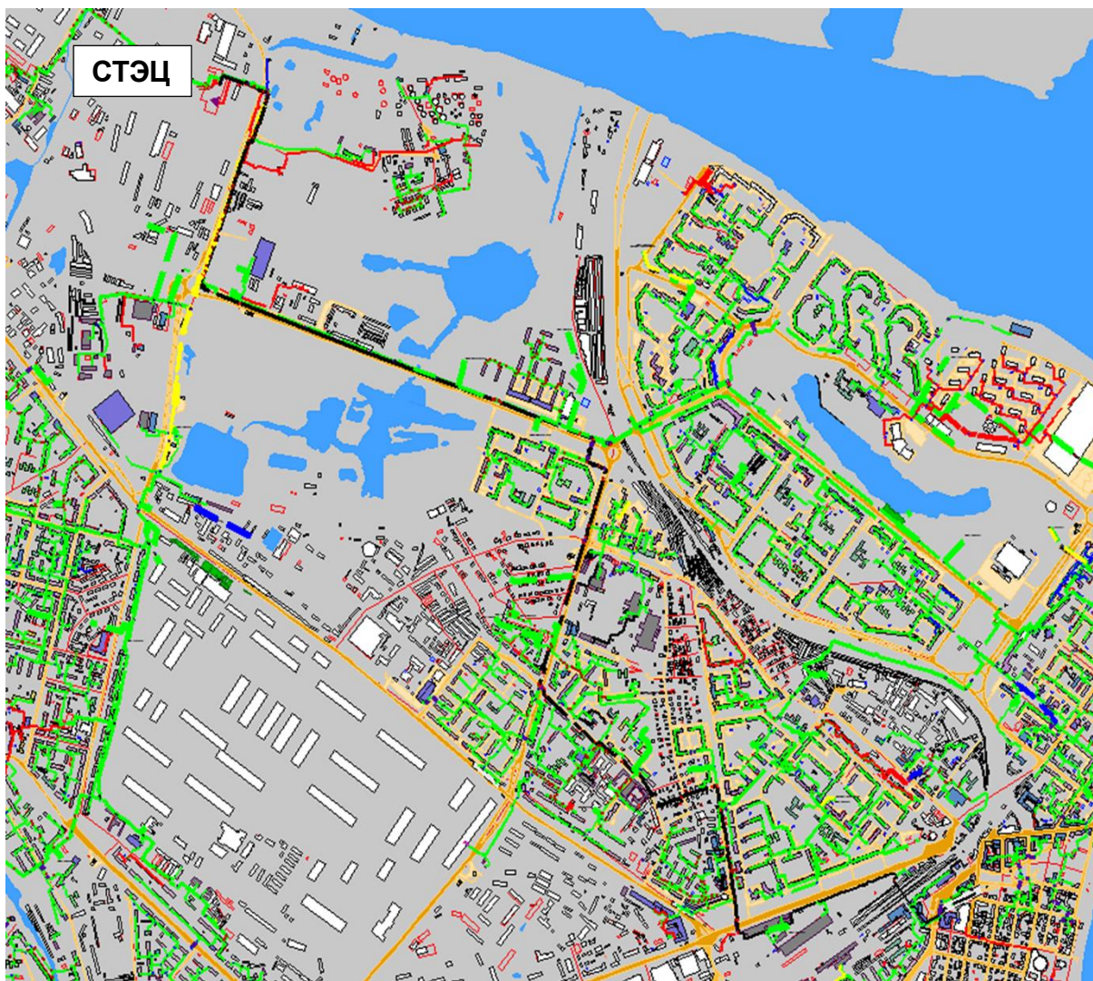
Рисунок 0.78 - Результат гидравлического расчета - расчетный путь теплоносителя от СТЭЦ до ПТ-пл.Револ,7 вест2
