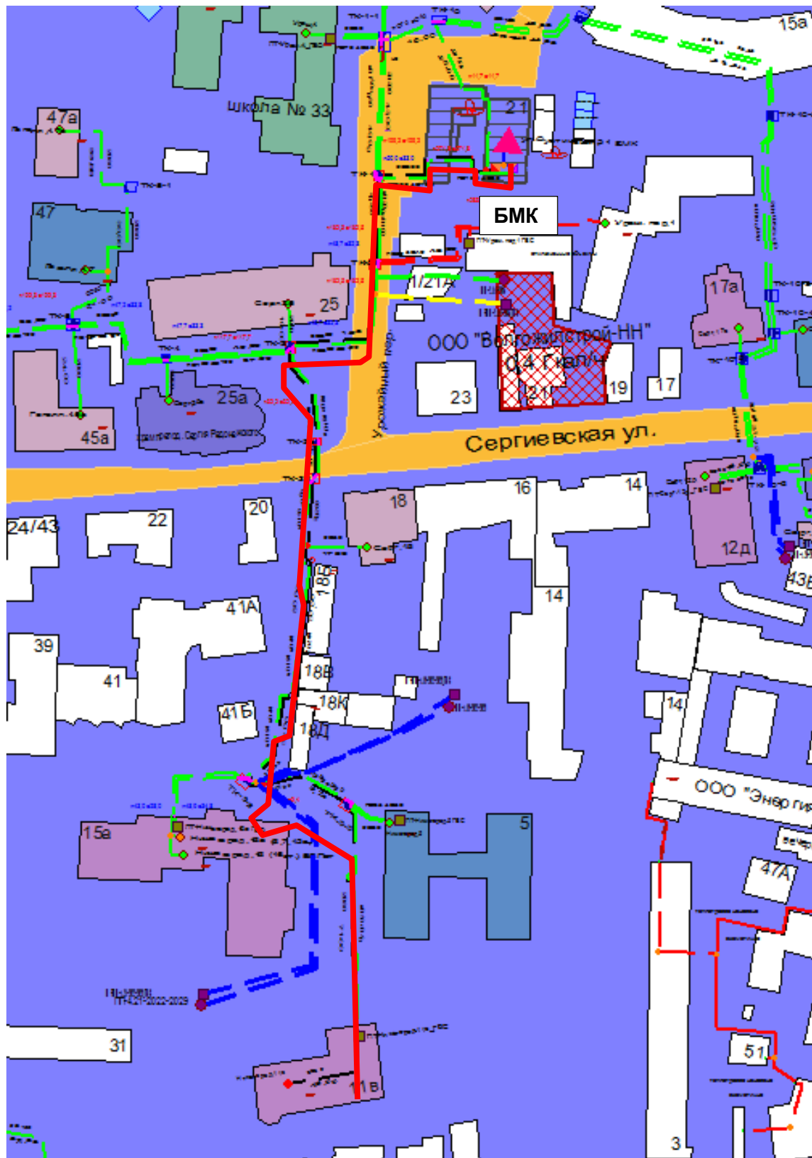
Рисунок 0.82 – Результат гидравлического расчета - расчетный путь теплоносителя от котельной Суевинская, 21 до ПТ-Нижнегород, 11в
