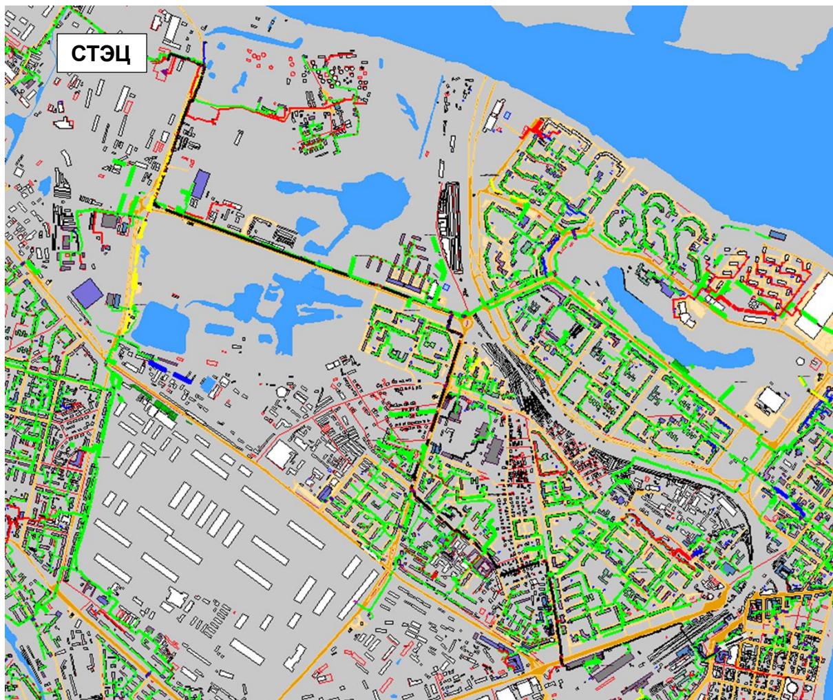
Рисунок 0.5 - Результат гидравлического расчета - расчетный путь теплоносителя от СТЭЦ до ПТ-пл.Револ,7 вест2
