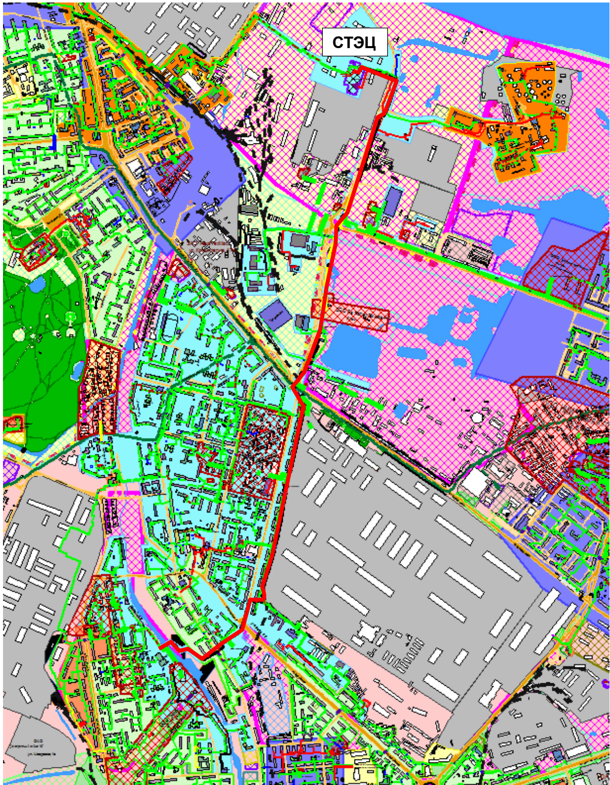
Рисунок 0.74 - Результат гидравлического расчета - расчетный путь теплоносителя от СТЭЦ до ПТ-Люкина,5 аптека
