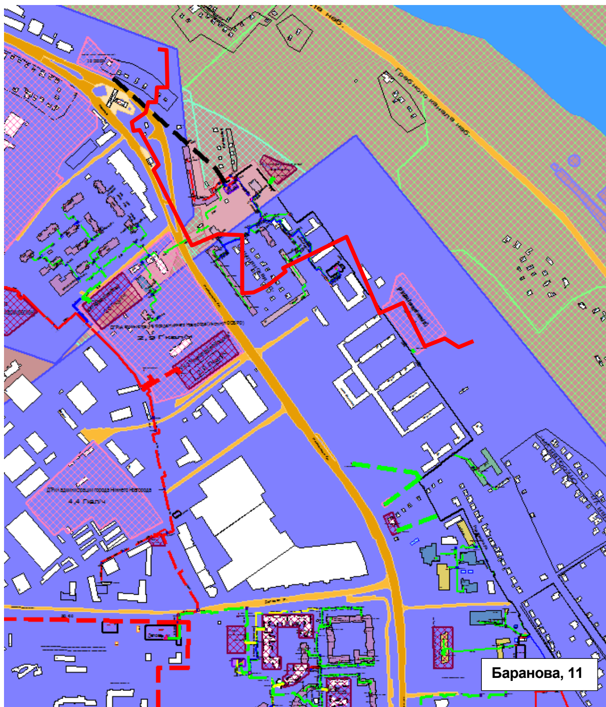
Рисунок 0.98 – Результат гидравлического расчета - расчетный путь теплоносителя от котельной ул. Родионова, 1946 до ПТ-ПП-2.67-2017
