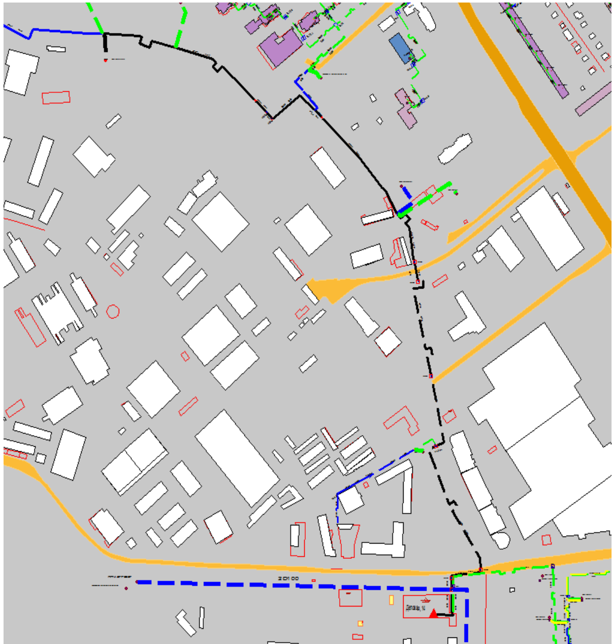
Рисунок 0.92 – Результат гидравлического расчета - расчетный путь теплоносителя от котельной Деловая, 14 до ПТ-ПП-2.99-2017-2018
