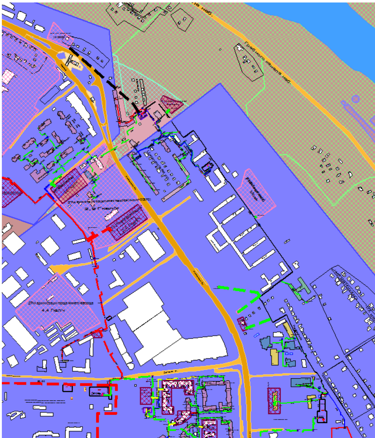
Рисунок 0.71 – Результат гидравлического расчета - расчетный путь теплоносителя от котельной ул. Родионова, 194б до ПТ-ПП-2.67-2017
