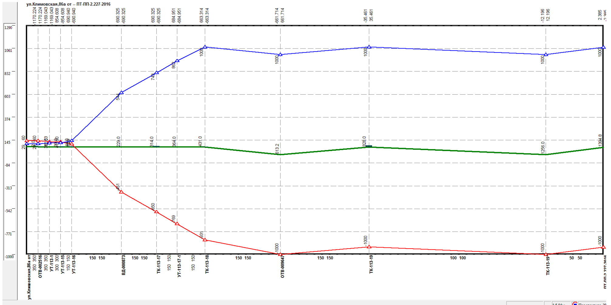
Рисунок 0.105 –Результат гидравлического расчета - график гидравлических режимов по пути теплоносителя от котельной Климовская, 86а до ПТ-ПП-2.227-2016
