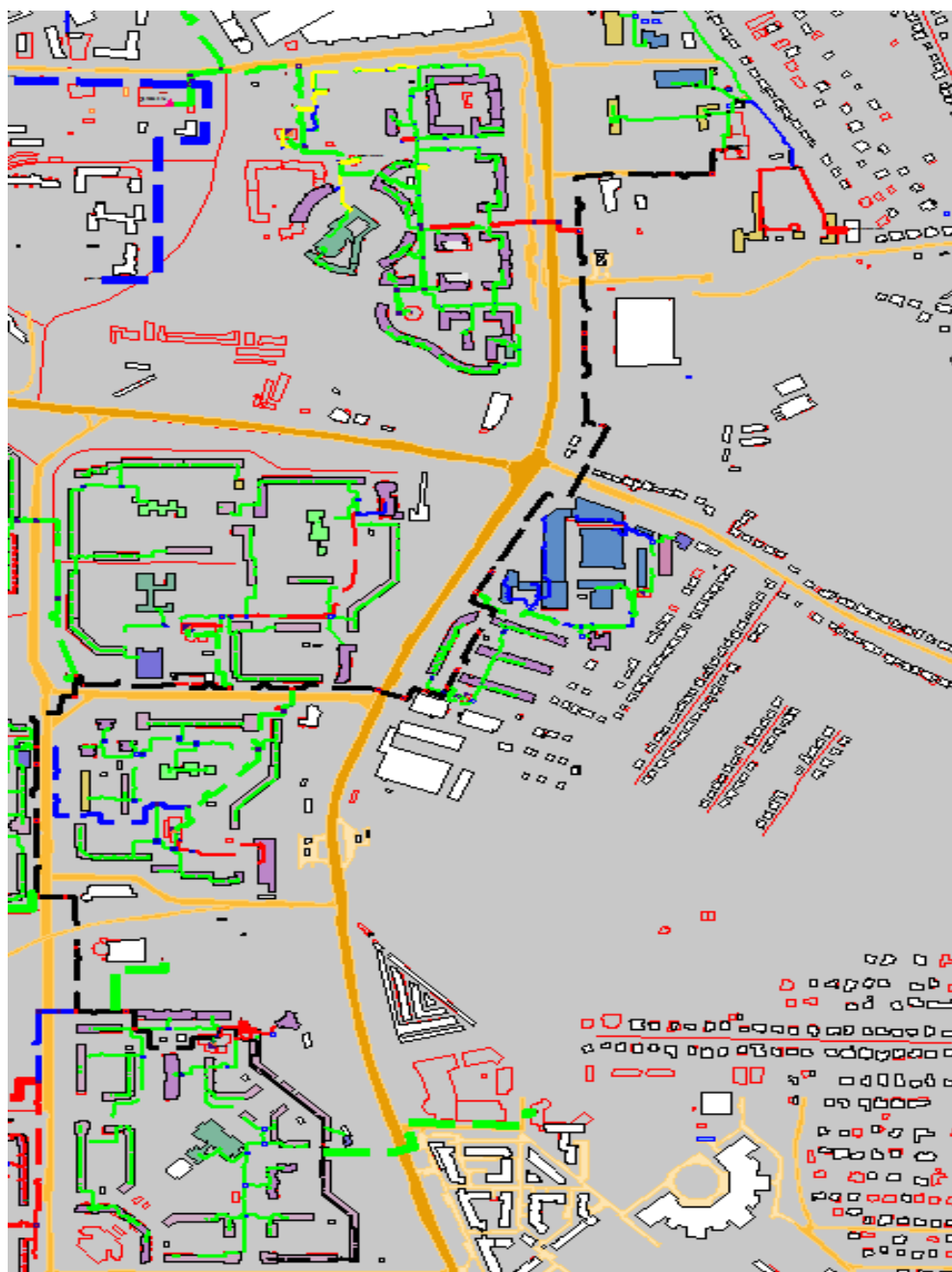
Рисунок 0.733 – Результат гидравлического расчета - расчетный путь теплоносителя от котельной ул. Родионова, 194б до ПТ-Богдан, 1 пр.
