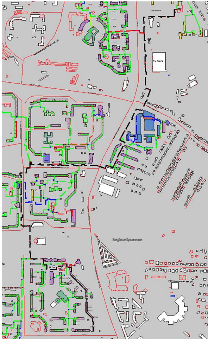
Рисунок 3.136 – Трассировка теплопровода от котельной ООО «Нижневтеплоэнерго» по ул. Родионова, д. 194Б до конечного потребителя «ПТ-Богдан.1 пр»
