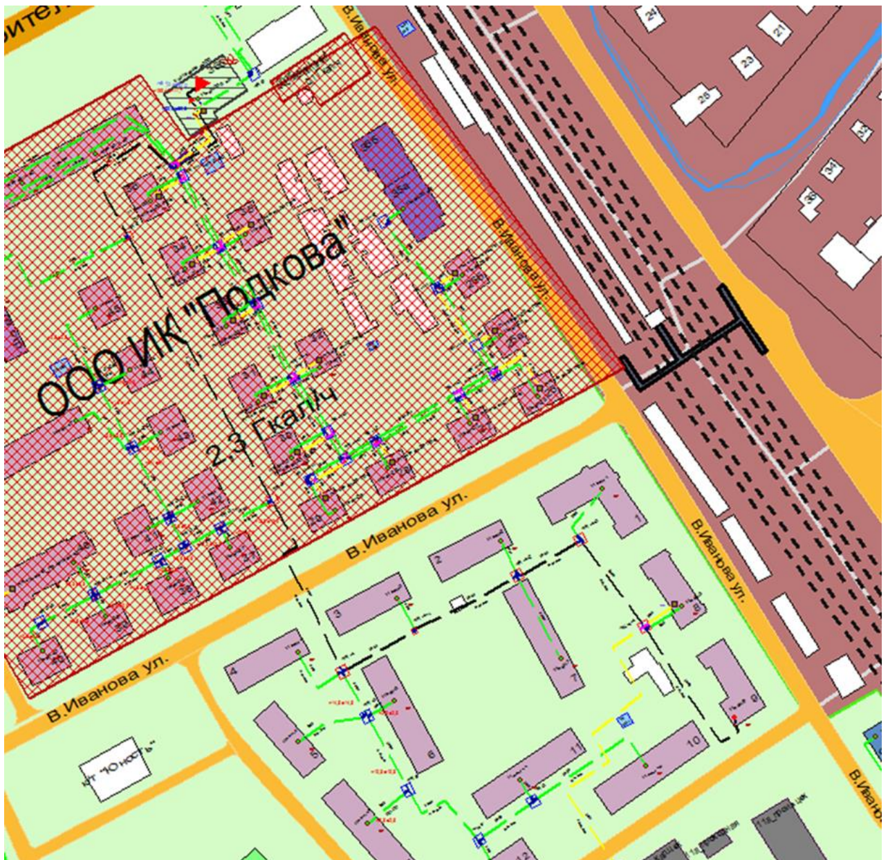
Рисунок 3.124 – Трассировка теплопровода от котельной АО «Теплоэнерго» по ул. Иванова, д. 36Б до конечного потребителя «ПТ-Иван,9»
