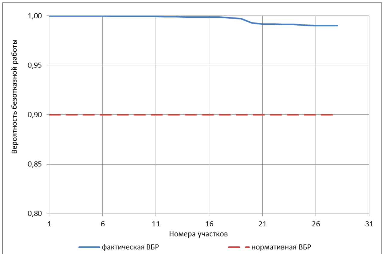
Рисунок 3.44 – ВБР относительно ТК конечного потребителя «ПТ-Июльские, 10 школа» теплопроводов зоны котельной АО «Теплоэнерго» по ул. Июльских дней, д. 1 (расчетный путь 8-1) к 2030 году
