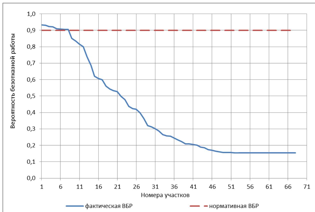
Рисунок 3.14 – ВБР относительно ТК потребителя «ПТ-Карьерная, 1а» тепловодов зоны Автозаводской ТЭЦ (расчетный путь 2-1) к 2030 году без проведения мероприятий по реконструкции участков тепловой сети
