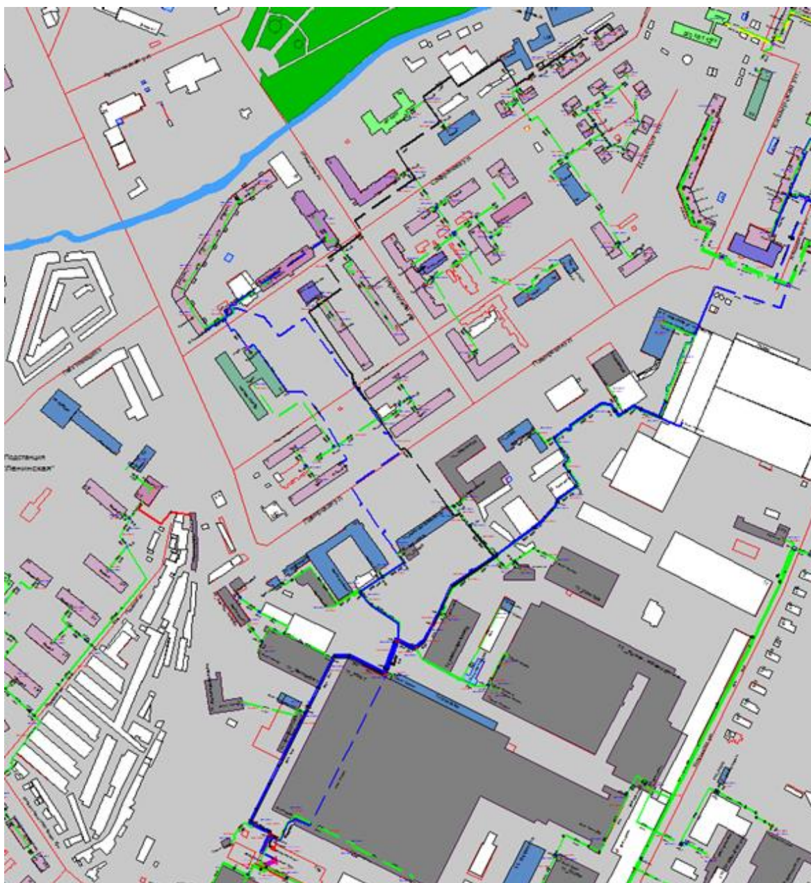
Рисунок 1.13 Результат гидравлического расчета - расчетный путь теплоносителя от котельной Памирская, 11 до ПТ-Сафрон,15 вв2
