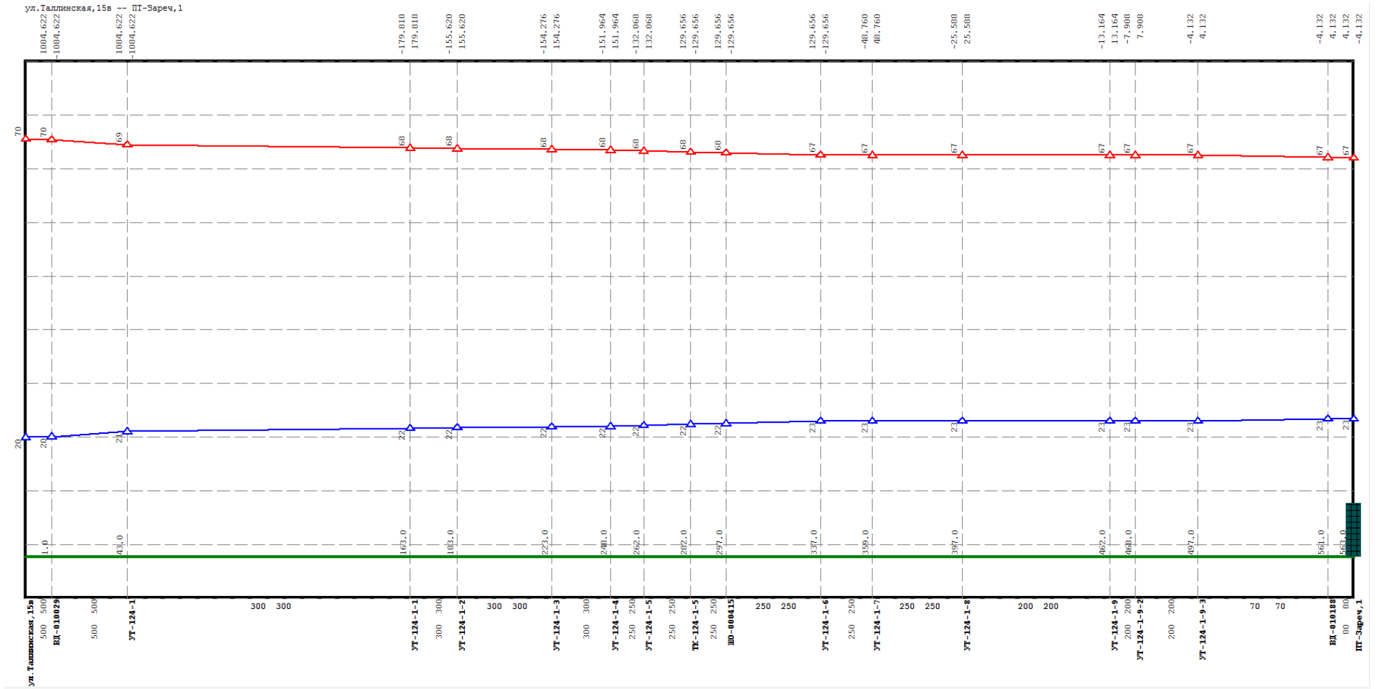
Рисунок 1.100 Результат гидравлического расчета - график гидравлических режимов по пути теплоносителя от котельной Таллинская, 15б до ПТ-Зареч,1
