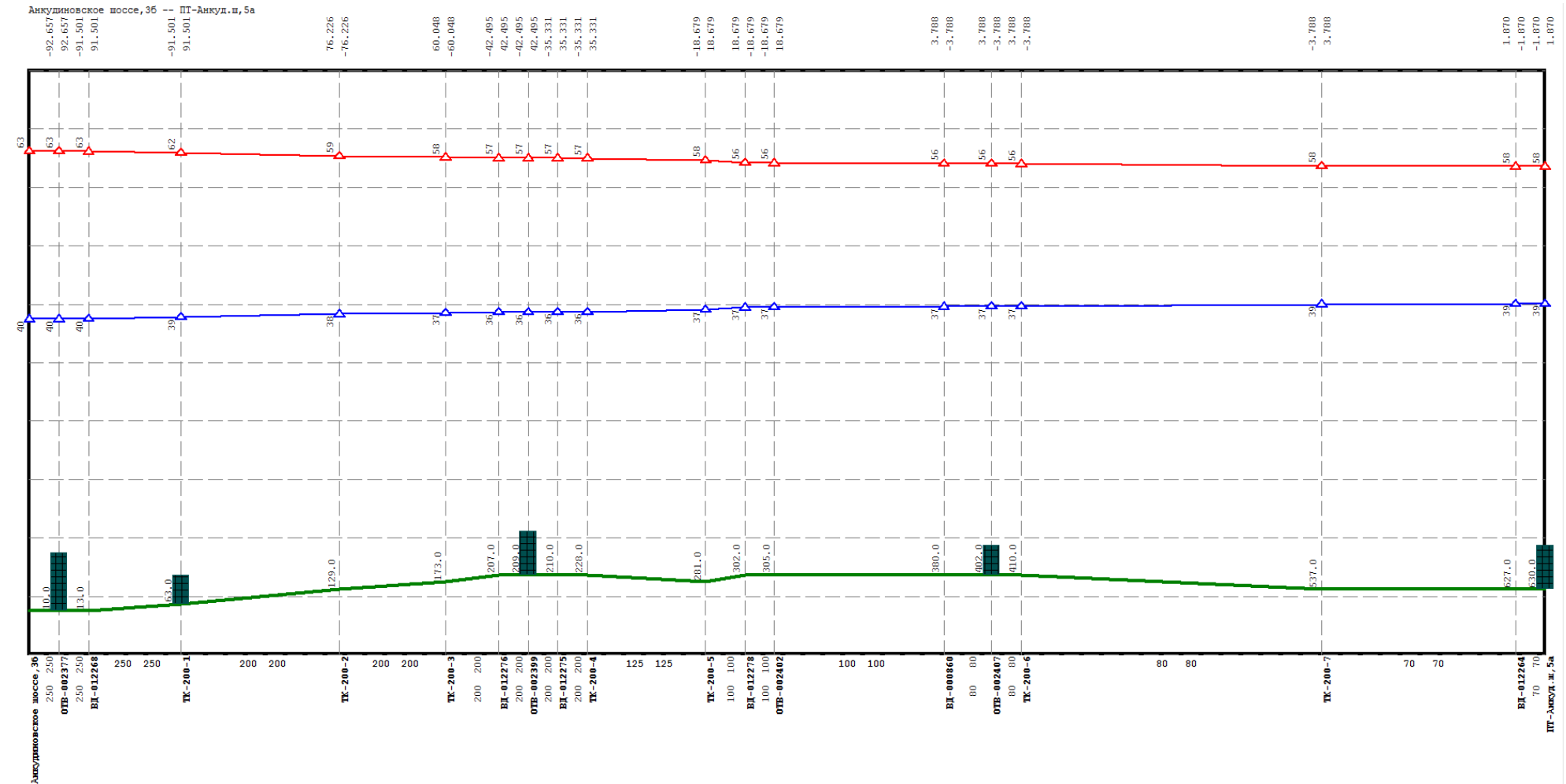
Рисунок 1.92 Результат гидравлического расчета - график гидравлических режимов по пути теплоносителя от котельной Ангудиновское шоссе, 3-б до ПТ-Анкул.ш,5а
