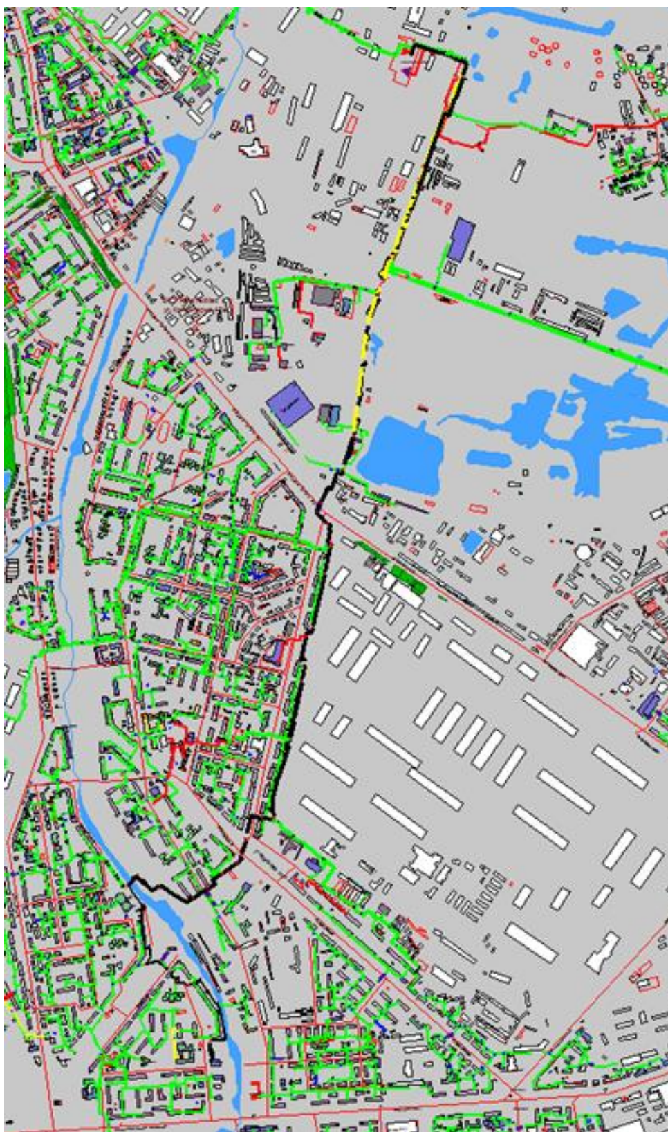
Рисунок 1.1 Результат гидравлического расчета - расчетный путь теплоносителя от СТЭЦ до ПТ-Люкина,5 аптека
