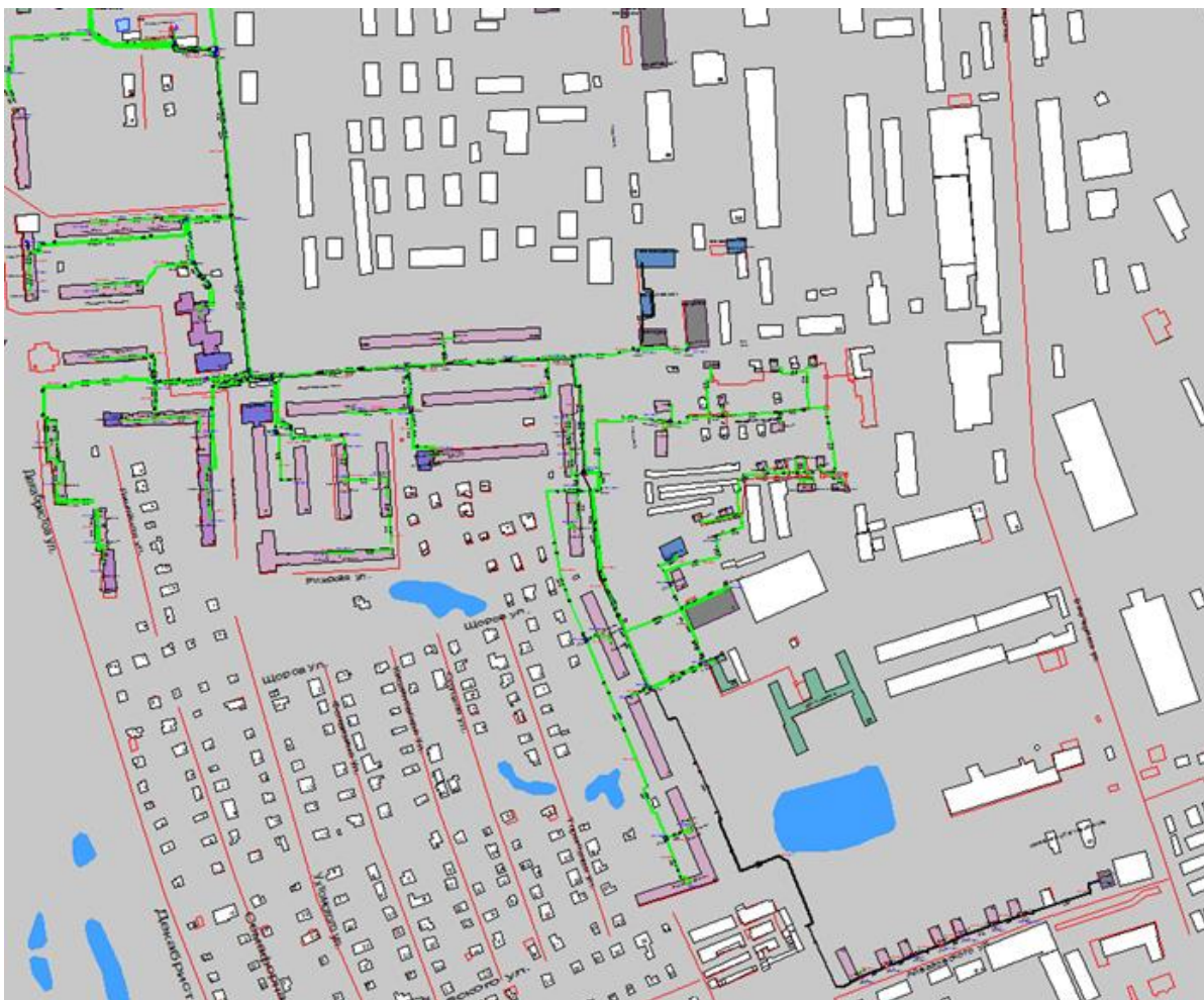
Рисунок 1.17 Результат гидравлического расчета - расчетный путь теплоносителя от котельной Лесной городок, 6в до ПТ-Вторчер,6а
