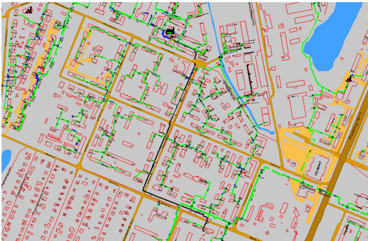
Рисунок 1.107 Результат гидравлического расчета - расчетный путь теплоносителя от котельной Премудрова, 12а до ПТ-Дружбы,56
