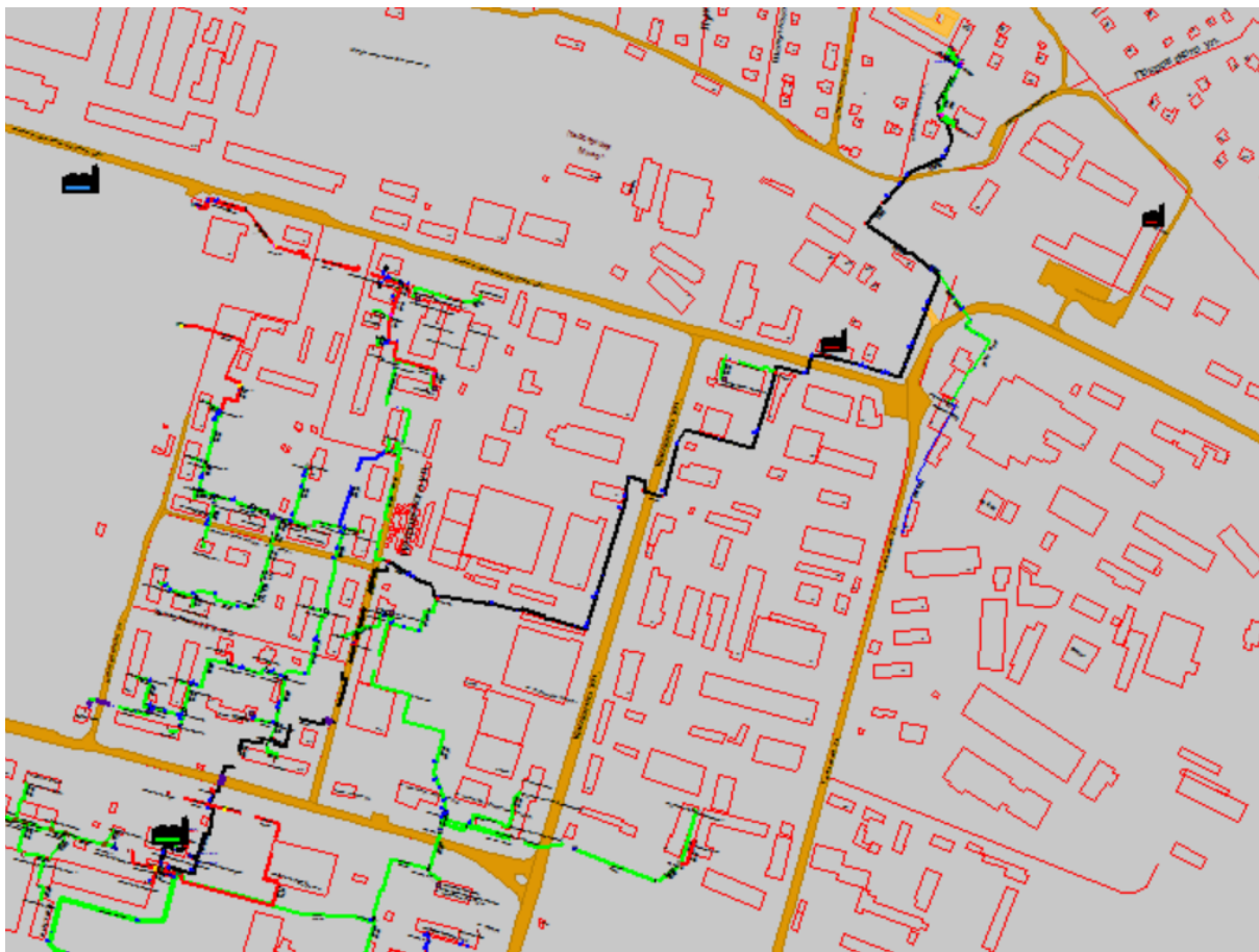
Рисунок 1.59 Результат гидравлического расчета - расчетный путь теплоносителя от котельной пр. Гагарина, 1786 до ЦТП-706
