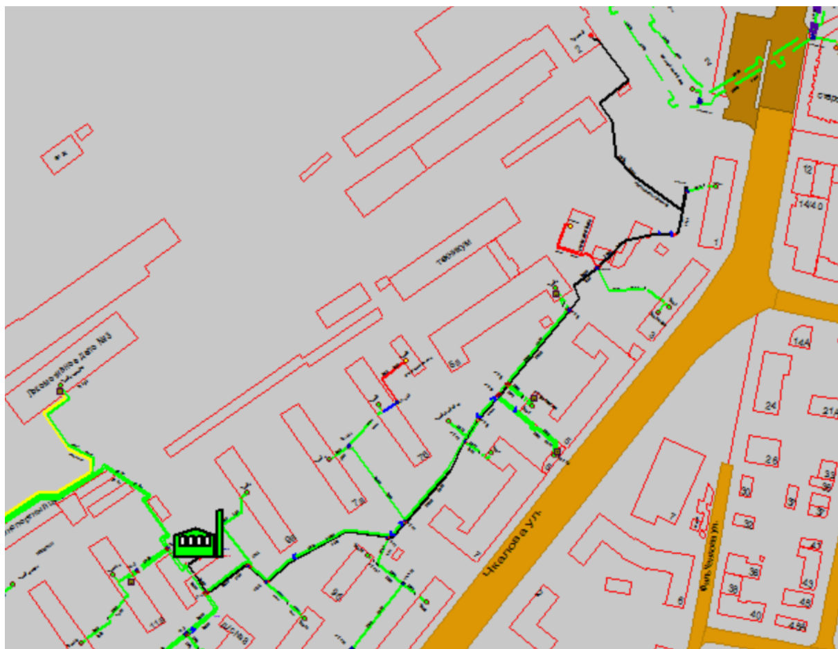
Рисунок 1.95 Результат гидравлического расчета - расчетный путь теплоносителя от котельной Чкалова, 9д до ПТ-Революц.пл,2
