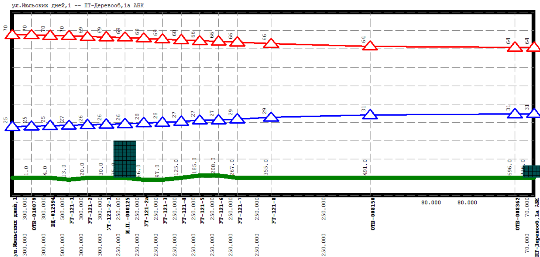
Рисунок 1.26 Результат гидравлического расчета - график гидравлических режимов по пути теплоносителя от котельной Июльских дней, 1 до ПТ-Деревооб,1а АВК
