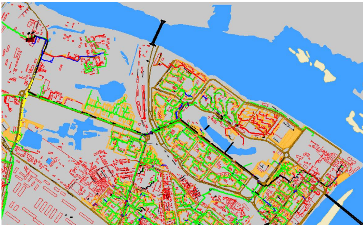
Рисунок 1.5 Результат гидравлического расчета - расчетный путь теплоносителя от СТЭЦ до ПТ-Стрел,19
