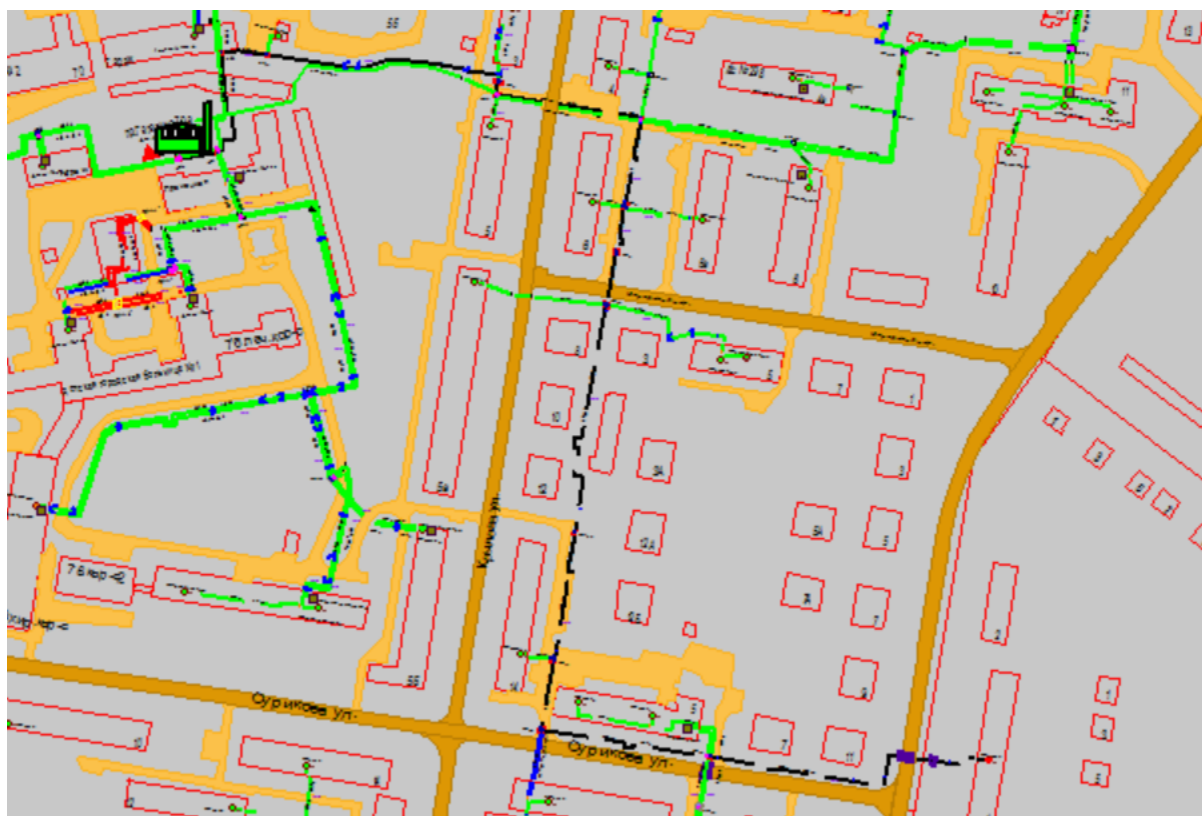
Рисунок 1.45 Результат гидравлического расчета - расчетный путь теплоносителя от котельной пр. Гагарина, 70а до ПТ-Корейск,4
