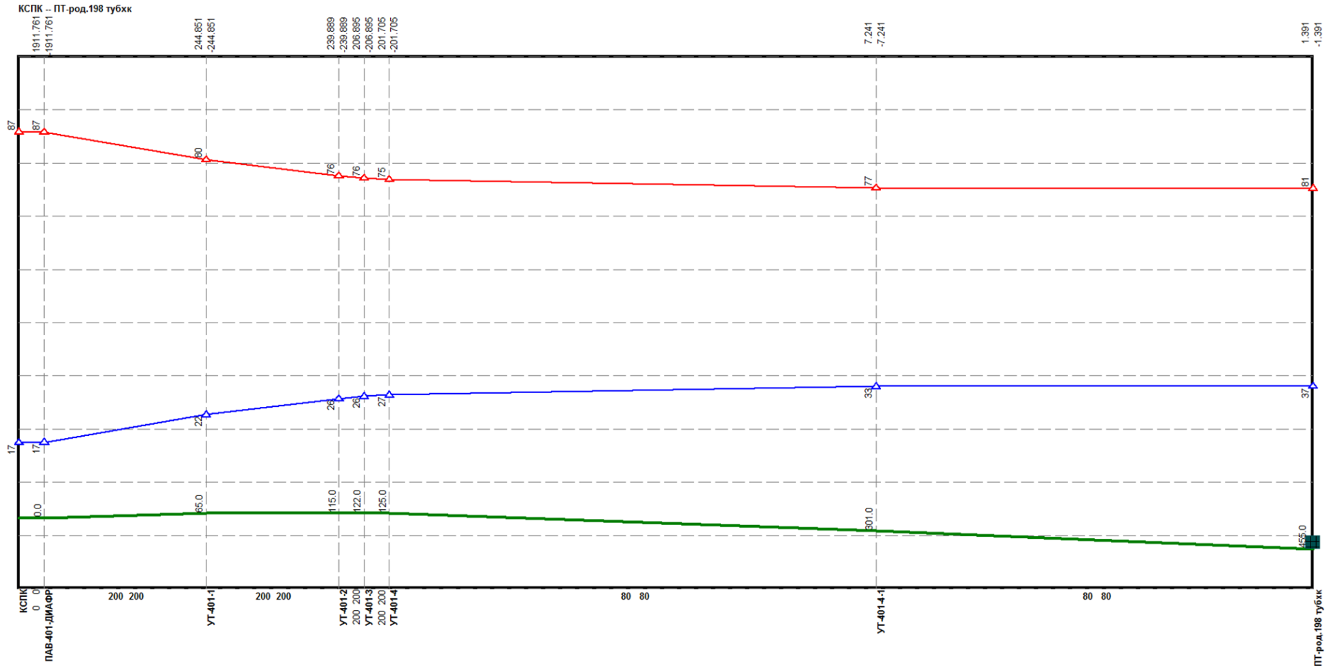
Рисунок 1.68 Результат гидравлического расчета - график гидравлических режимов по пути теплоносителя от котельной ул. Родионова, 194б до ПТ-род.198 тубхк
