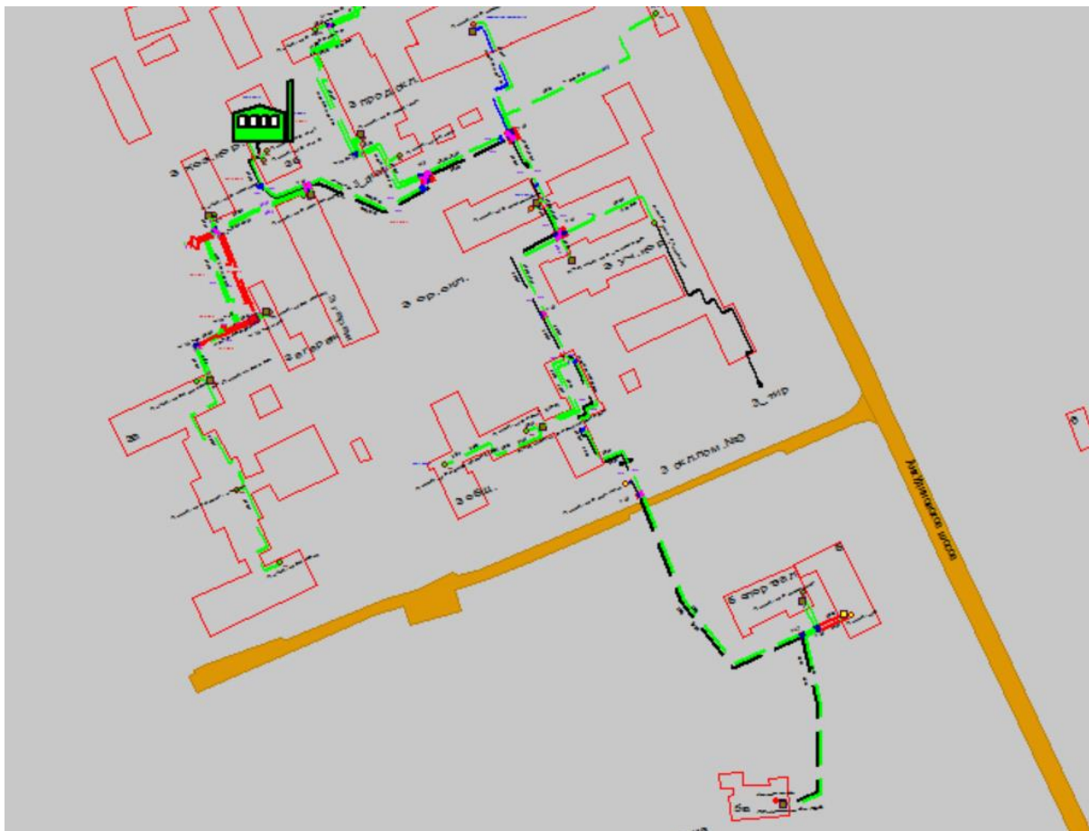
Рисунок 1.91 Результат гидравлического расчета - расчетный путь теплоносителя от котельной Анкудиновское шоссе, 3-б до ПТ-Анкуд.ш,5а
