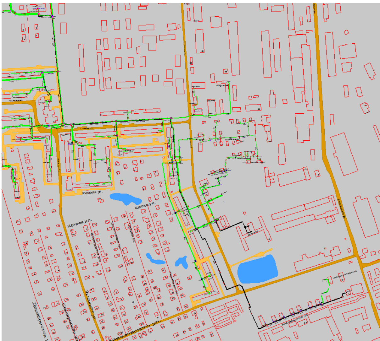
Рисунок 1.17 Результат гидравлического расчета - расчетный путь теплоносителя от котельной Лесной городок, 6в до ПТ-Вторчер,6а
