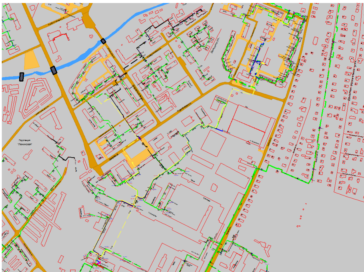
Рисунок 1.13 Результат гидравлического расчета - расчетный путь теплоносителя от котельной Памирская, 11 до ПТ-Сафрон, 15 вв2
