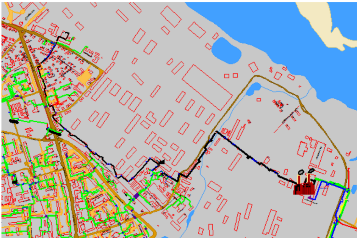
Рисунок 1.7 Результат гидравлического расчета - расчетный путь теплоносителя от СТЭЦ до ПТ-Свободы,57 ПЭКпр.1эт
