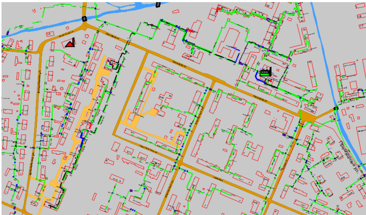
Рисунок 1.109 Результат гидравлического расчета - расчетный путь теплоносителя от котельной Премудрова, 12а до ПТ-Днепр,16 э4
