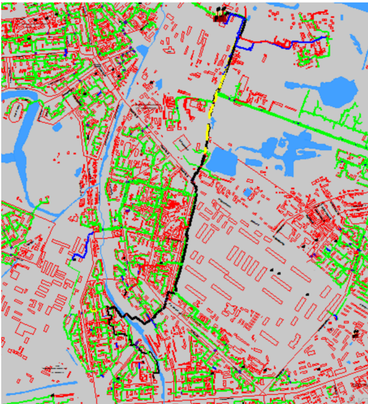
Рисунок 1.1 Результат гидравлического расчета - расчетный путь теплоносителя от СТЭЦ до ПТ-Люкина,5 аптека
