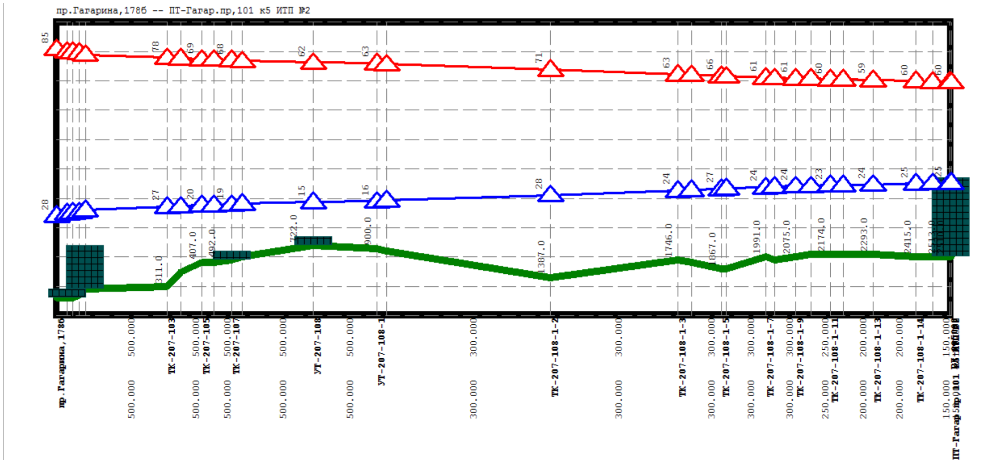
Рисунок 1.58 Результат гидравлического расчета - график гидравлических режимов по пути теплоносителя от котельной пр. Гагарина, 1786 до ИТ-Гагар.пр,101/5 ИТП №2
