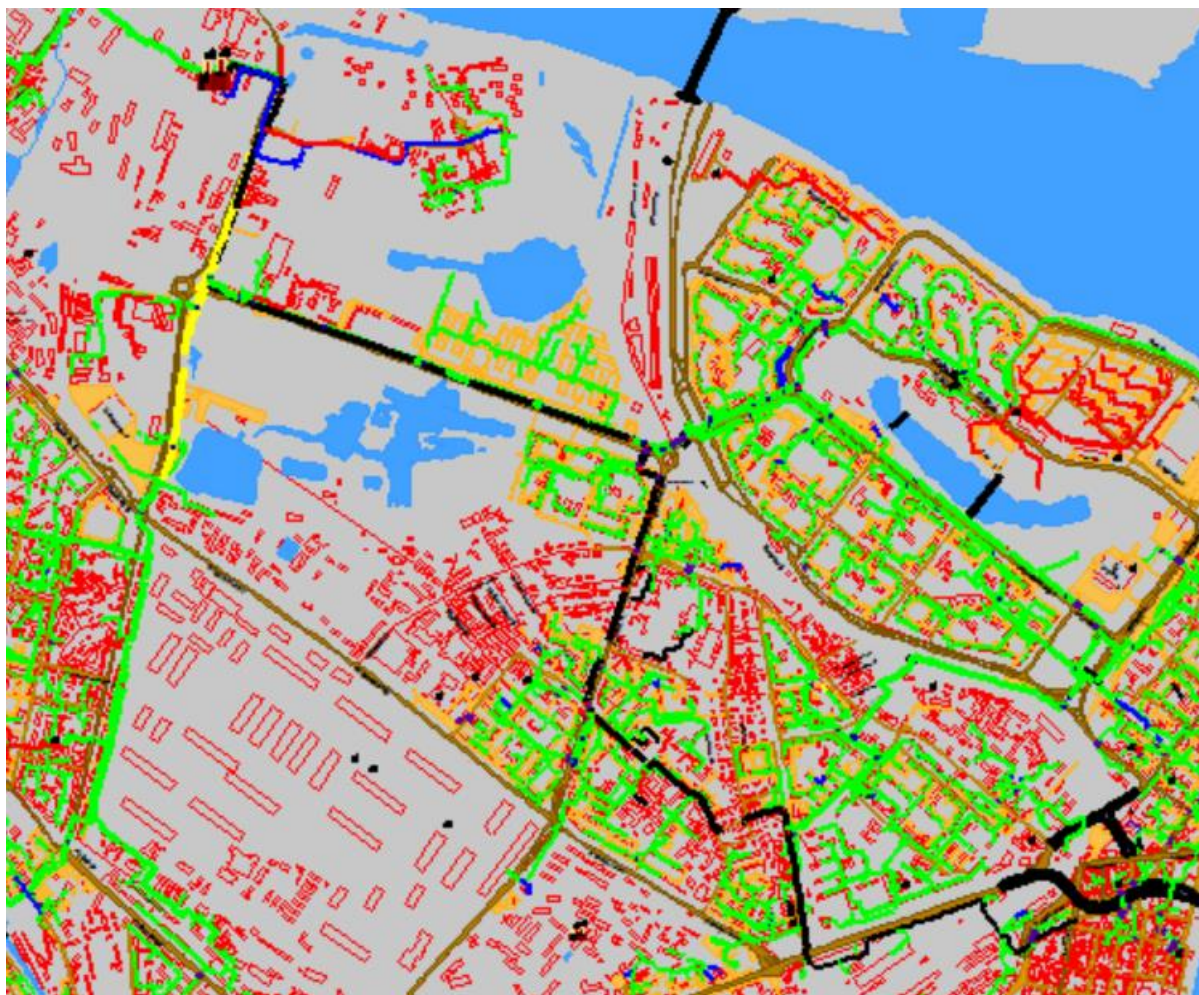
Рисунок 1.3 Результат гидравлического расчета - расчетный путь теплоносителя от СТЭЦ до ПТ-пл.Револ,7 вест2
