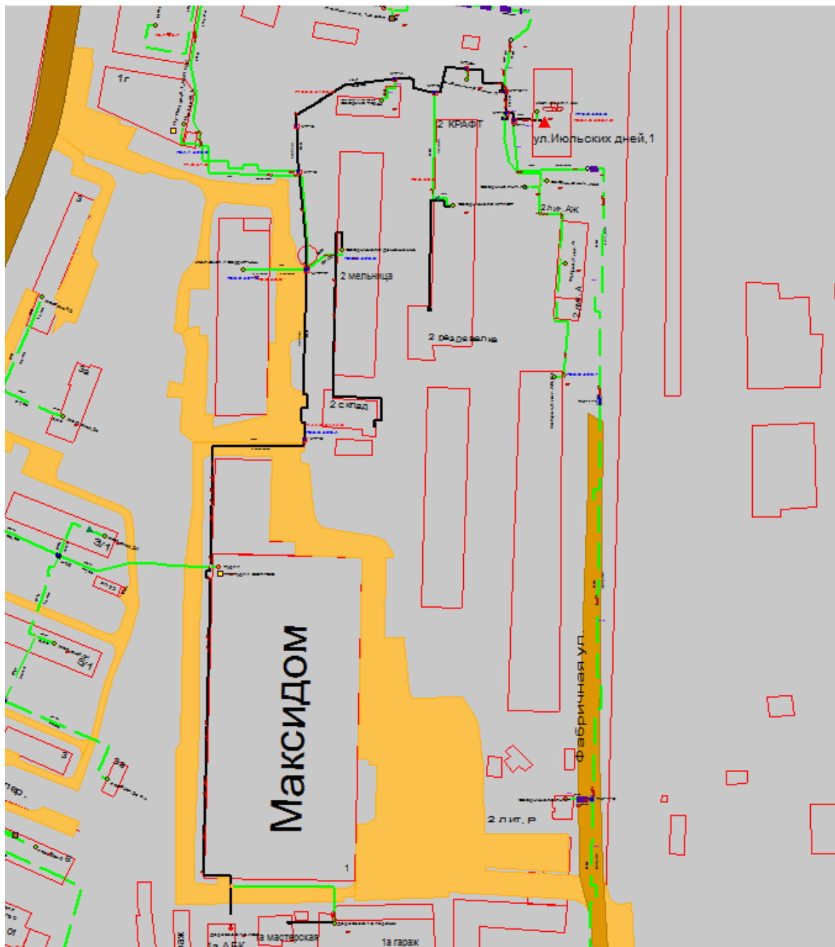
Рисунок 1.25 Результат гидравлического расчета - расчетный путь теплоносителя от Июльских дней, 1 до ПТ-Деревооб,1а АБК
