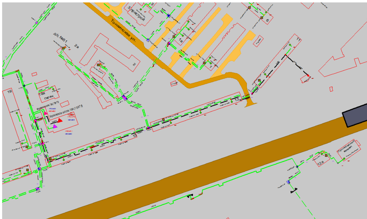
Рисунок 1.27 Результат гидравлического расчета - расчетный путь теплоносителя от котельной Московское шоссе, 15а до ПТ-Моск.ш,11а
