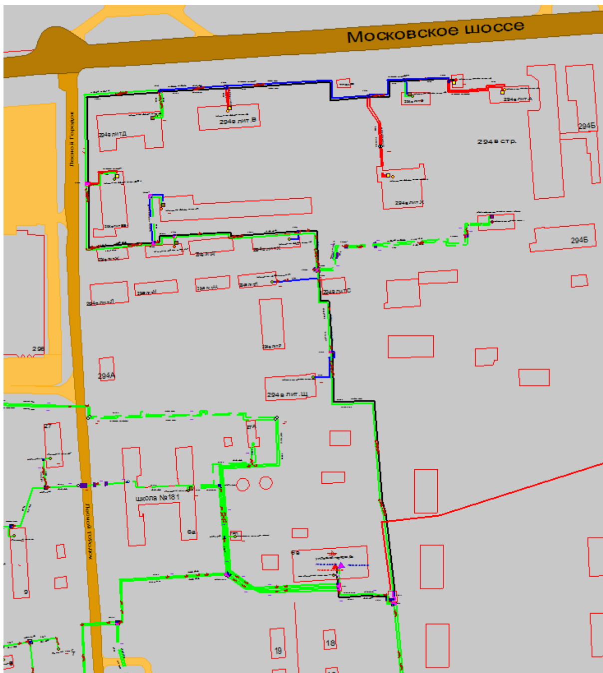
Рисунок 1.19 Результат гидравлического расчета - расчетный путь теплоносителя от котельной Лесной городок, 6в до ПТ-Моск.ш,294в лит.Б
