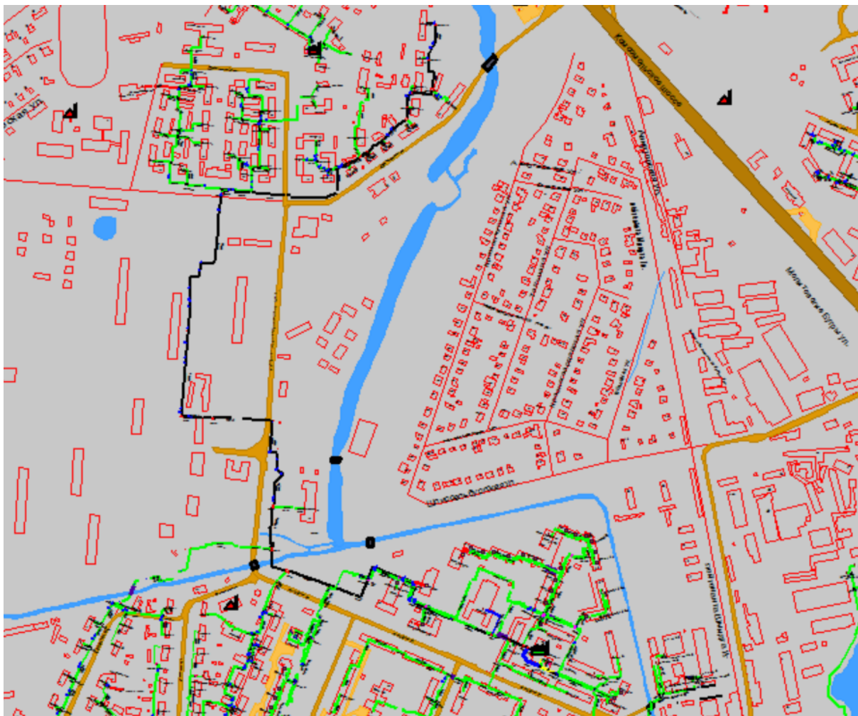
Рисунок 1.111 Результат гидравлического расчета - расчетный путь теплоносителя от котельной Премудрова, 12а до ПТ-Дачная,14)
