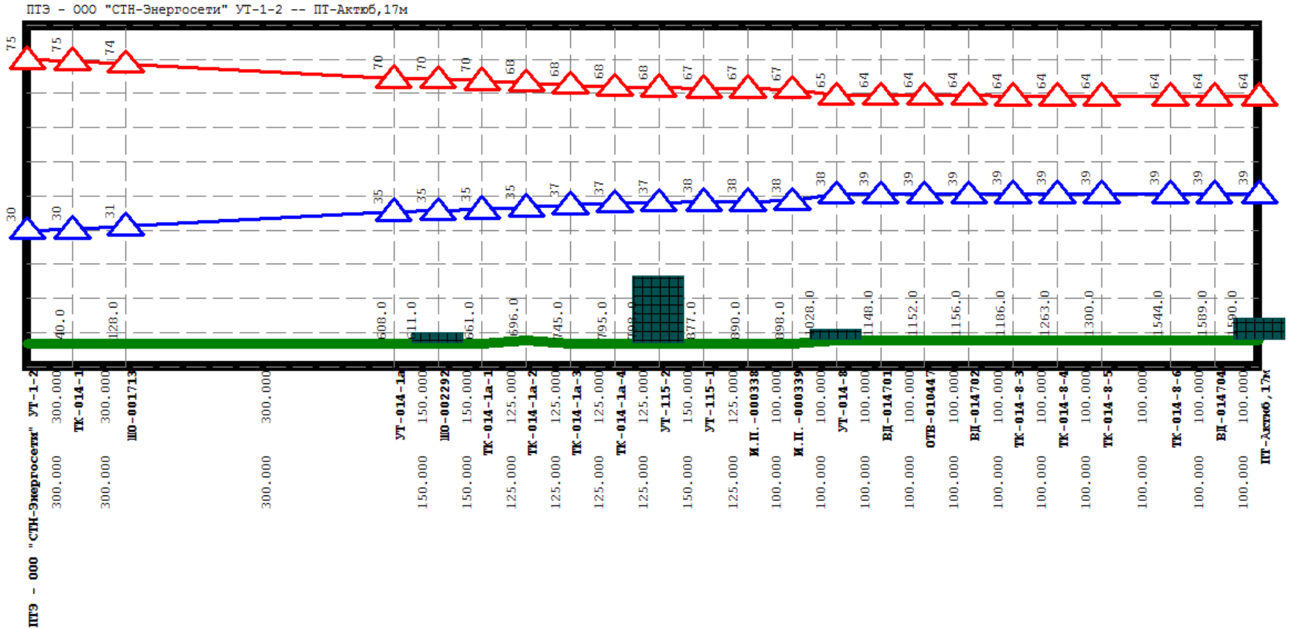
Рисунок 1.84 Результат гидравлического расчета - график гидравлических режимов по пути теплоносителя от котельной Московское шоссе, 62 до ПТ-Актьб.17м.
