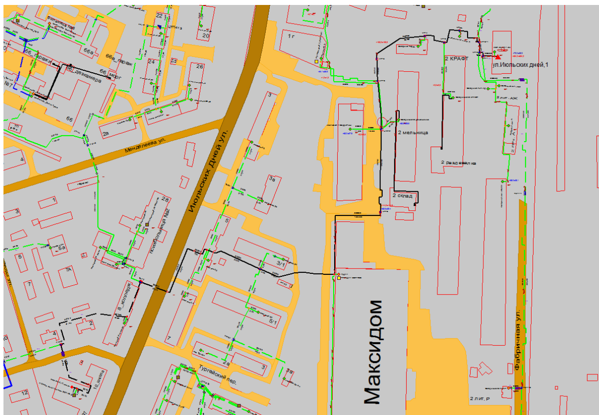
Рисунок 1.23 Результат гидравлического расчета - расчетный путь теплоносителя от Июльских дней, 1 до ПТ-Июл.дней,10 школа
