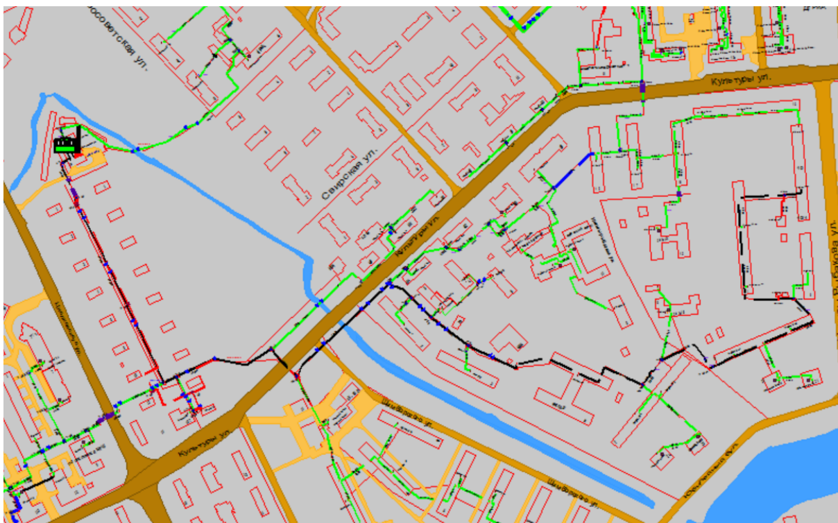
Рисунок 1.121 Результат гидравлического расчета - расчетный путь теплоносителя от котельной Коперника, 1-а до ПТ-Рыбак,10/1
