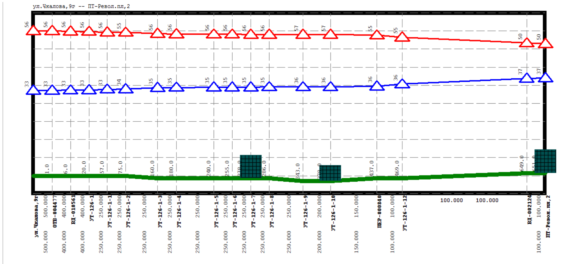
Рисунок 1.96 Результат гидравлического расчета - график гидравлических режимов по пути теплоносителя от котельной Чкалова, 9 до ПТ-Революция, 2
