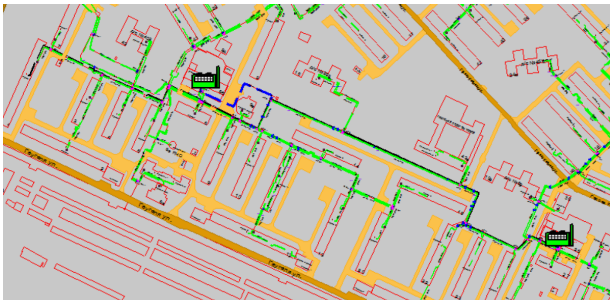
Рисунок 1.71 Результат гидравлического расчета - расчетный путь теплоносителя от котельной ул. Гаугеля, 25 до ПТ-Гаугеля,1
