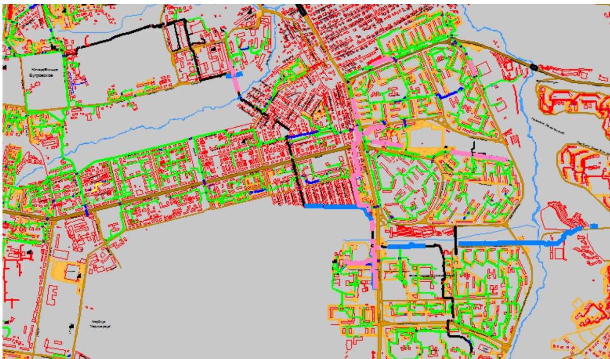
Рисунок 1.49 Результат гидравлического расчета - расчетный путь теплоносителя от котельной НТЦ до ПТ-Малин,2 пристрой
