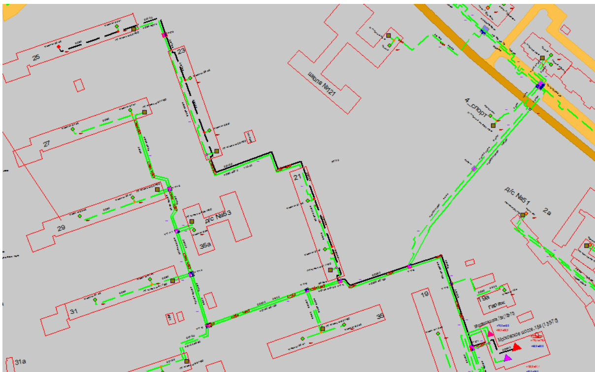
Рисунок 1.29 Результат гидравлического расчета - расчетный путь теплоносителя от котельной Московское шоссе, 15а до ПТ-Моск.ш,25 э2
