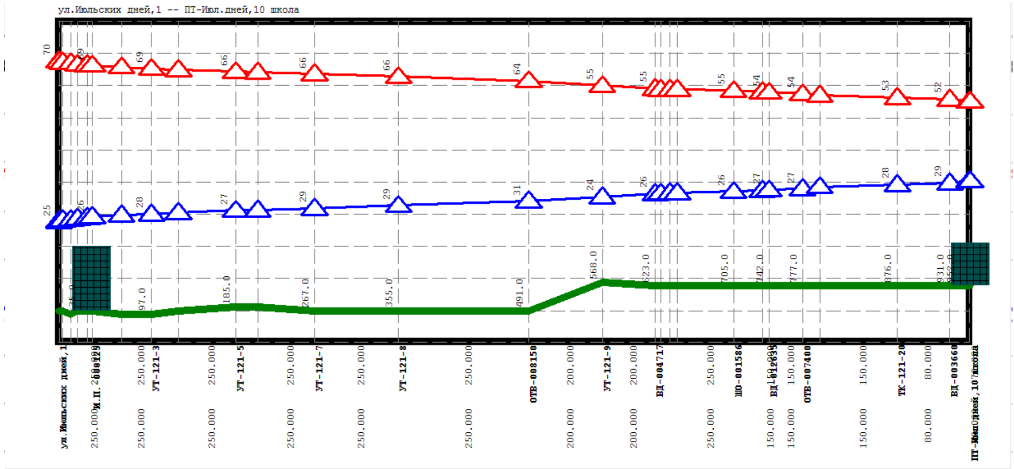
Рисунок 1.24 Результат гидравлического расчета - график гидравлических режимов по пути теплоносителя от Июльских дней, 1 ПТ-Июльские дни, 10 школа
