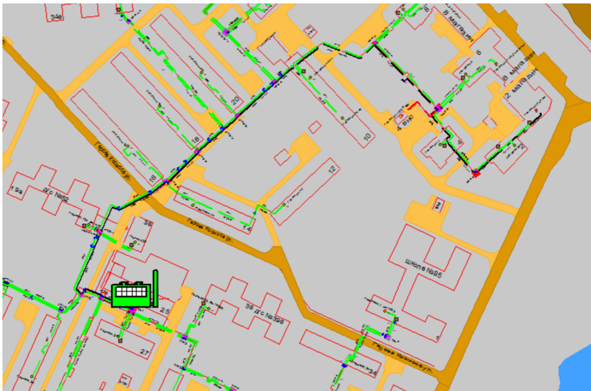
Рисунок 1.73 Результат гидравлического расчета - расчетный путь теплоносителя от котельной ул. Гаугеля, 25 до ПТ-Гаугеля,1 до ПТ-Гер.Косм,2 кафе
