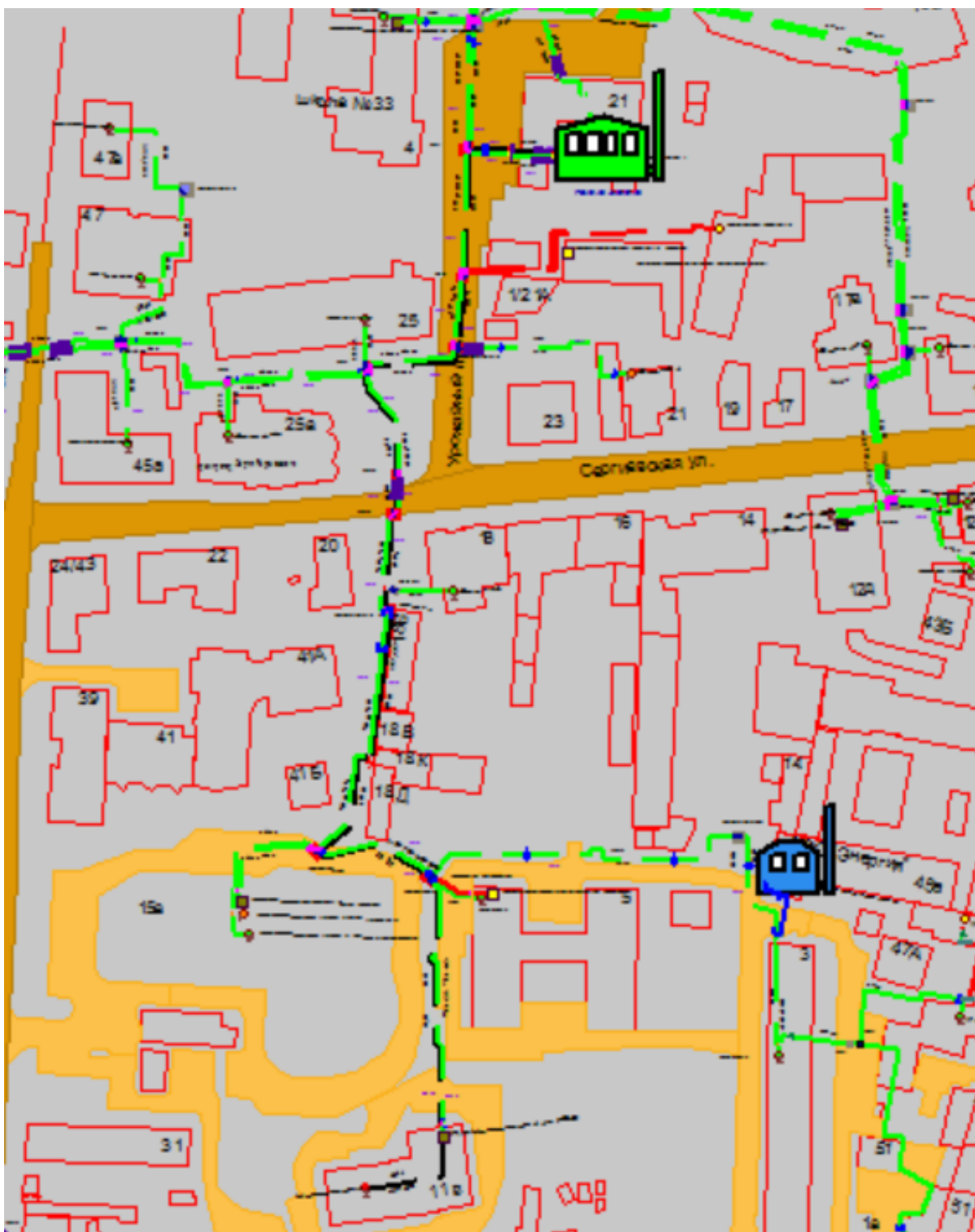
Рисунок 1.9 Результат гидравлического расчета - расчетный путь теплоносителя от котельной Суетинская, 21 до ПТ-Нтжегород,11в
