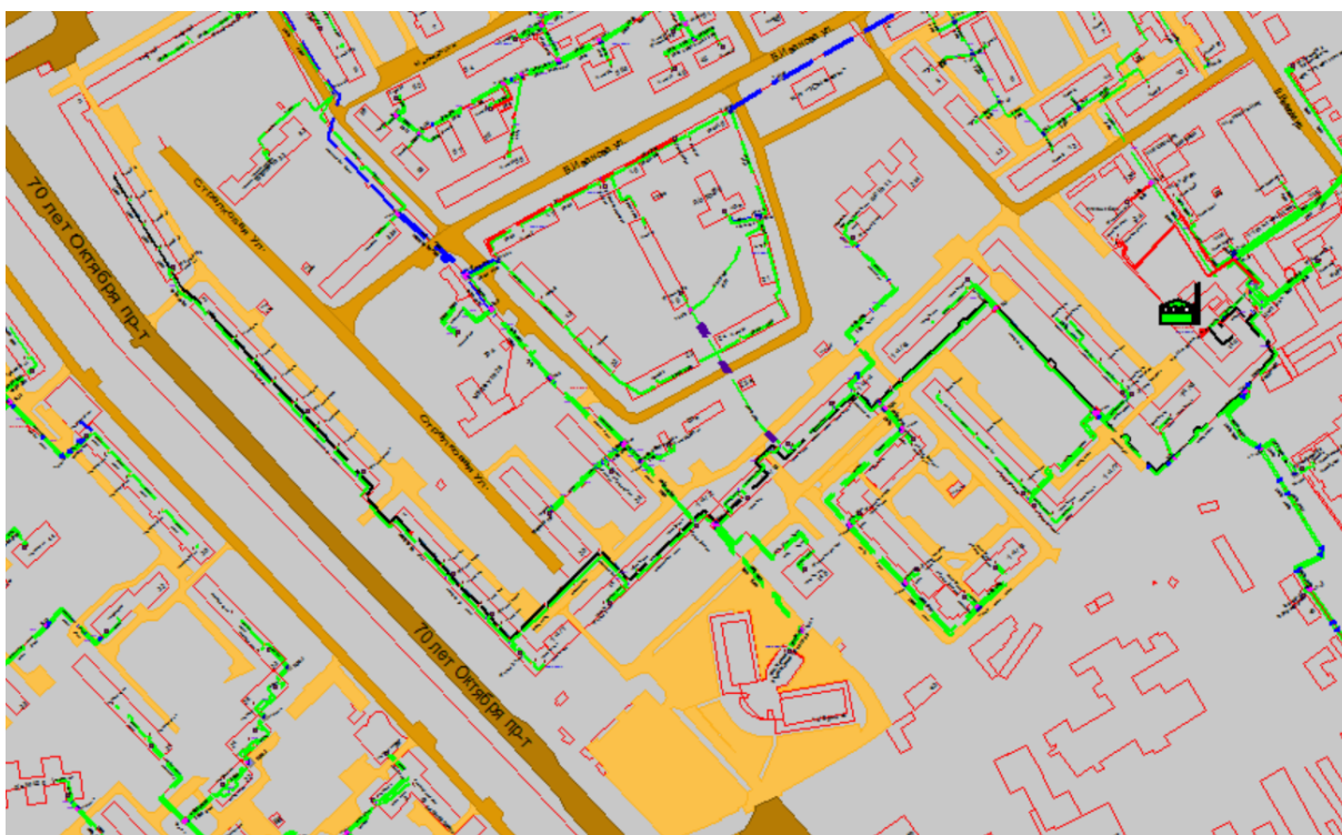
Рисунок 1.75 Результат гидравлического расчета - расчетный путь теплоносителя от котельной ул. Иванова, 14д до ПТ-Телег.3_э5
