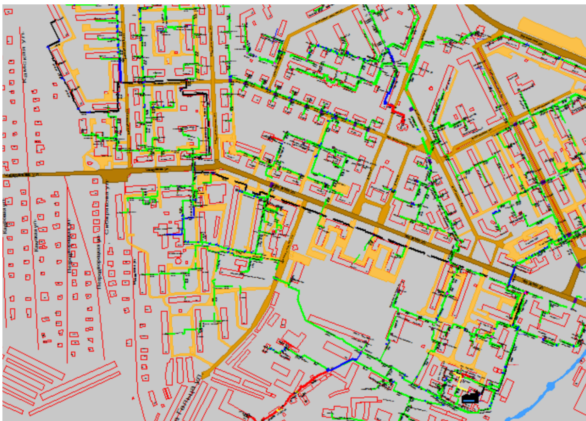
Рисунок 1.93 Результат гидравлического расчета - расчетный путь теплоносителя от котельной Чаадаева, 10 до ПТ-Мечн,63.
