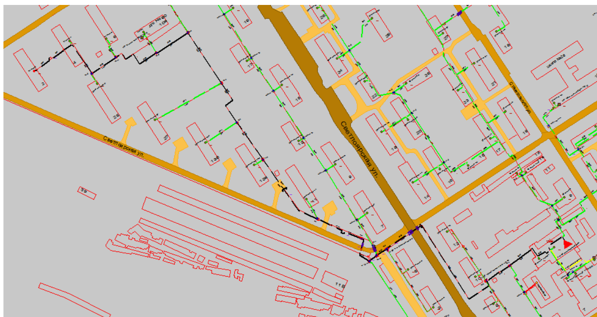
Рисунок 1.41 Результат гидравлического расчета - расчетный путь теплоносителя от котельной Станиславского, 3 до ПТ-Мокр,2
