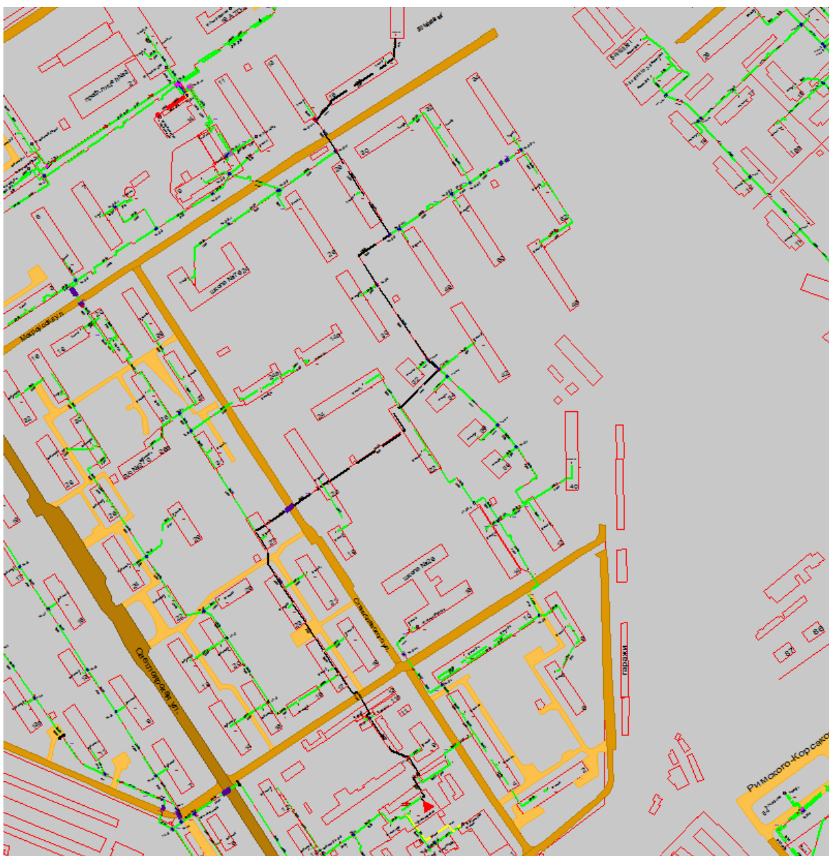
Рисунок 1.43 Результат гидравлического расчета - расчетный путь теплоносителя от котельной Станиславского, 3 до ПТ-Мокр,17
