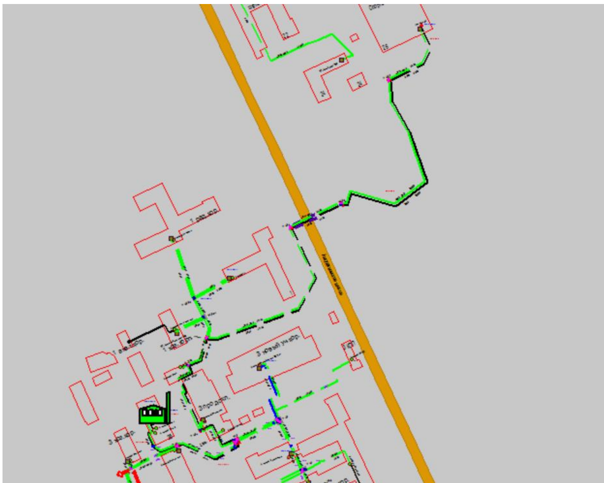
Рисунок 1.89 Результат гидравлического расчета - расчетный путь теплоносителя от котельной Анкудиновское шоссе, 3-б до ПТ-Корейск,26
