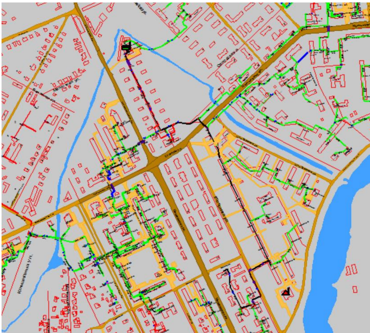
Рисунок 1.119 Результат гидравлического расчета - расчетный путь теплоносителя от котельной Коперника, 1-а до ПТ-Циол,32
