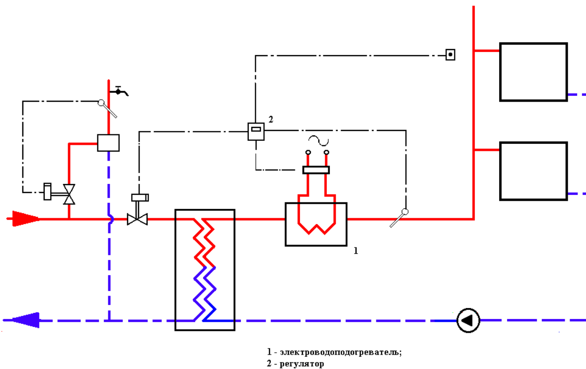
Рисунок 5.2 – – Схема теплового пункта с электроводоподогревателем
