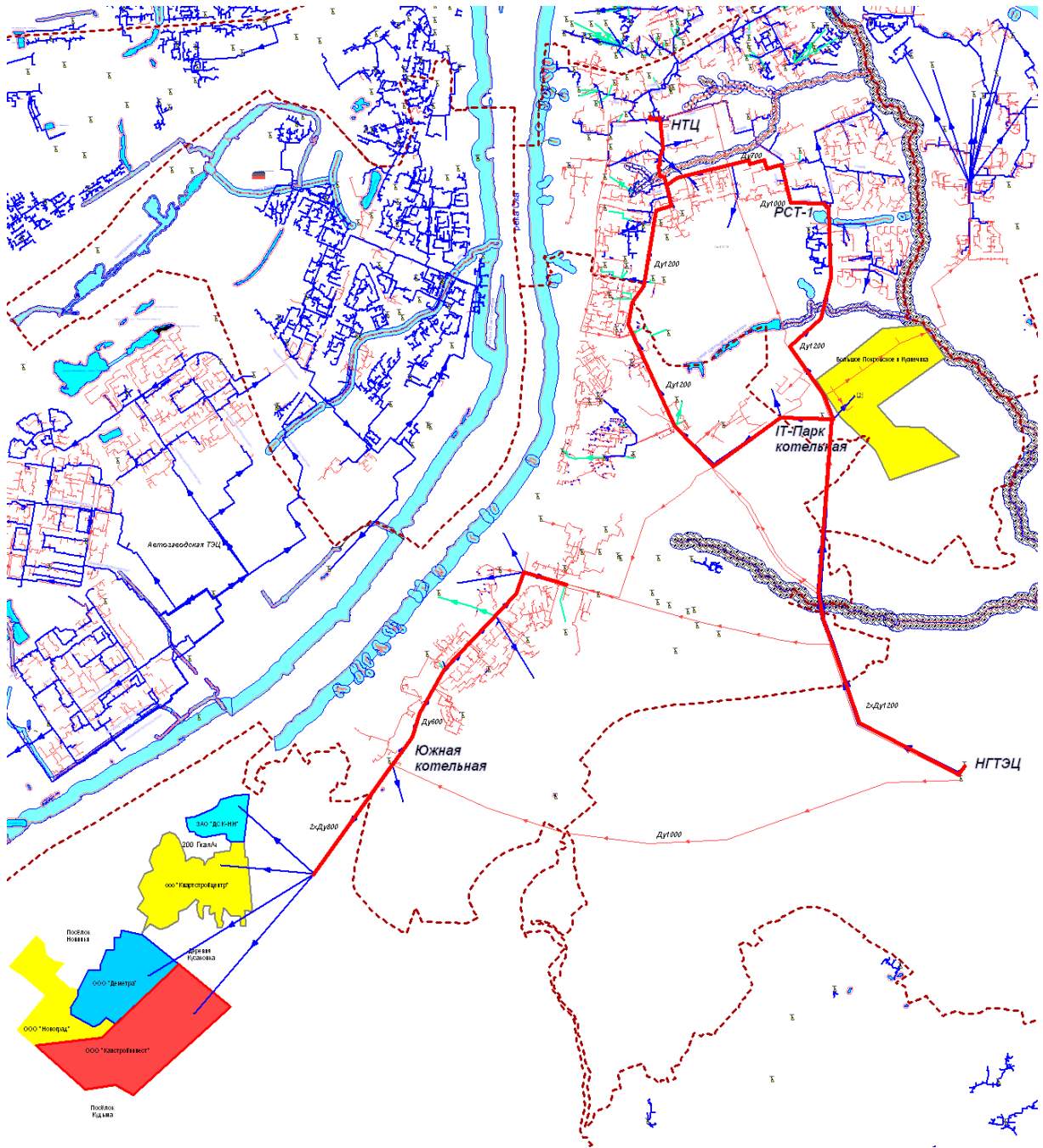
Рисунок 2.1 –Схема теплоснабжения зоны НТЦ от НГТЭС и котельной IT-Парк через РСТ-1 по т/м 1 и 3 очередей НТЦ и новой т/м Нартова
