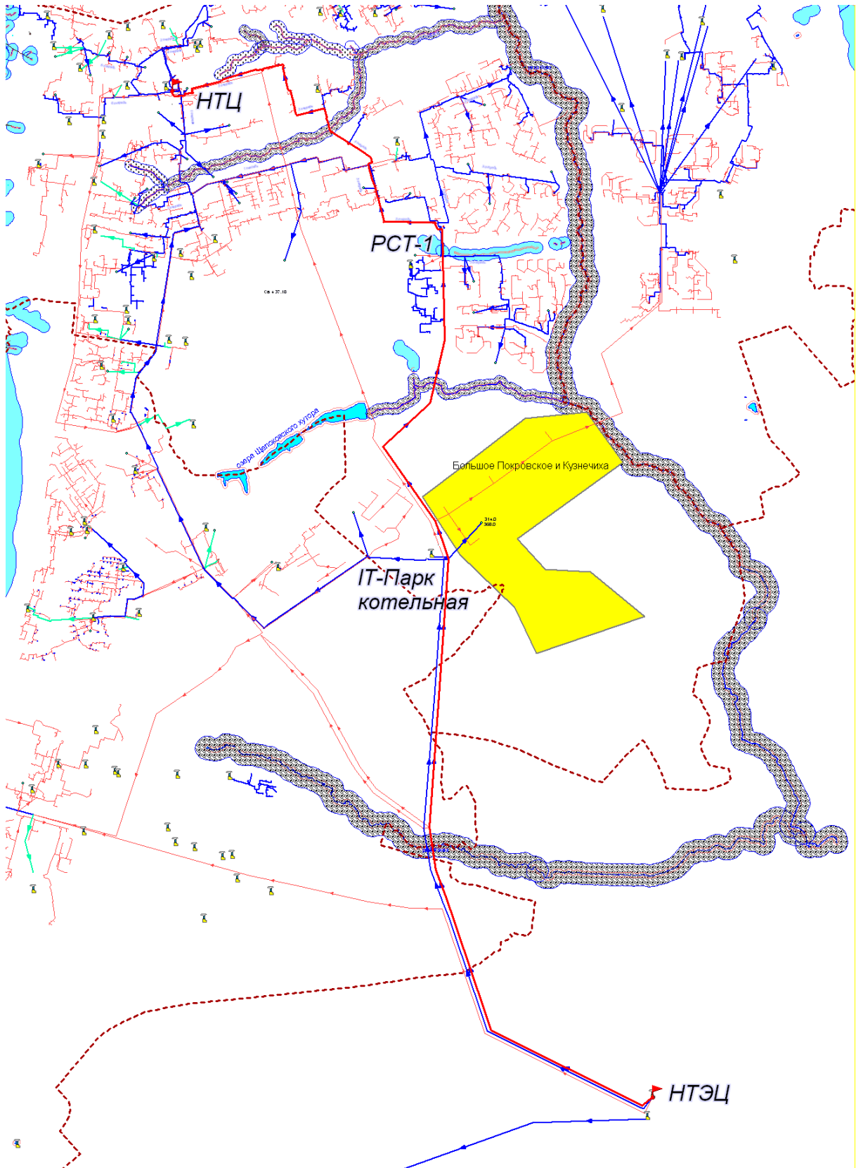
Рисунок 2.2 – Трасса от НПТЭЦ через котельную ИТ-Парка, через РСТ-1 по т/м «3 очередь» до НТЦ
