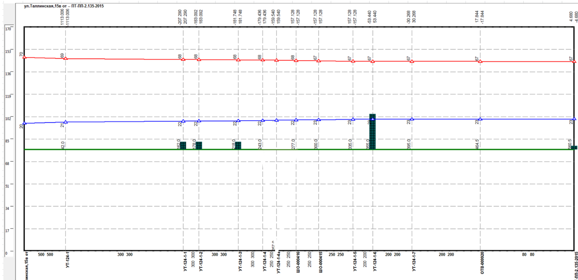
Рисунок 1.124 –Результат гидравлического расчета - график гидравлических режимов по пути теплоносителя от котельной Таллинская, 15в до ОТВ-009920
