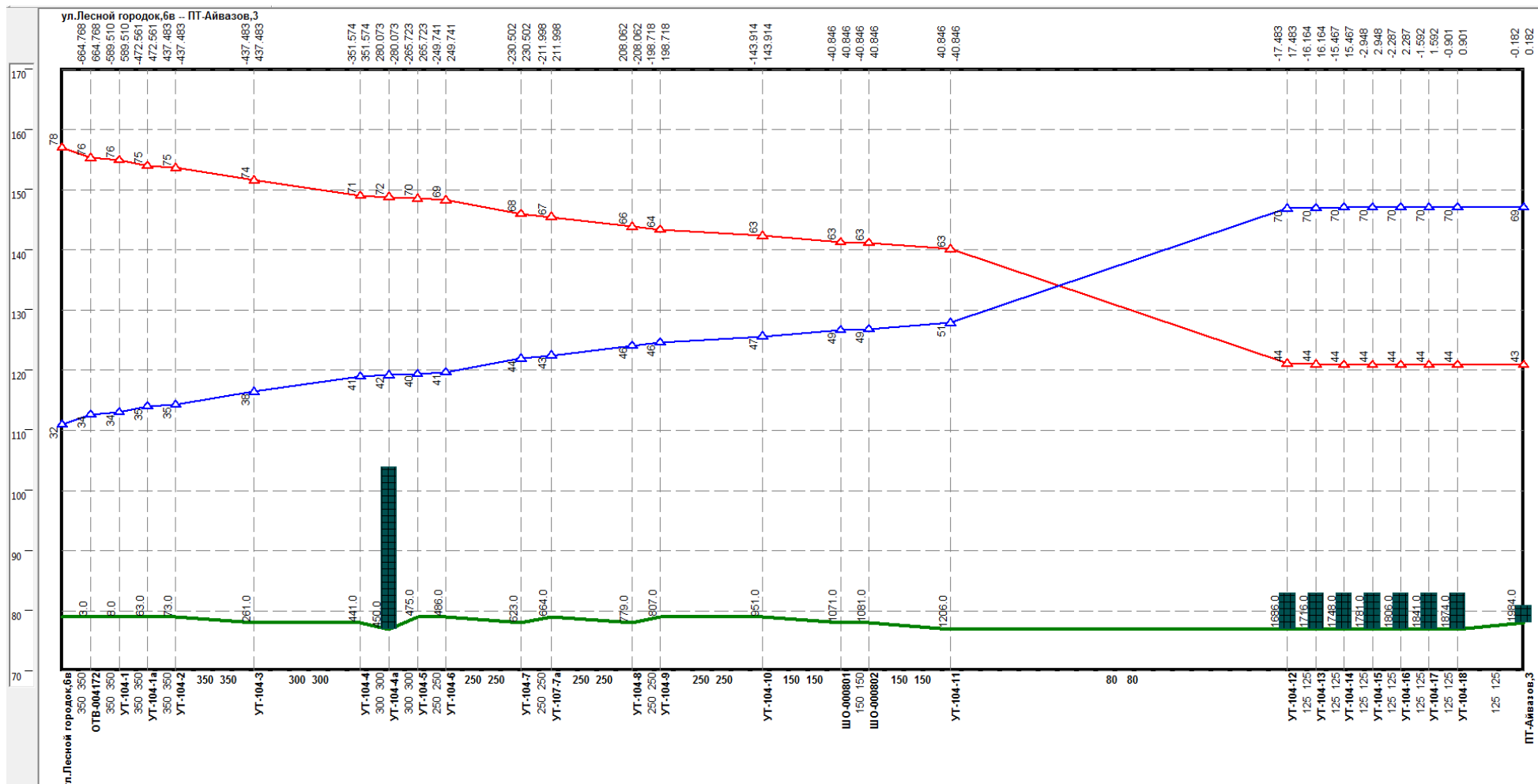
Рисунок 1.18 –Результат гидравлического расчета - график гидравлических режимов по пути теплоносителя от котельной Лесной городок, 6в до ПТ-Айвазов,3
