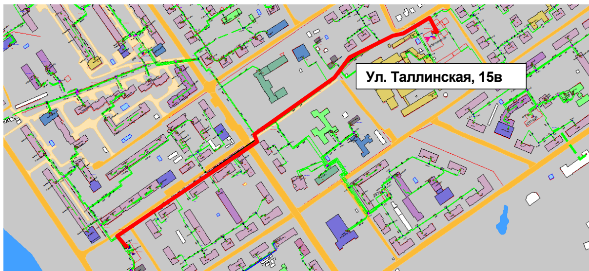
Рисунок 1.125 – Результат гидравлического расчета - расчетный путь теплоносителя от котельной Таллинская, 15в до ЦТП-204
