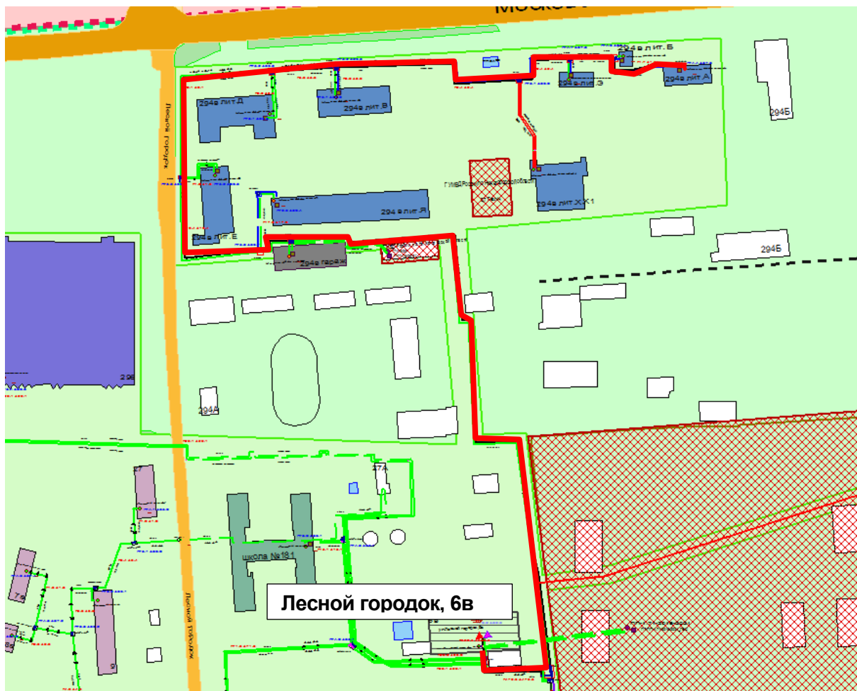
Рисунок 1.19 – Результат гидравлического расчета - расчетный путь теплоносителя от котельной Лесной городок 6в до ПТ-Моск.ш,294в лит.А
