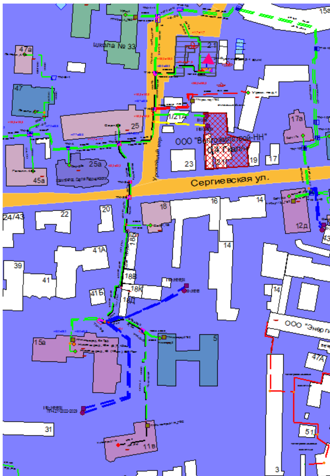
Рисунок 1.9 – Результат гидравлического расчета - расчетный путь теплоносителя от котельной Суетинская, 21 до ПТ-Нтжегород,11в
