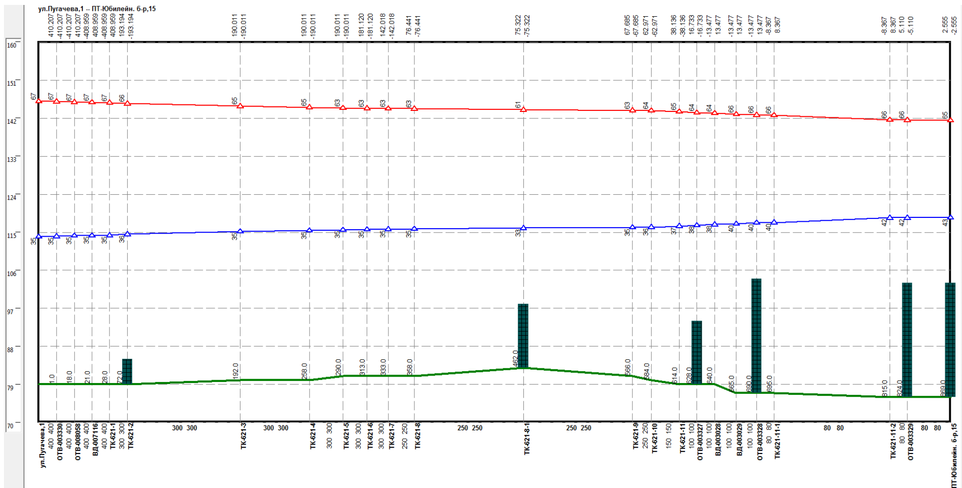
Рисунок 1.130 –Результат гидравлического расчета - график гидравлических режимов по пути теплоносителя от котельной Пугачева, 1 до ПТ-Юбилейн. б.р,15
