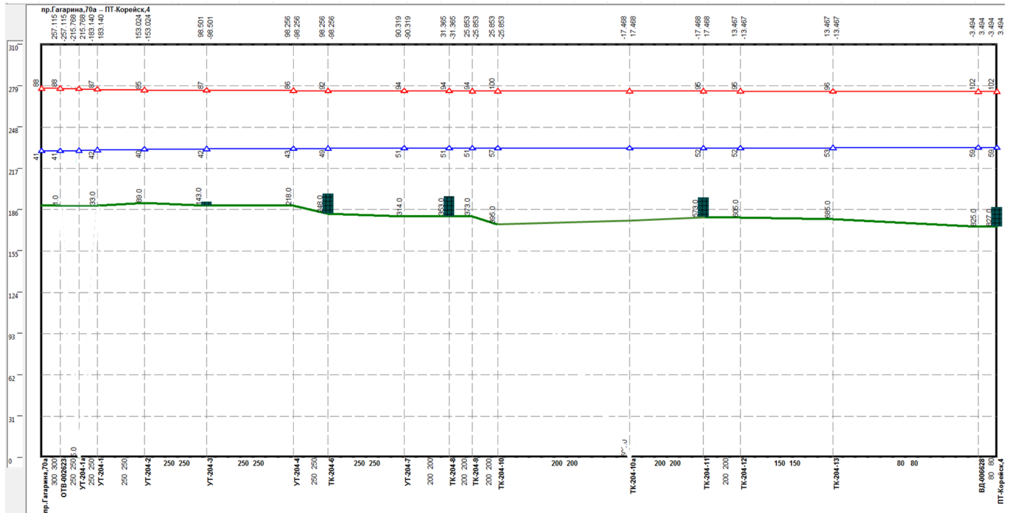
Рисунок 1.54 –Результат гидравлического расчета - график гидравлических режимов по пути теплоносителя от котельной пр. Гагарина, 70а до ПТ-Корейск,4
