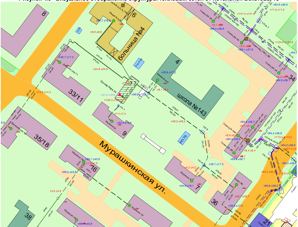
Рисунок 4.6 - Визуальное отображение структуры тепловых сетей от Котельной Бекетова, 13
