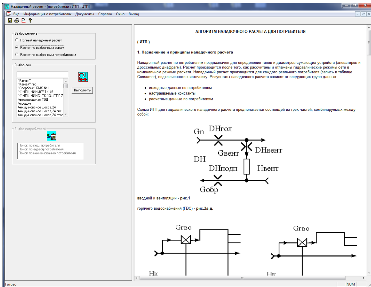
Рисунок 3.168 – Вид наладочного расчета
