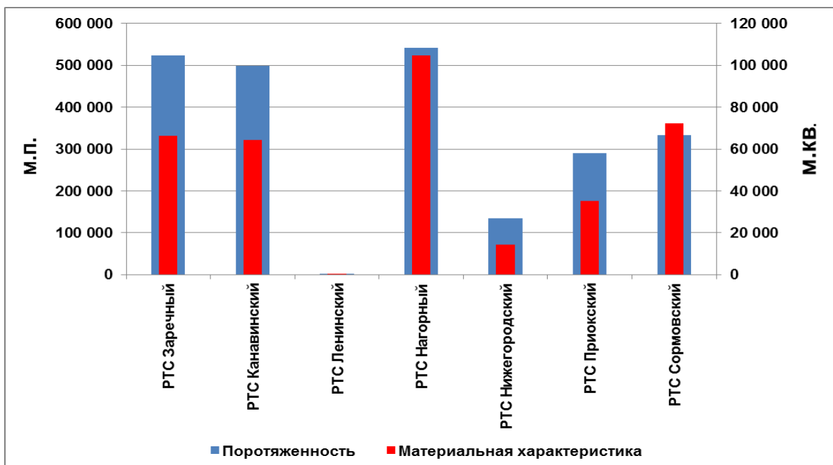
Рисунок 1.3 – Соотношение материальной характеристики и протяженности тепловых сетей ОАО «Теплоэнерго» по районам тепловых сетей
