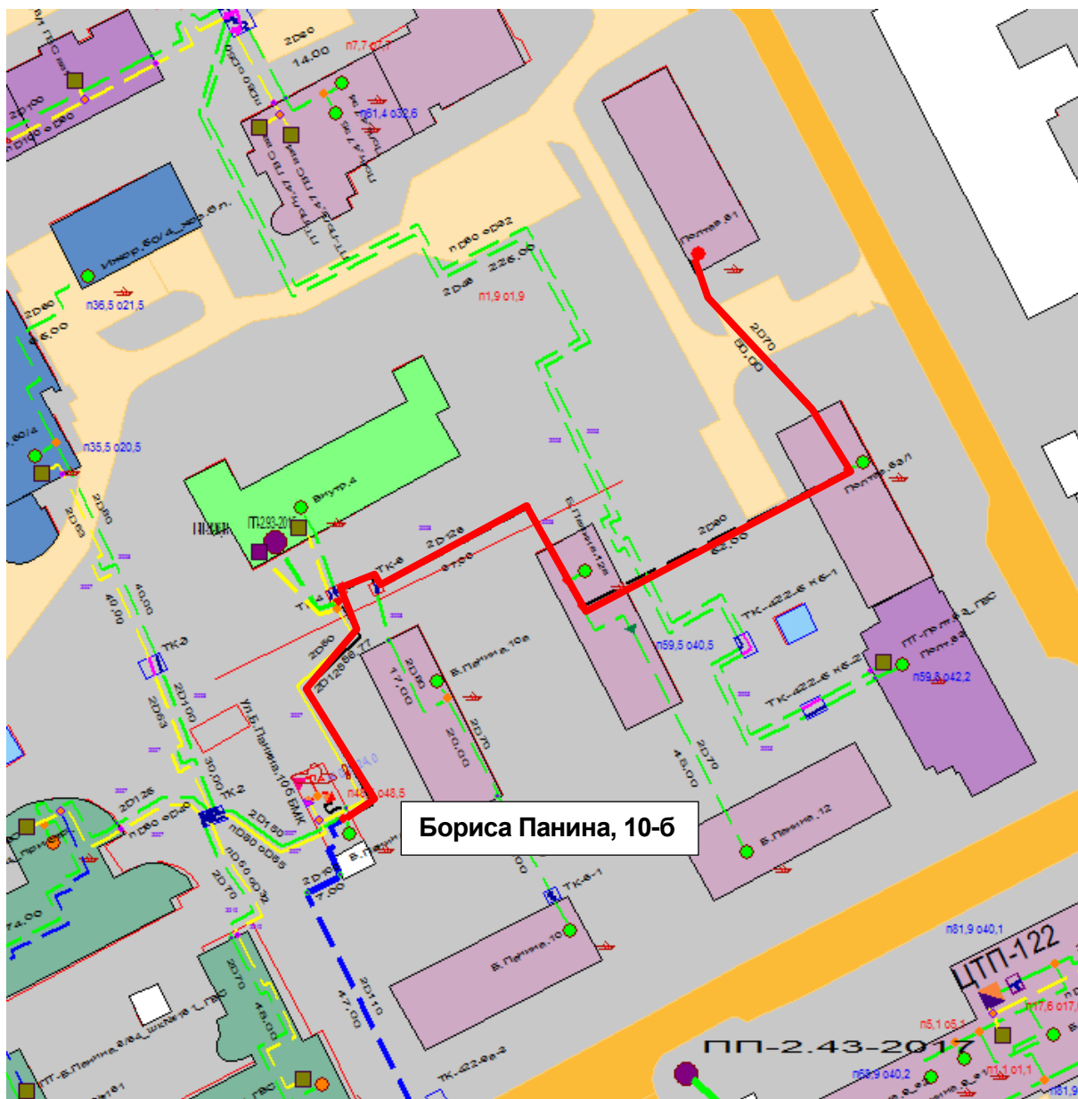
Рисунок Ошибка! Текст указанного стиля в документе отсутствует..177 – Результат гидравлического расчета - расчетный путь теплоносителя от котельной Бориса Панина, 10-б до ПТ-Полтав,51
