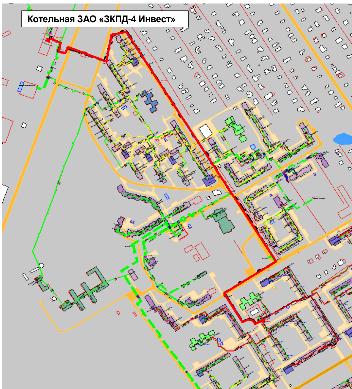
Рисунок Ошибка! Текст указанного стиля в документе отсутствует..149- Результат гидравлического расчета - расчетный путь теплоносителя от котельной ЗАО «ЗКПД-4 Инвест» до ПТ-Кораб,26/2 аптека
