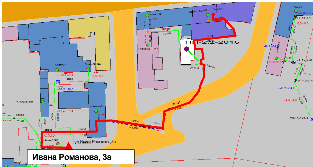
Рисунок 1.143 - Результат гидравлического расчета - расчетный путь теплоносителя от котельной Ивана Романова до ПТ-Совет, 11
