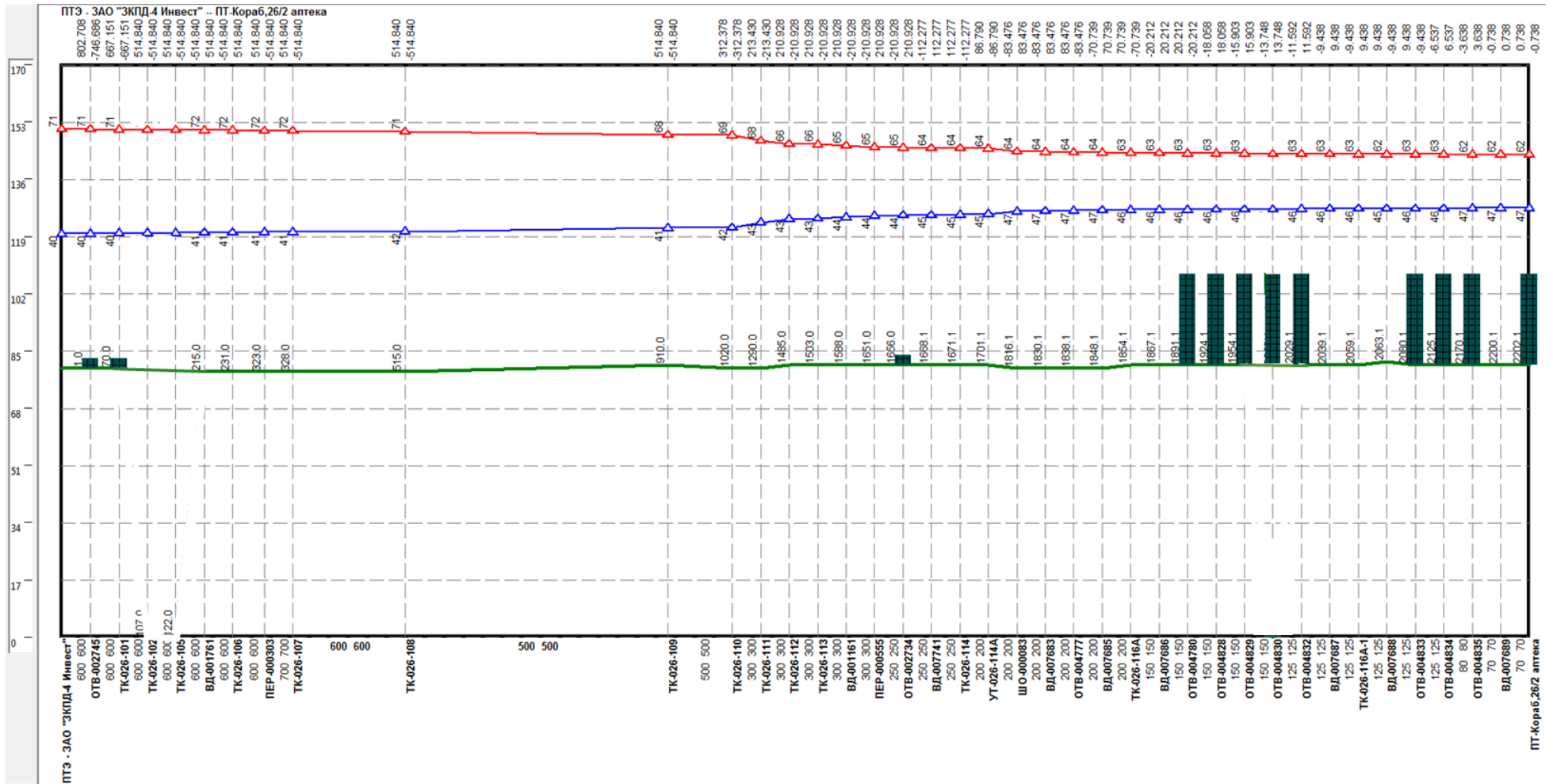
Рисунок Ошибка! Текст указанного стиля в документе отсутствует..150 –Результат гидравлического расчета - график гидравлических режимов по пути теплоносителя от котельной ЗАО «ЗКПД-4 Инвест» до ПТ-Кораб,26/2 аптека
