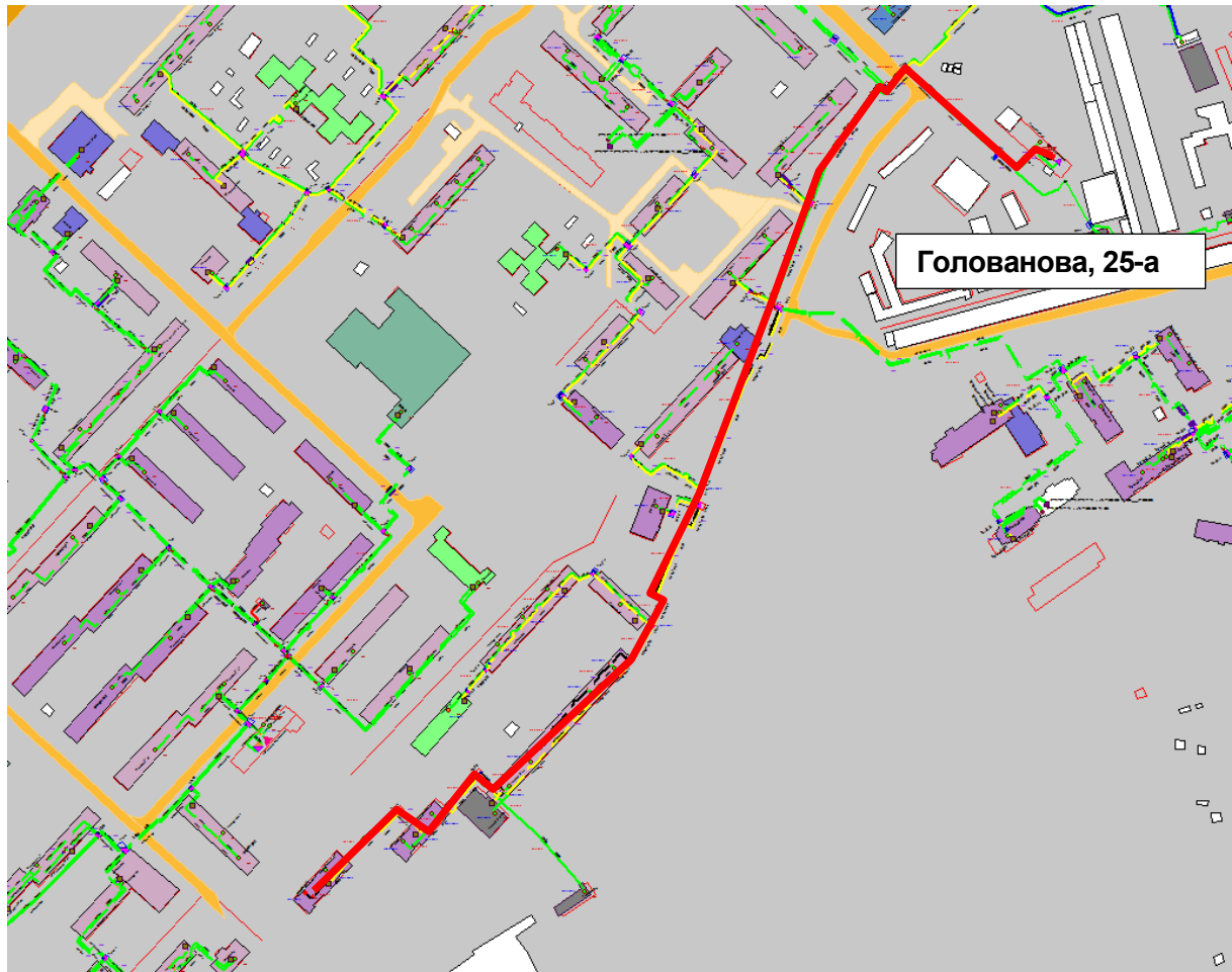
Рисунок Ошибка! Текст указанного стиля в документе отсутствует..219 – Результат гидравлического расчета - расчетный путь теплоносителя от котельной Голованова, 25-а до ПТ-Голован,57 э2
