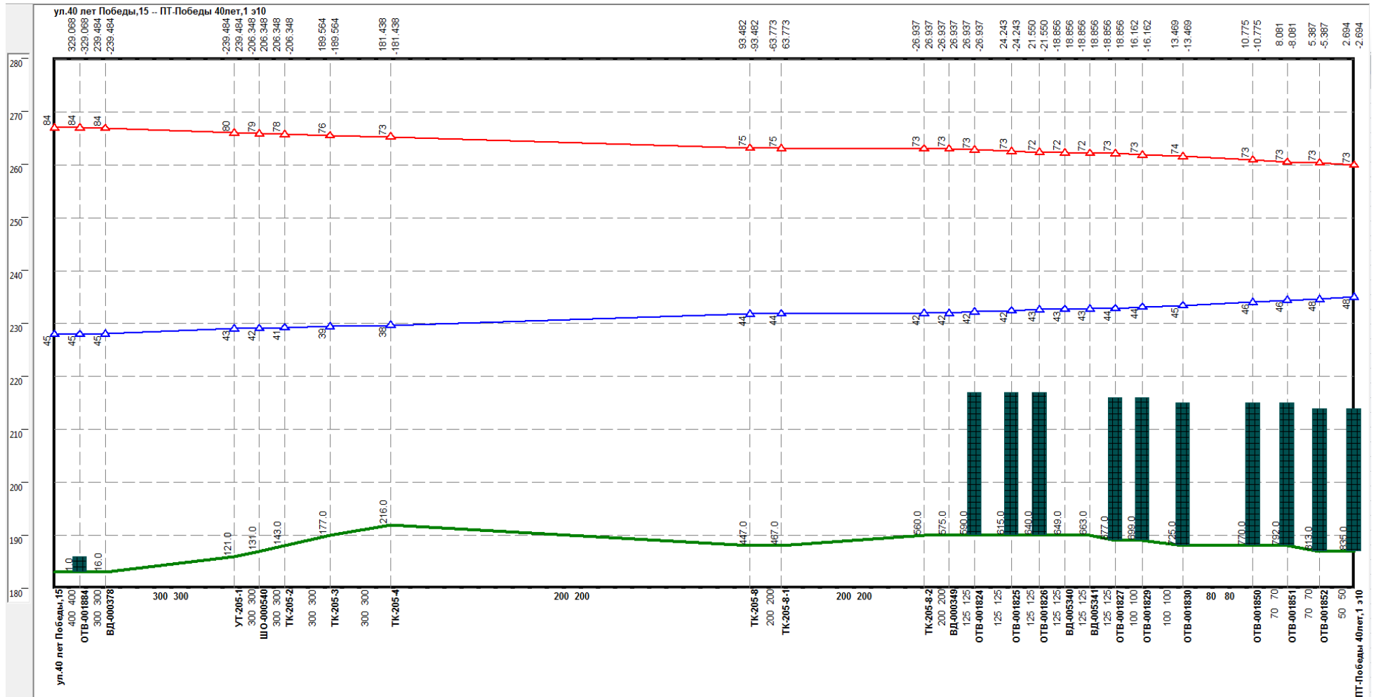
Рисунок Ошибка! Текст указанного стиля в документе отсутствует...204 –Результат гидравлического расчета - график гидравлических режимов по пути теплоносителя от котельной 40 лет Победы, д.15 до ПТ-Победы 40лет,1 э10
