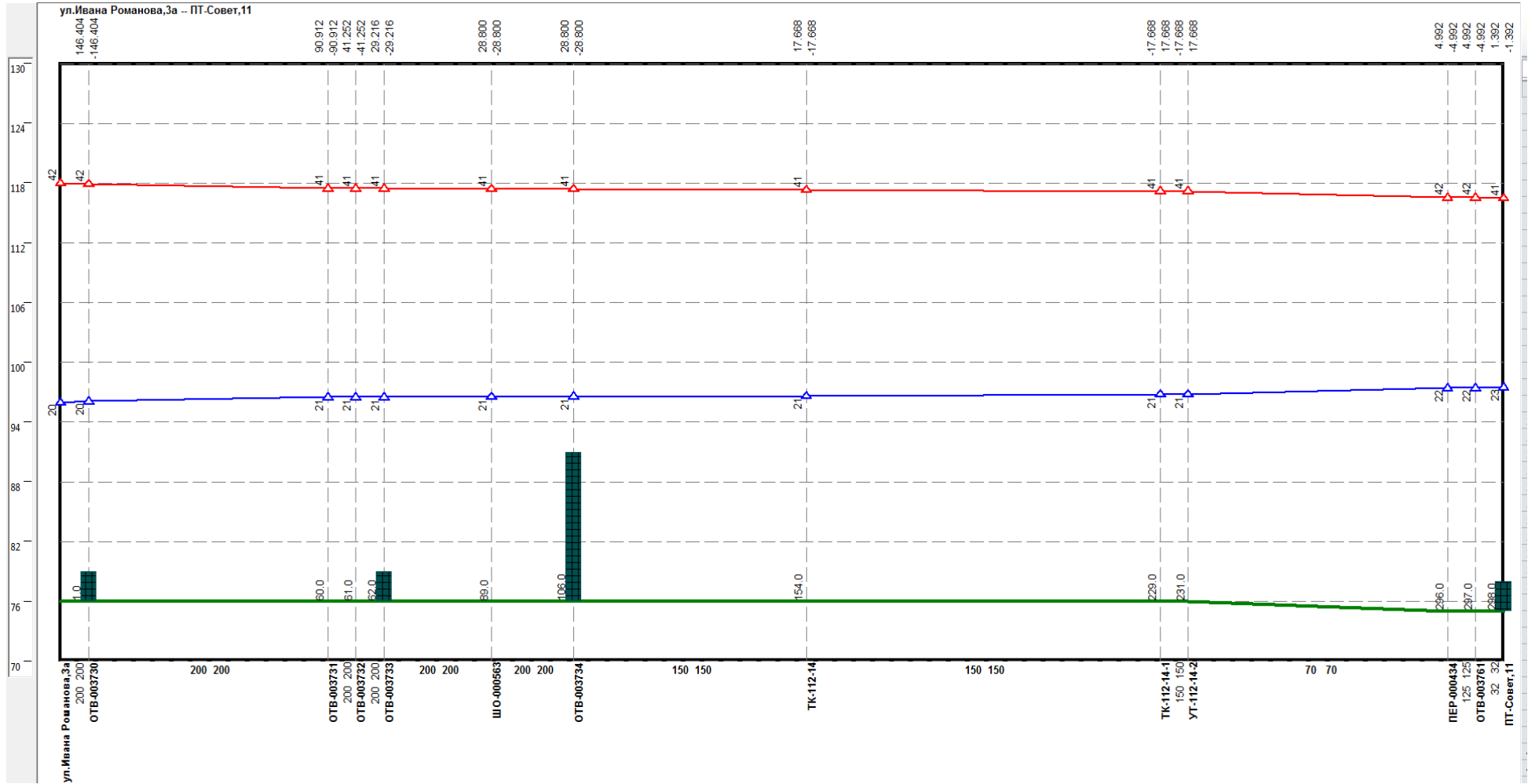
Рисунок 1.144 –Результат гидравлического расчета - график гидравлических режимов по пути теплоносителя от котельной Ивана Романова до ПТ-Совет,11
