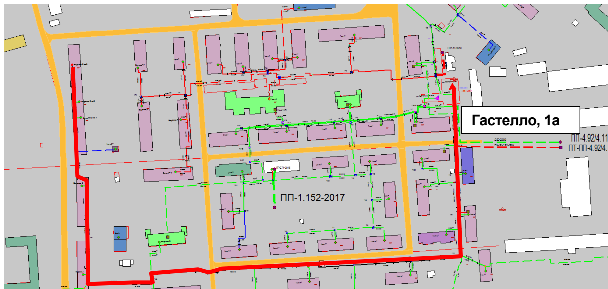
Рисунок Ошибка! Текст указанного стиля в документе отсутствует..151 – Результат гидравлического расчета - расчетный путь теплоносителя от котельной Гастелло, д. 1а до ПТ-Березов,5 вв3
