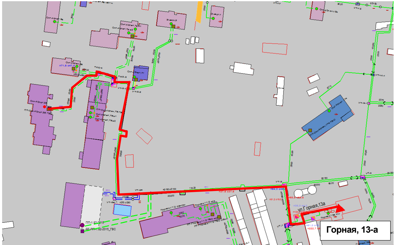
Рисунок Ошибка! Текст указанного стиля в документе отсутствует..181 – Результат гидравлического расчета - расчетный путь теплоносителя 2 от котельной Горная, 13-а до ПТ-Окт.40лет,56
