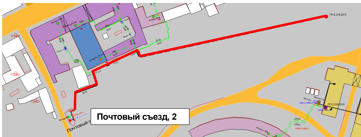
Рисунок Ошибка! Текст указанного стиля в документе отсутствует..207 – Результат гидравлического расчета - расчетный путь теплоносителя от котельной Почтовый съезд, 2, 24 до ПТ-ПП-2.216-2015
