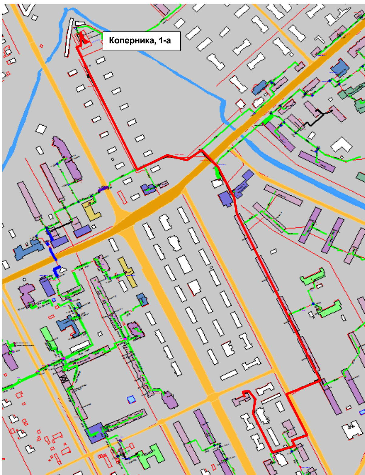
Рисунок Ошибка! Текст указанного стиля в документе отсутствует..217 – Результат гидравлического расчета - расчетный путь теплоносителя от котельной Коперника, 1-а до ПТ-Циол,32
