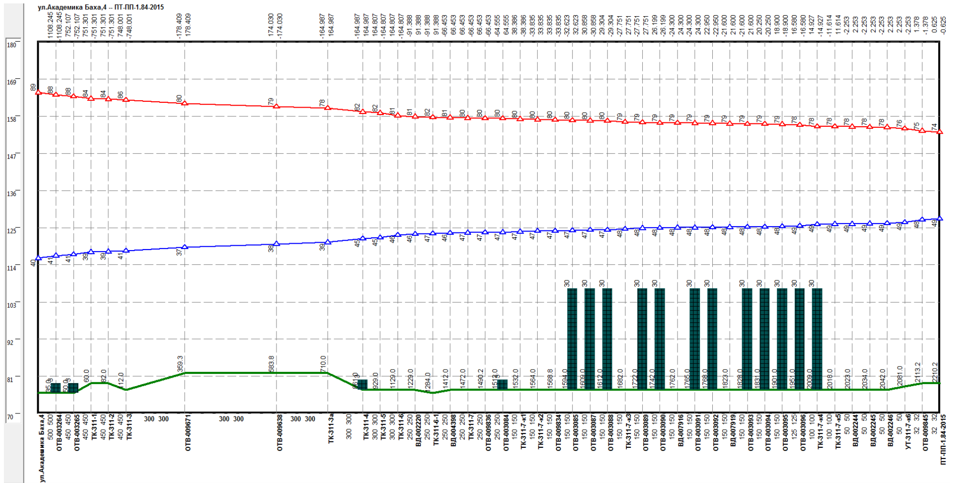
Рисунок Ошибка! Текст указанного стиля в документе отсутствует..206 –Результат гидравлического расчета - график гидравлических режимов по пути теплоносителя от котельной Академика Баха, 4-а до ПТ-ПП-1.84-2015
