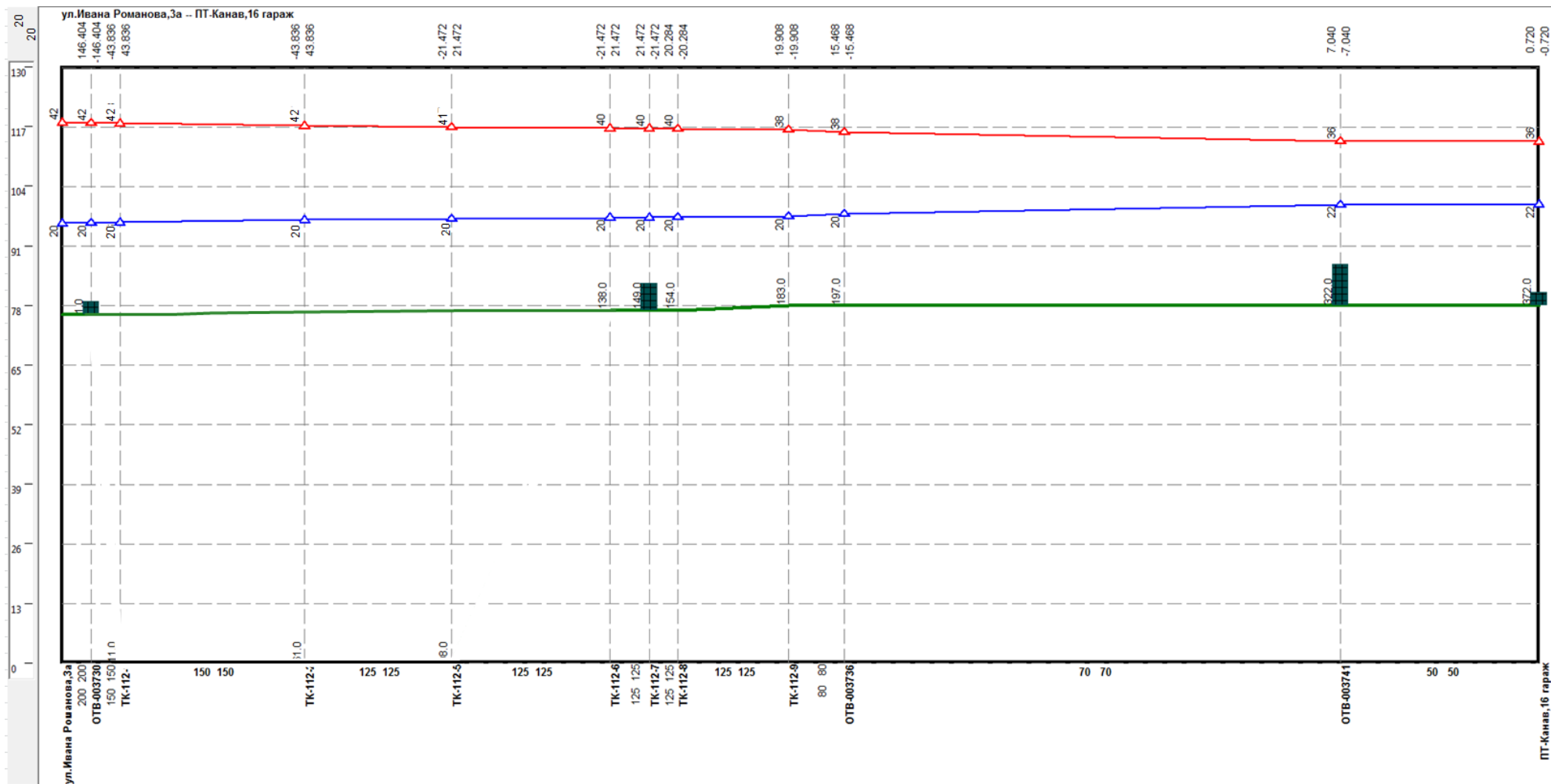
Рисунок Ошибка! Текст указанного стиля в документе отсутствует..146 –Результат гидравлического расчета - график гидравлических режимов по пути теплоносителя от котельной Ивана Романова, 3а до ПТ-Канав, 16 гараж
