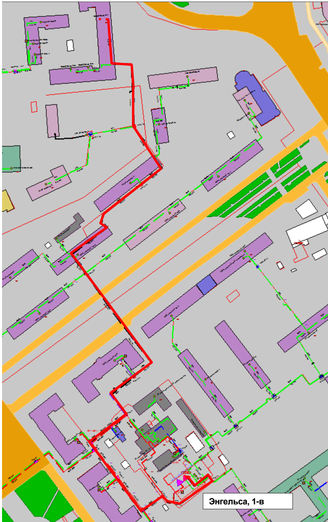
Рисунок Ошибка! Текст указанного стиля в документе отсутствует..195 – Результат гидравлического расчета - расчетный путь теплоносителя от котельной Энгельса, 1-в до ПТ-Ефрем,2 з1
