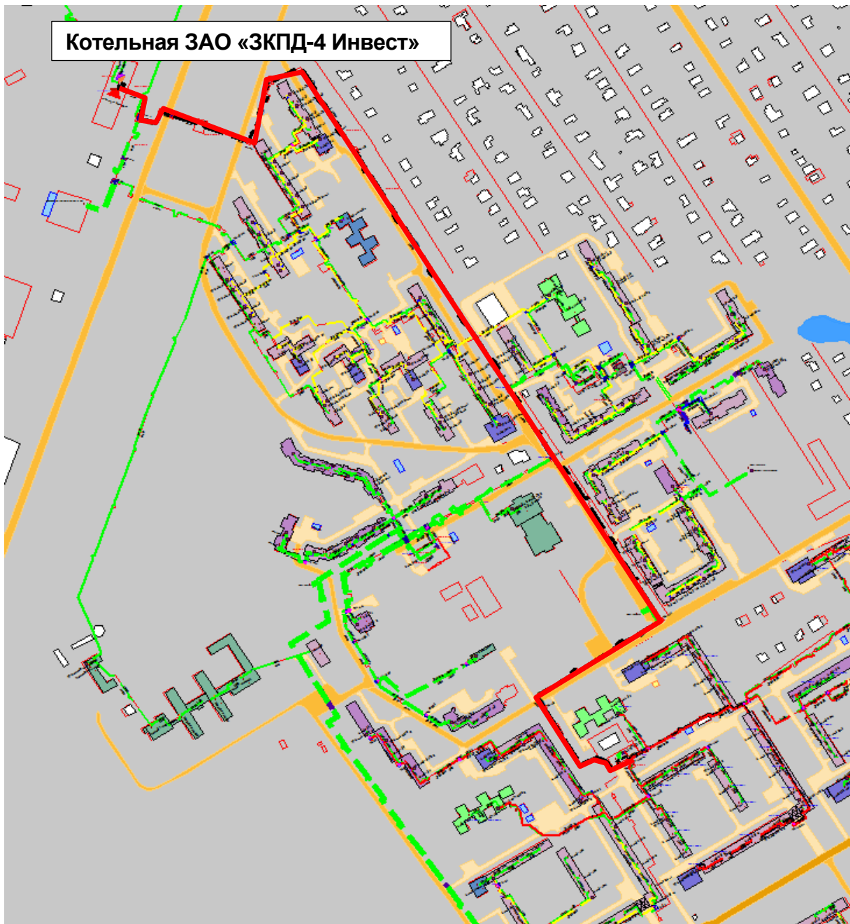
Рисунок Ошибка! Текст указанного стиля в документе отсутствует. 149- Результат гидравлического расчета - расчетный путь теплоносителя от котельной ЗАО «ЗКПД-4 Инвест» до ПТ-Кораб,26/2 аптека Основные характеристики теплопровода и режимные параметры теплоносителя приведены в таблице 1.117.
