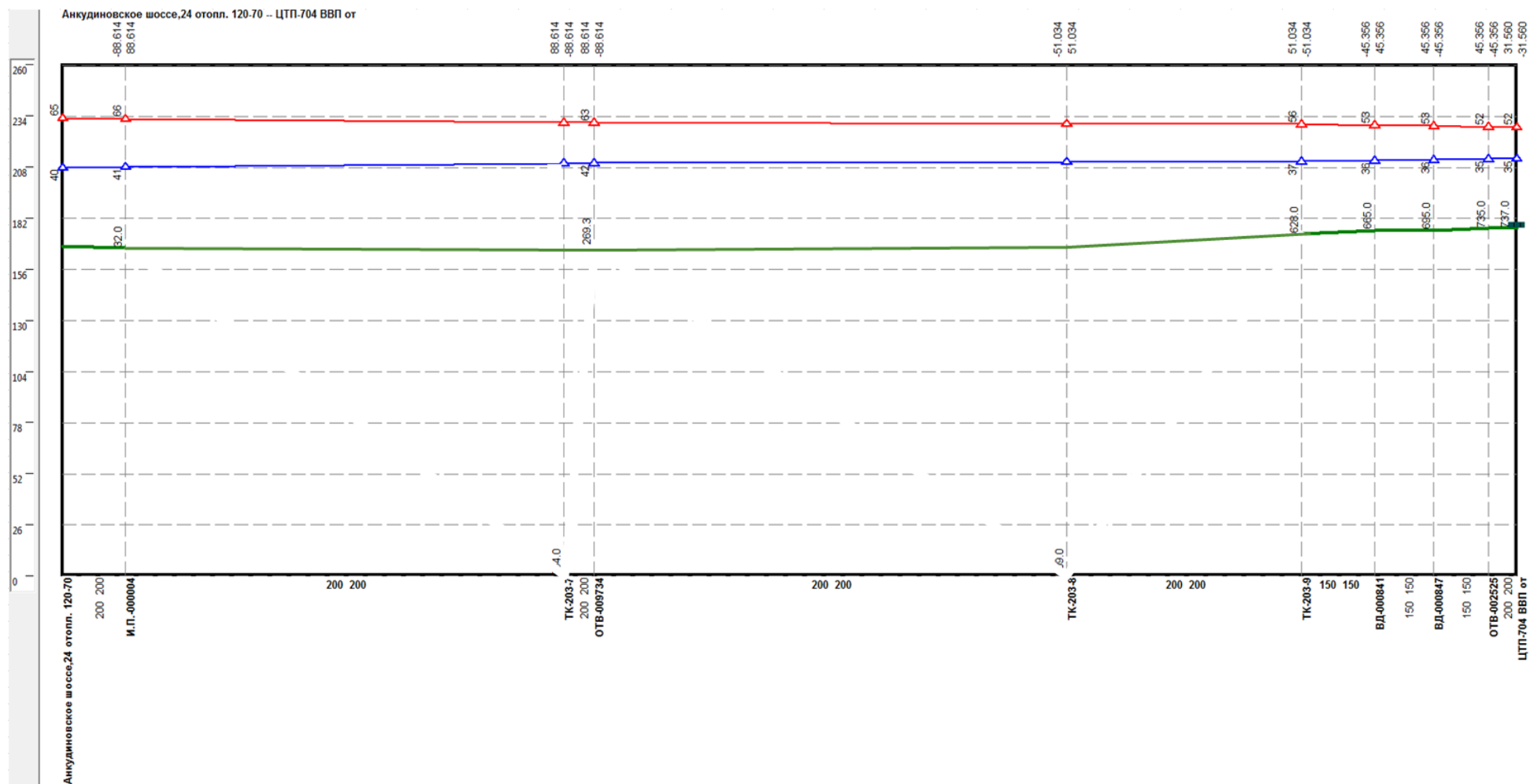
Рисунок Ошибка! Текст указанного стиля в документе отсутствует..194 –Результат гидравлического расчета - график гидравлических режимов по пути теплоносителя от котельной Анкудиновское шоссе, 24 до ЦТП-704 ВВП от
