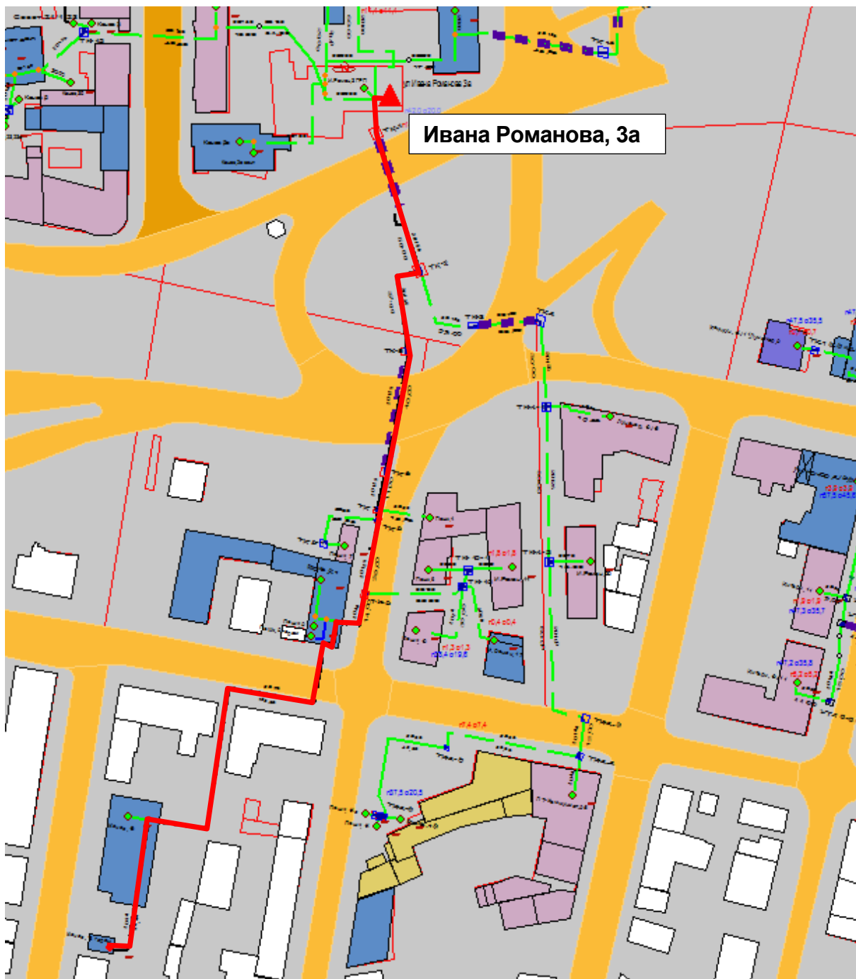
Рисунок 1.145 - Результат гидравлического расчета - расчетный путь теплоносителя от котельной Ивана Романова, 3а до ПТ-Канав,16 гараж
