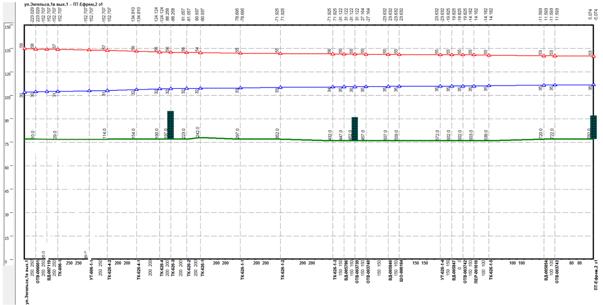
Рисунок Ошибка! Текст указанного стиля в документе отсутствует..196 –Результат гидравлического расчета - график гидравлических режимов по пути теплоносителя от котельной Энгельса, 1-в до ПТ-Ефрем,2 э1
