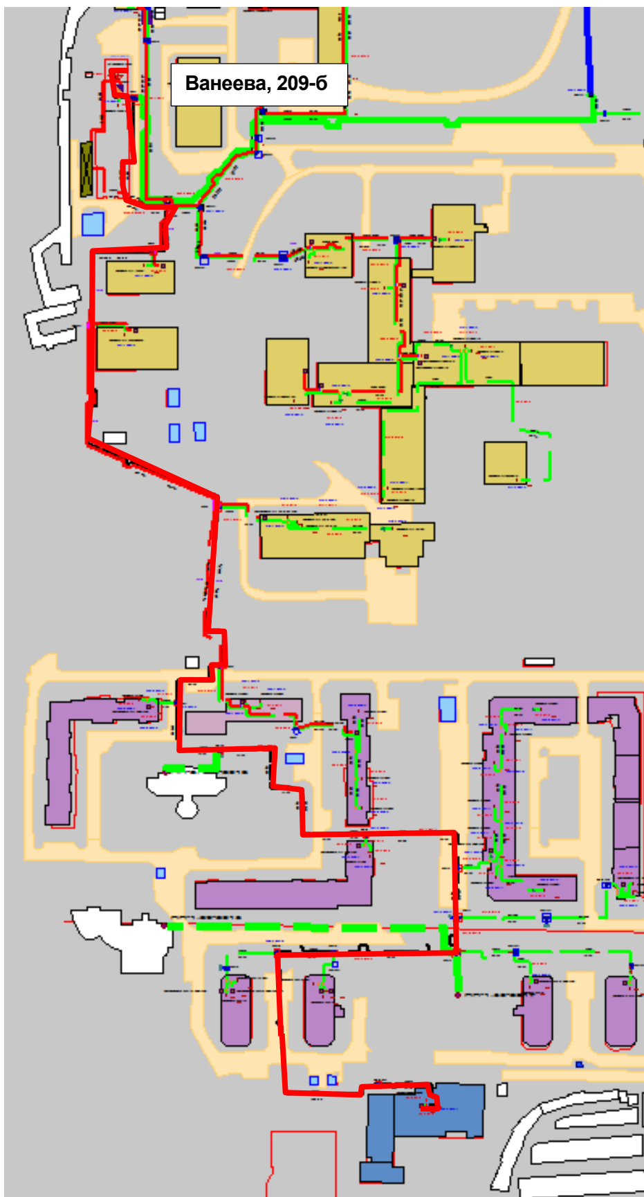
Рисунок Ошибка! Текст указанного стиля в документе отсутствует..175 – Результат гидравлического расчета - расчетный путь теплоносителя от котельной Ванеева, д.209-б до ПТ-Ванеева_Пож.дело
