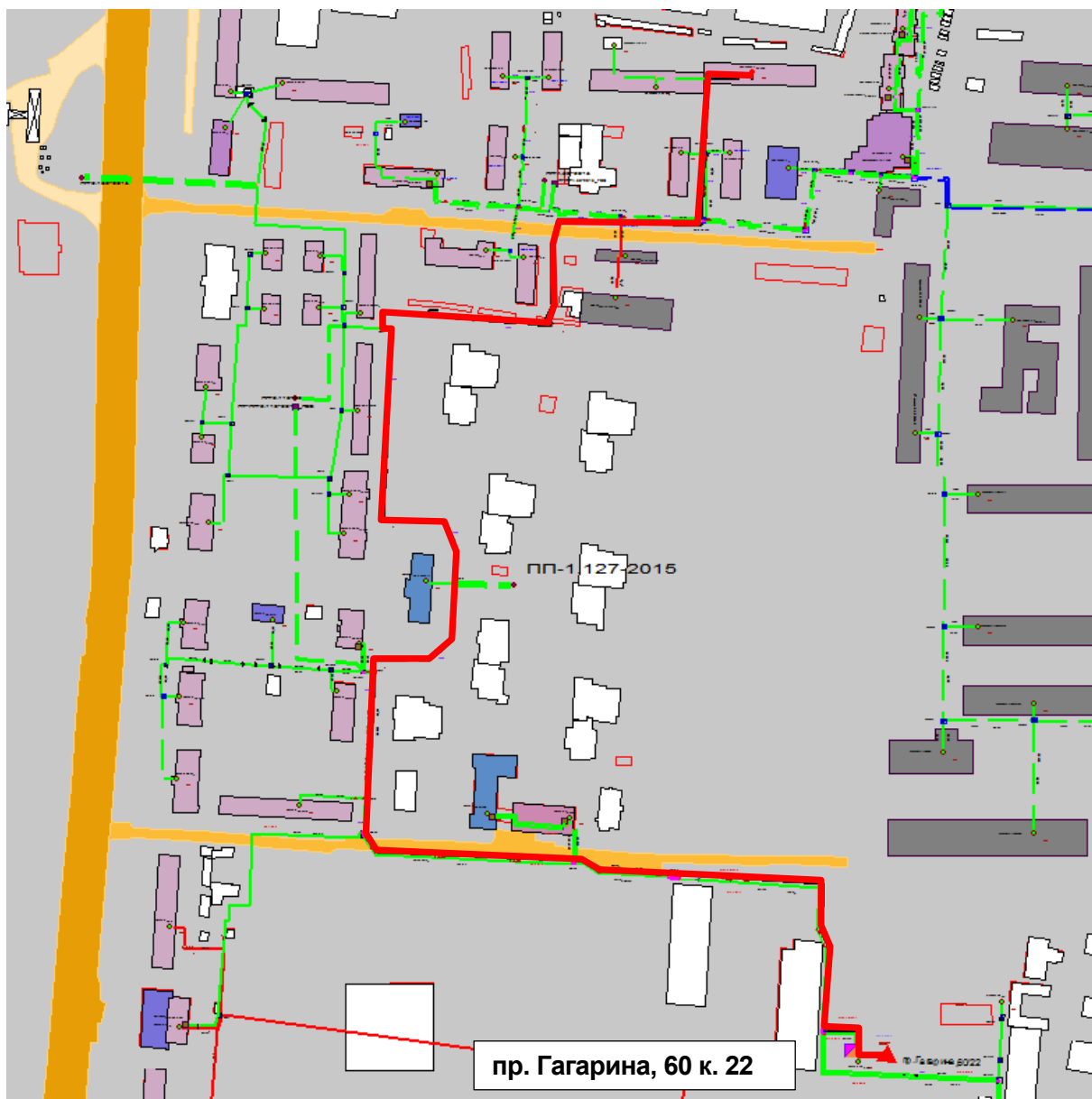
Рисунок Ошибка! Текст указанного стиля в документе отсутствует..171 – Результат гидравлического расчета - расчетный путь теплоносителя от котельной Гагарина, 60 к.22 до ПТ-Краснов,12а вв2
