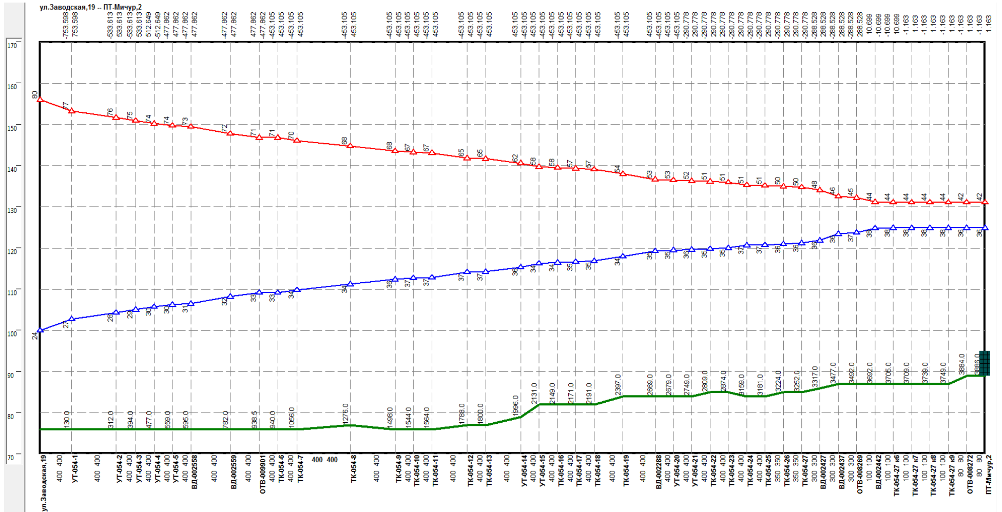
Рисунок Ошибка! Текст указанного стиля в документе отсутствует..166 –Результат гидравлического расчета - график гидравлических режимов по пути теплоносителя от котельной ФГУП НПП «Полет» до ПТ-Мичур.2
