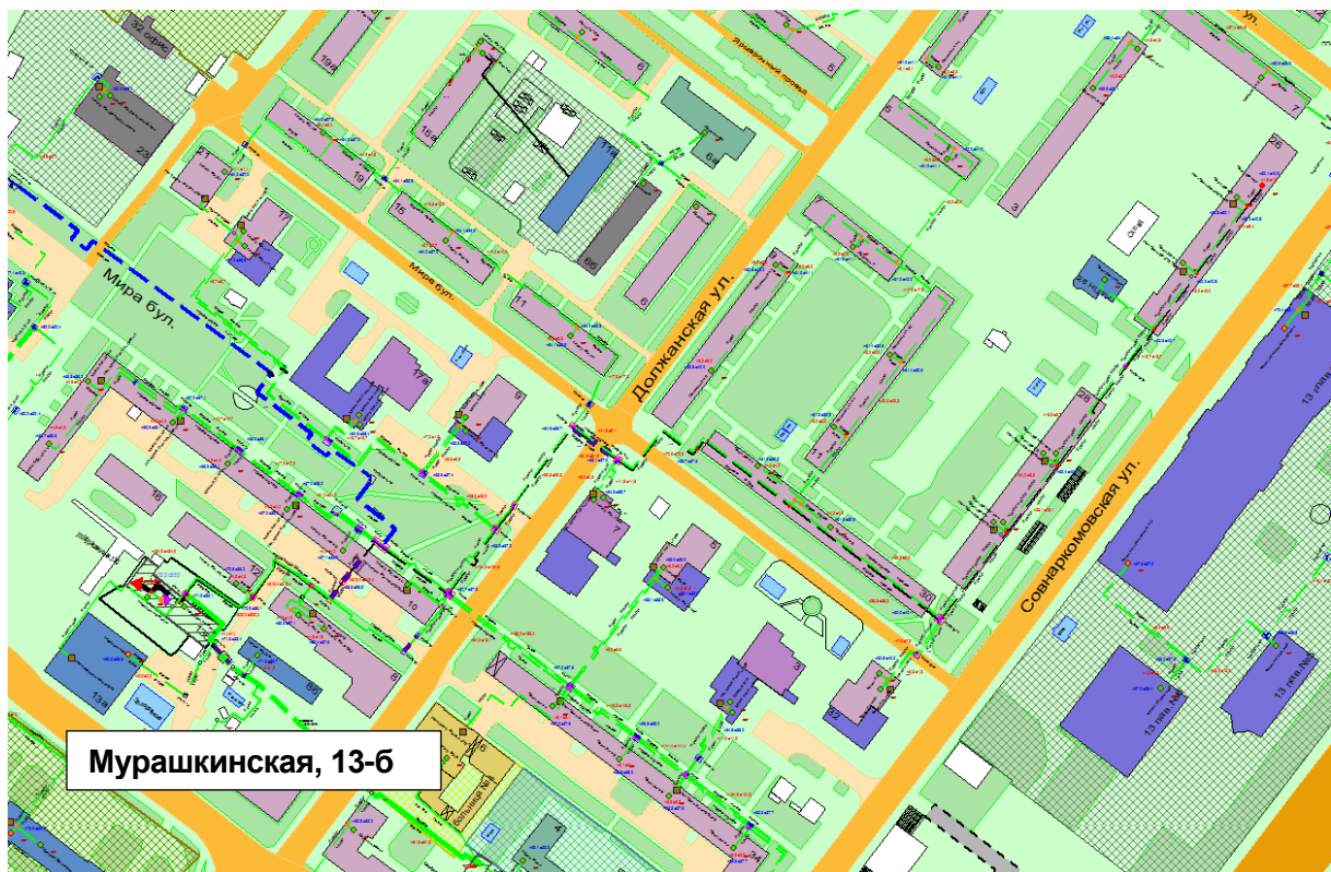
Рисунок Ошибка! Текст указанного стиля в документе отсутствует..151 – Результат гидравлического расчета - расчетный путь теплоносителя от котельной Мурашкинская, 13-б до ПТ-Совн,26 маг
