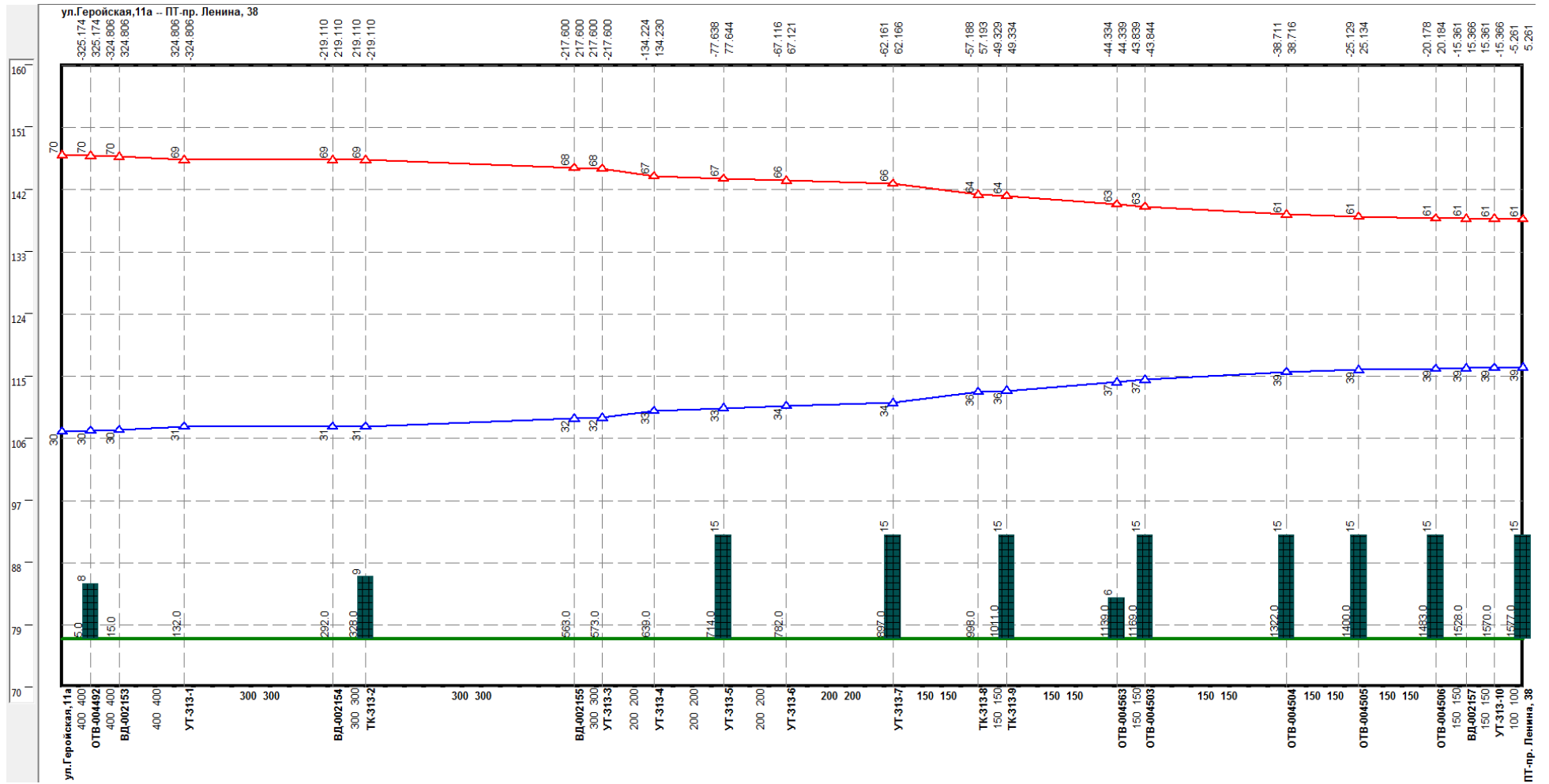
Рисунок Ошибка! Текст указанного стиля в документе отсутствует..162 –Результат гидравлического расчета - график гидравлических режимов по пути теплоносителя от котельной Геройская, 11а до ПТ-пр. Ленина, 38
