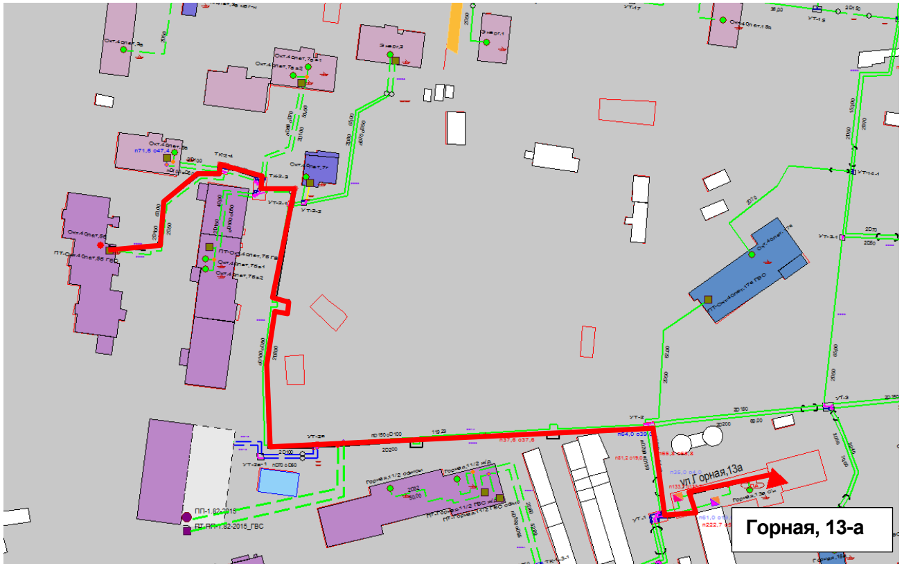
Рисунок Ошибка! Текст указанного стиля в документе отсутствует..179 – Результат гидравлического расчета - расчетный путь теплоносителя 2 от котельной Горная, 13-а до ПТ-Окт.40лет,5б
