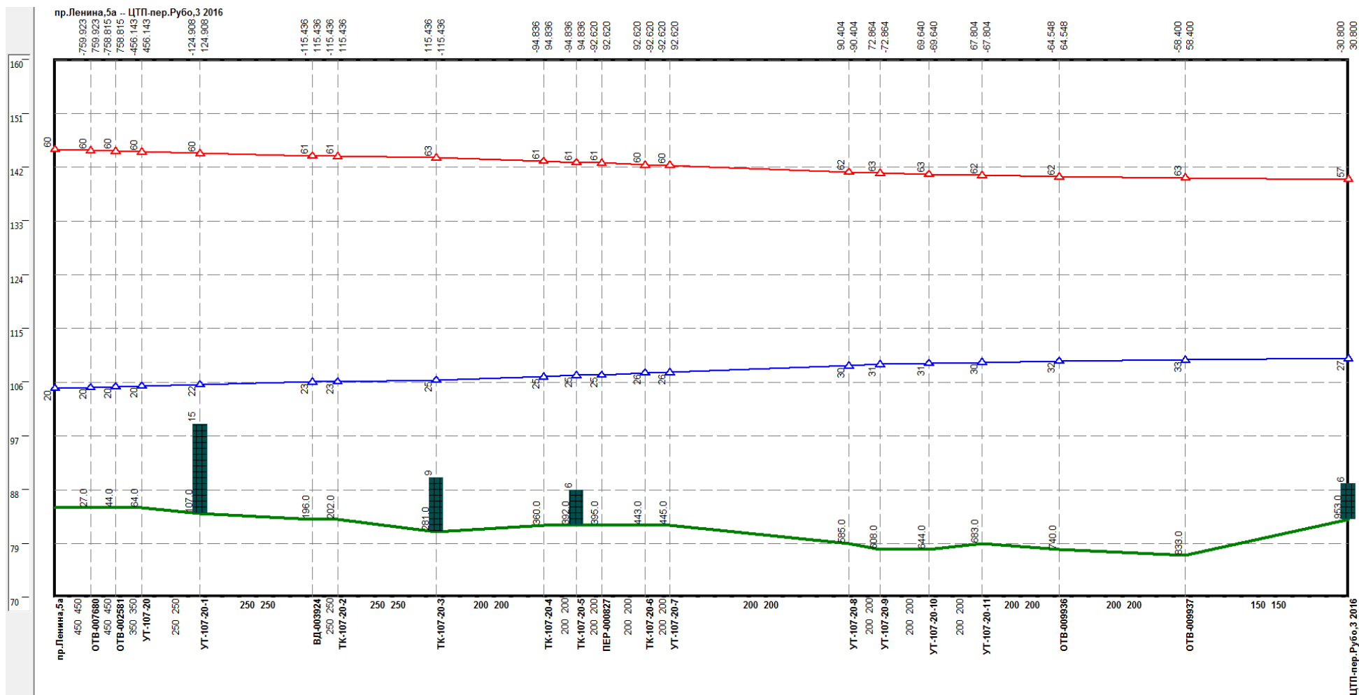
Рисунок Ошибка! Текст указанного стиля в документе отсутствует..190 –Результат гидравлического расчета - график гидравлических режимов по пути теплоносителя от котельной пр. Ленина, 5-а до ЦТП-пер.Рубо,3 2016
