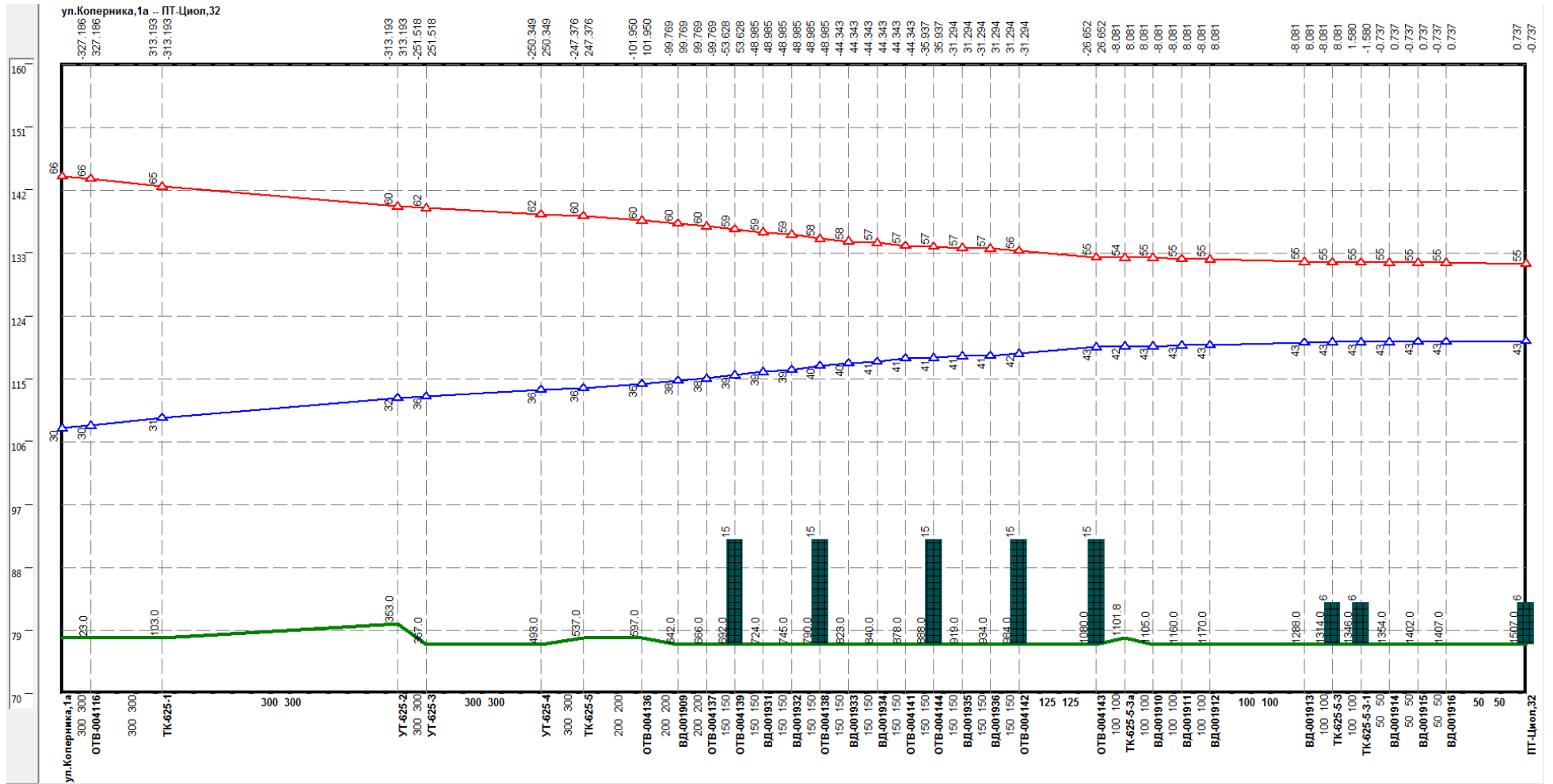
Рисунок Ошибка! Текст указанного стиля в документе отсутствует..218 –Результат гидравлического расчета - график гидравлических режимов по пути теплоносителя от котельной Коперника, 1-а до ПТ-Циол,32
