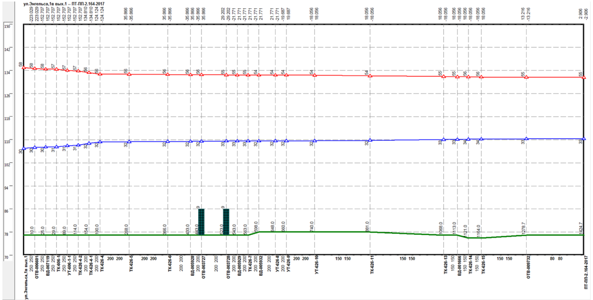
Рисунок Ошибка! Текст указанного стиля в документе отсутствует..198 –Результат гидравлического расчета - график гидравлических режимов по пути теплоносителя от котельной Энгельса, 1-в до ПТ-ПП-2.164.2017
