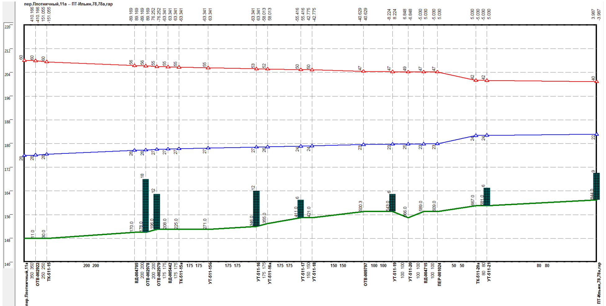
Рисунок Ошибка! Текст указанного стиля в документе отсутствует..182 –Результат гидравлического расчета - график гидравлических режимов по пути теплоносителя от котельной пер. Плотничный, 11 до ПТ-Ильин,78,78а,гар
