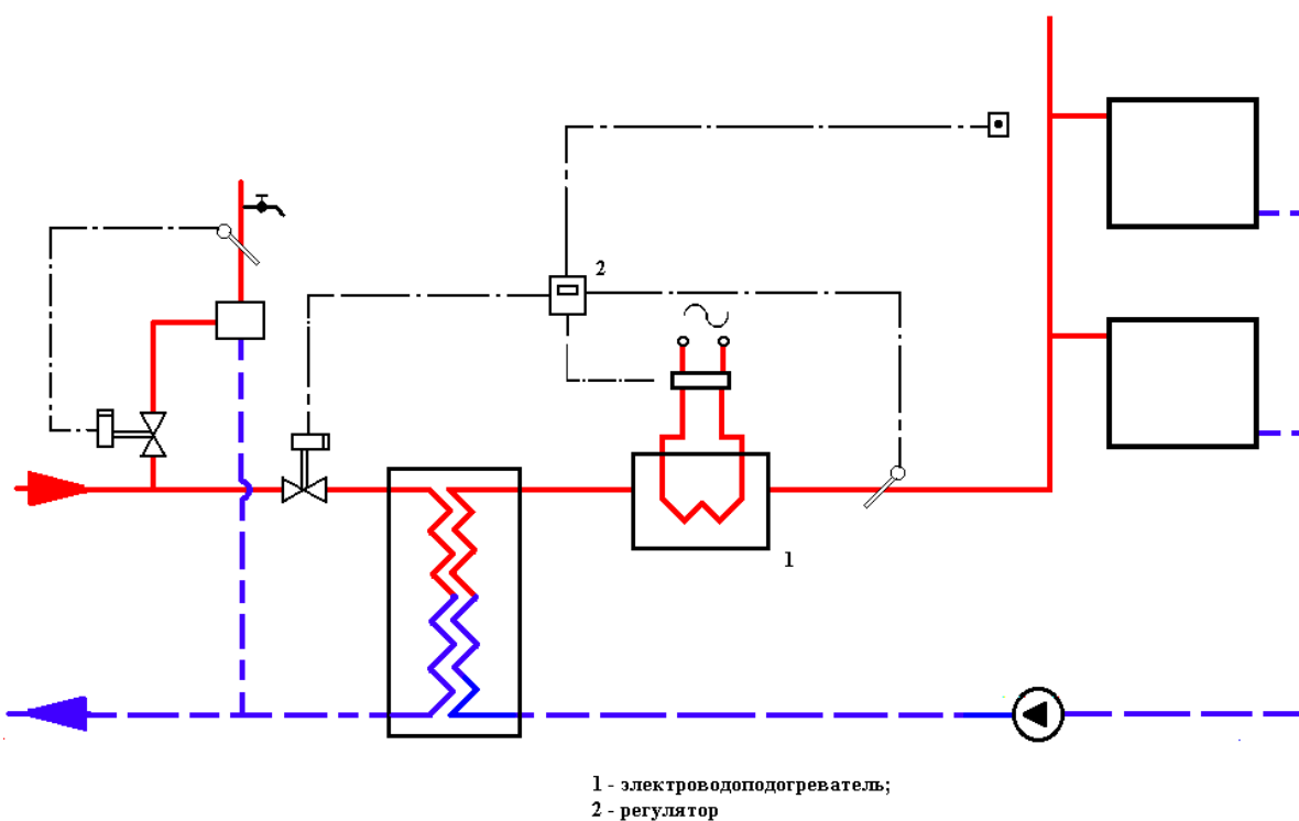
Рисунок 5.2 – – Схема теплового пункта с электроводоподогревателем
